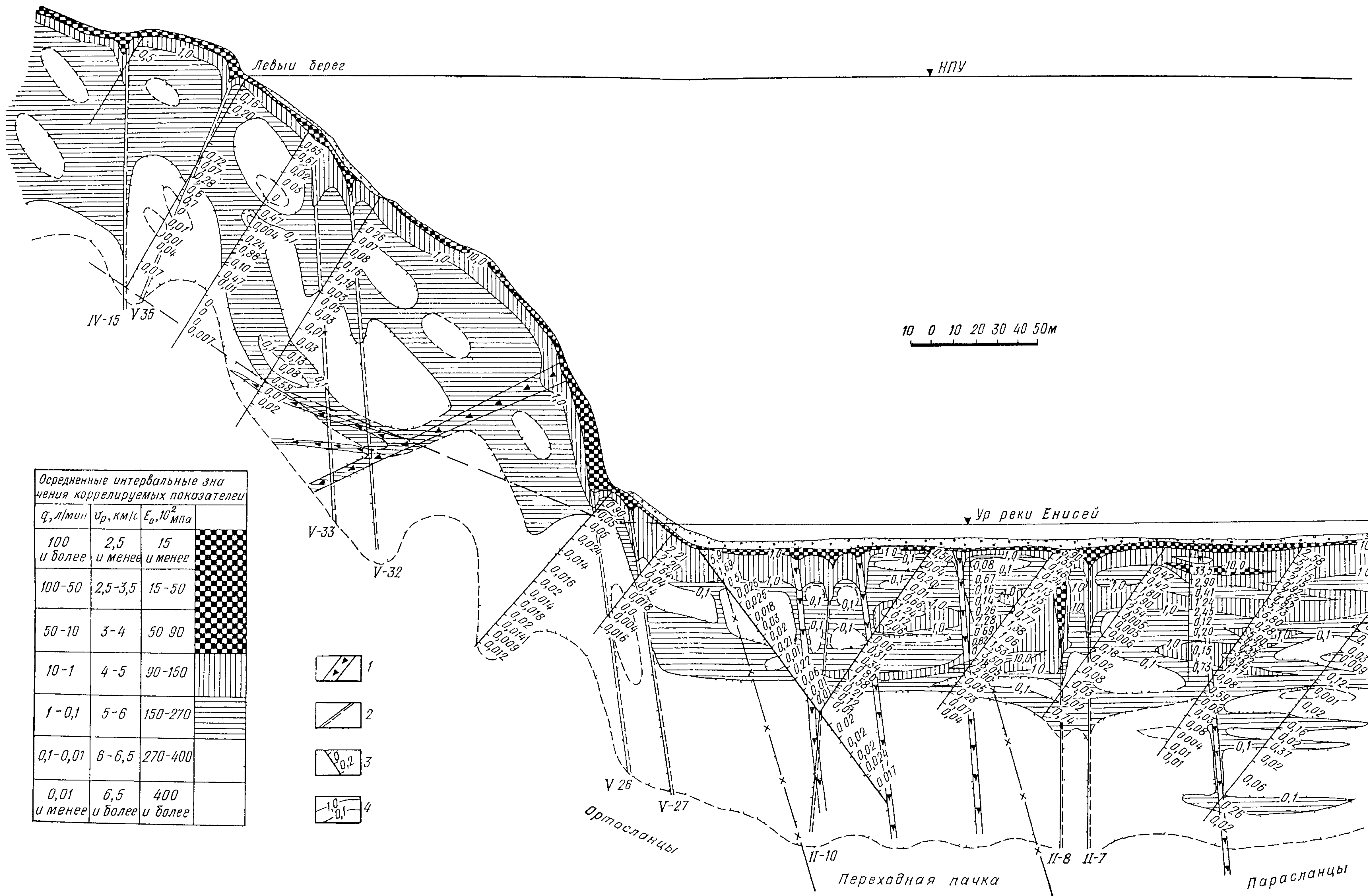
Рис. 3.9. Фрагмент уточненной модели водопроницаемости естественного скального массива. Разрез I—I по хорде арочно-гравитационной плотины Саяно-Шушенской ГЭС. 1 — дайки диоритов; 2 — тектонические нарушения и их номера; 3 — интервальные значения q (л/мин); 4 —
