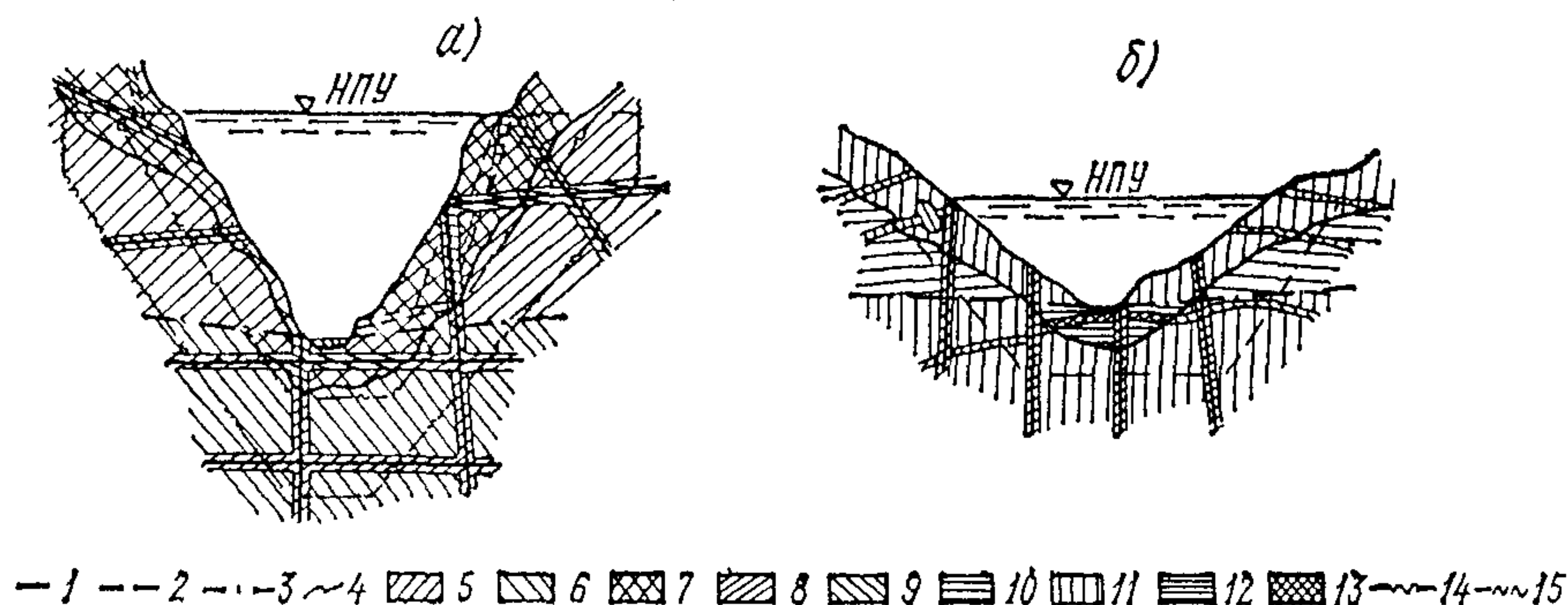
Рис. 16. Фрагменты моделей водопроницаемости
