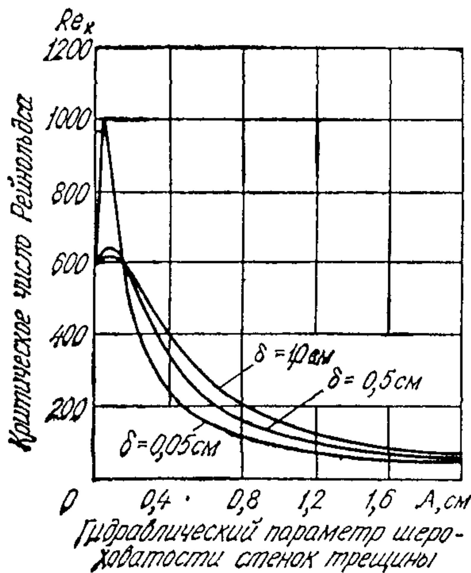
Рис 1-2 Графики изменения критического числа Рейнольдса потока воды в трещине в зависимости от гидравлического параметра шероховатости ее стенок (при t_b = 20^\circ\text{C} ) (по В. Н. Жиленкову)
