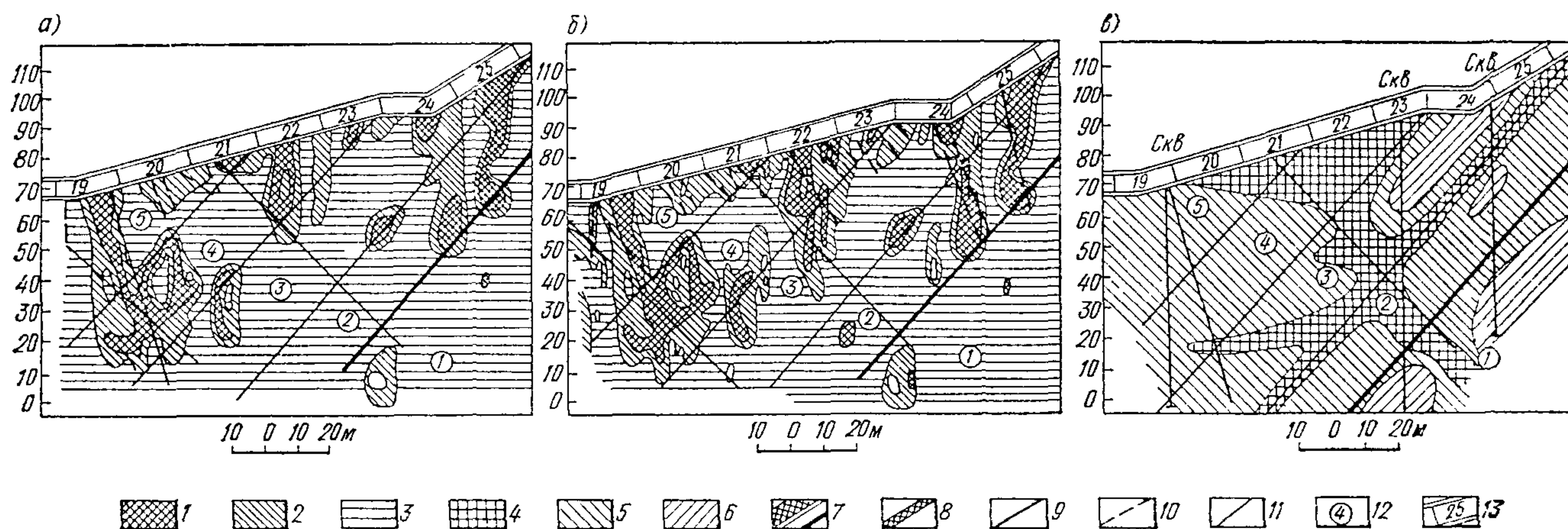
Рис. 3-7 Фрагменты схемы водопроницаемости основания Чарвакского гидроузла
