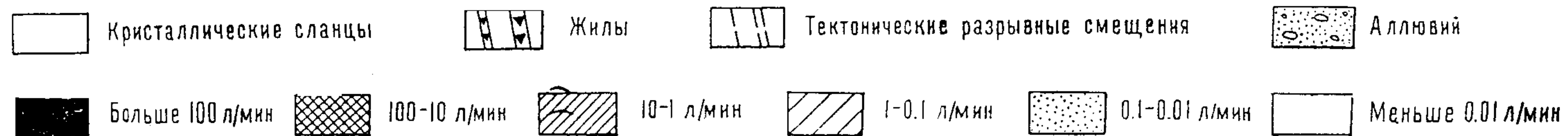
Рис. 3-10. Разрез основания Саяно-Шушенской ГЭС по водопроницаемости (подрусловая часть массива, разрез по долине р. Енисей).
