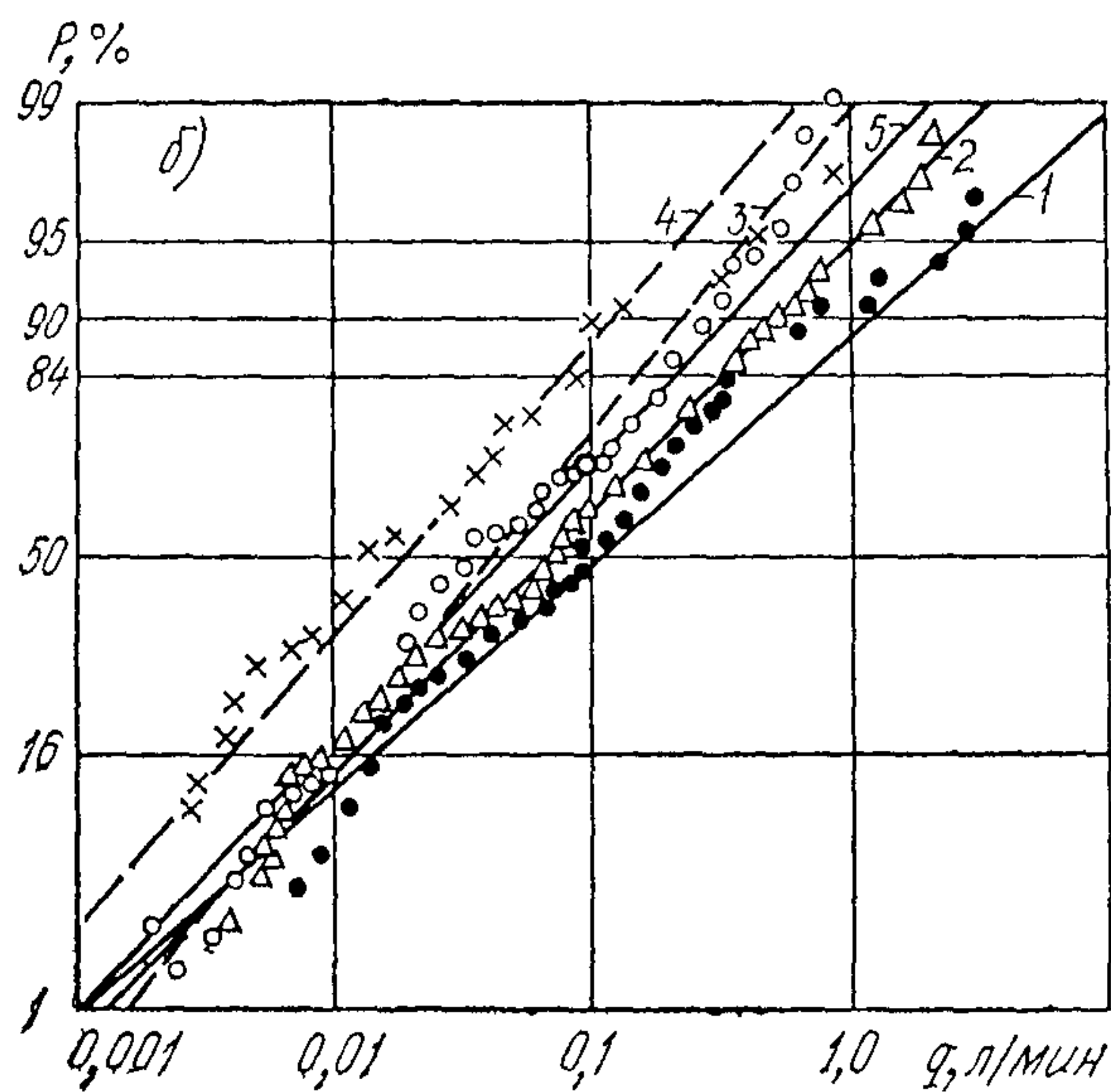
Рис. 17. Примеры распределения значений q на вероятностной (а) и логарифмически-вероятностной (б) бумаге:
