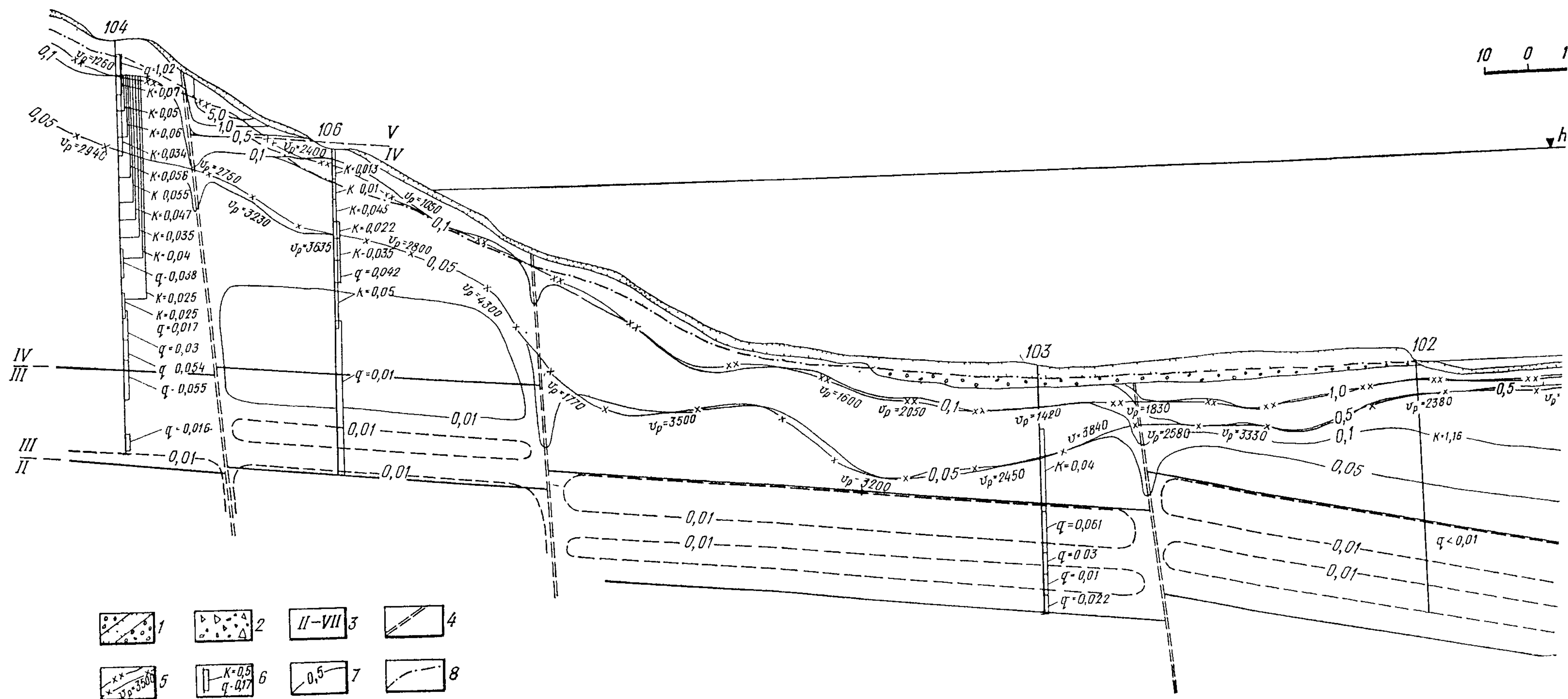
Рис 29 Фрагмент модели водопроницаемости массива основ
