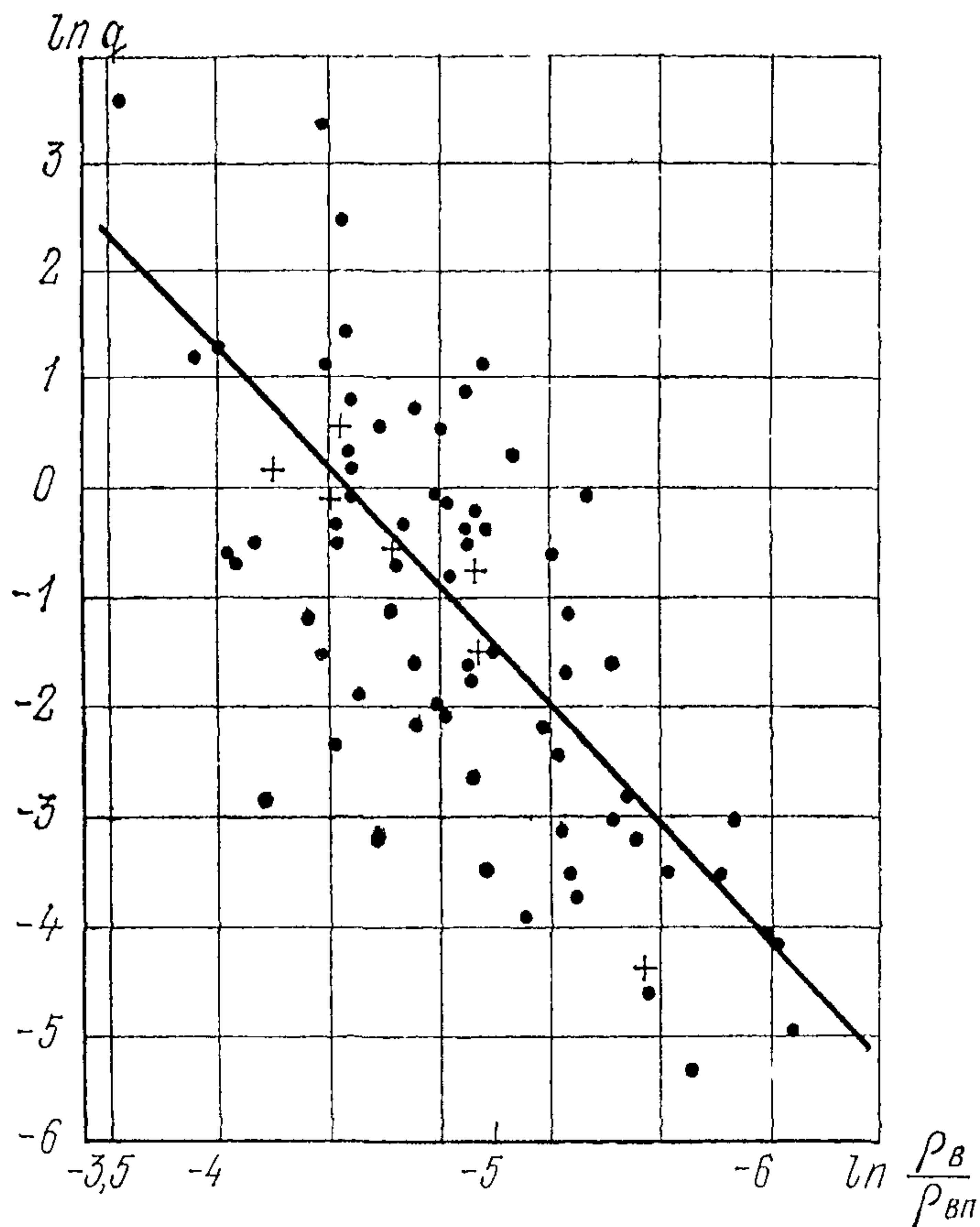
Рис 2.2 Связь q с обратной величиной относительного элект- рического сопротивления ( \rho_{vp}/\rho_v ) в массиве диоритов осно- вания Зейской ГЭС
