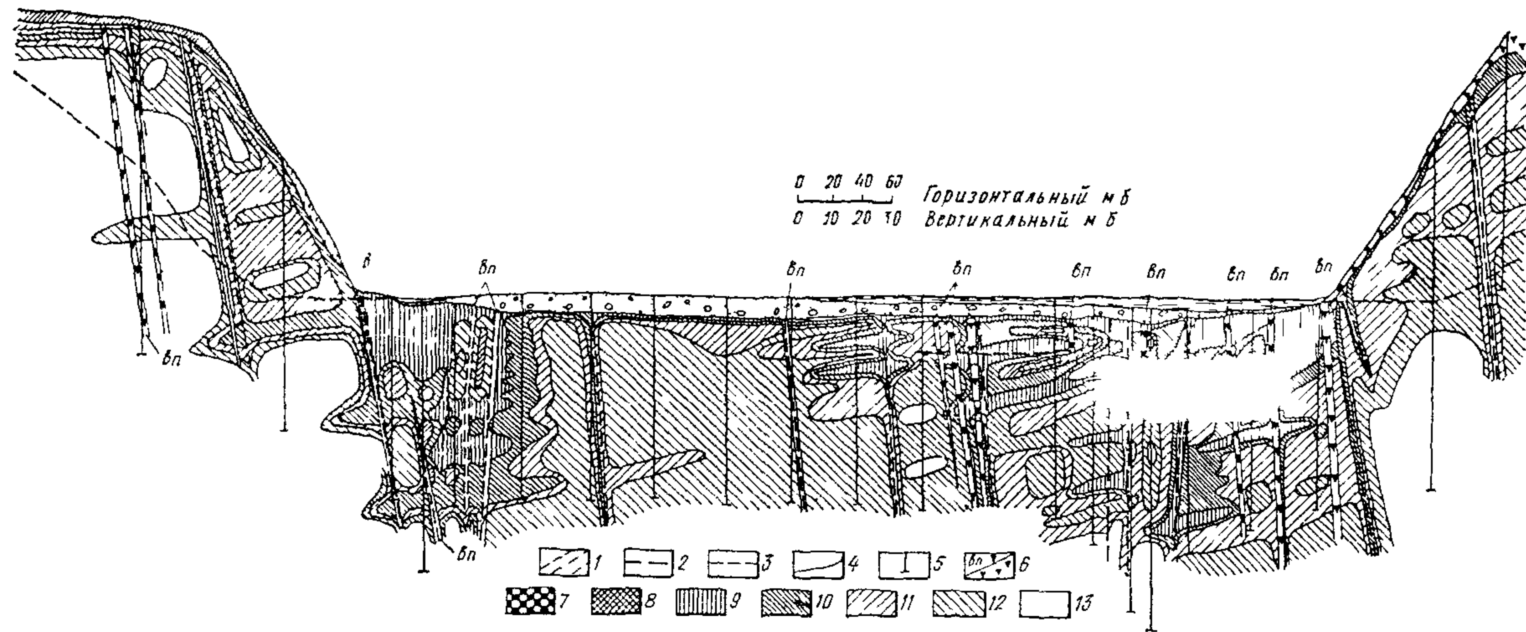
Рис 30 Фрагмент модели водопроницаемости скального основания Красноярской ГЭС
