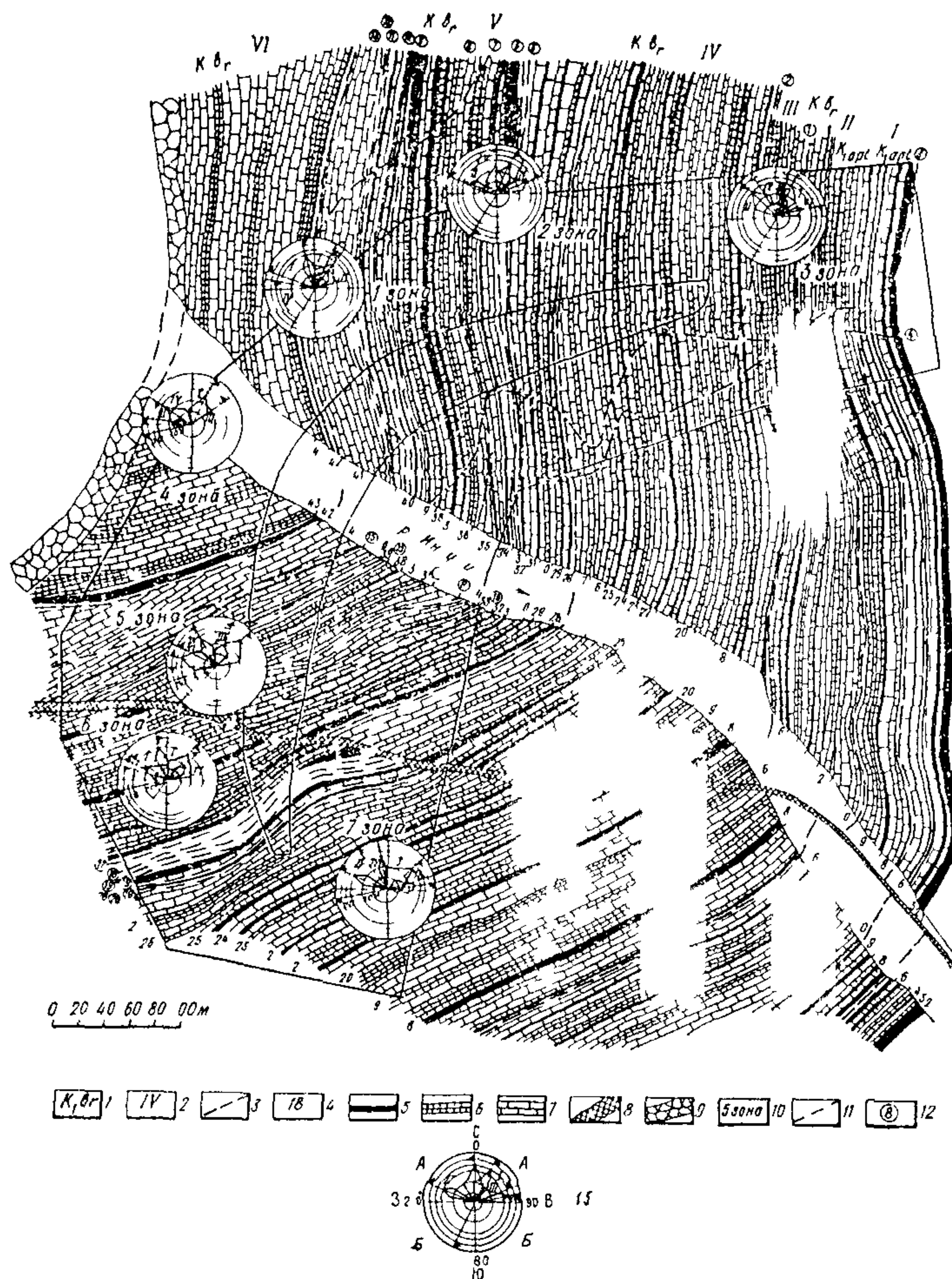
Рис 21 Геоструктурная схема участка плотины Ингури ГЭС
