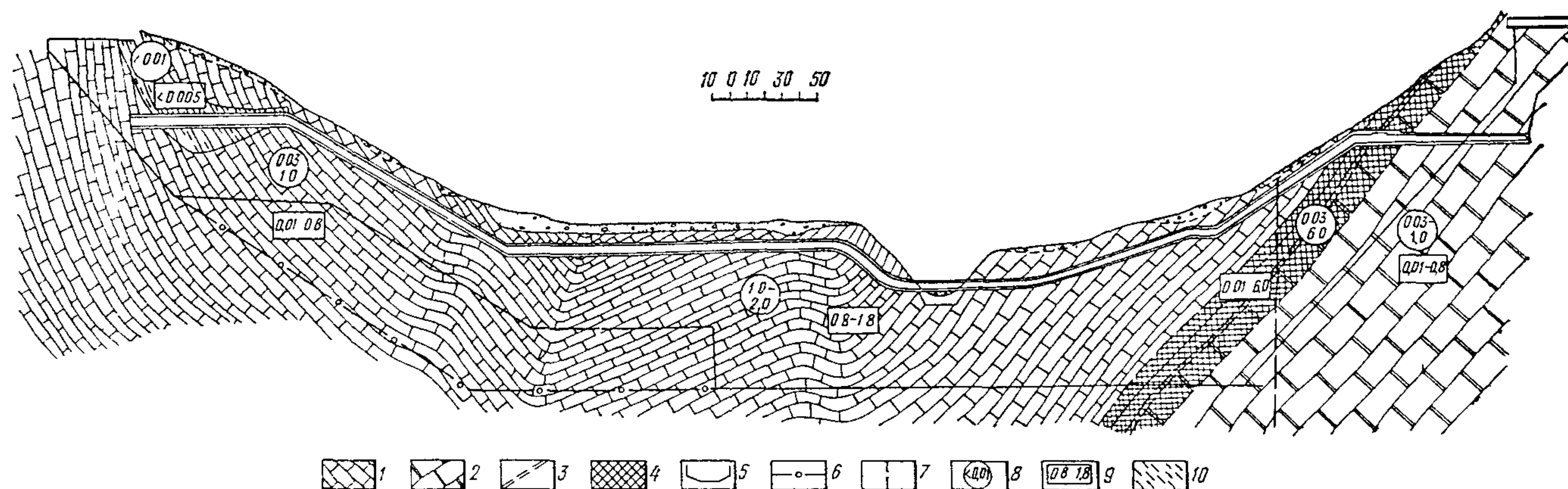
Рис 3-2 Гидрогеологический разрез основания Чарвакского гидроузла (по В В Каякину)
