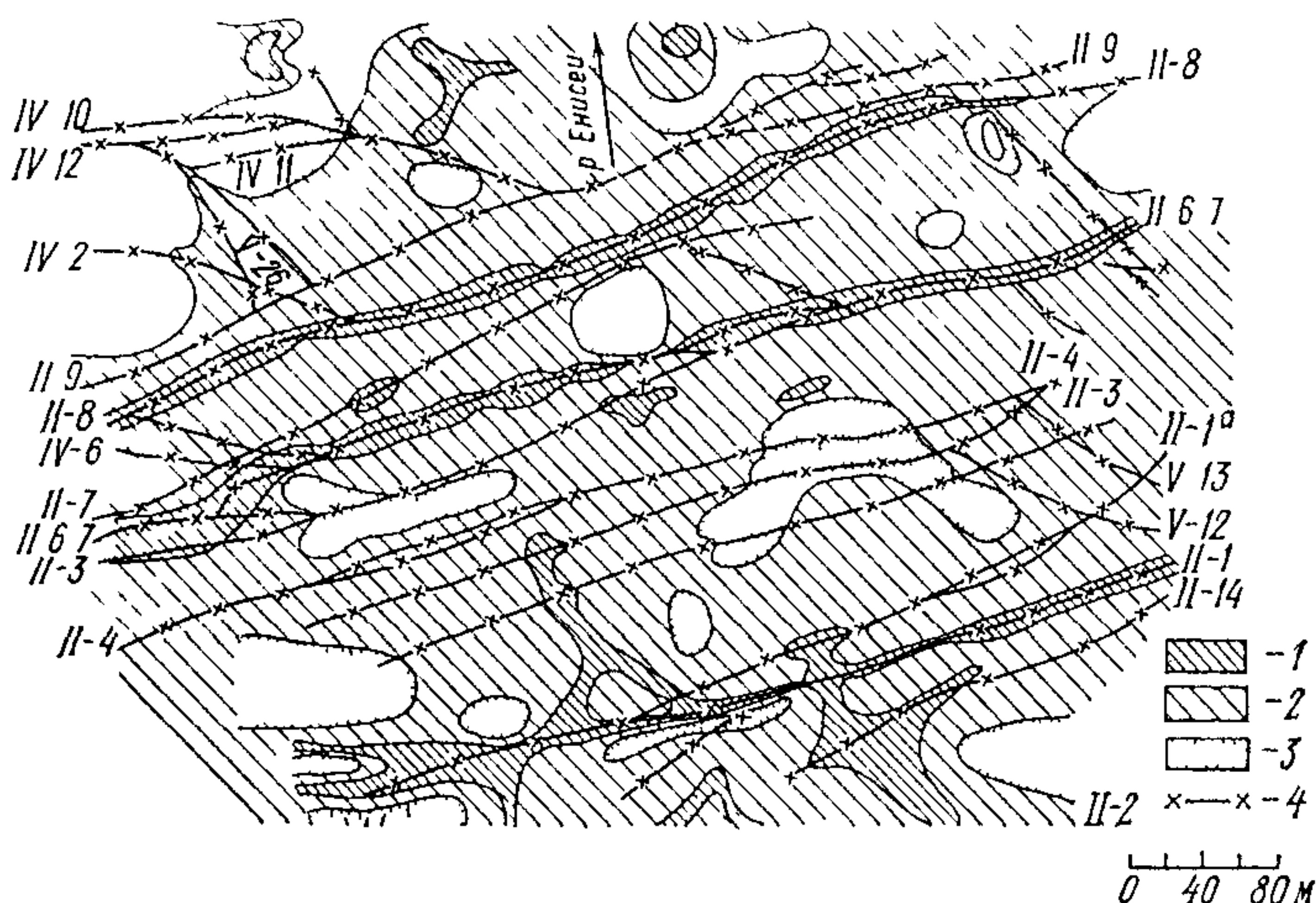
Рис 2-3 Схема водопроницаемости основания плотины Саяно-Шушенской ГЭС, построенная по данным сейсморазведки. Срез отвечает отметкам массива ниже зоны поверхностного выветривания и разуплотнения
