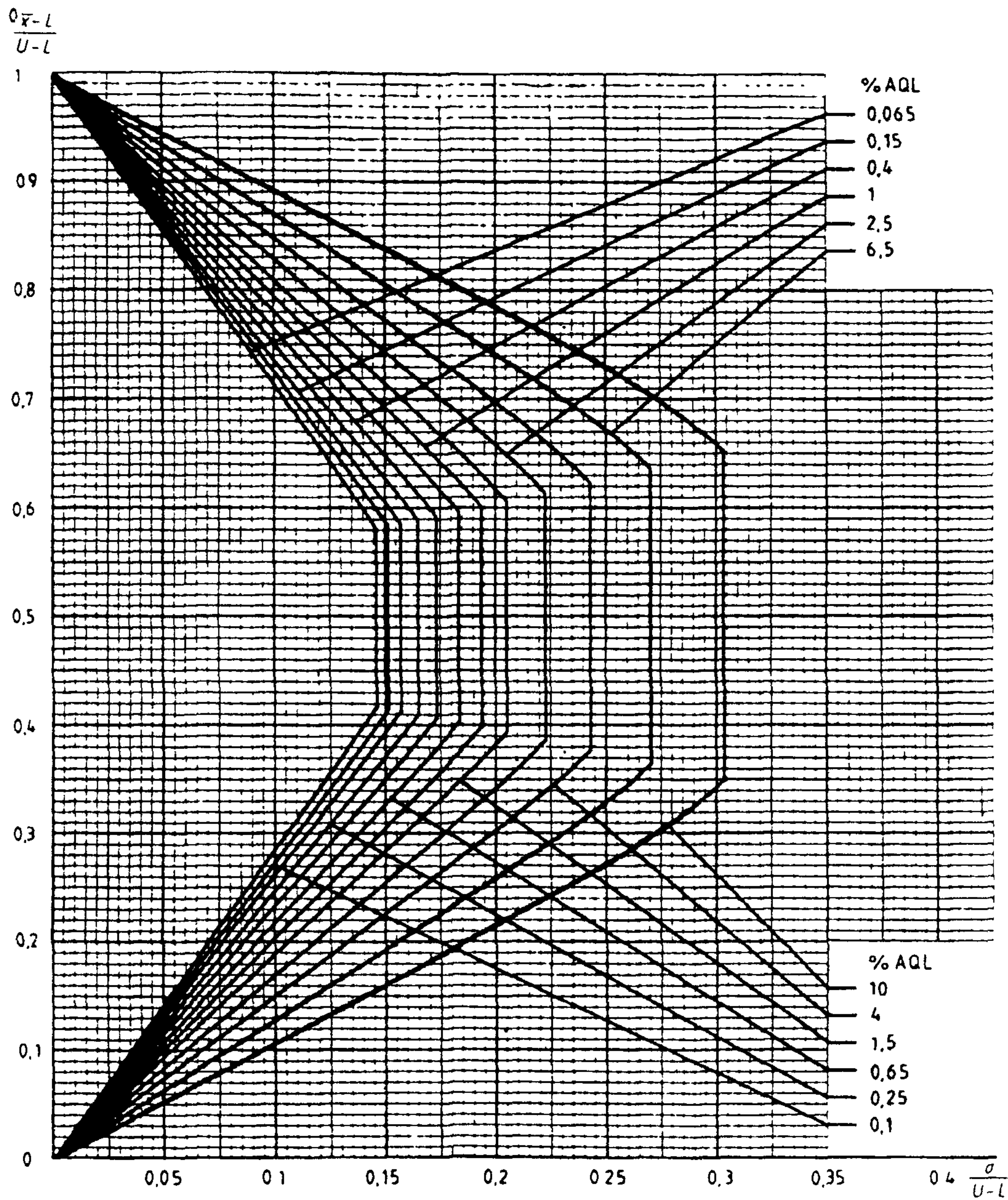
Диаграмма \sigma -P — Кривые приемки для предельных значений с общим уровнем качества: \sigma -метод для кода объема выборки P
