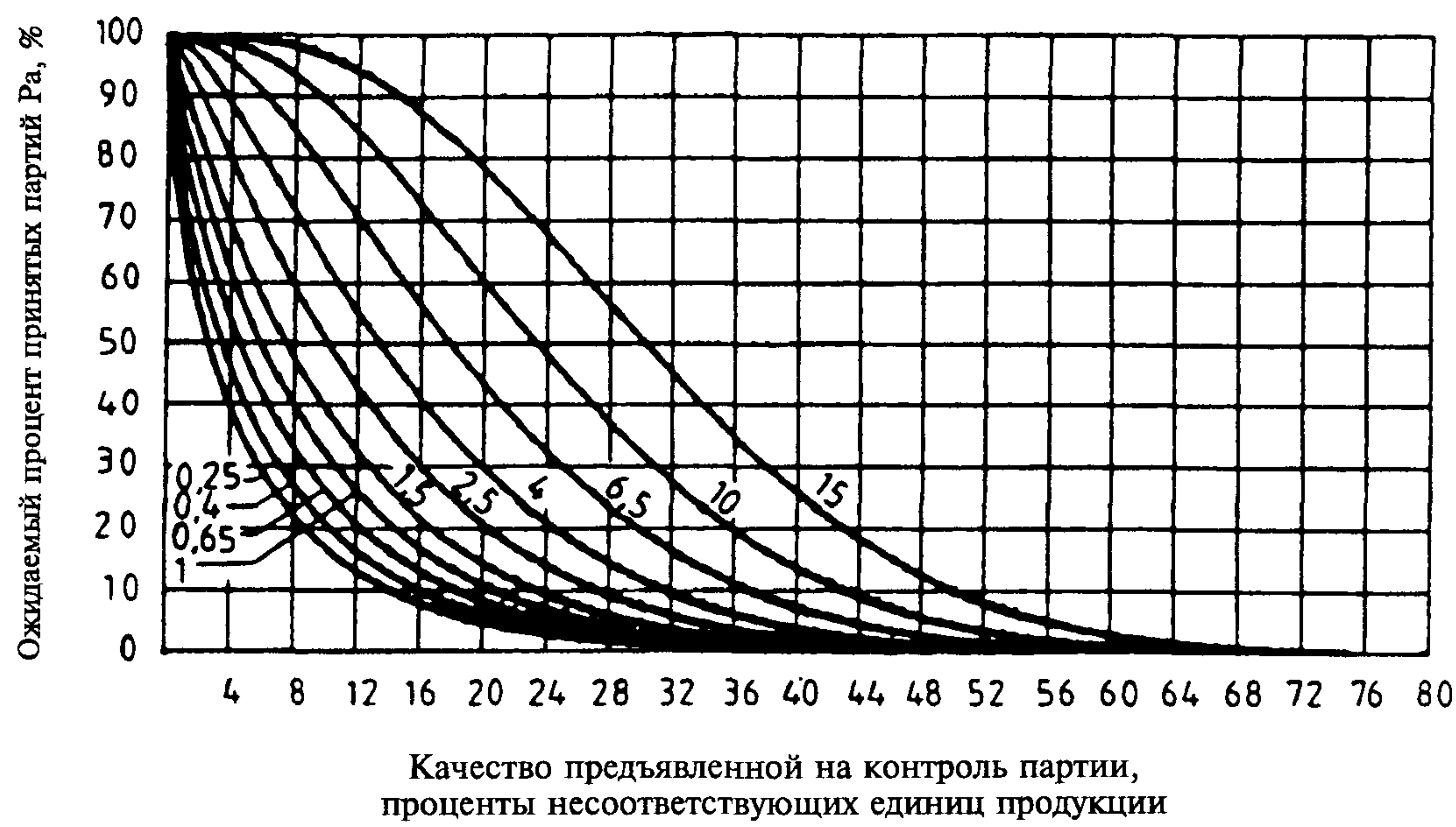
График VE — Оперативные характеристики для одноступенчатых выборочных планов контроля
