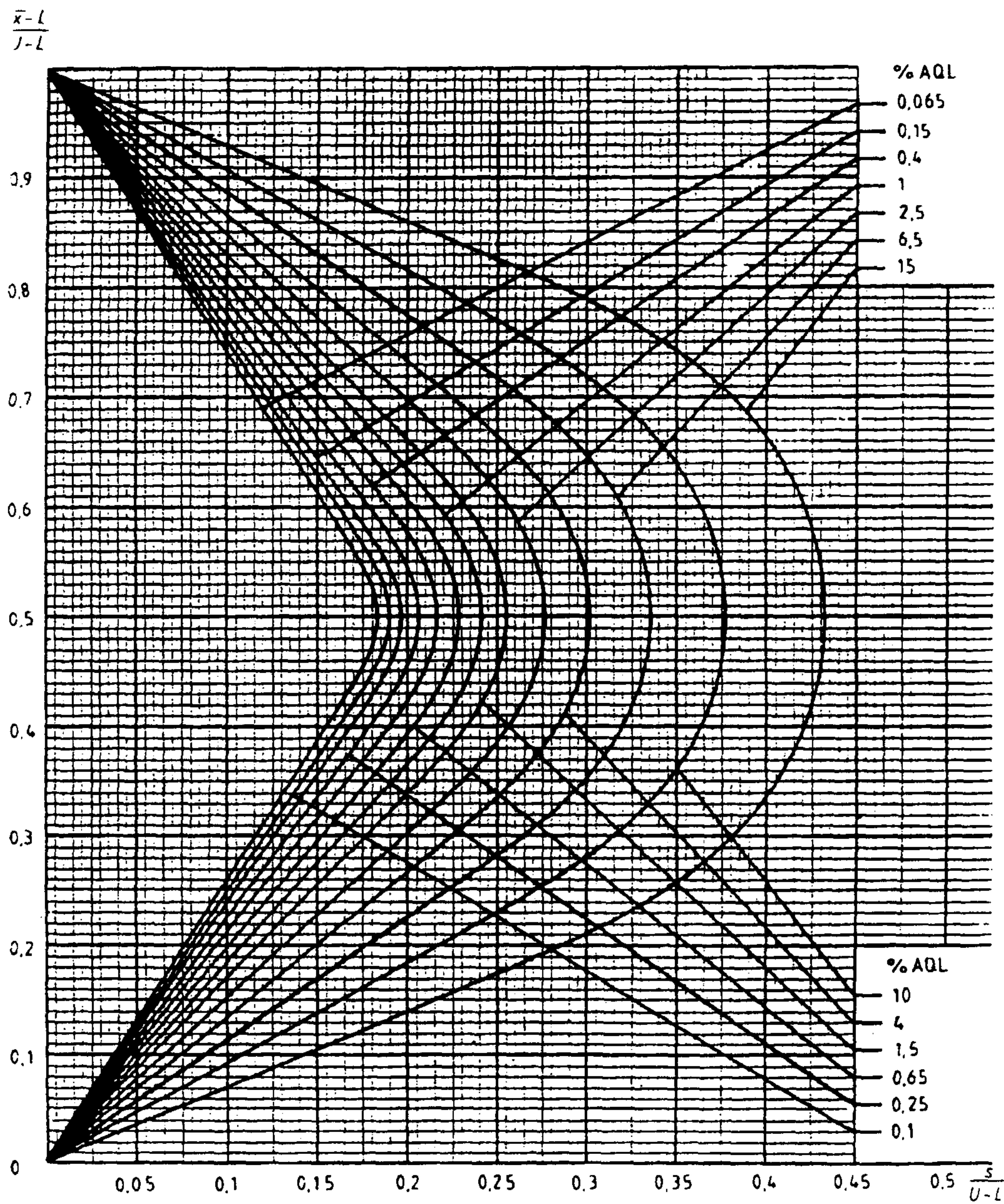
Диаграмма s-H — Кривые приемки для предельных значений с общим уровнем качества: s-метод для кода объема выборки Н (объем выборки — 20)
