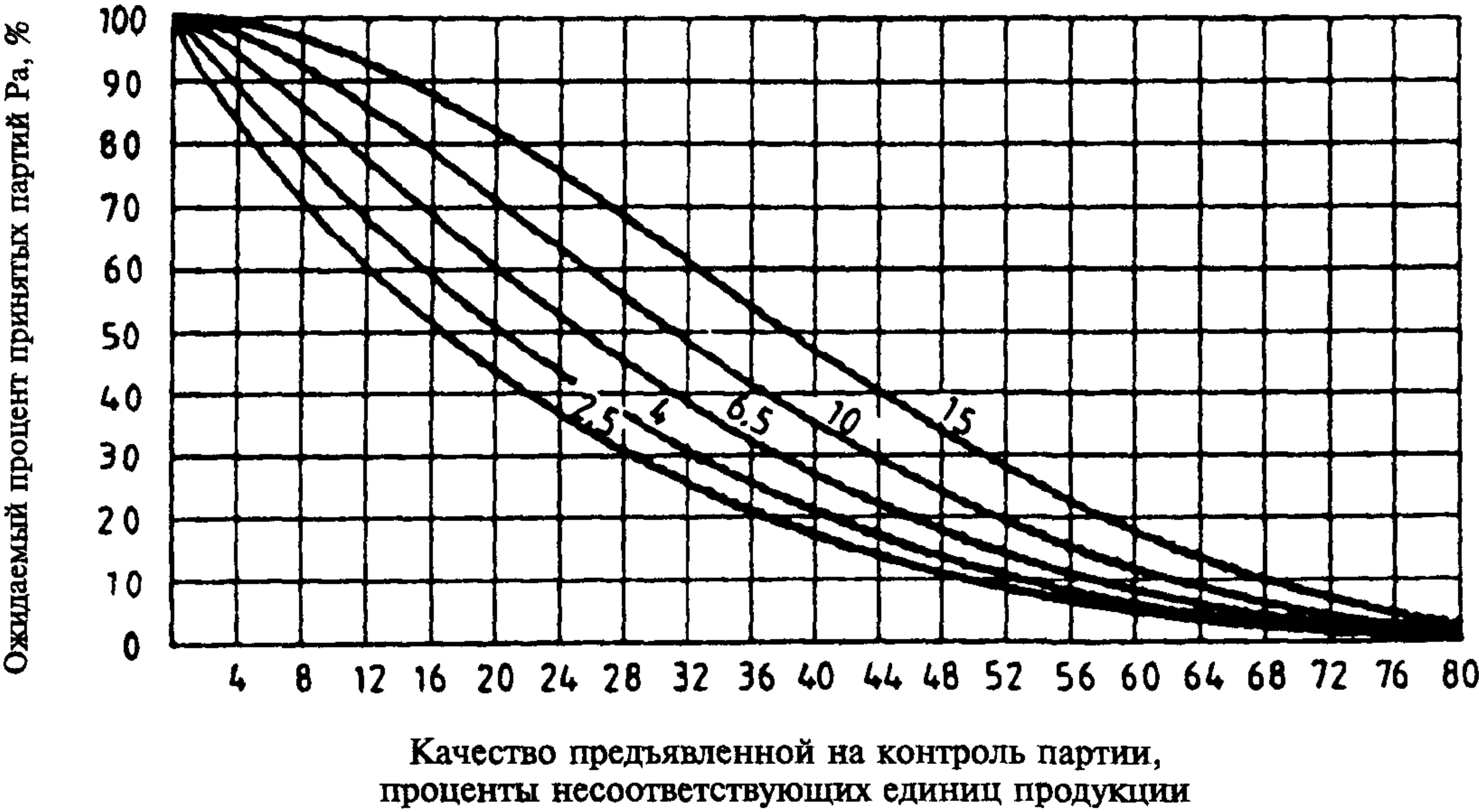
График VB — Оперативные характеристики для одноступенчатых выборочных планов контроля
