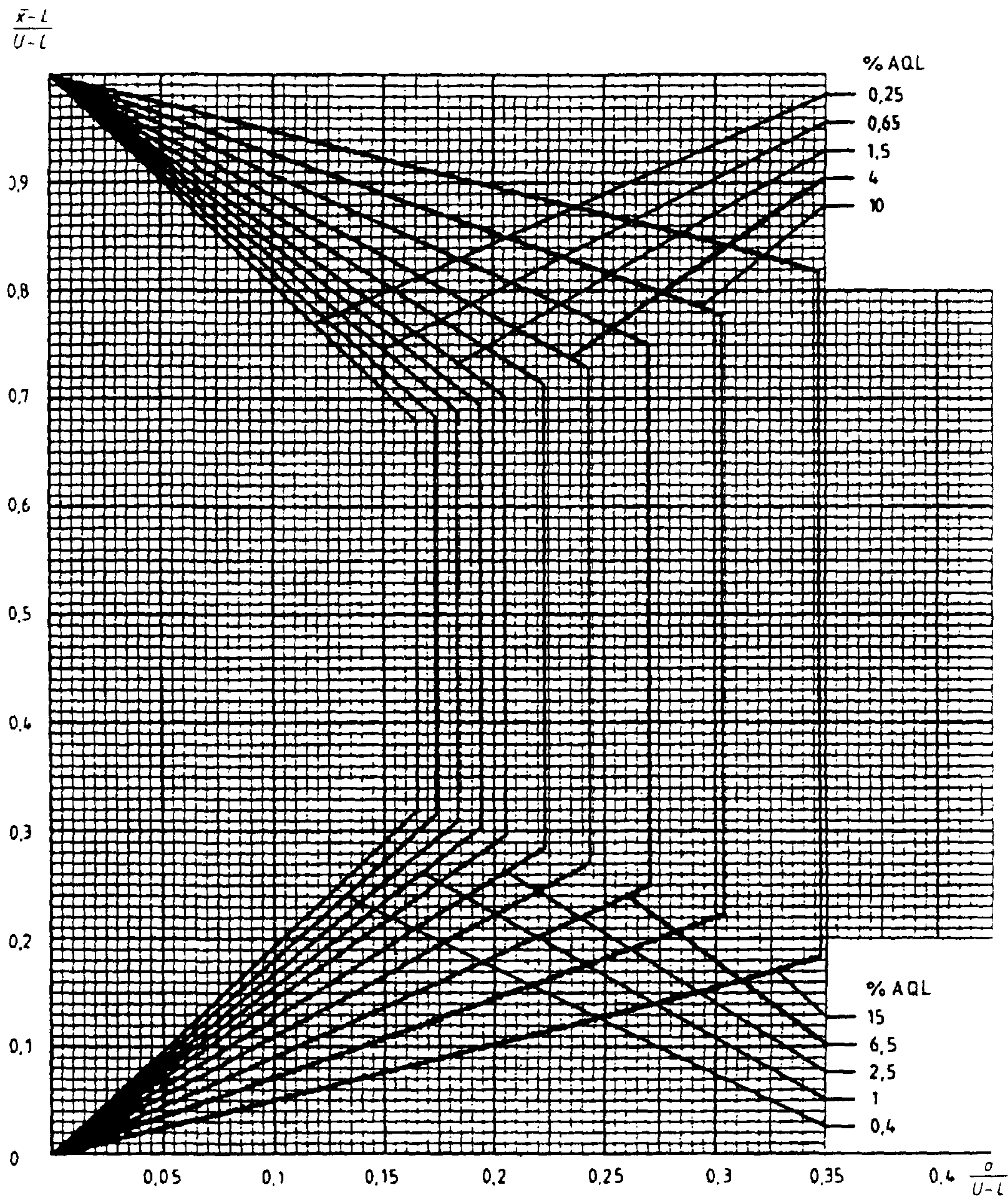
Диаграмма σ-E — Кривые приемки для предельных значений с общим уровнем качества: σ-метод для кода объема выборки E
