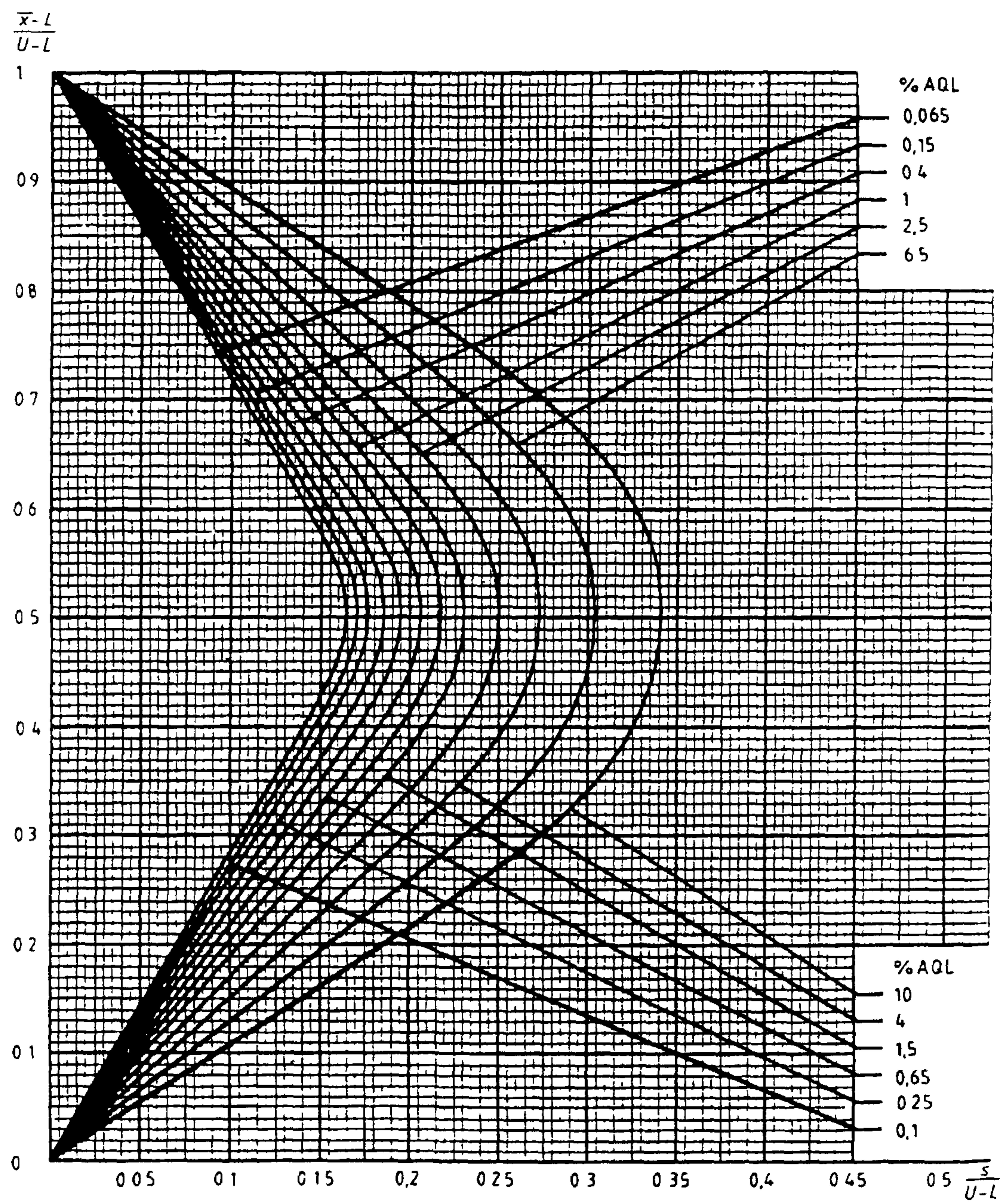
Диаграмма s-P — Кривые приемки для предельных значений с общим уровнем качества: s-метод для кода объема выборки Р (объем выборки — 200)
