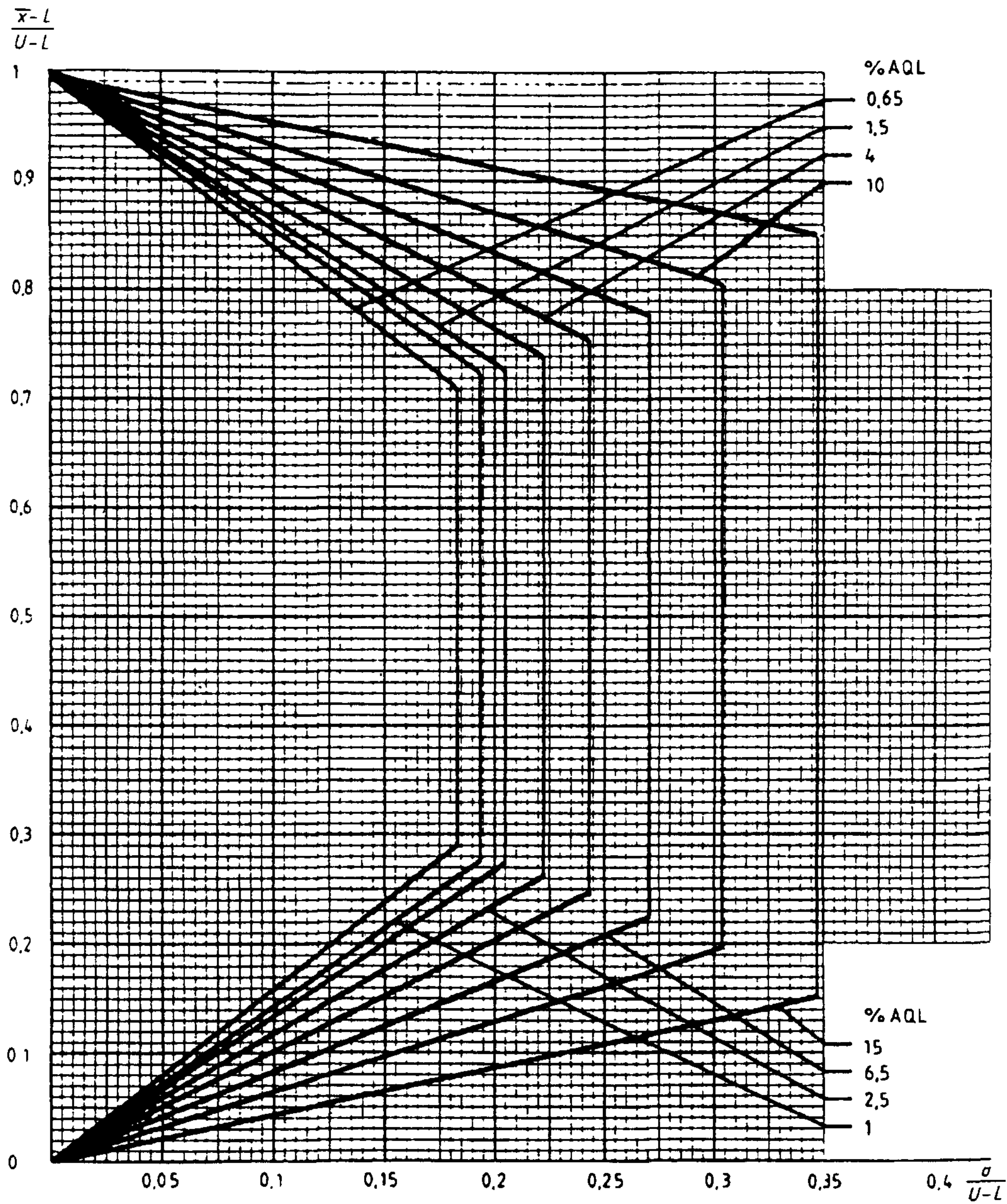
Диаграмма \sigma -D — Кривые приемки для предельных значений с общим уровнем качества: \sigma -метод для кода объема выборки D
