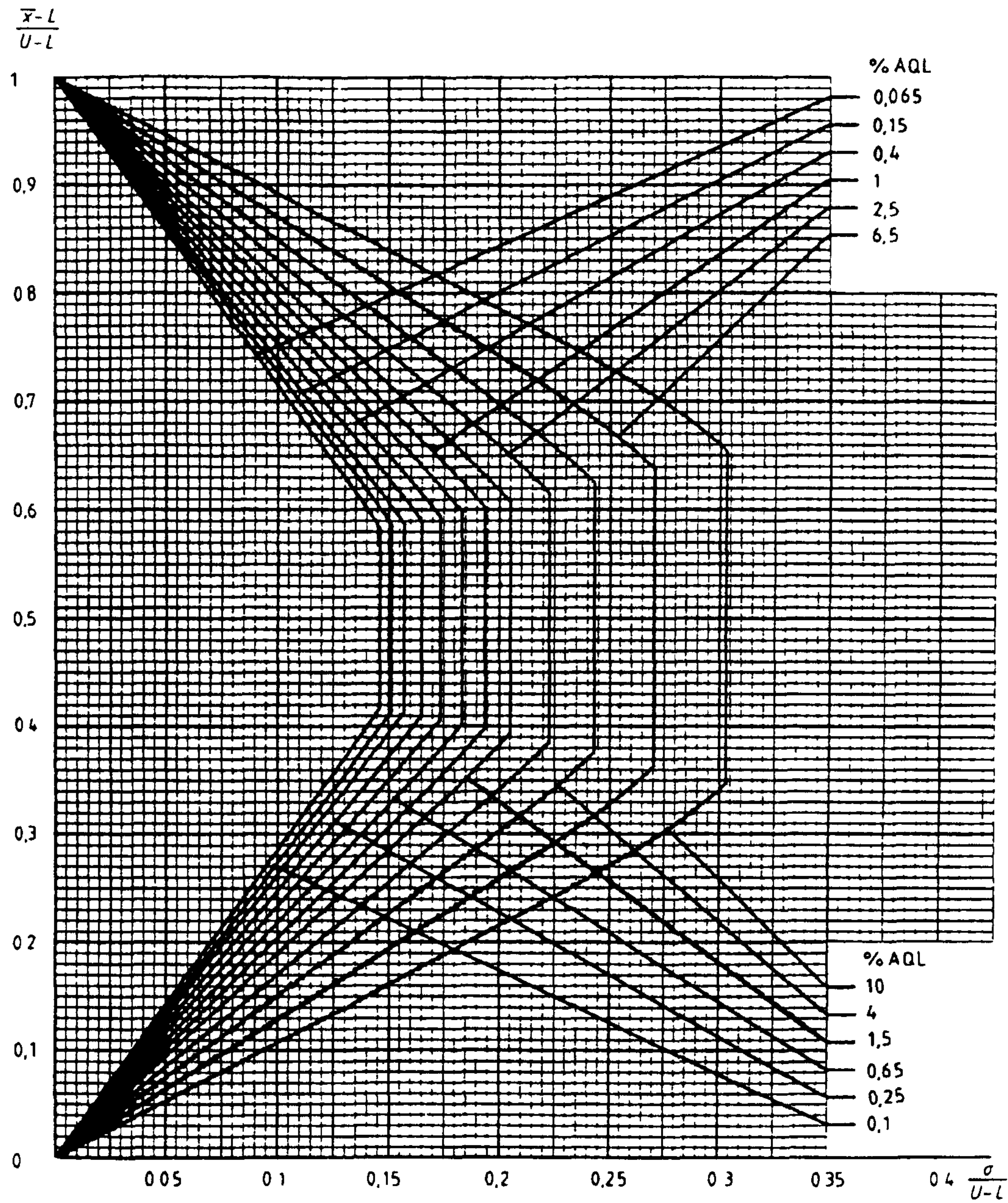
Диаграмма \sigma -N — Кривые приемки для предельных значений с общим уровнем качества: \sigma -метод для кода объема выборки N
