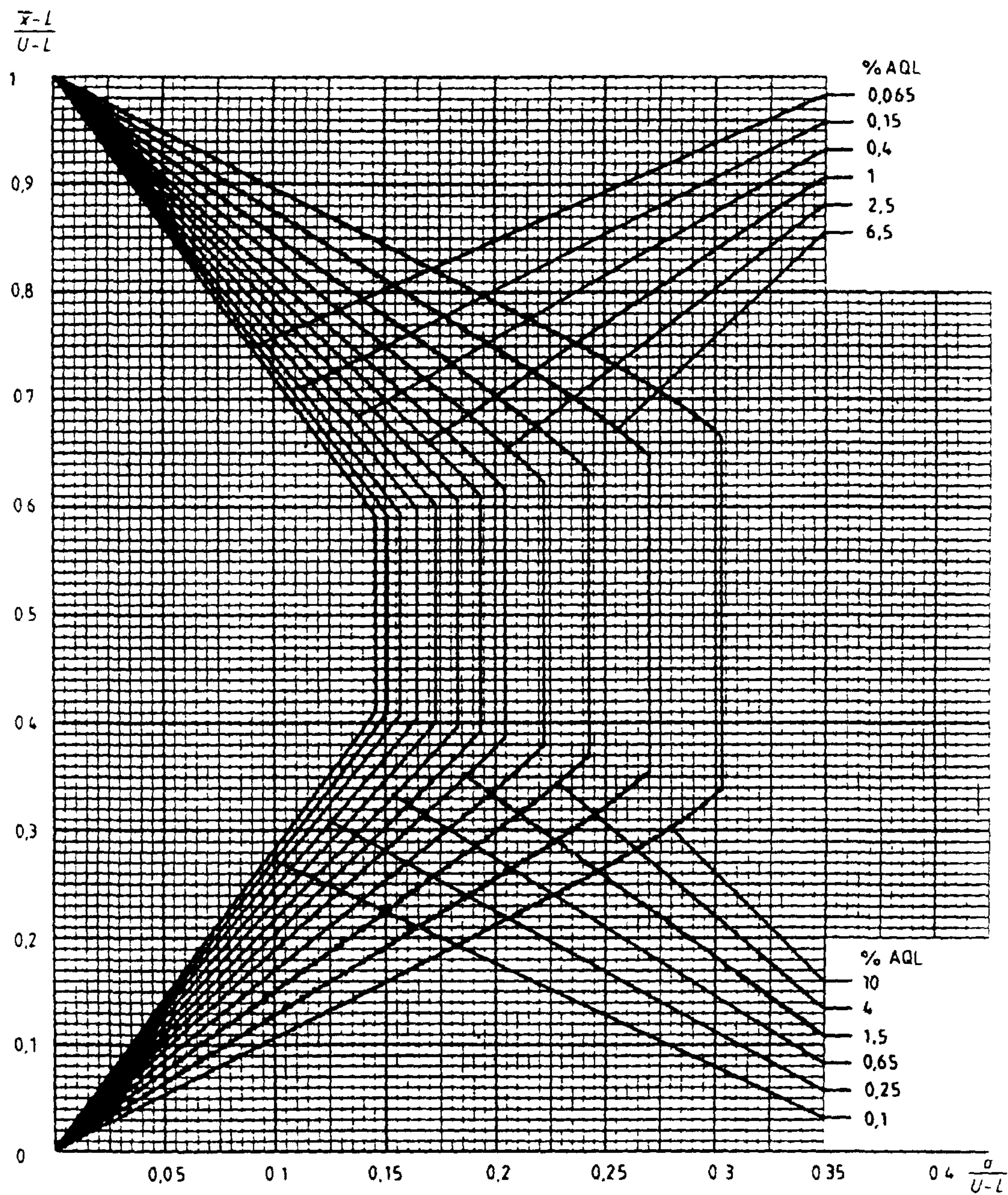
Диаграмма σ-M — Кривые приемки для предельных значений с общим уровнем качества: σ-метод для кода объема выборки M
