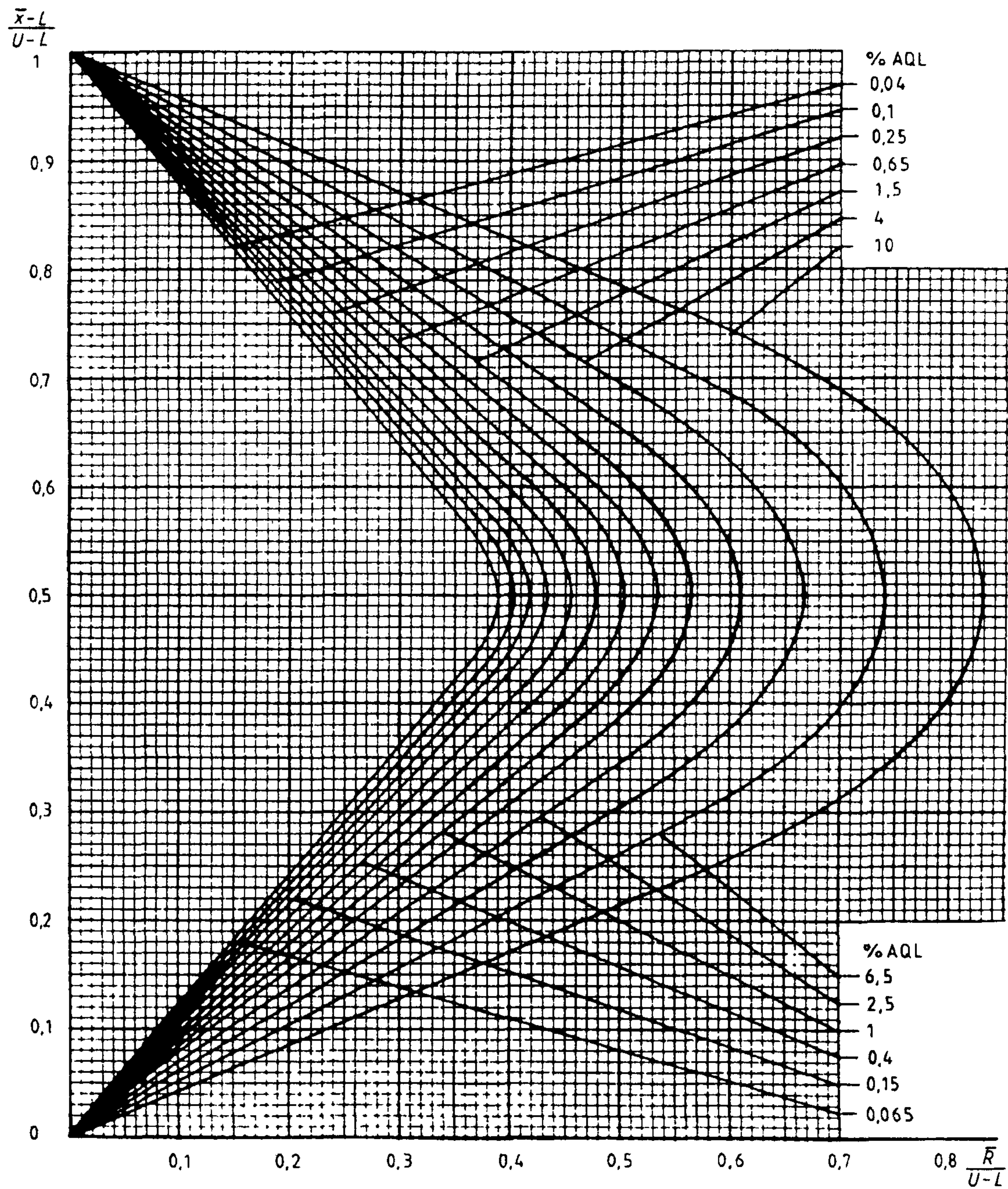
Диаграмма R-K — Кривые приемки для предельных значений с общим уровнем качества: R-метод для кода объема выборки K (объем выборки — 60)
