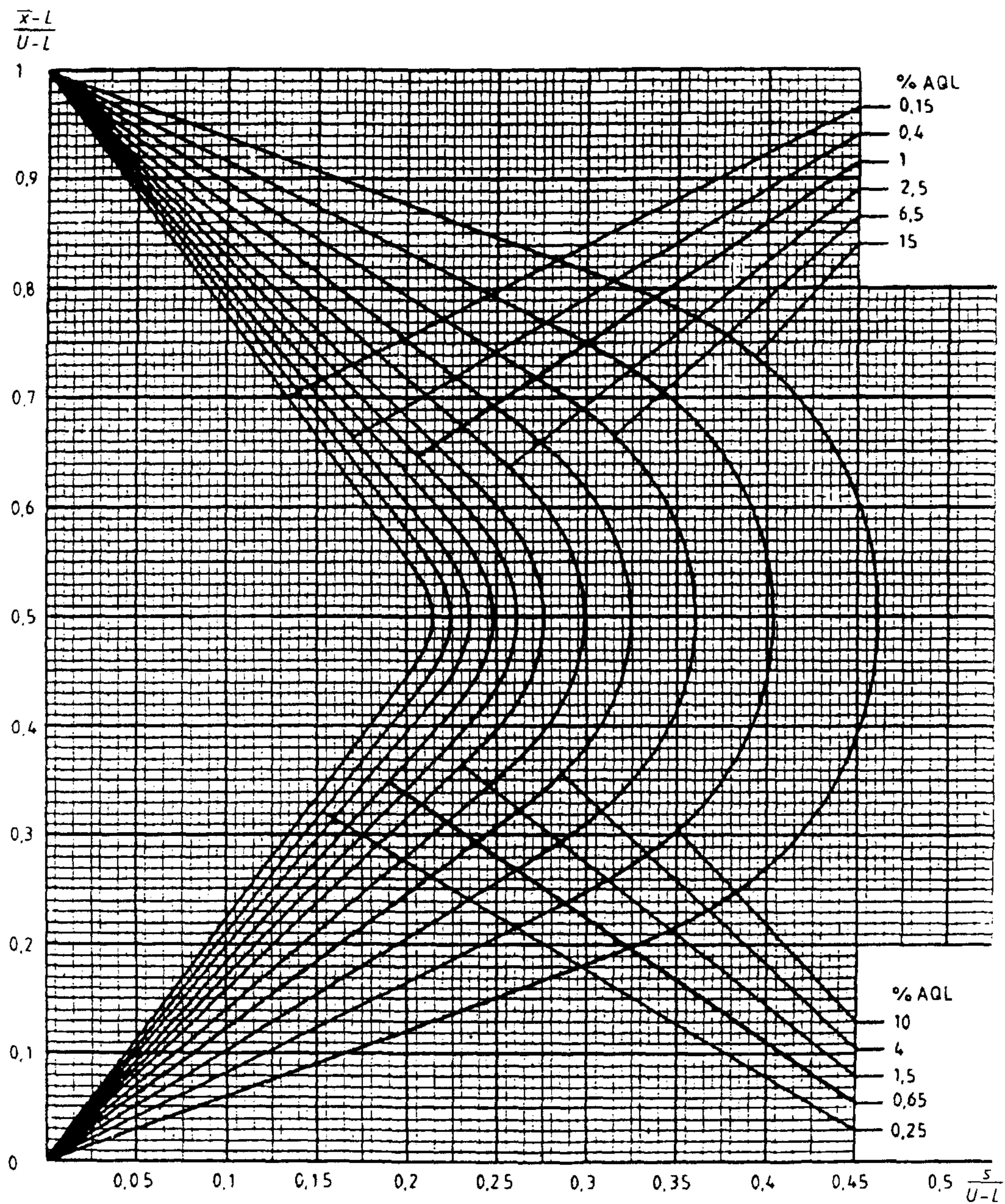
Диаграмма s-F — Кривые приемки для предельных значений с общим уровнем качества: s-метод для кода объема выборки F (объем выборки — 10)
