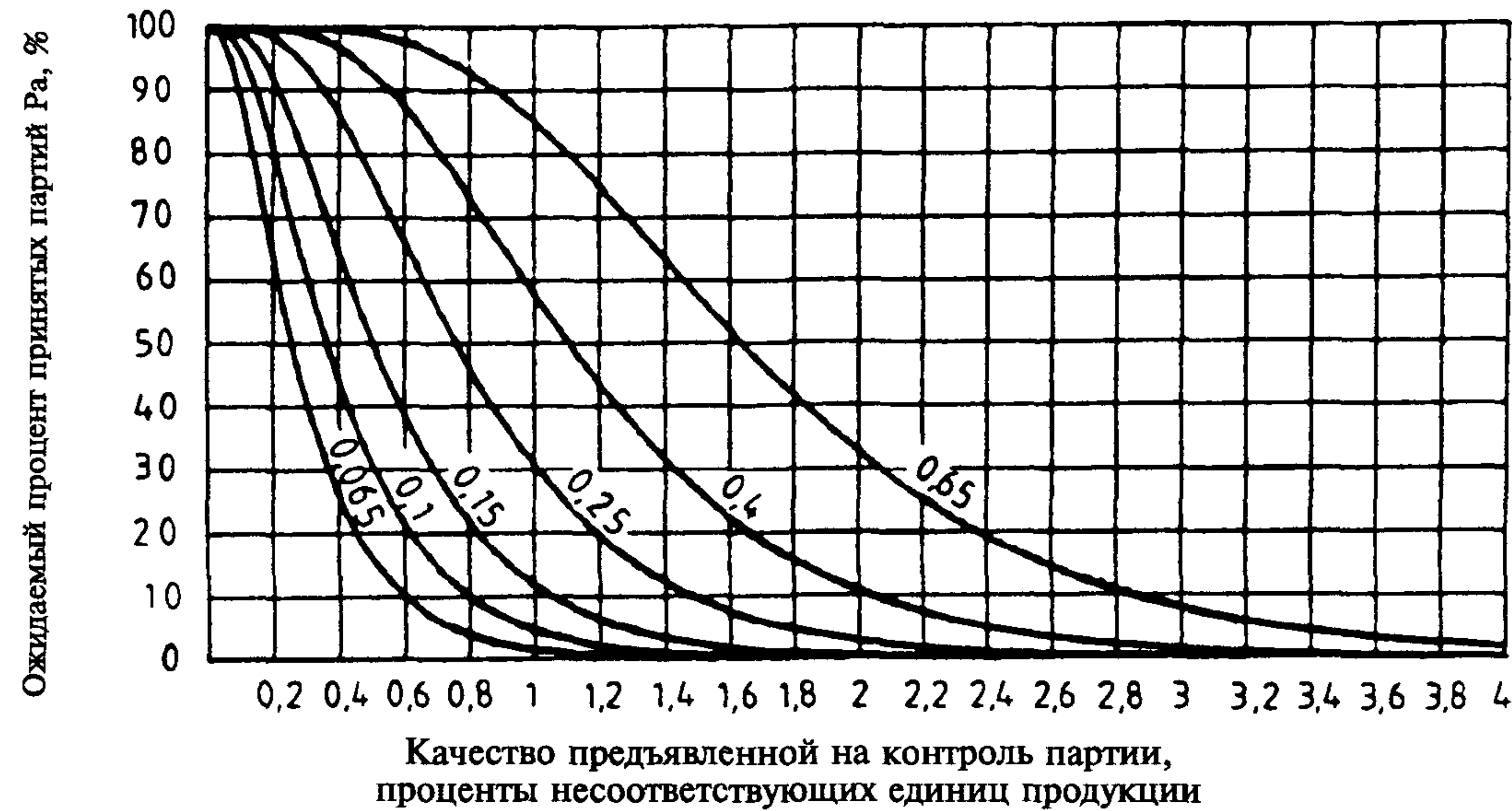
График VM — Оперативные характеристики для одноступенчатых выборочных планов контроля
