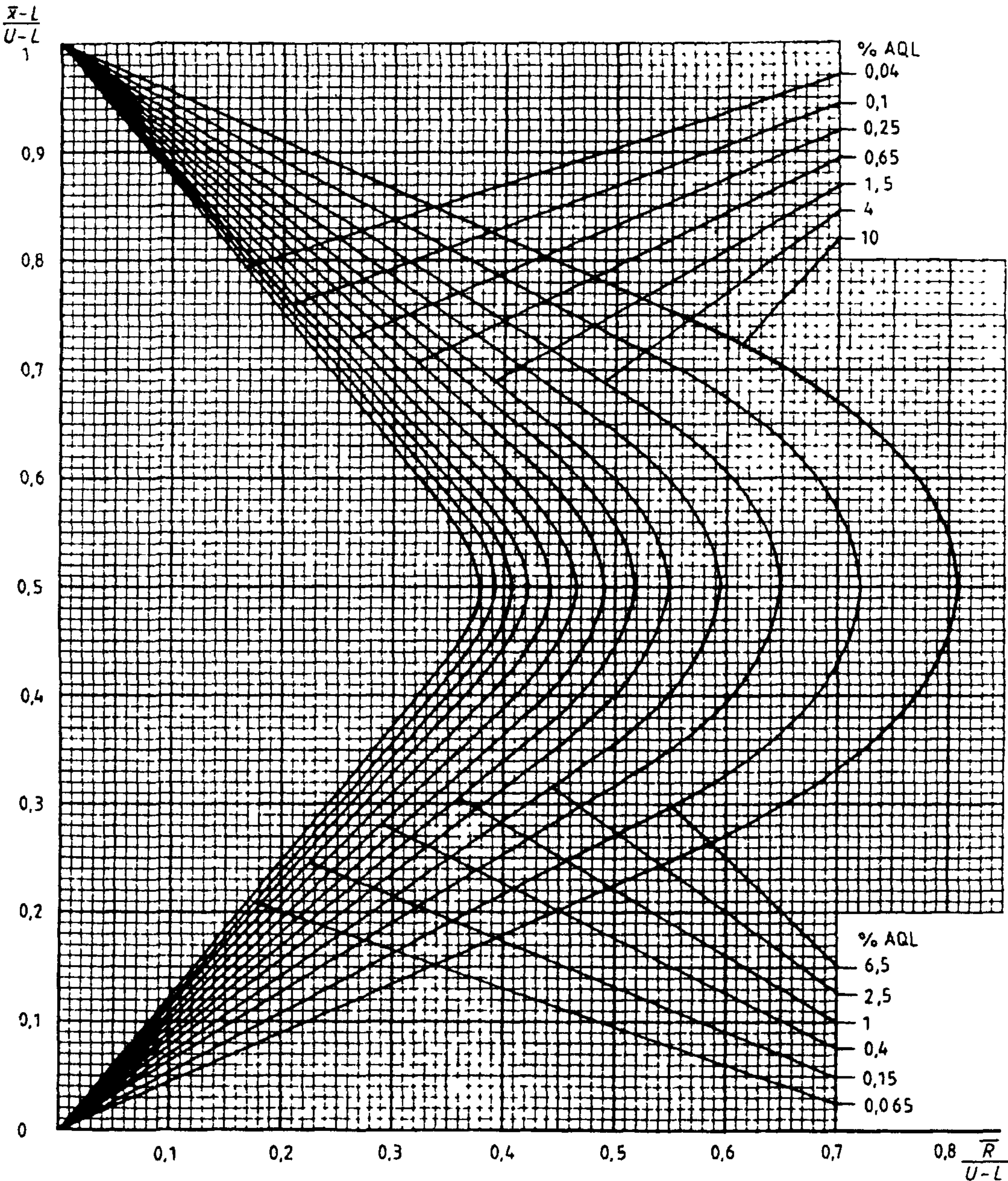
Диаграмма R-M — Кривые приемки для предельных значений с общим уровнем качества R-метод для кода объема выборки M (объем выборки — 115)
