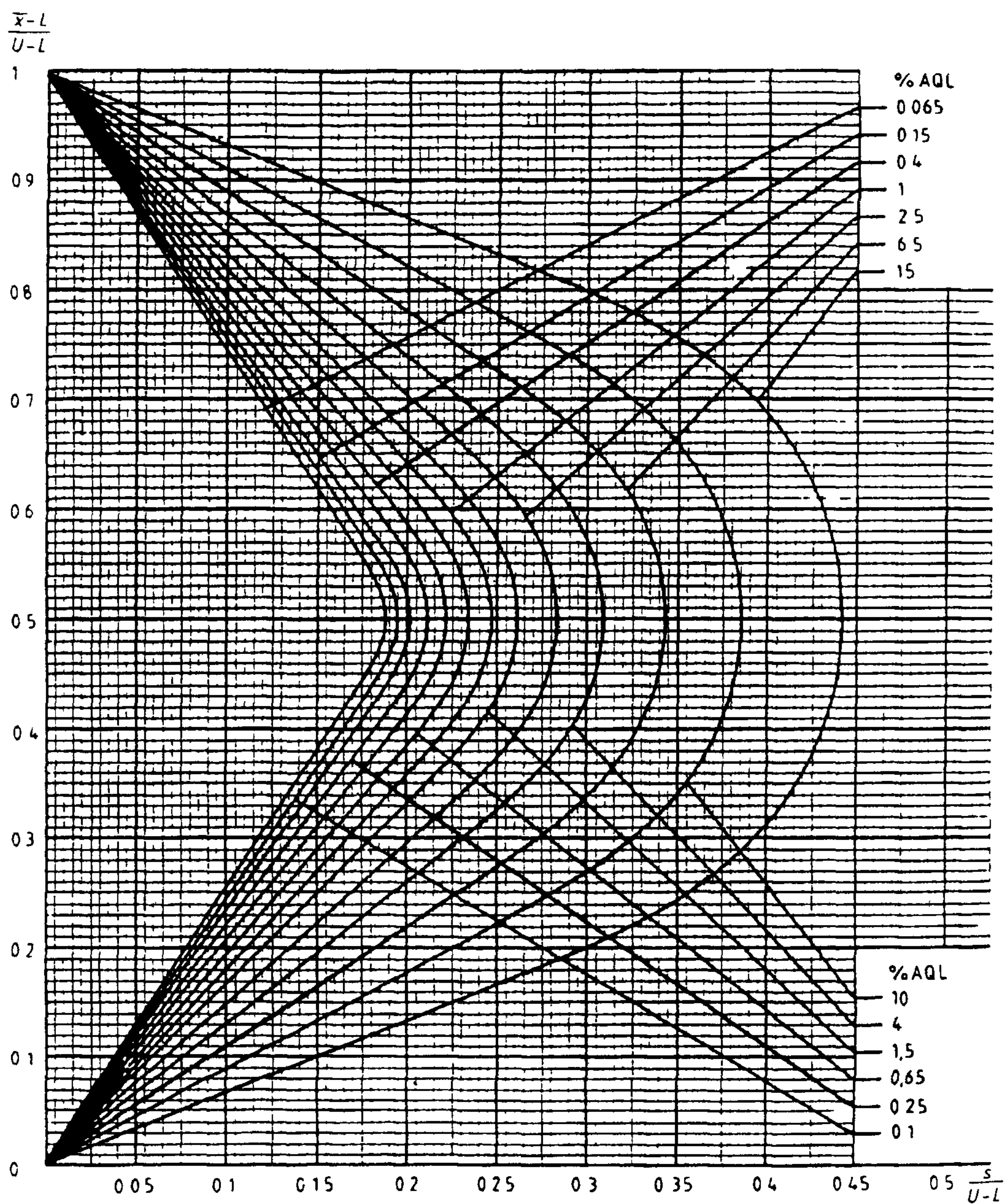
Диаграмма s-G — Кривые приемки для предельных значений с общим уровнем качества: s-метод для кода объема выборки G (объем выборки — 15)
