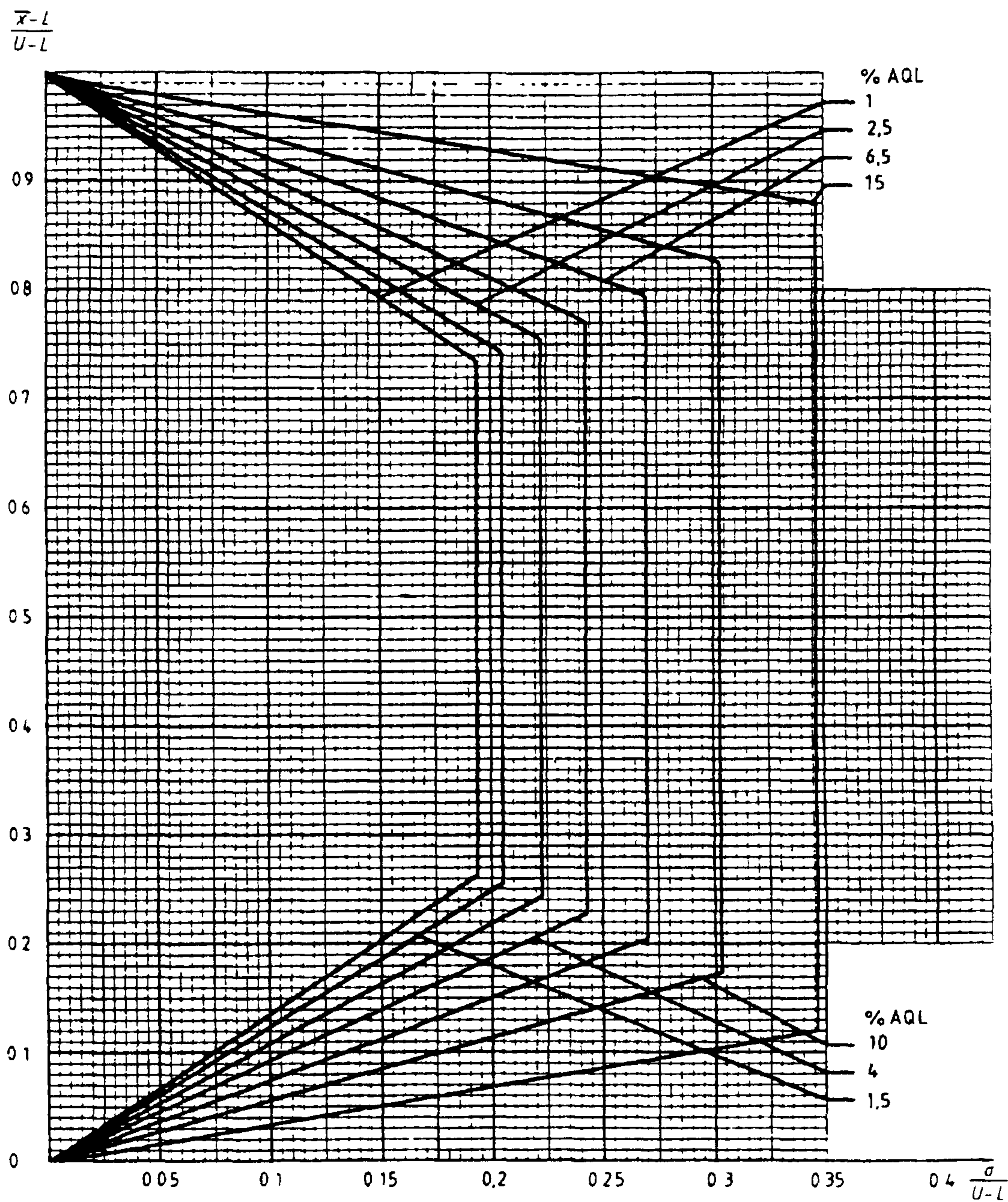
Диаграмма \sigma -С — Кривые приемки для предельных значений с общим уровнем качества. \sigma -метод для кода объема выборки С
