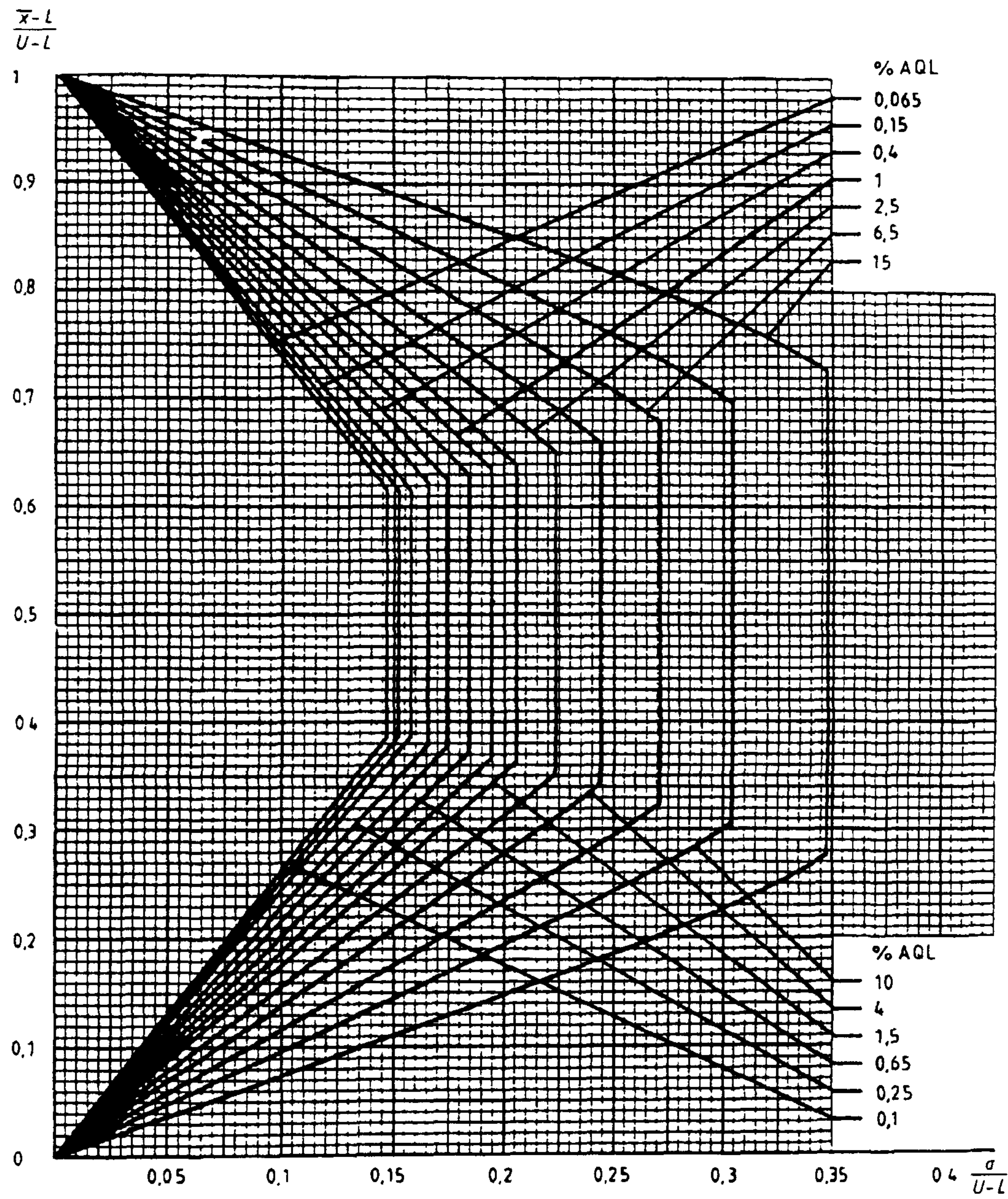
Диаграмма σ-J — Кривые приемки для предельных значений с общим уровнем качества: σ-метод для кода объема выборки J
