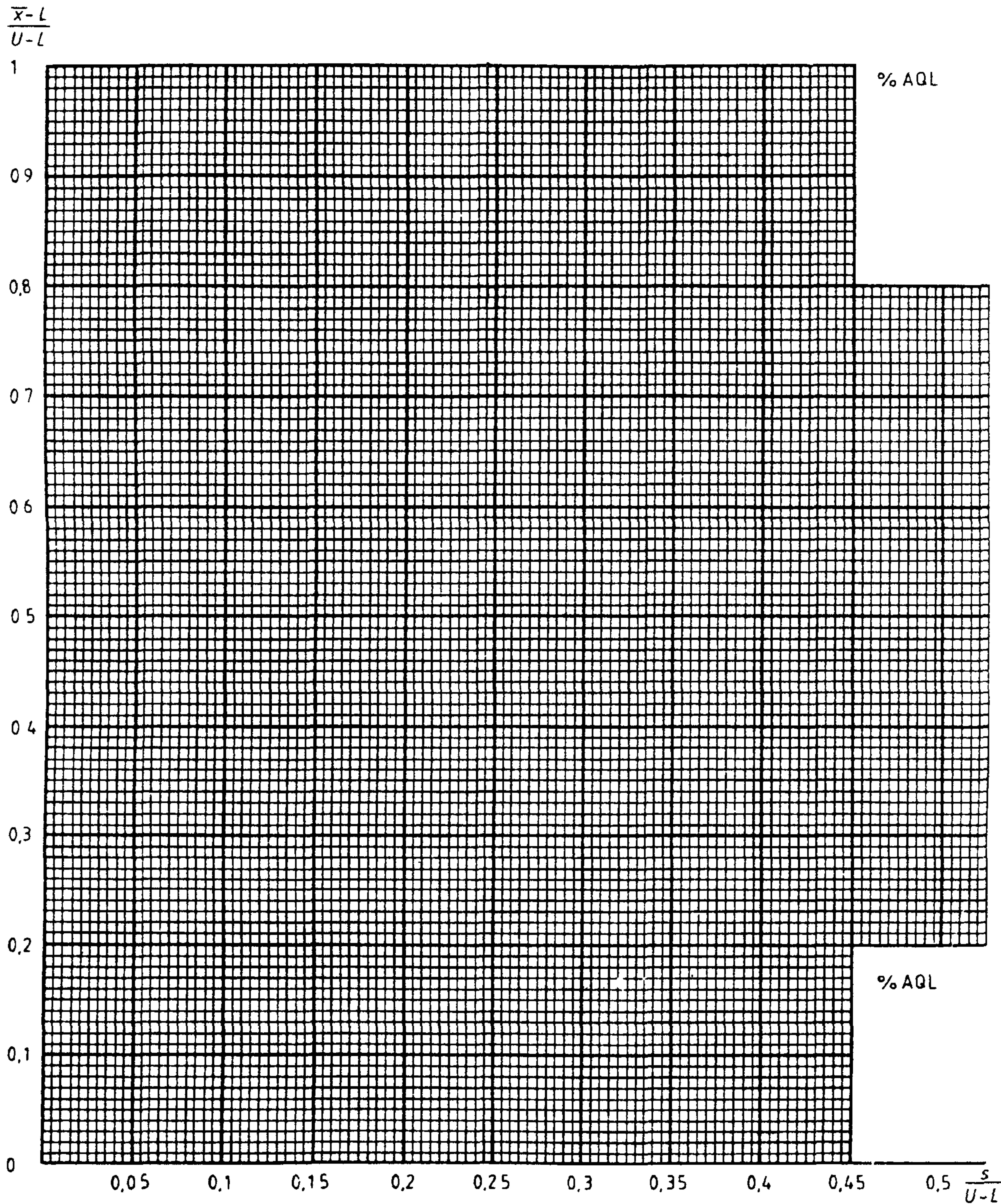
Рисунок 18 — Графическая бумага для s-метода
