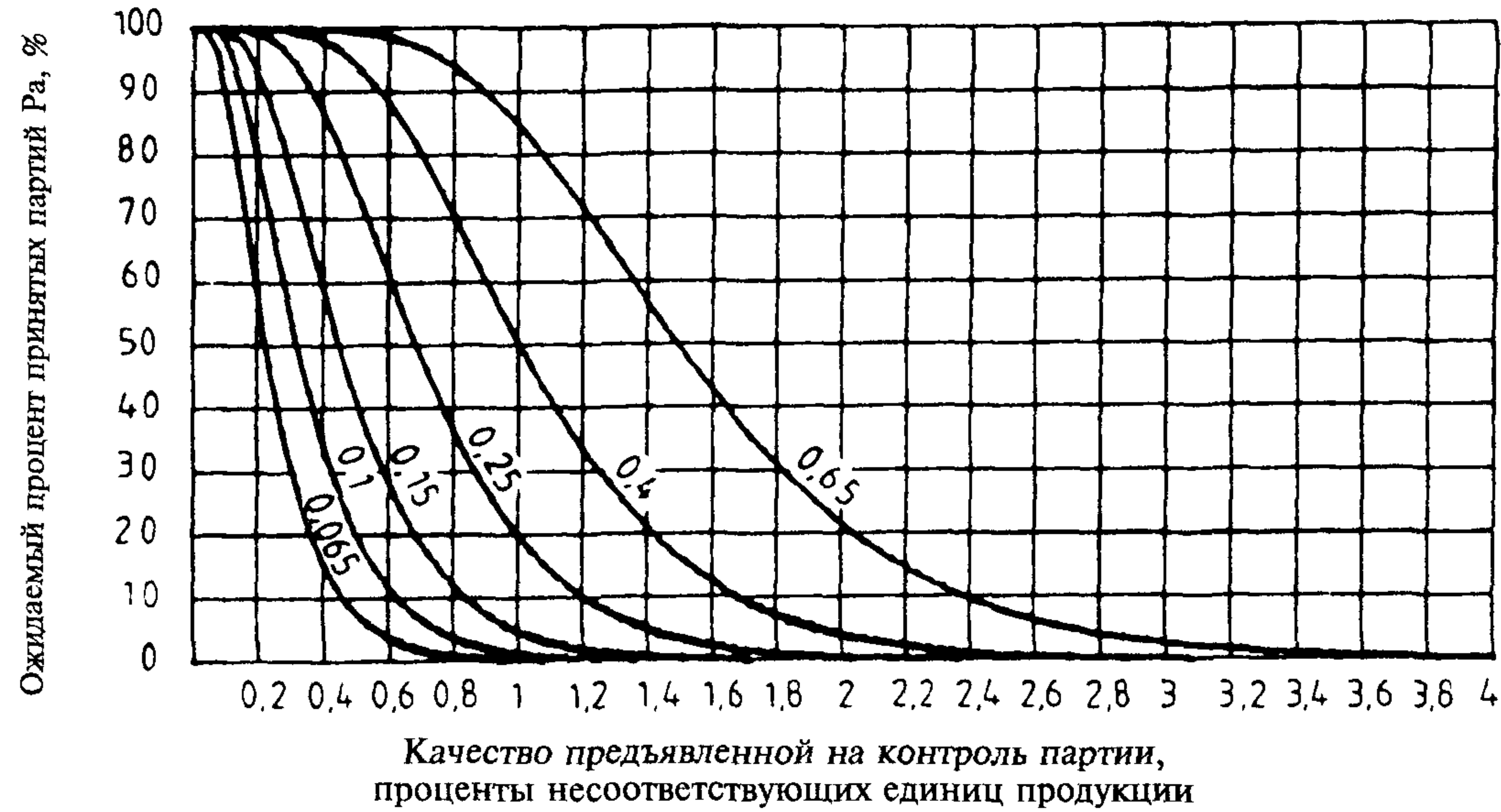
График VN — Оперативные характеристики для одноступенчатых выборочных планов контроля
