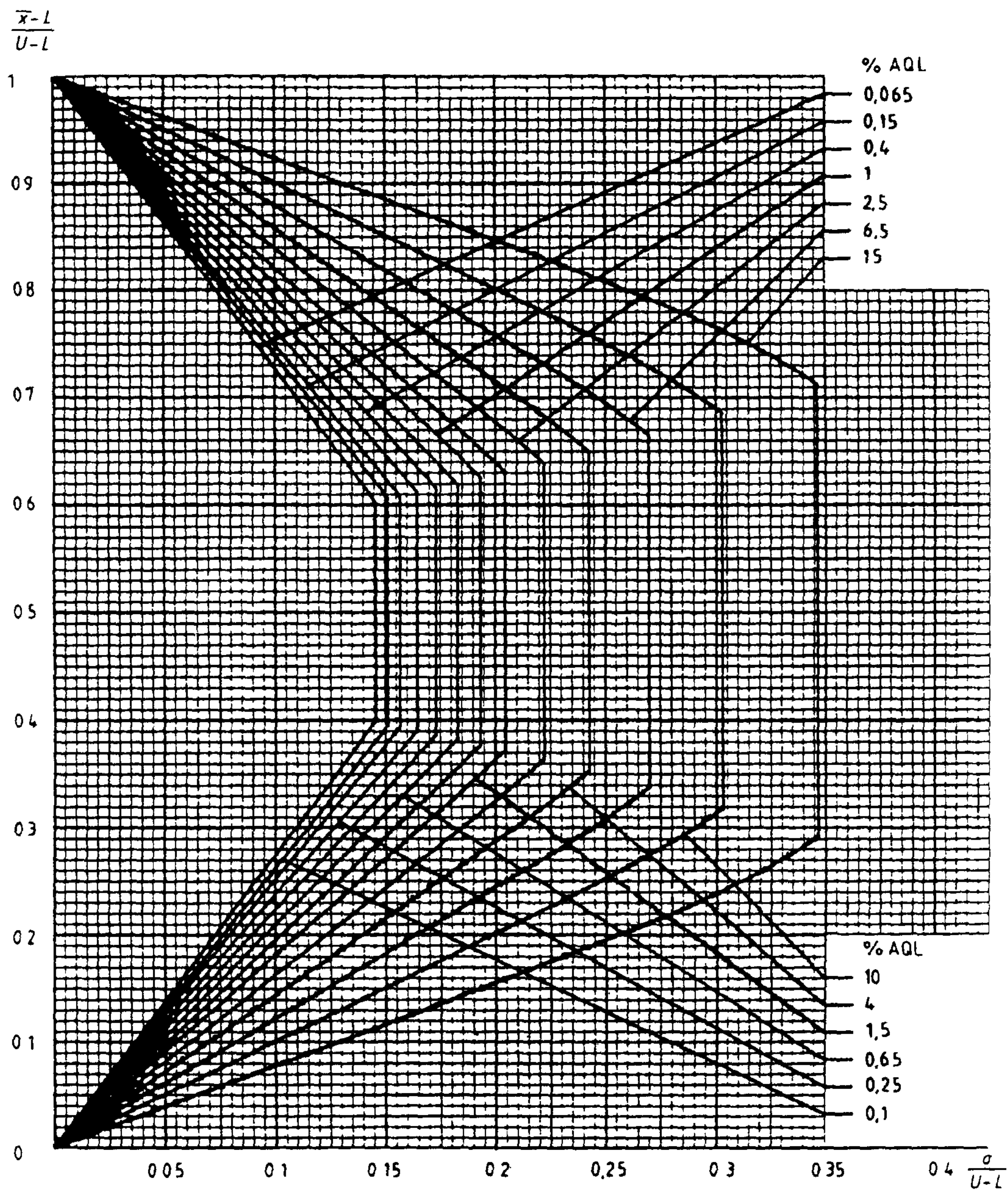
Диаграмма \sigma -K — Кривые приемки для предельных значений с общим уровнем качества. \sigma -метод для кода объема выборки K
