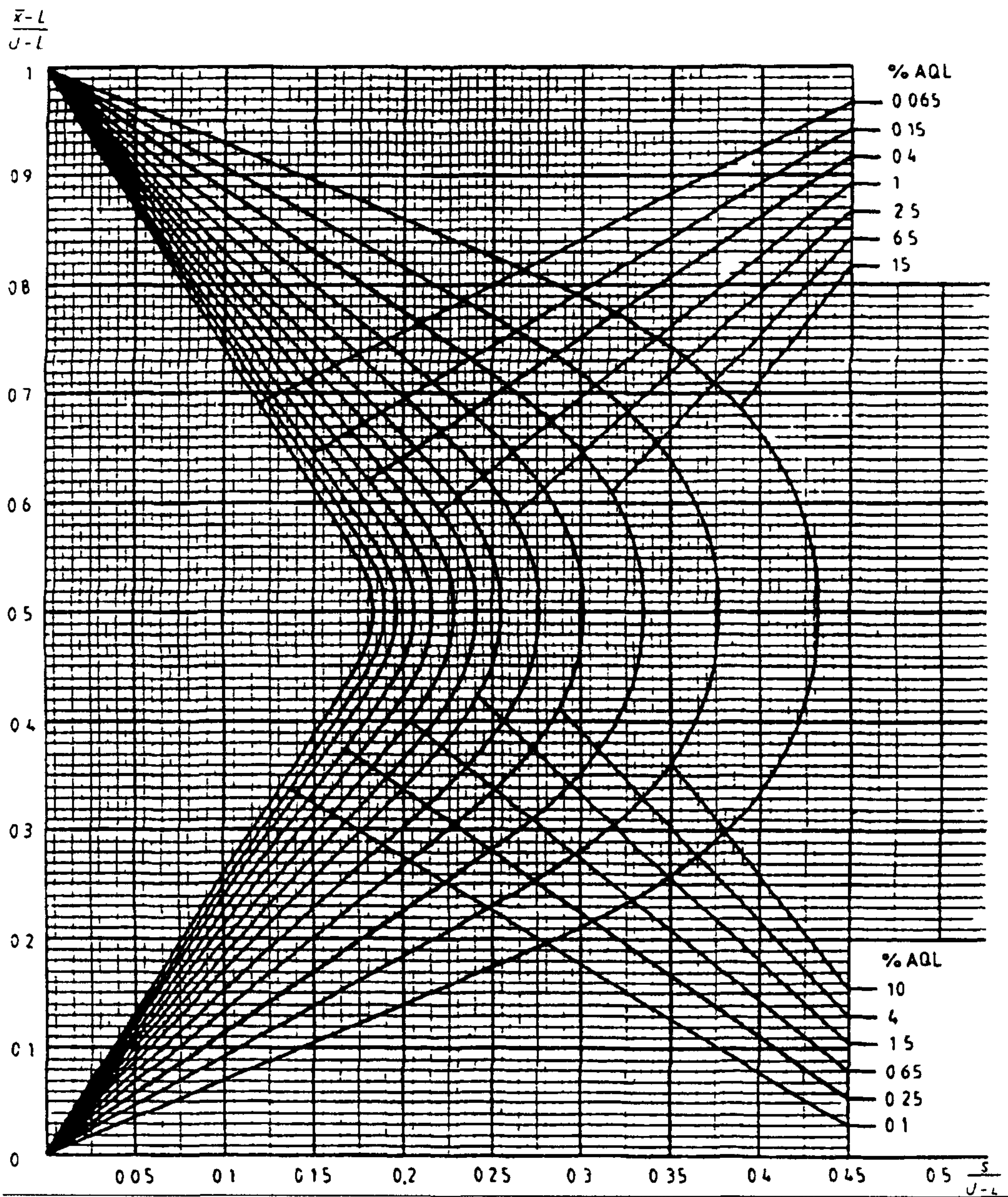
Диаграмма R-H — Кривые приемки для предельных значений с общим уровнем качества R-метод для кода объема выборки H (объем выборки — 20)
