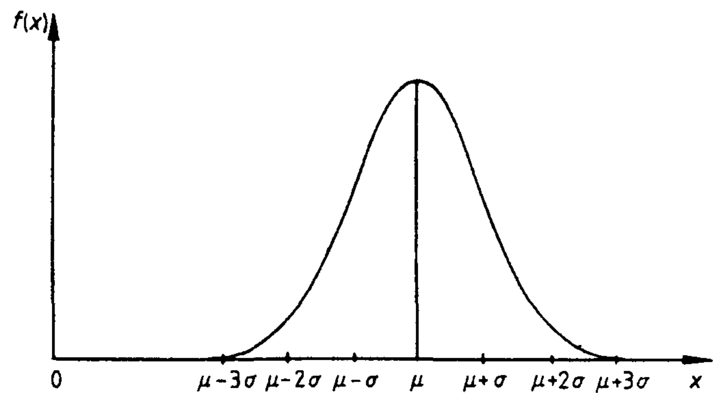
Рисунок 5 — Нормальное распределение
