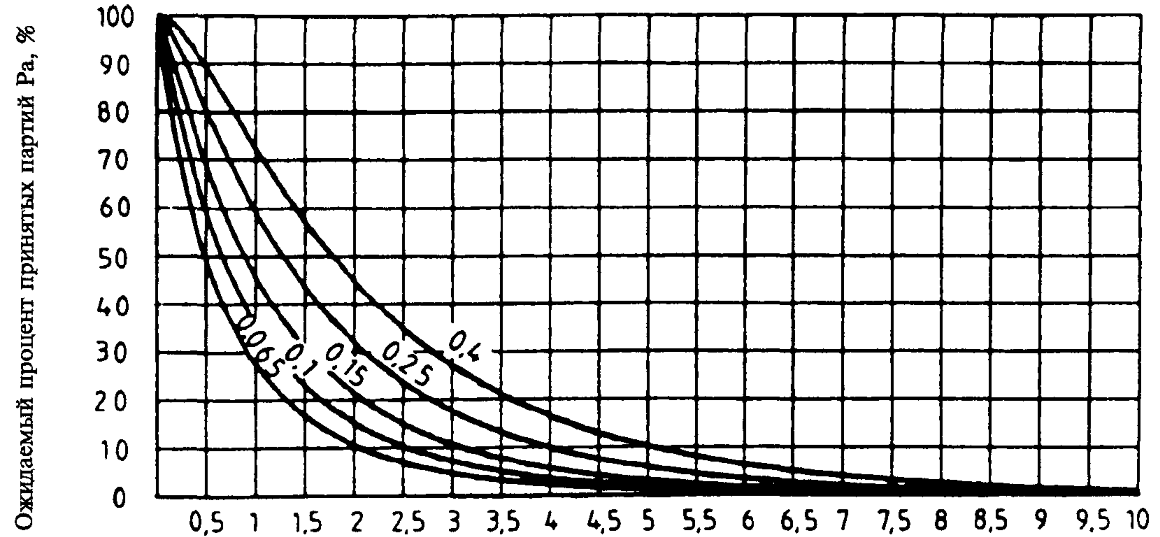
График VI — Оперативные характеристики для одноступенчатых выборочных планов контроля
