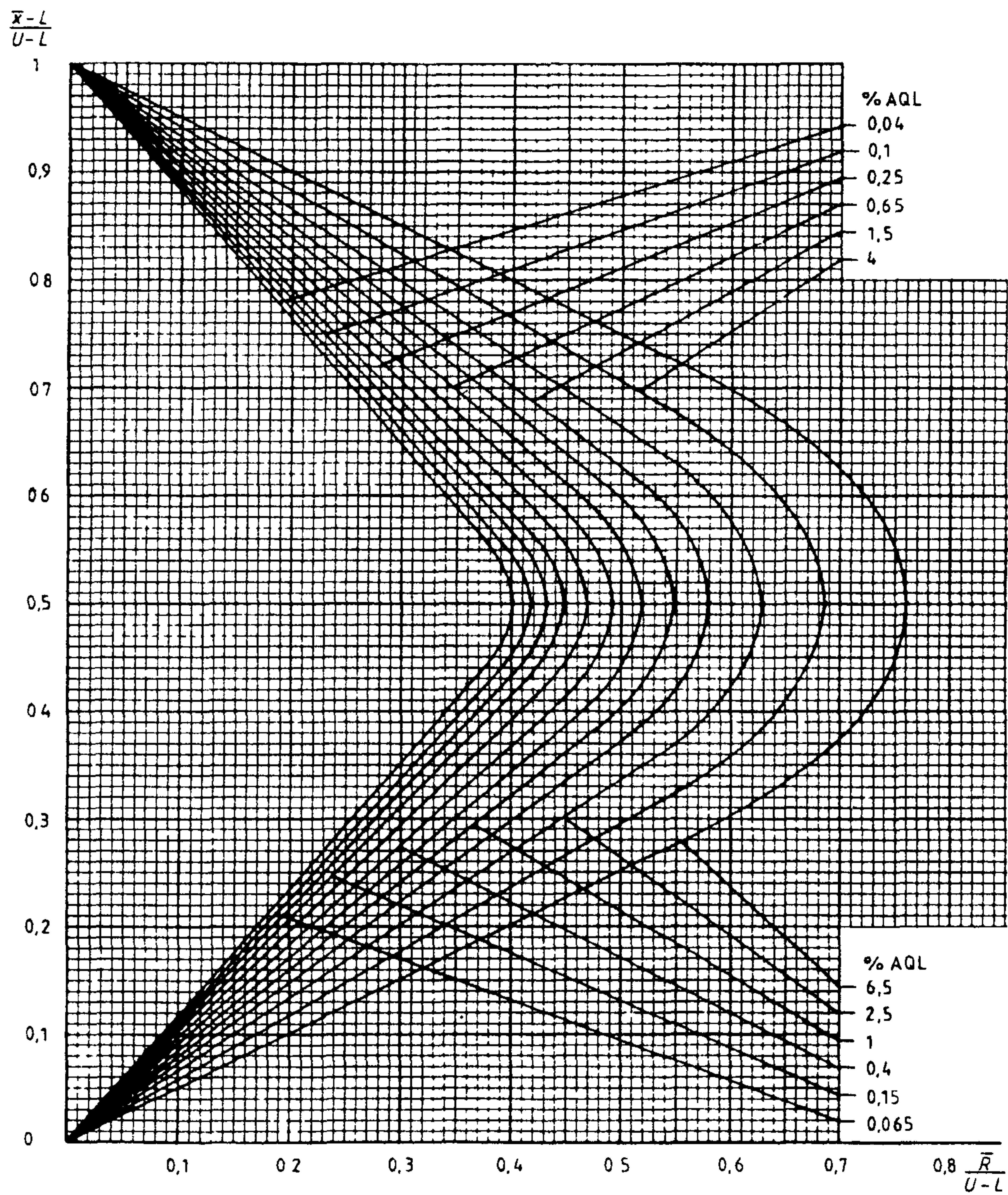
Диаграмма R-J — Кривые приемки для предельных значений с общим уровнем качества: R-метод для кода объема выборки J (объем выборки — 40)
