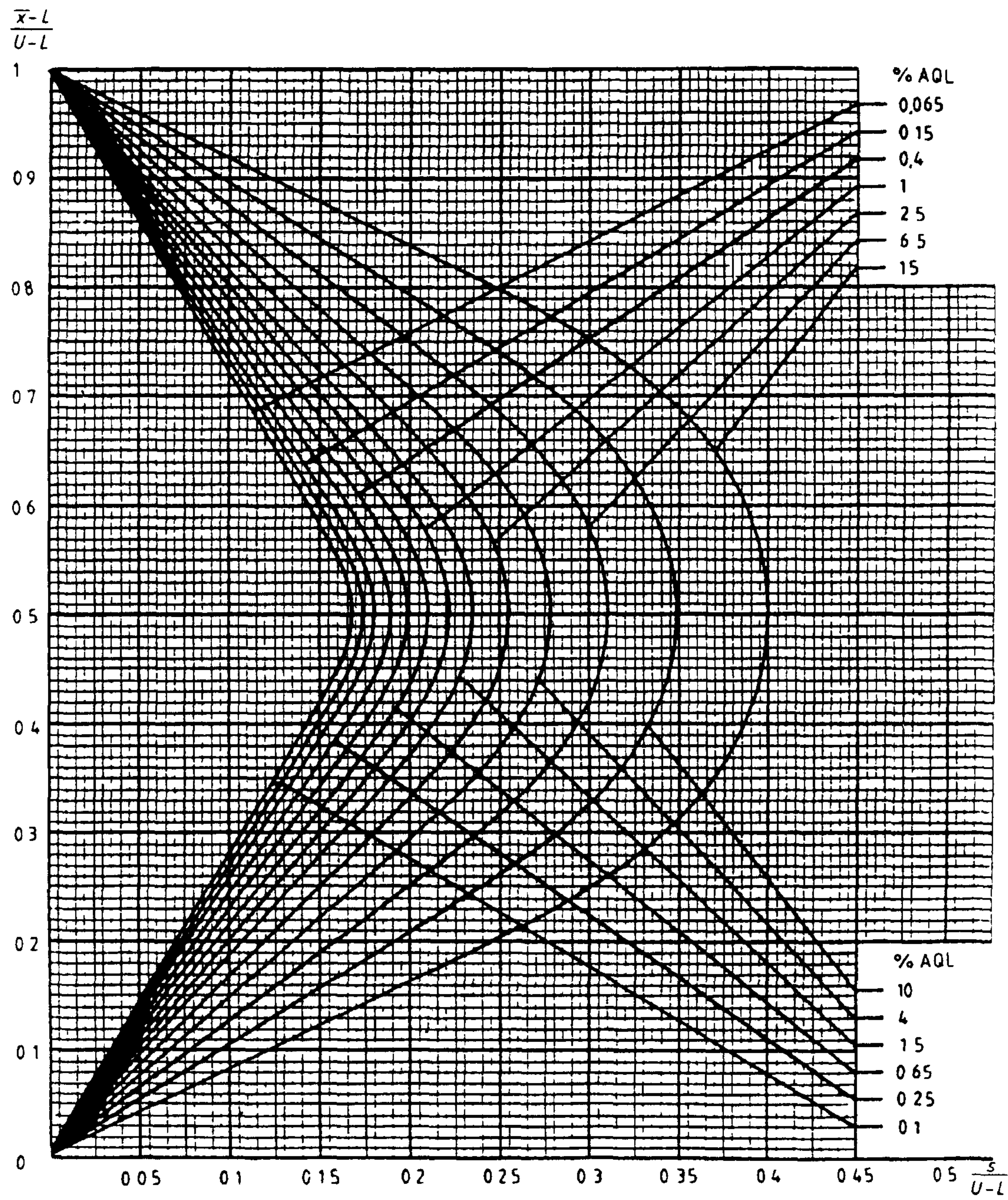
Диаграмма s-L — Кривые приемки для предельных значений с общим уровнем качества s-метод для кода объема выборки L (объем выборки — 75)
