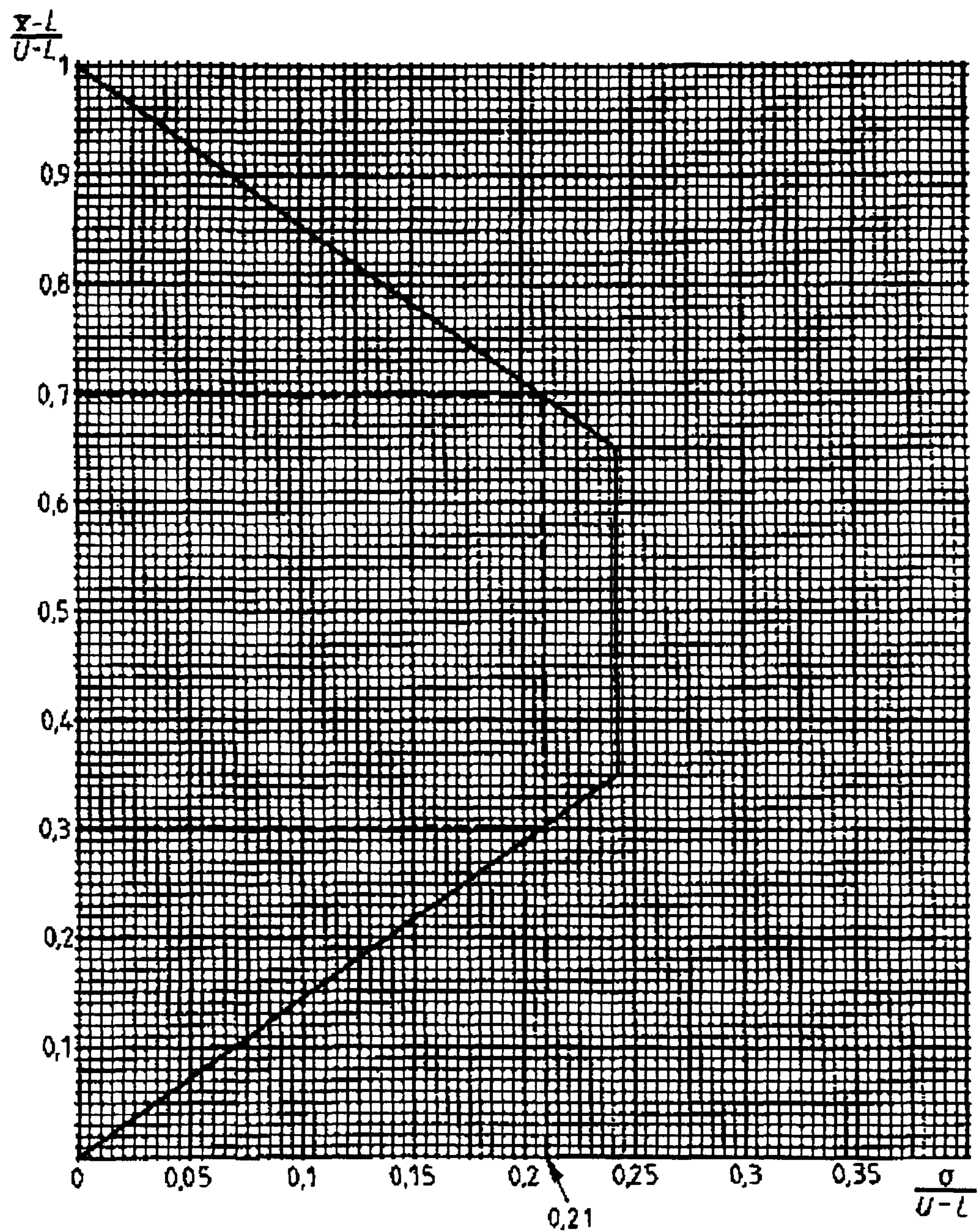
Рисунок 4 — Пример применения приемочной карты для предельных значений двустороннего допуска с общим AQL (σ-метод)
