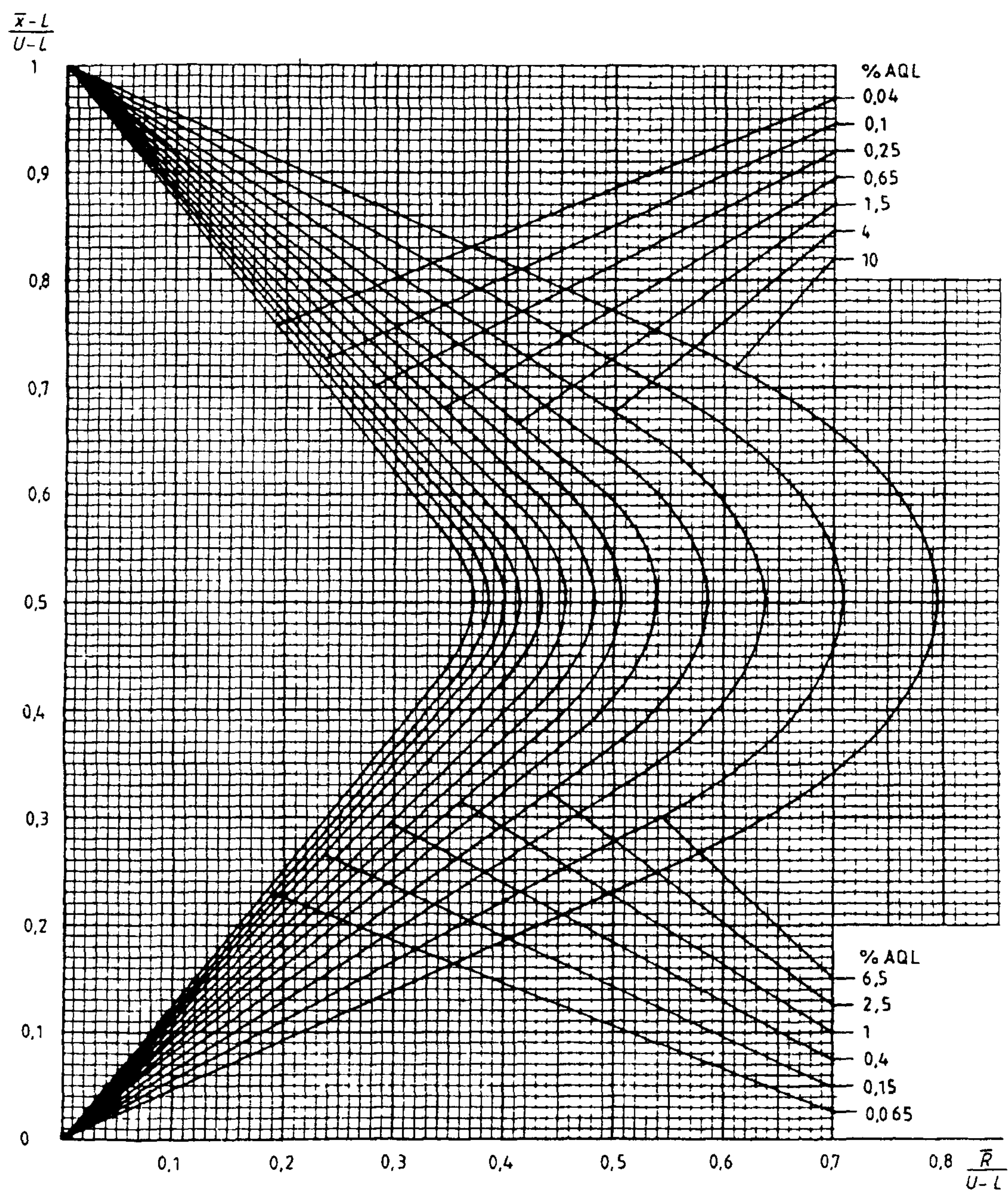
Диаграмма R-N — Кривые приемки для предельных значений с общим уровнем качества: R-метод для кода объема выборки N (объем выборки — 175)
