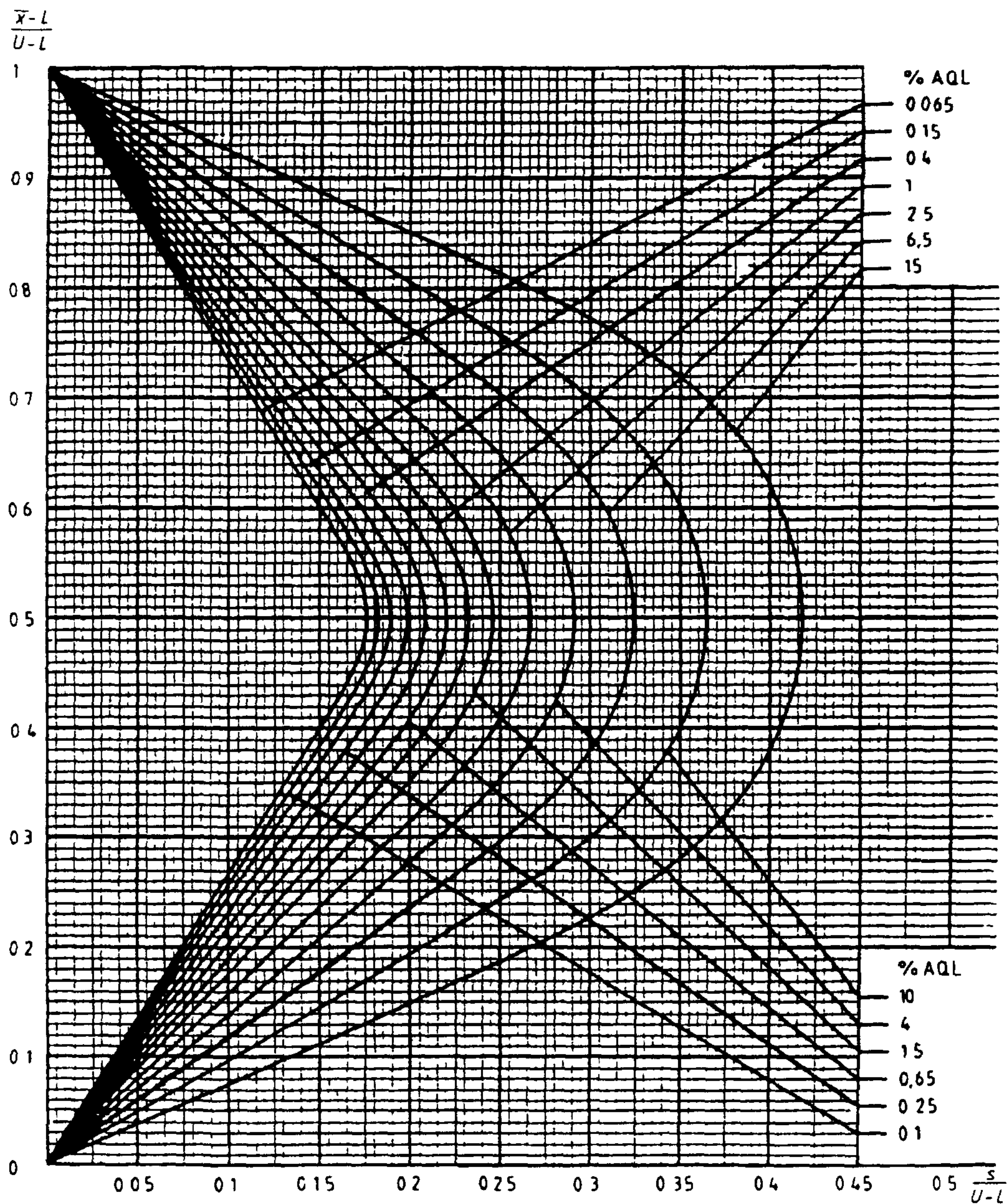
Диаграмма s-J — Кривые приемки для предельных значений с общим уровнем качества: s-метод для кода объема выборки J (объем выборки — 35)
