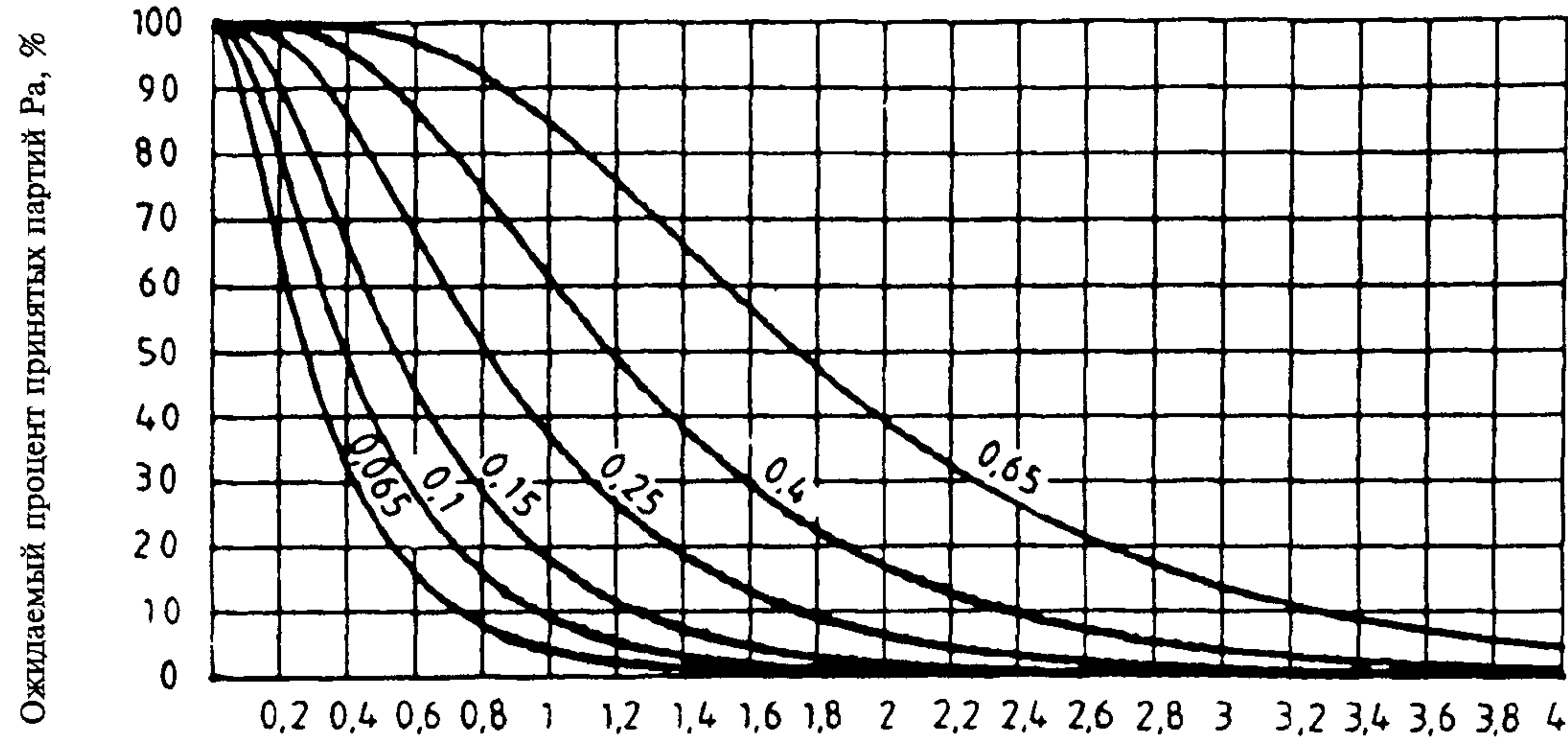
График VL — Оперативные характеристики для одноступенчатых выборочных планов контроля
