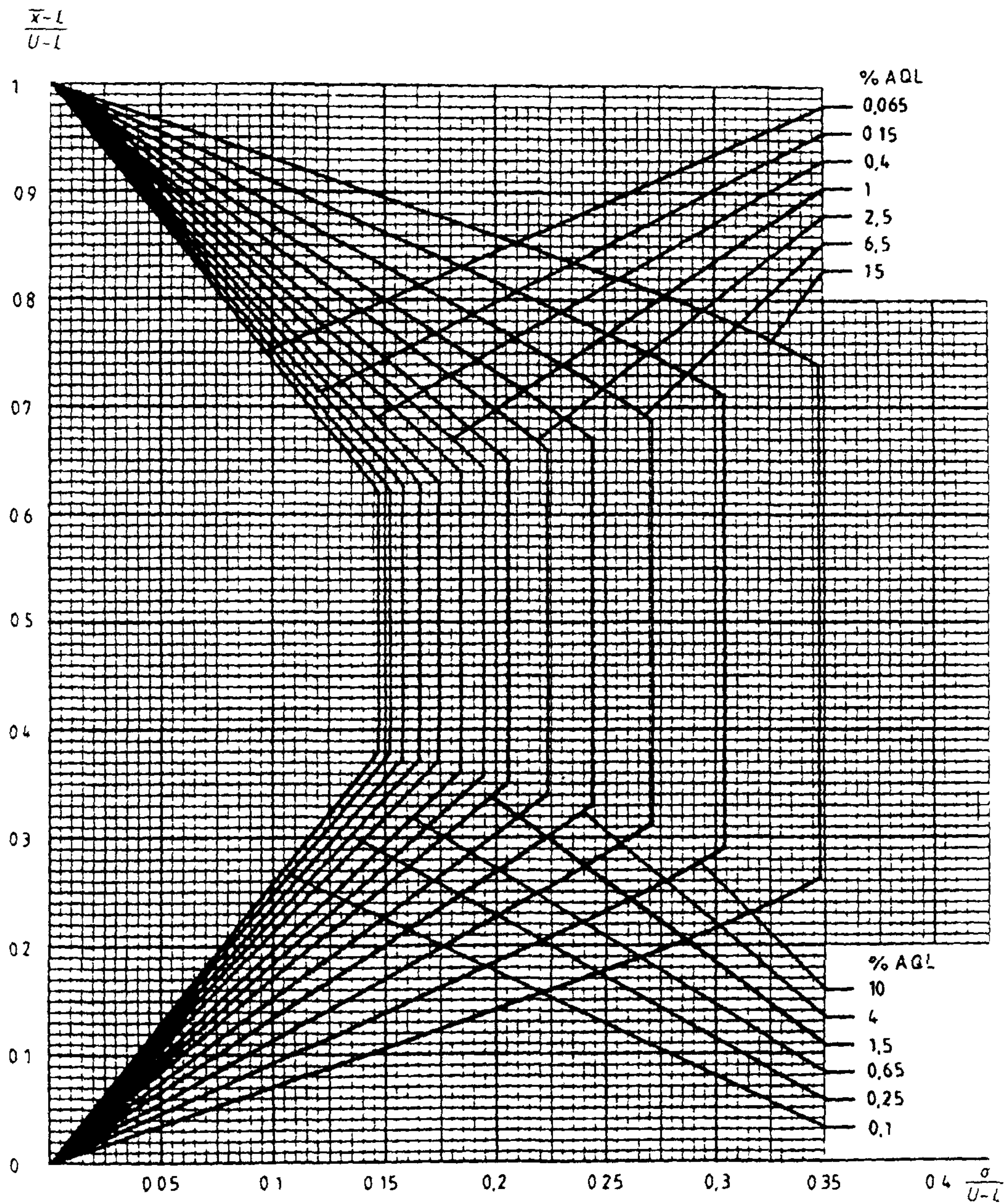
Диаграмма σ-I — Кривые приемки для предельных значений с общим уровнем качества. σ-метод для кода объема выборки J
