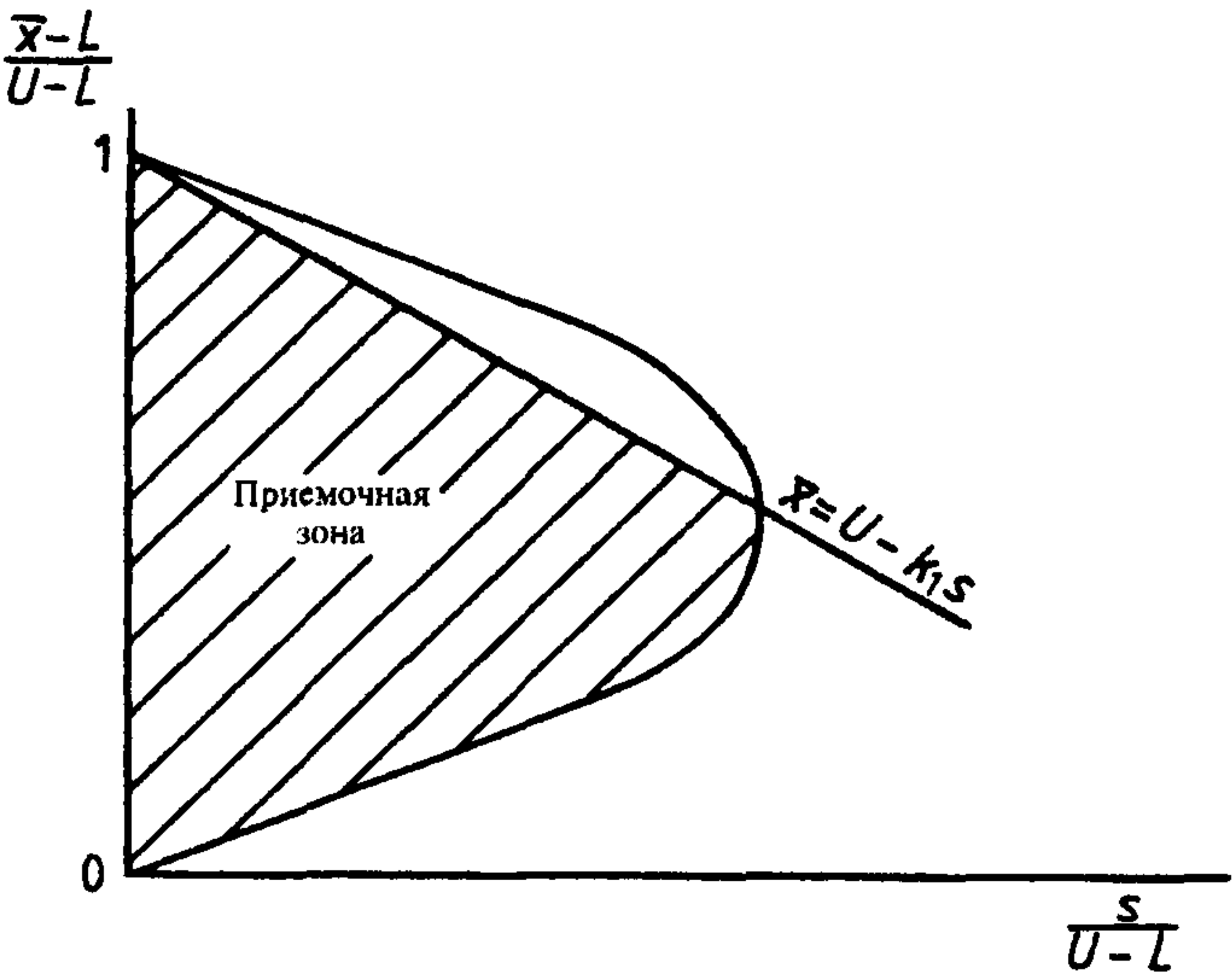
Рисунок 15 — Карта приемки для комбинированных пределов поля допуска (s-метод)
