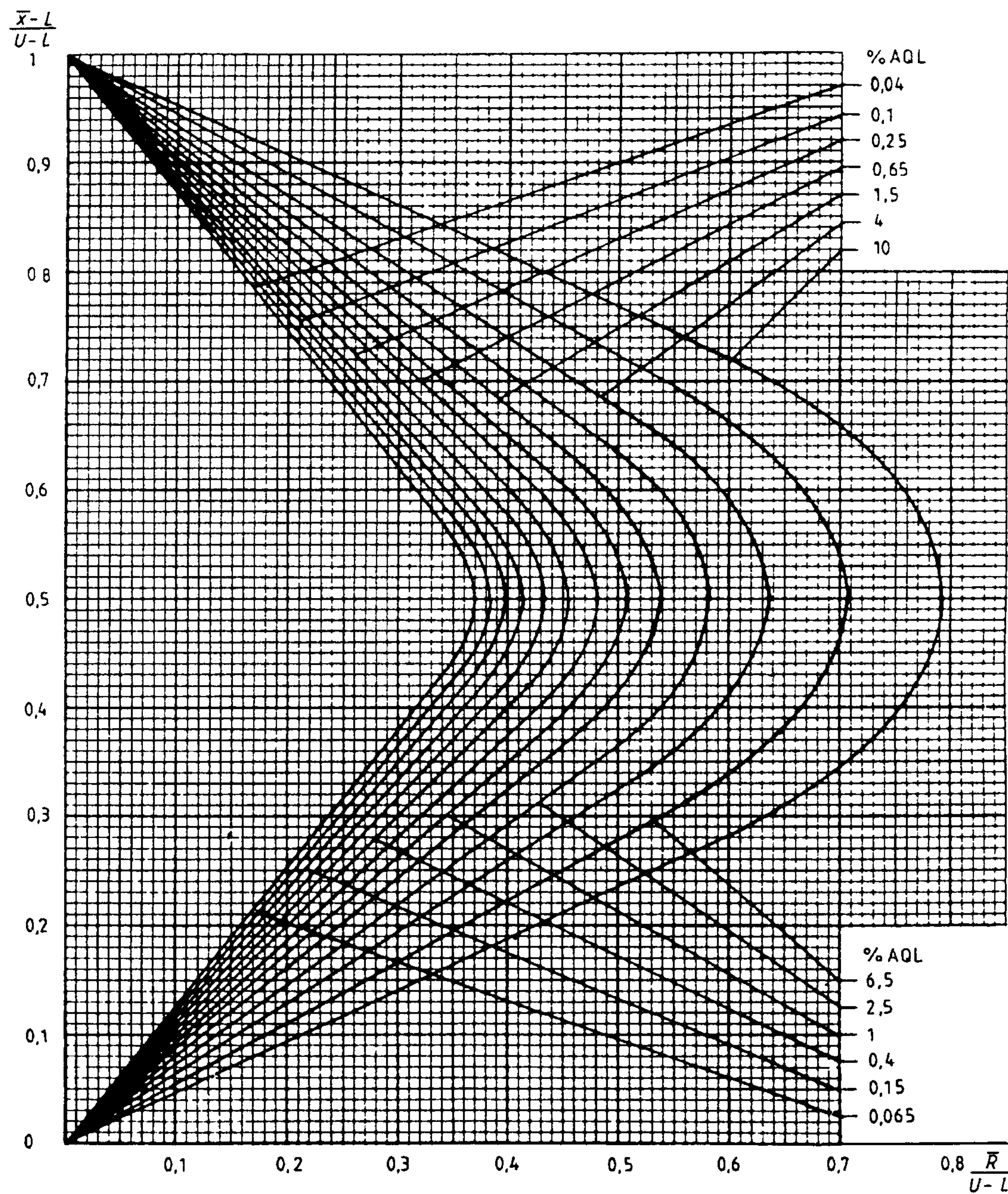
Диаграмма R-P — Кривые приемки для предельных значений с общим уровнем качества R-метод для кода объема выборки Р (объем выборки — 230)
