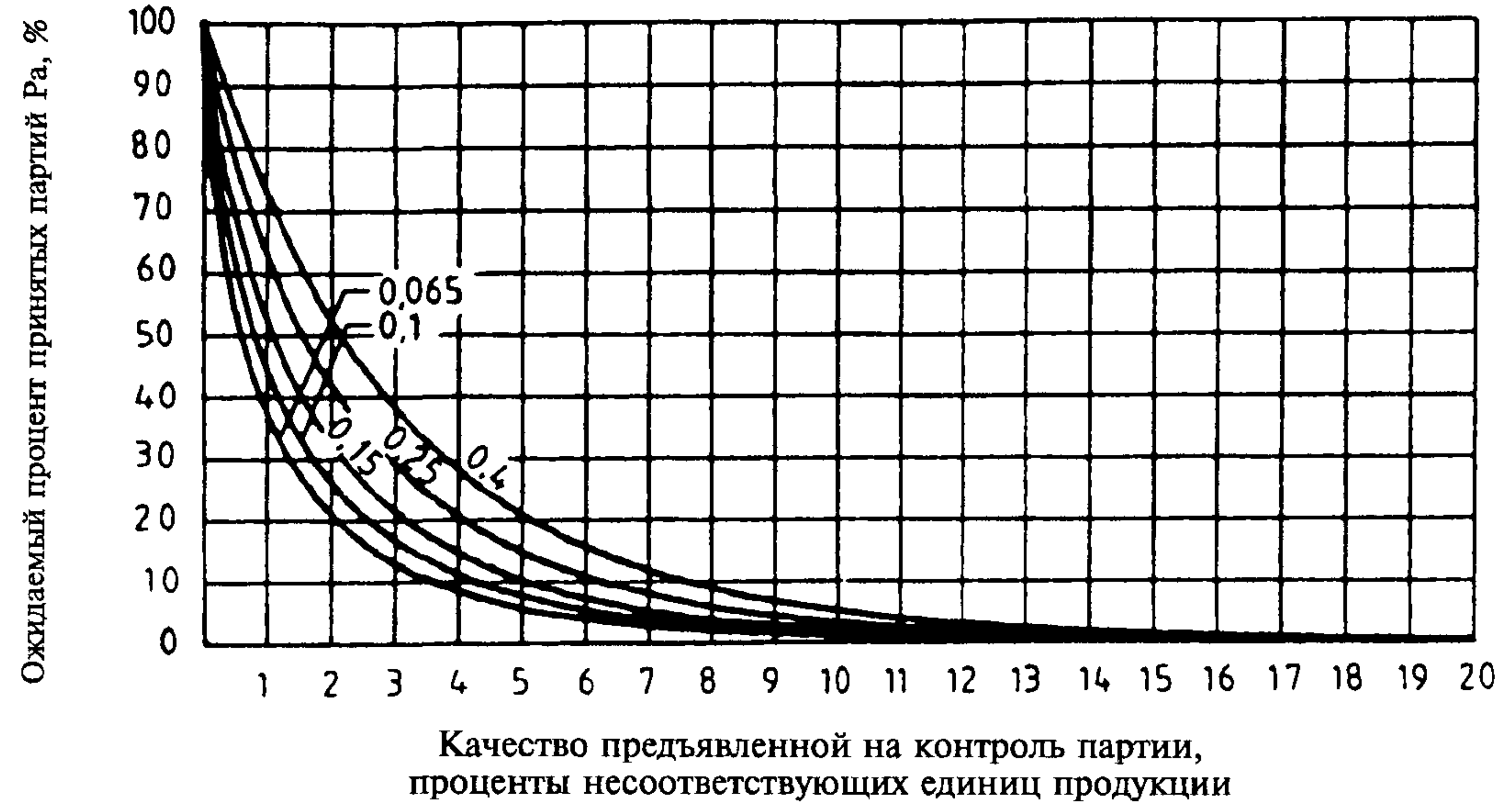
График VG — Оперативные характеристики для одноступенчатых выборочных планов контроля
