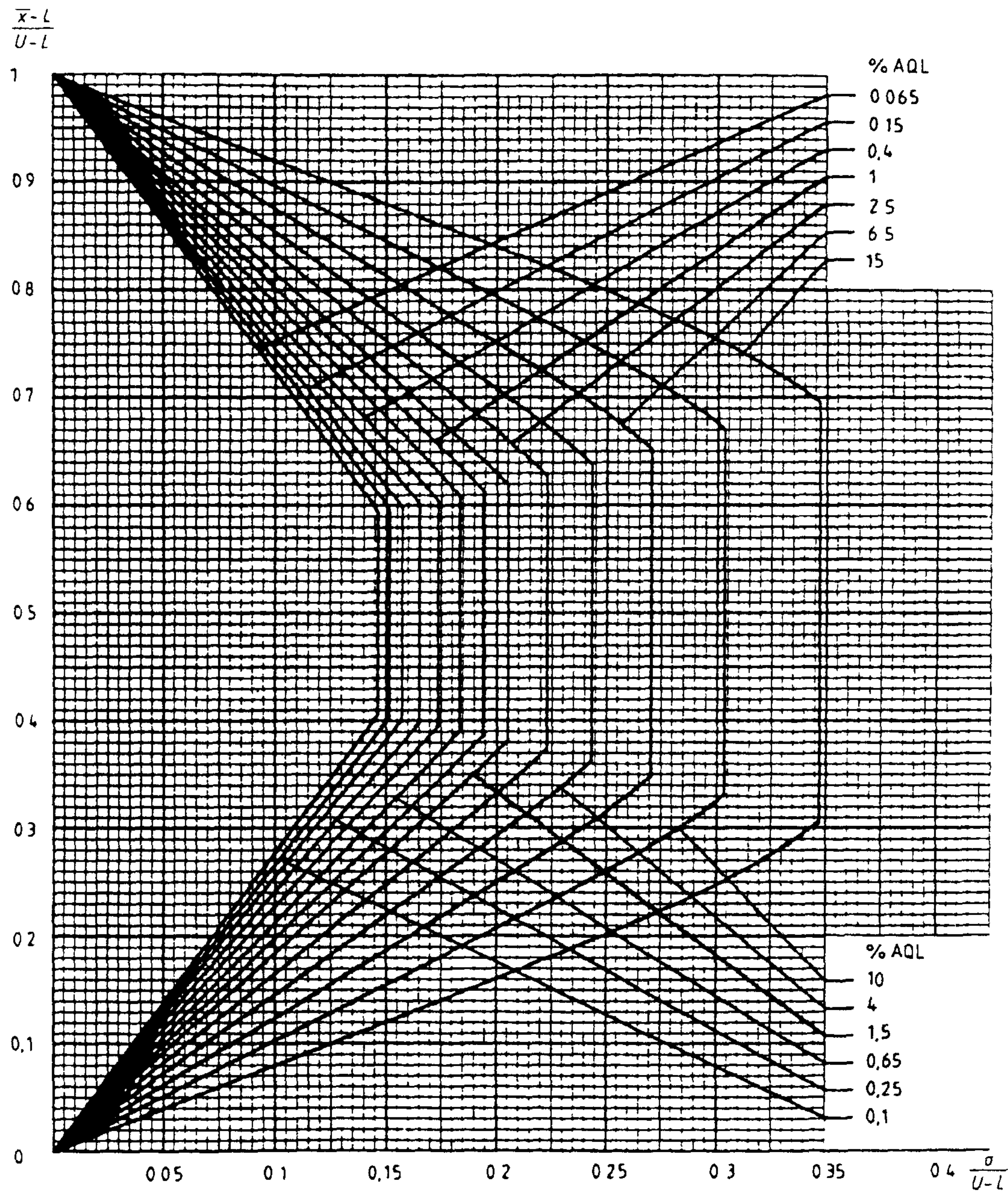
Диаграмма \sigma -L — Кривые приемки для предельных значений с общим уровнем качества \sigma -метод для кода объема выборки L
