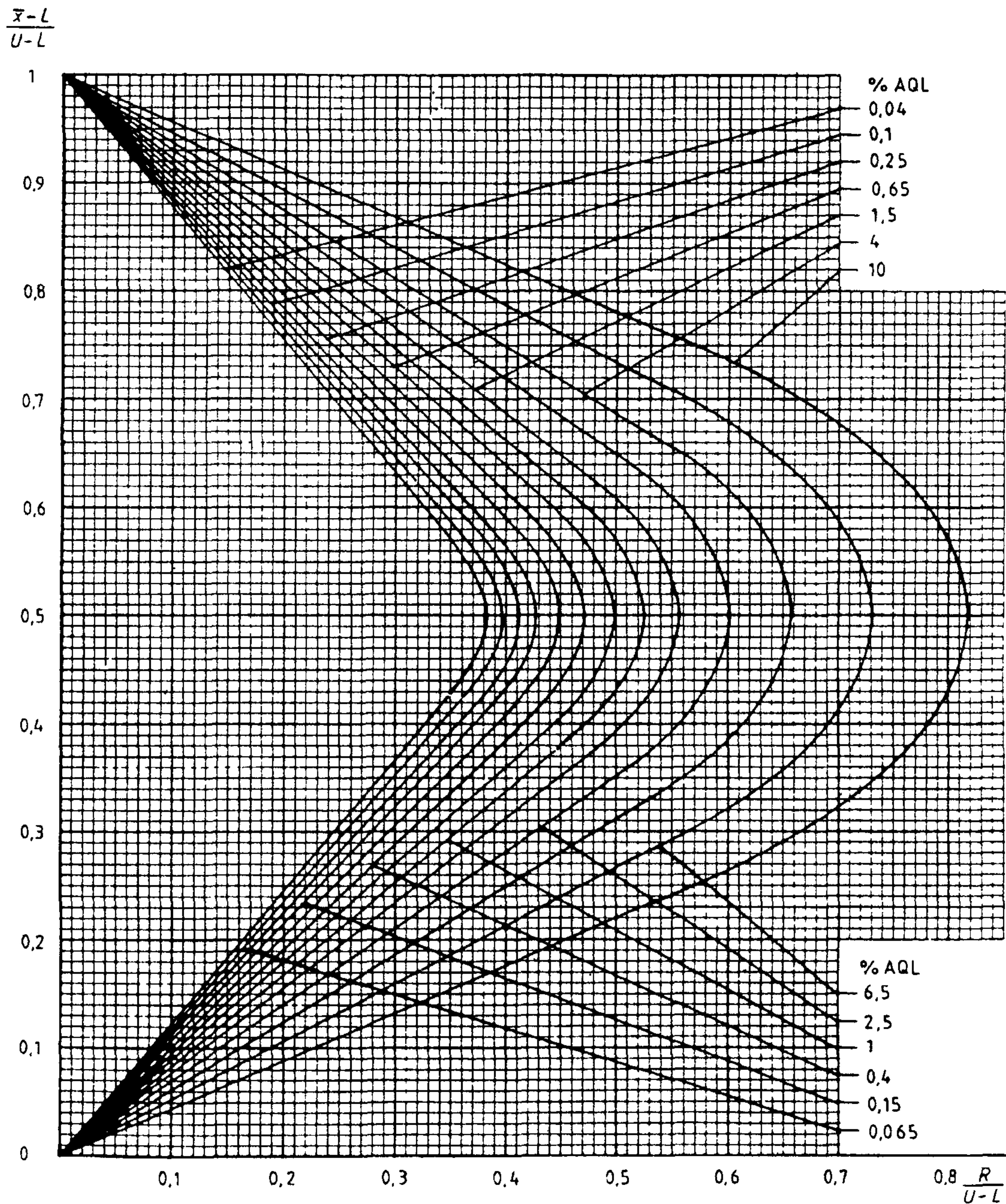
Диаграмма R-L — Кривые приемки для предельных значений с общим уровнем качества: R-метод для кода объема выборки L (объем выборки — 85)
