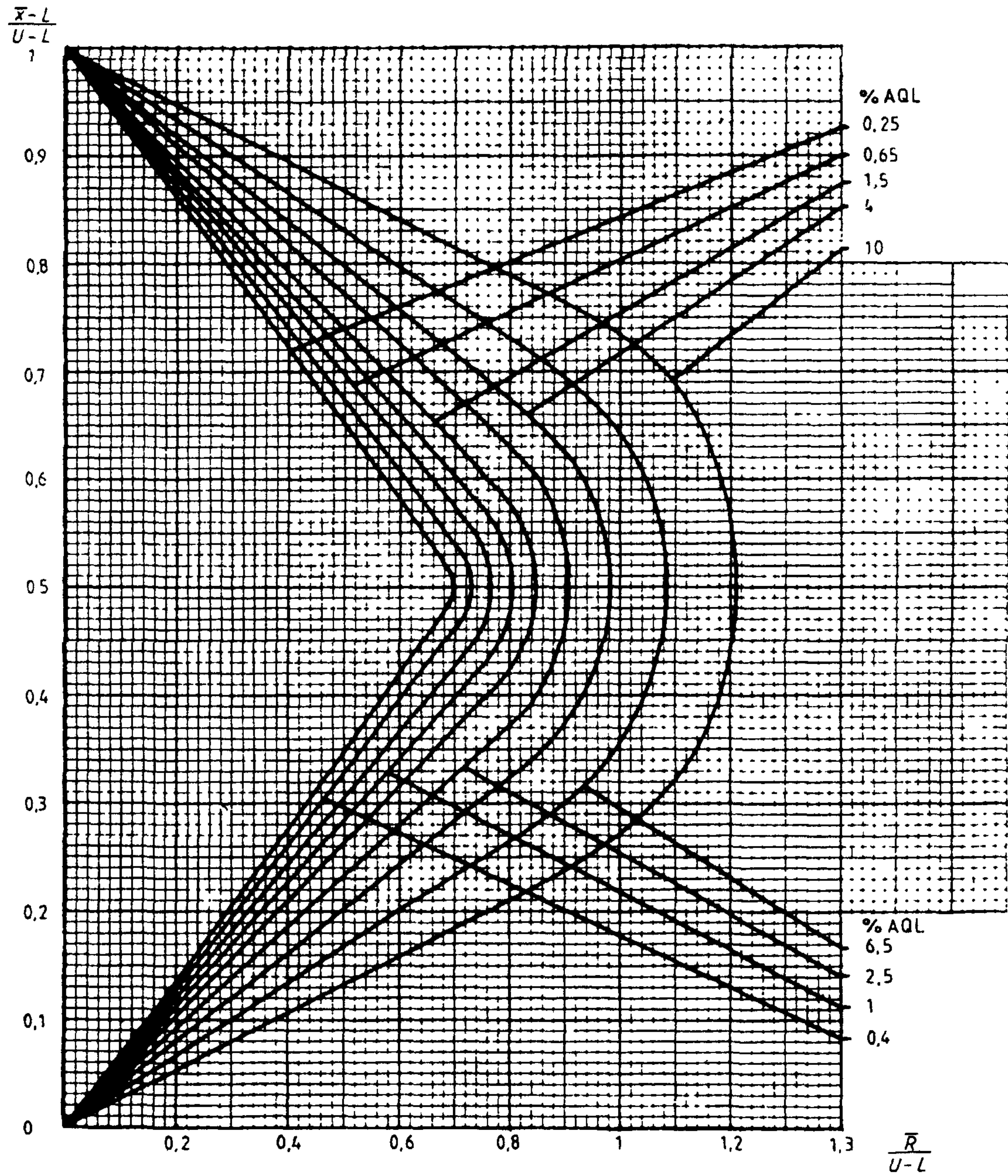
Диаграмма R-E — Кривые приемки для предельных значений с общим уровнем качества: R-метод для кода объема выборки E (объем выборки — 7)
