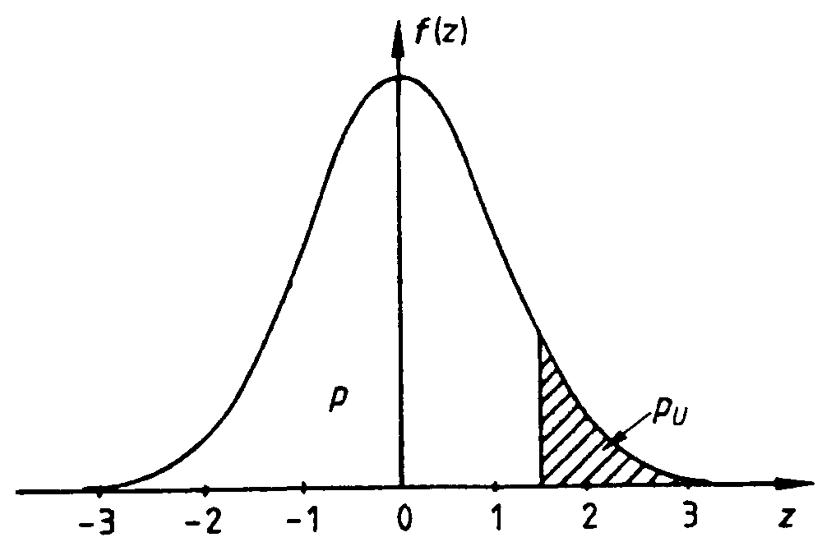
Рисунок 6 — Стандартное нормальное распределение
