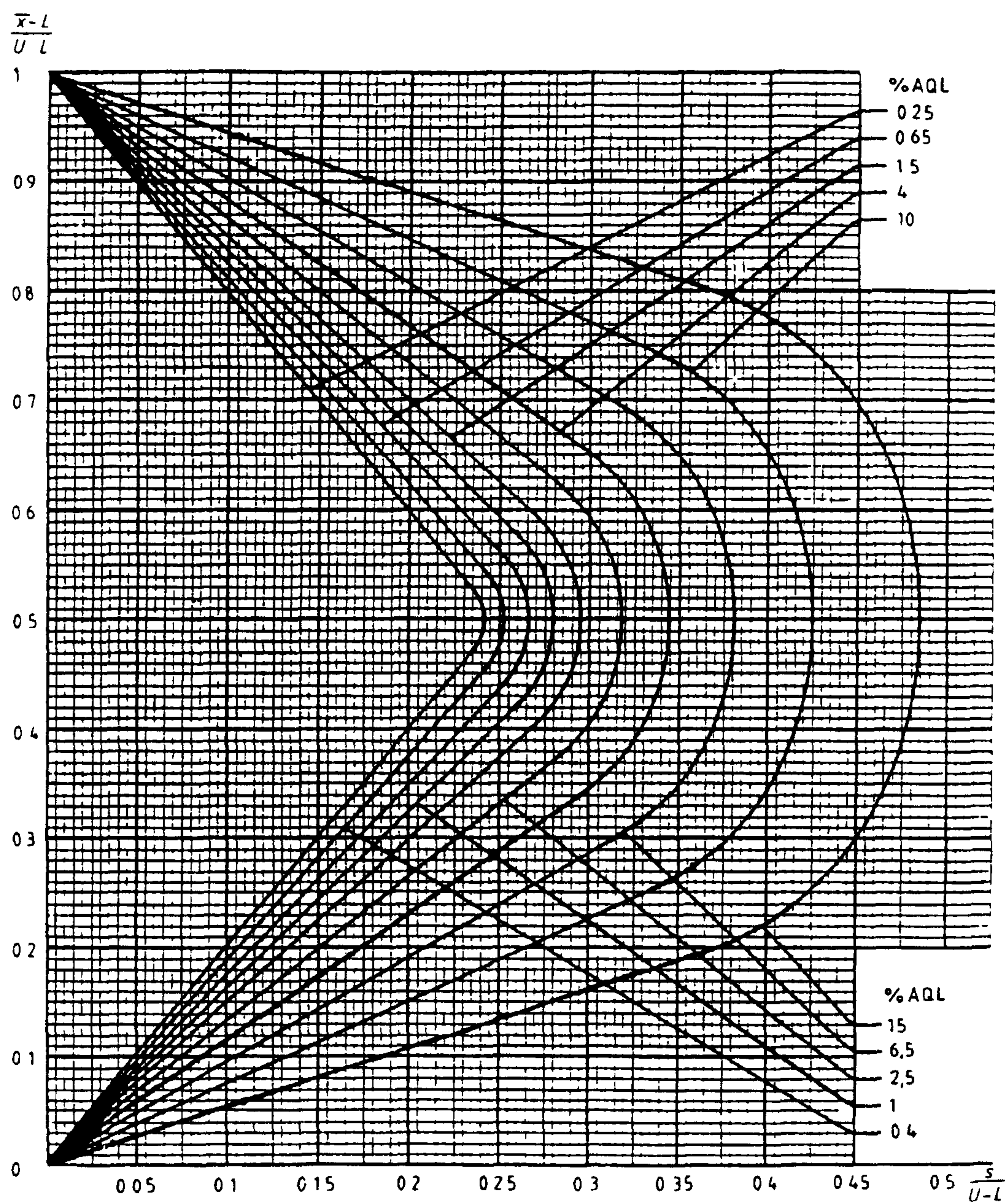
иаграмма s-E — Кривые приемки для предельных значений с общим уровнем качества s-метод для кода объема выборки E (объем выборки — 7)
