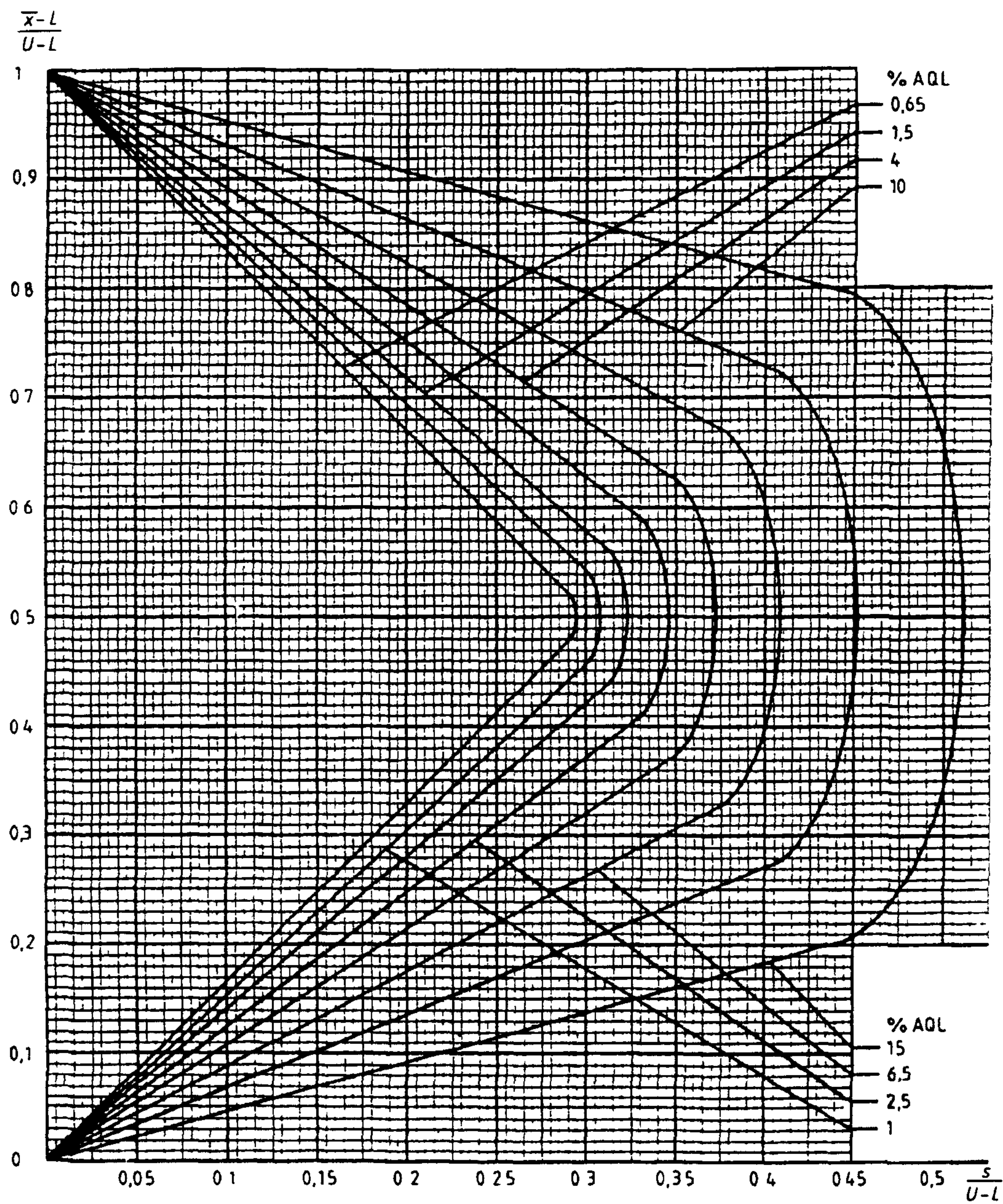
Диаграмма s-D — Кривые приемки для предельных значений с общим уровнем качества. s-метод для кода объема выборки D (объем выборки — 5)
