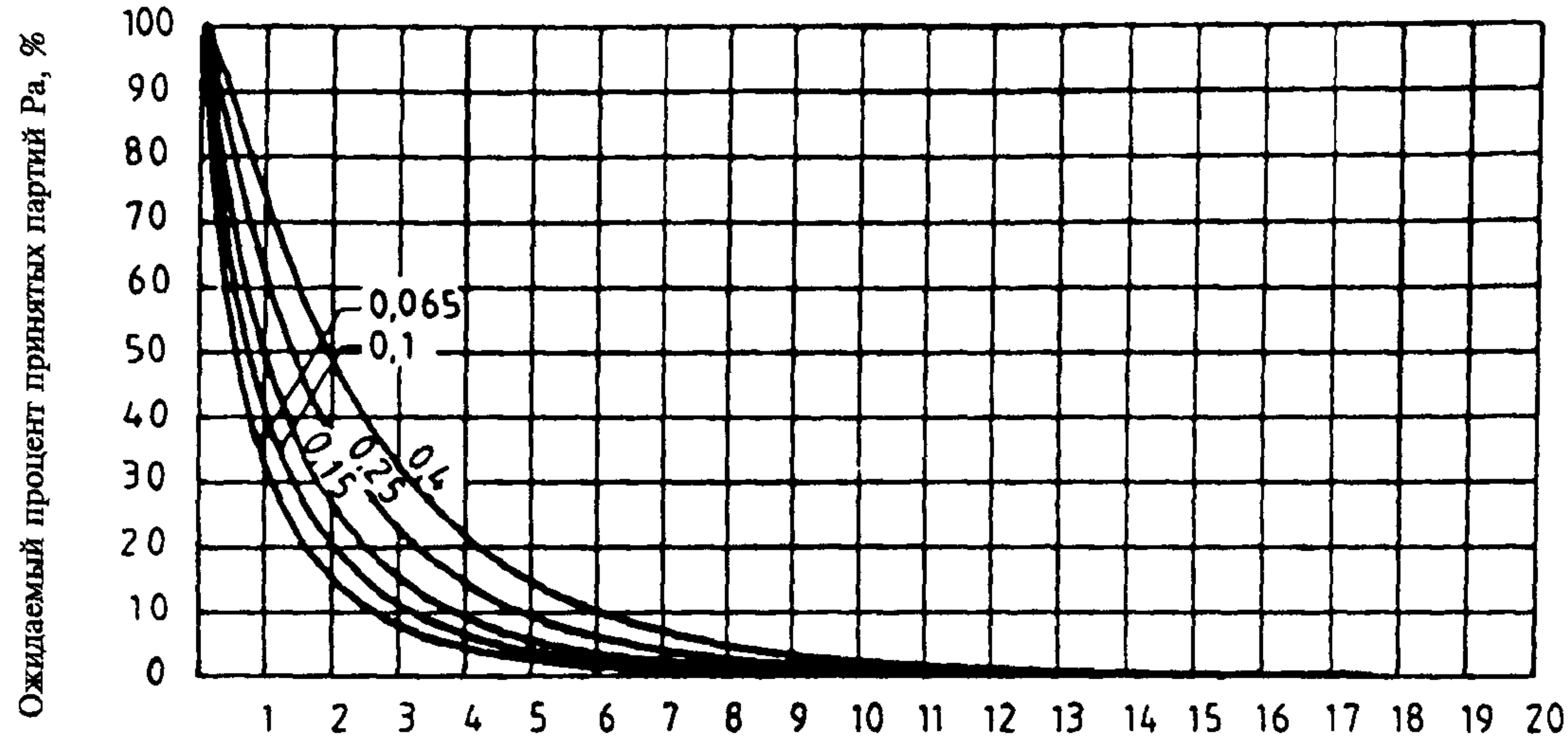
График VN — Оперативные характеристики для одноступенчатых выборочных планов контроля
