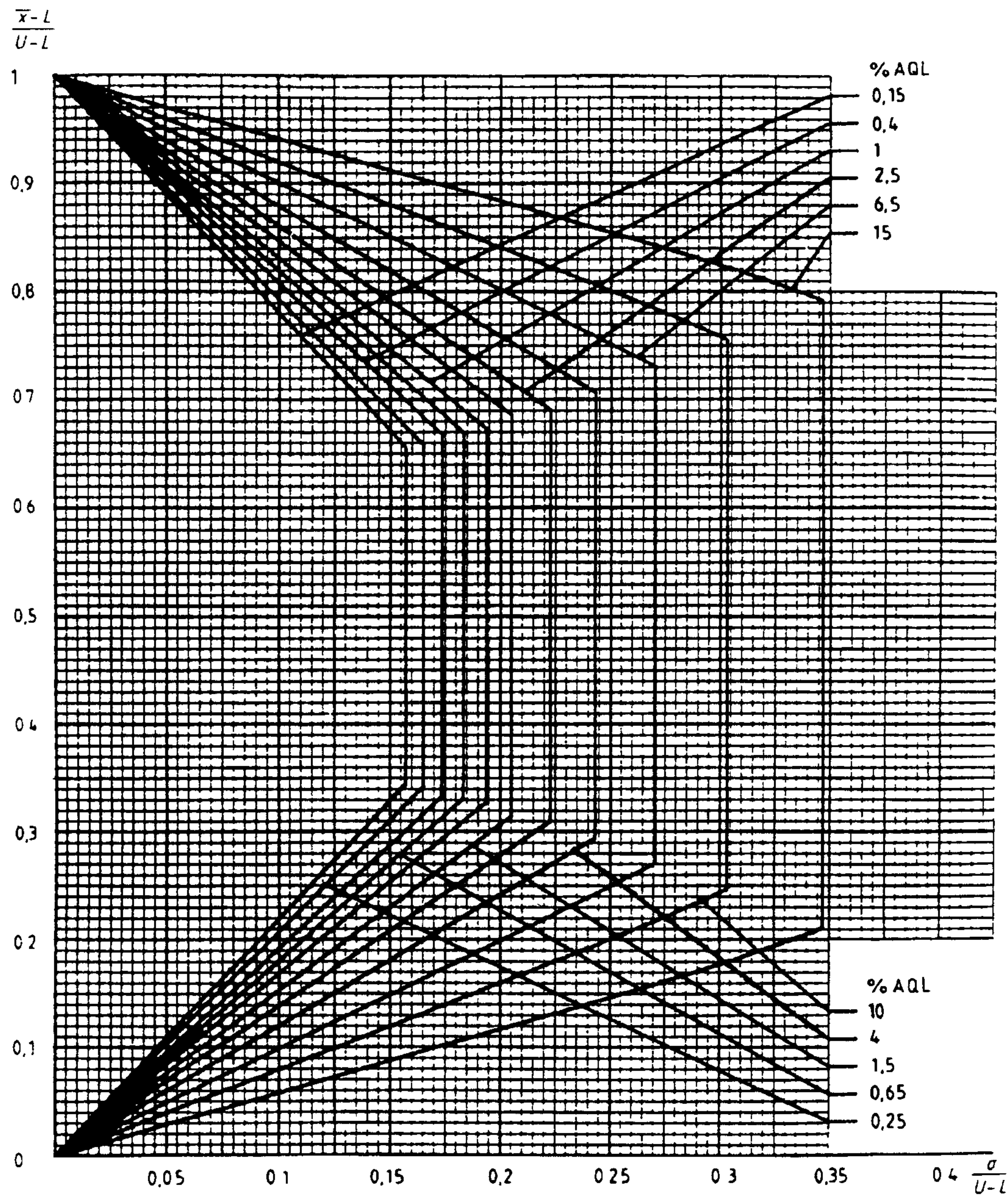
Диаграмма σ-F — Кривые приемки для предельных значений с общим уровнем качества: σ-метод для кода объема выборки F
