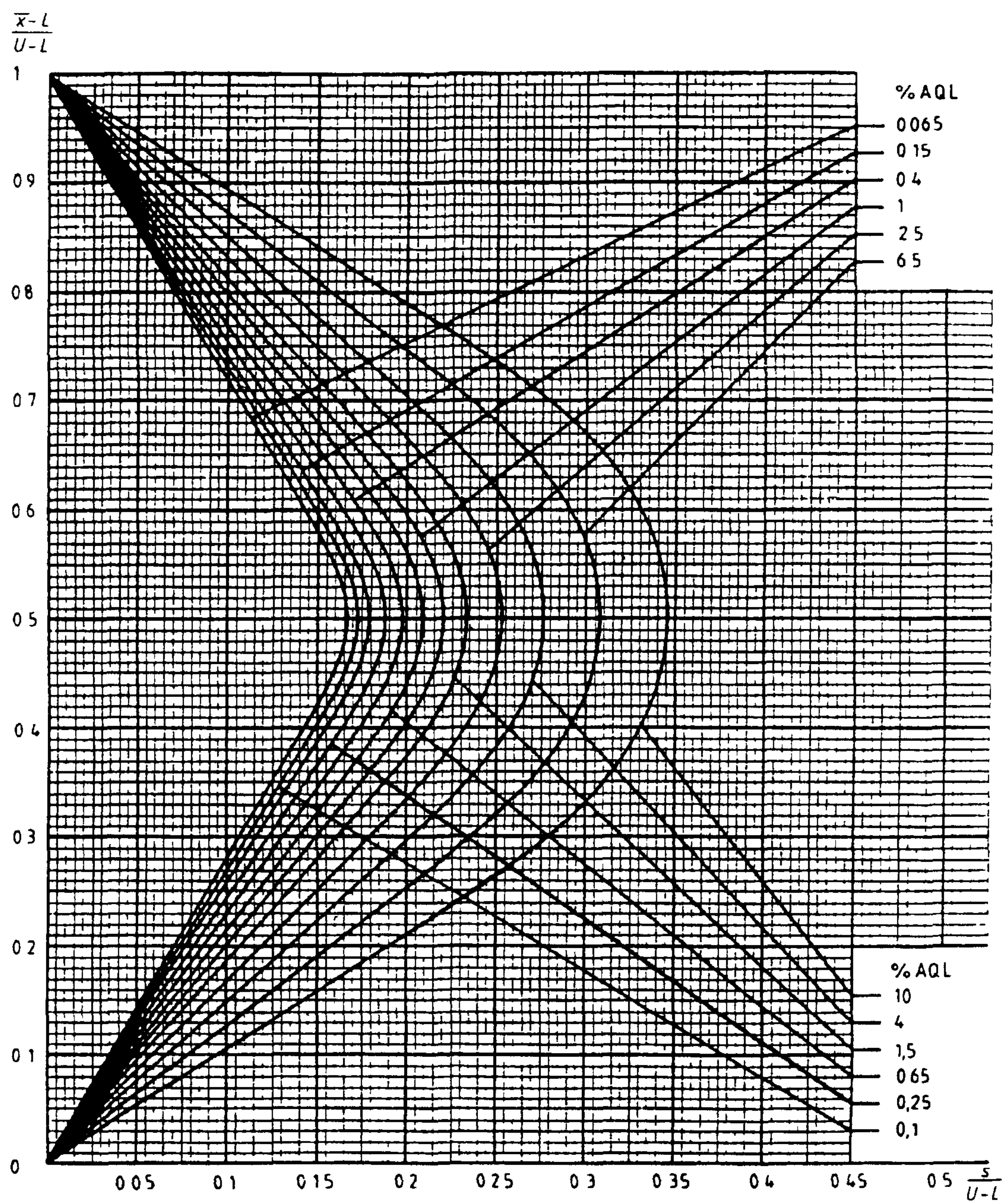
Диаграмма s-M — Кривые приемки для предельных значений с общим уровнем качества. s-метод для кода объема выборки M (объем выборки — 100)
