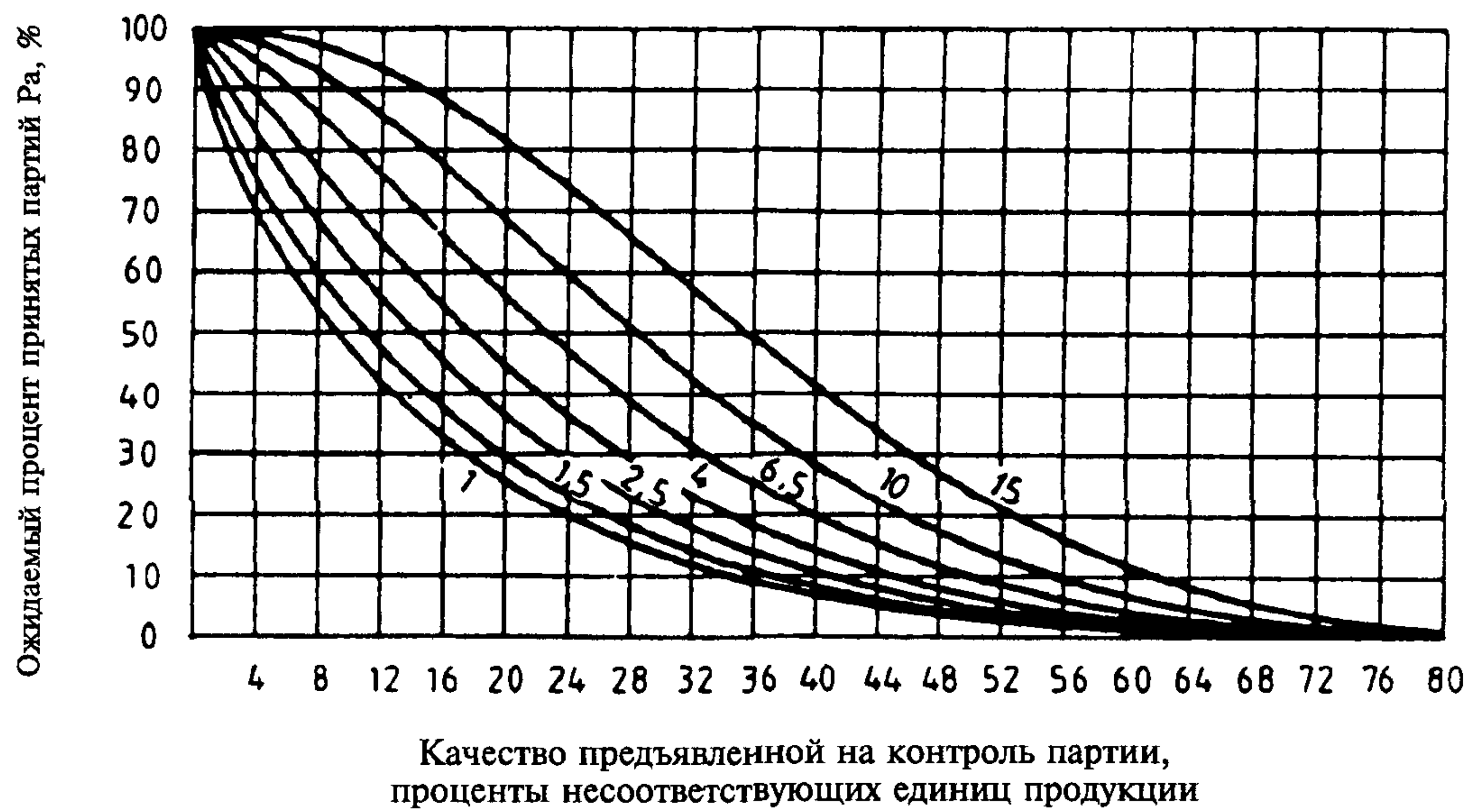
График VC — Оперативные характеристики для одноступенчатых выборочных планов контроля
