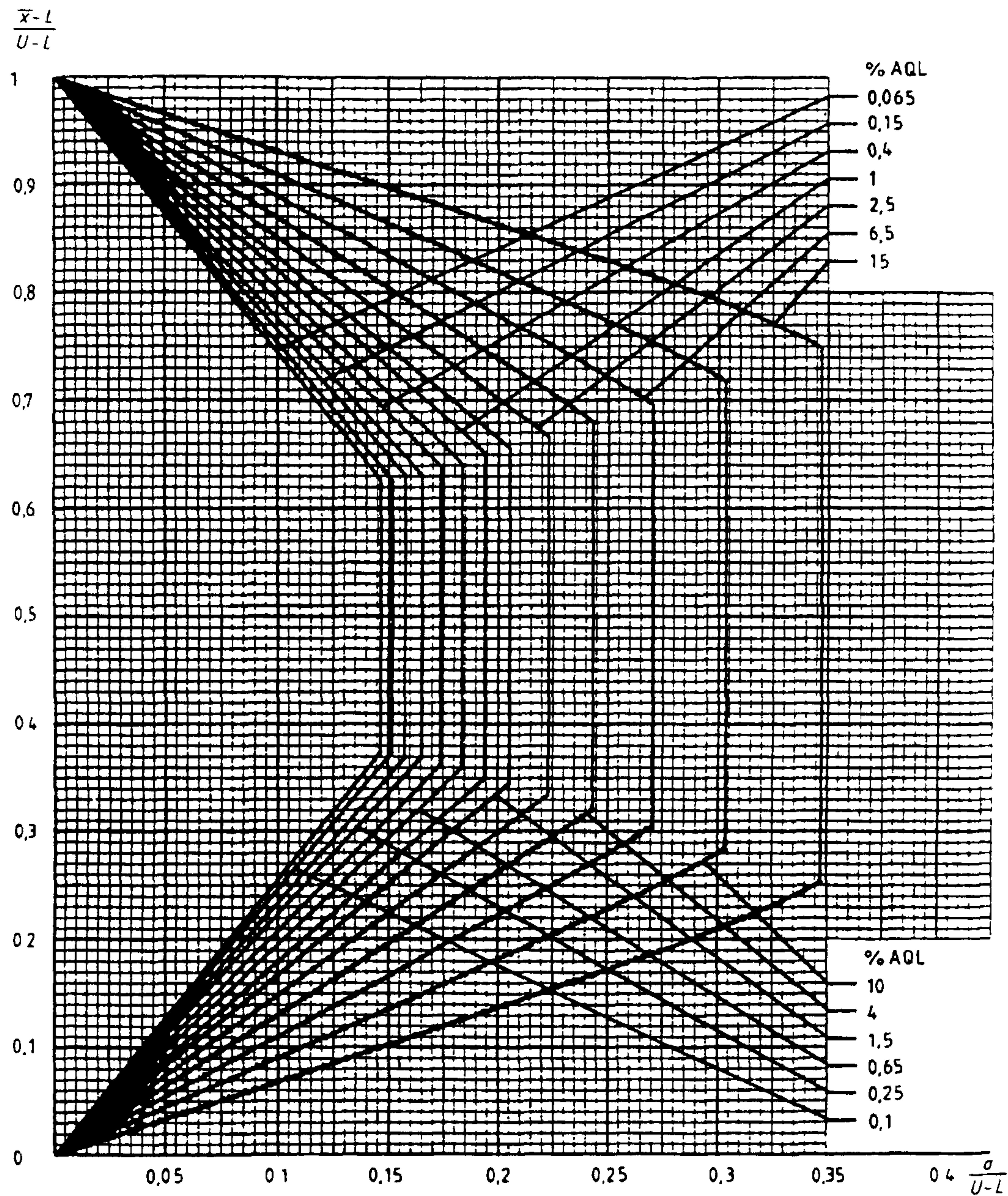
Диаграмма \sigma -Н — Кривые приемки для предельных значений с общим уровнем качества: \sigma -метод для кода объема выборки Н
