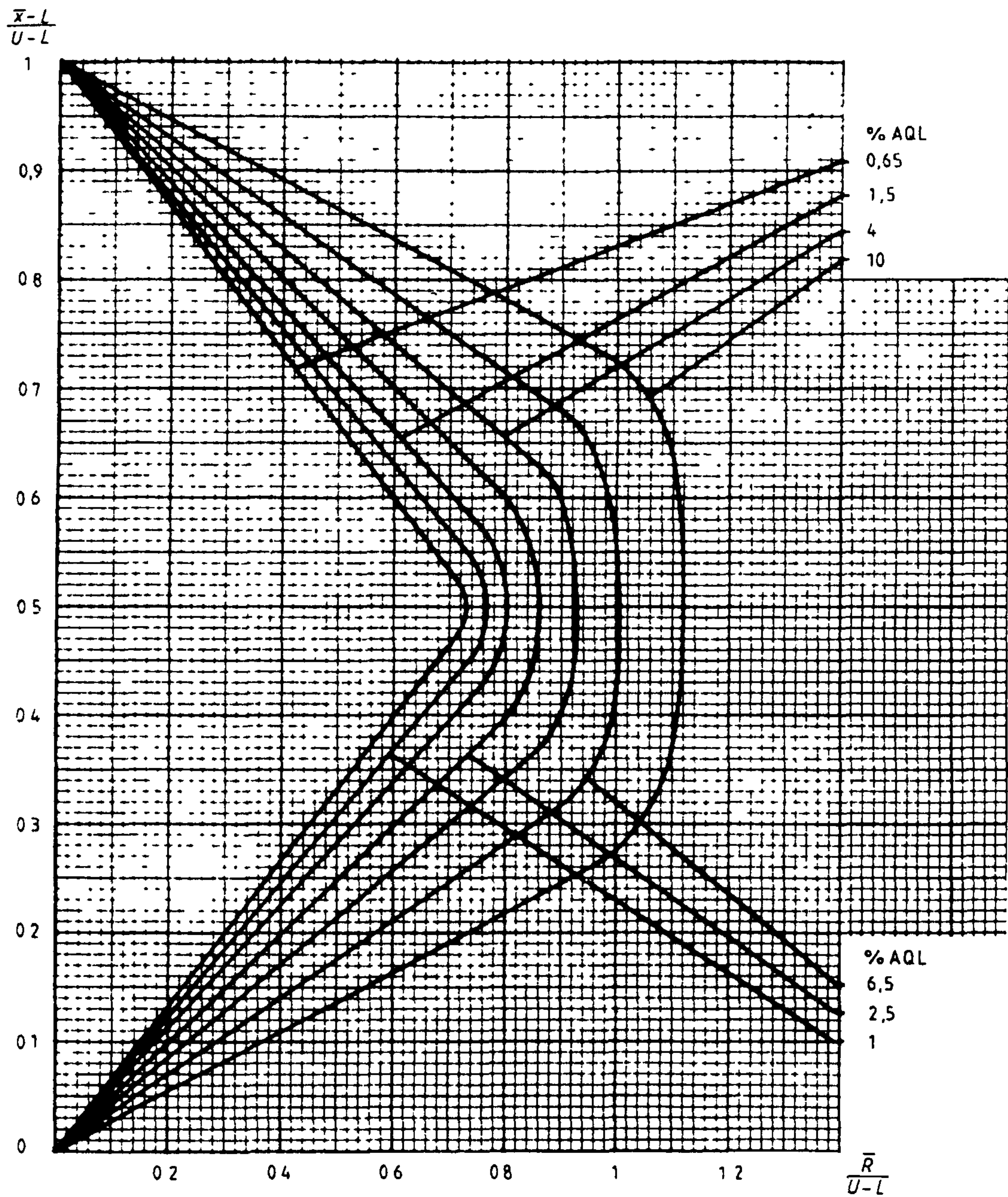
Диаграмма R-D — Кривые приемки для предельных значений с общим уровнем качества R-метод для кода объема выборки D (объем выборки — 5)
