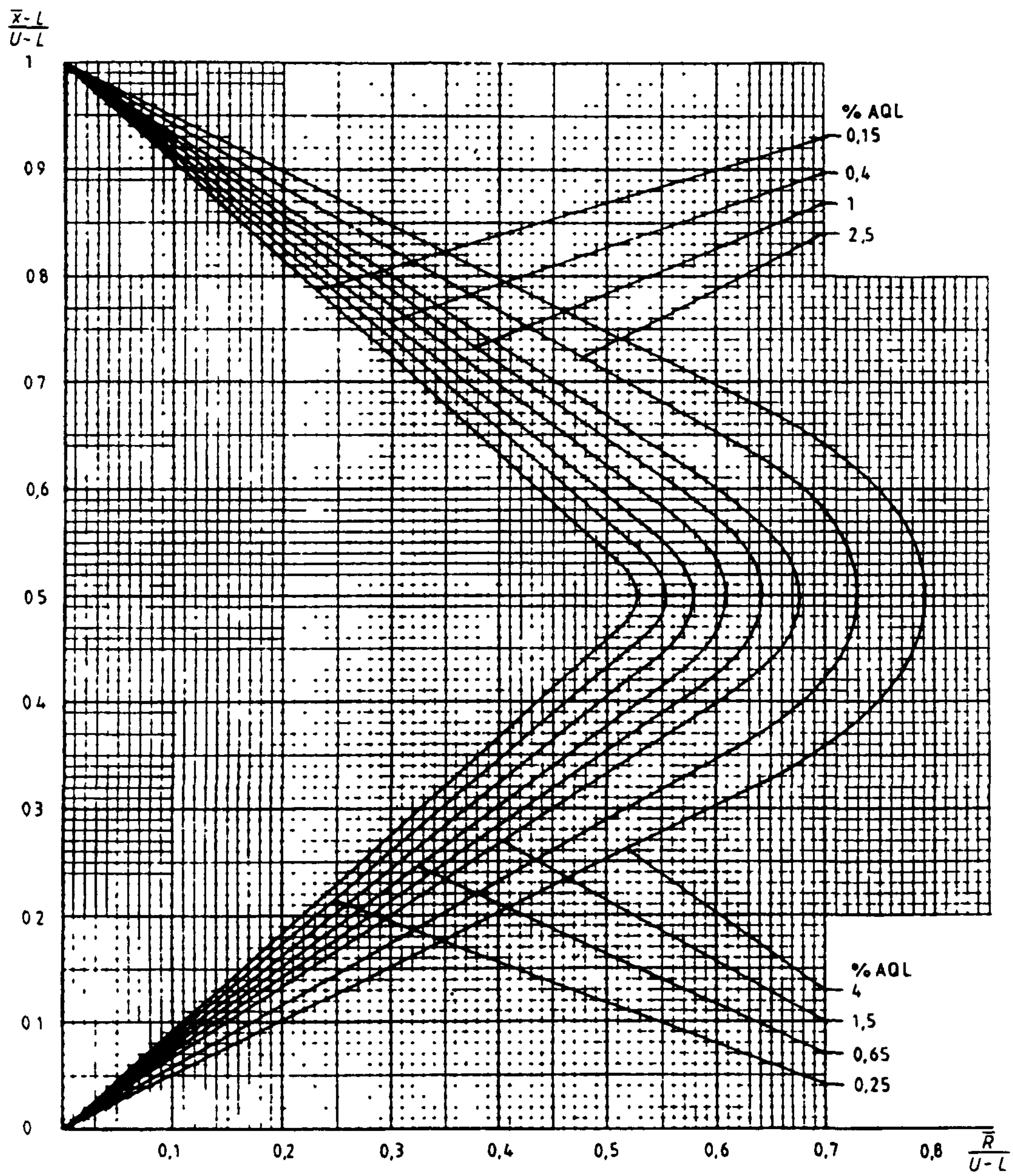
Диаграмма R-F — Кривые приемки для предельных значений с общим уровнем качества R-метод для кода объема выборки F (объем выборки — 10)
