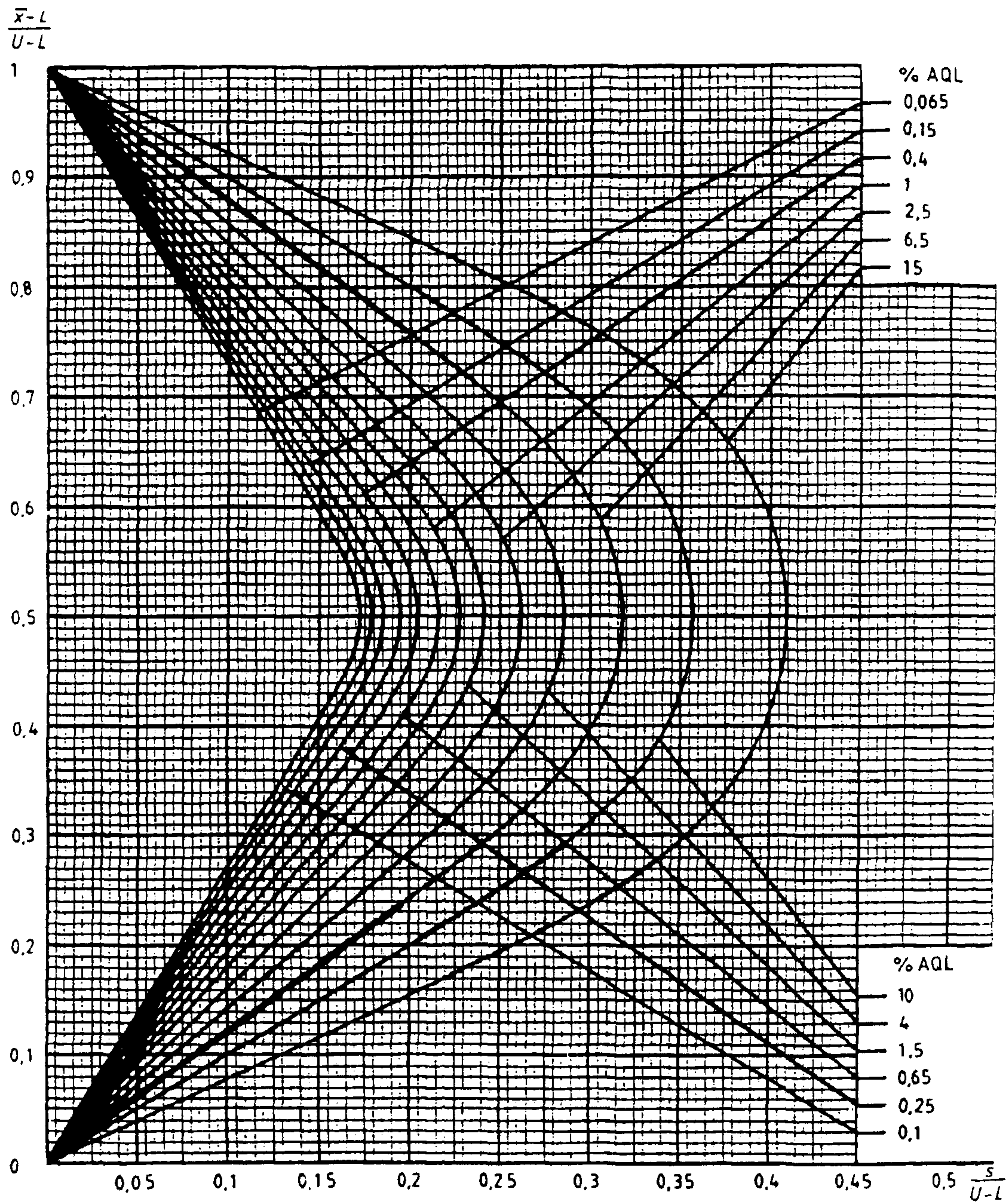
Диаграмма s-K — Кривые приемки для предельных значений с общим уровнем качества: s-метод для кода объема выборки K (объем выборки — 50)
