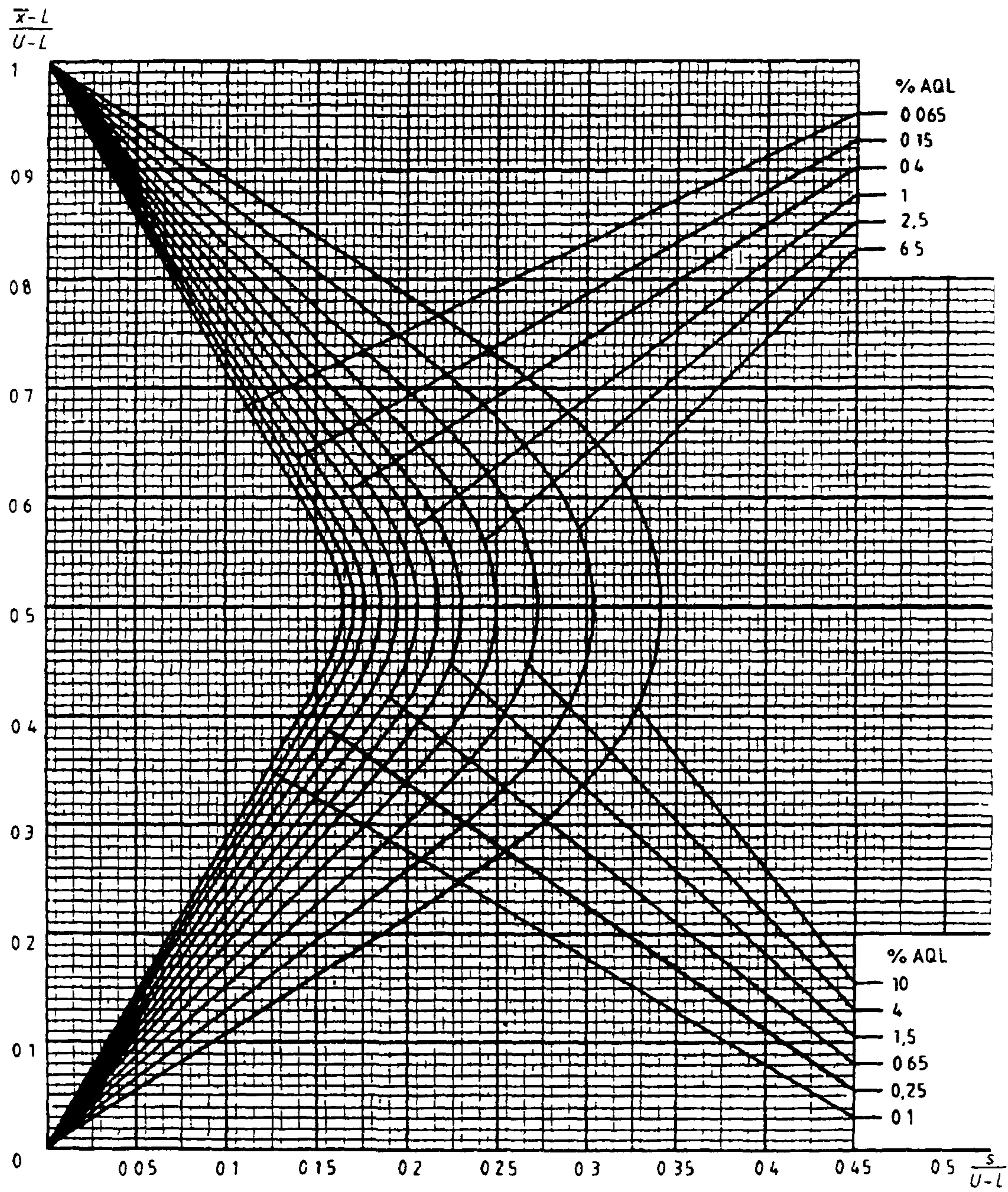
Диаграмма s-N — Кривые приемки для предельных значений с общим уровнем качества s-метод для кода объема выборки N (объем выборки — 150)
