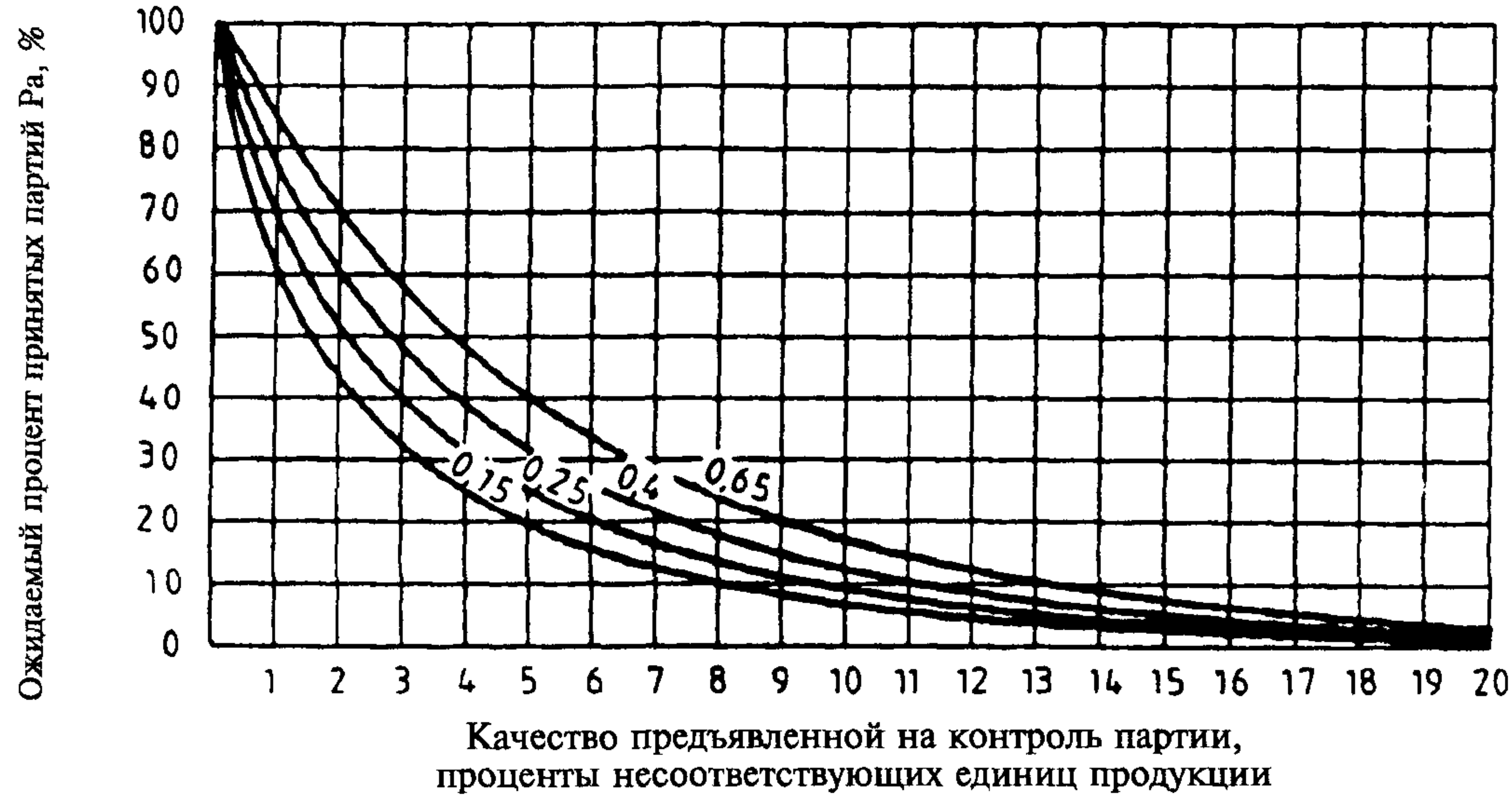
График VF — Оперативные характеристики для одноступенчатых выборочных планов контроля
