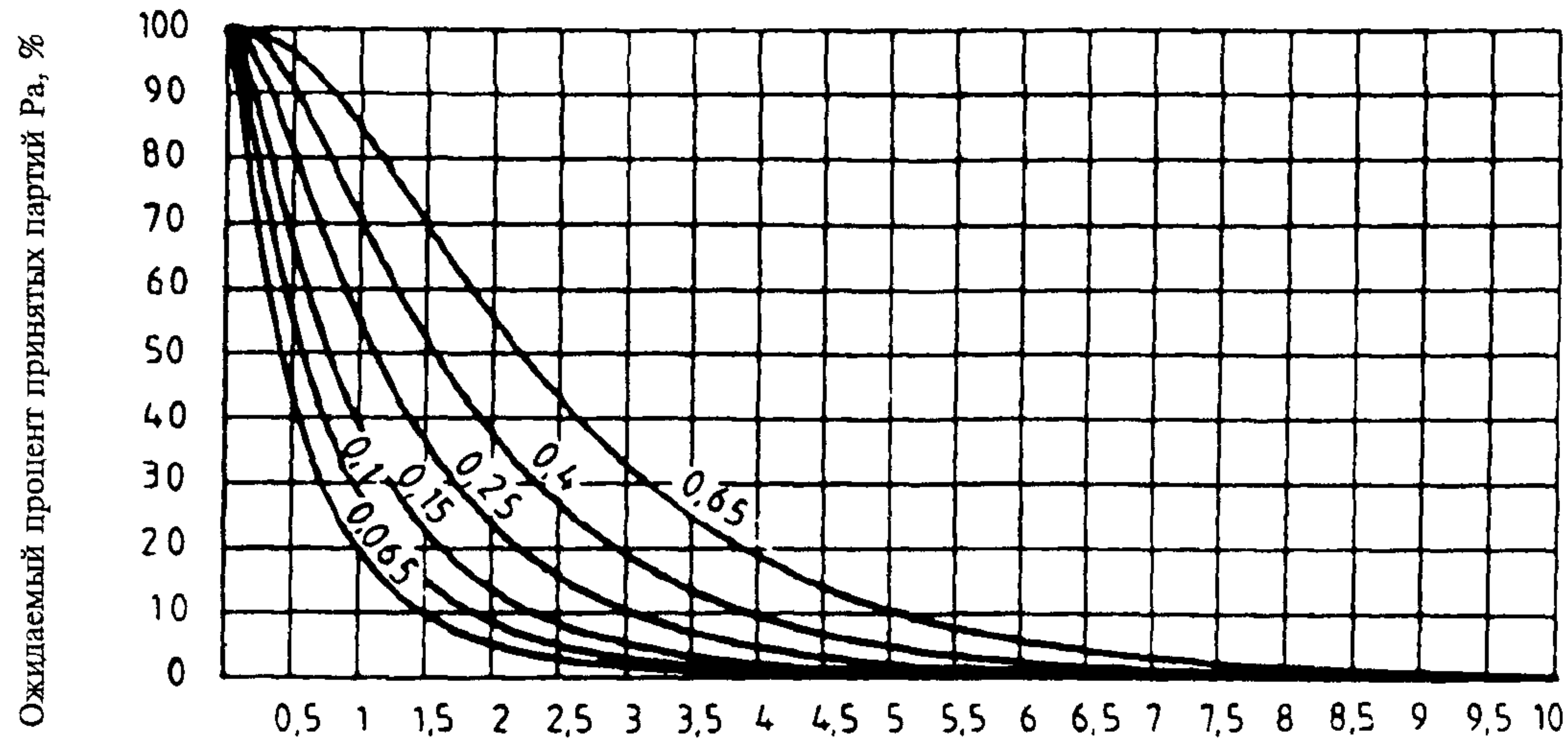
График VJ — Оперативные характеристики для одноступенчатых выборочных планов контроля
