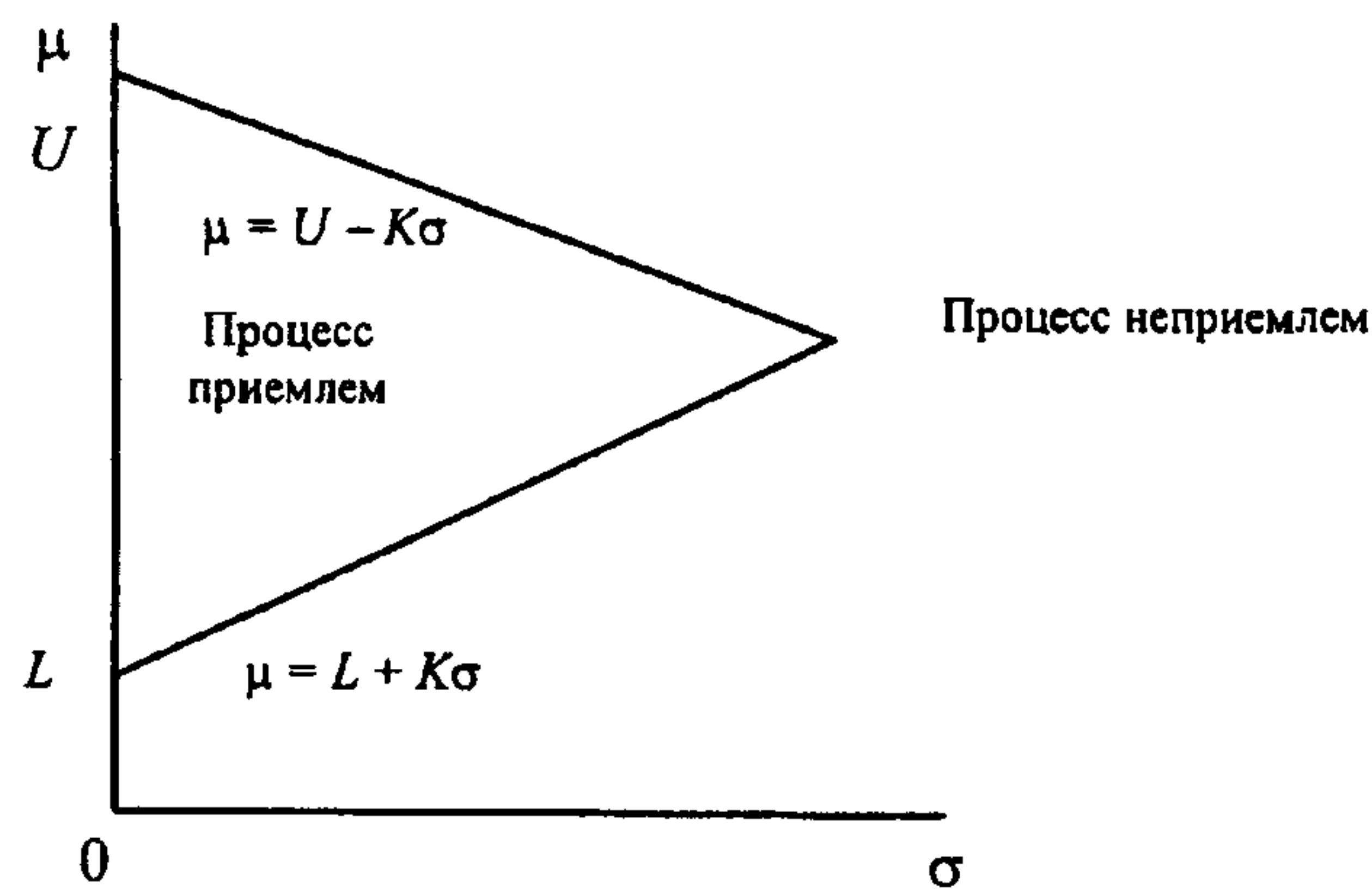
Рисунок 10 — Приемочная карта для двустороннего допуска (σ и μ известны)
