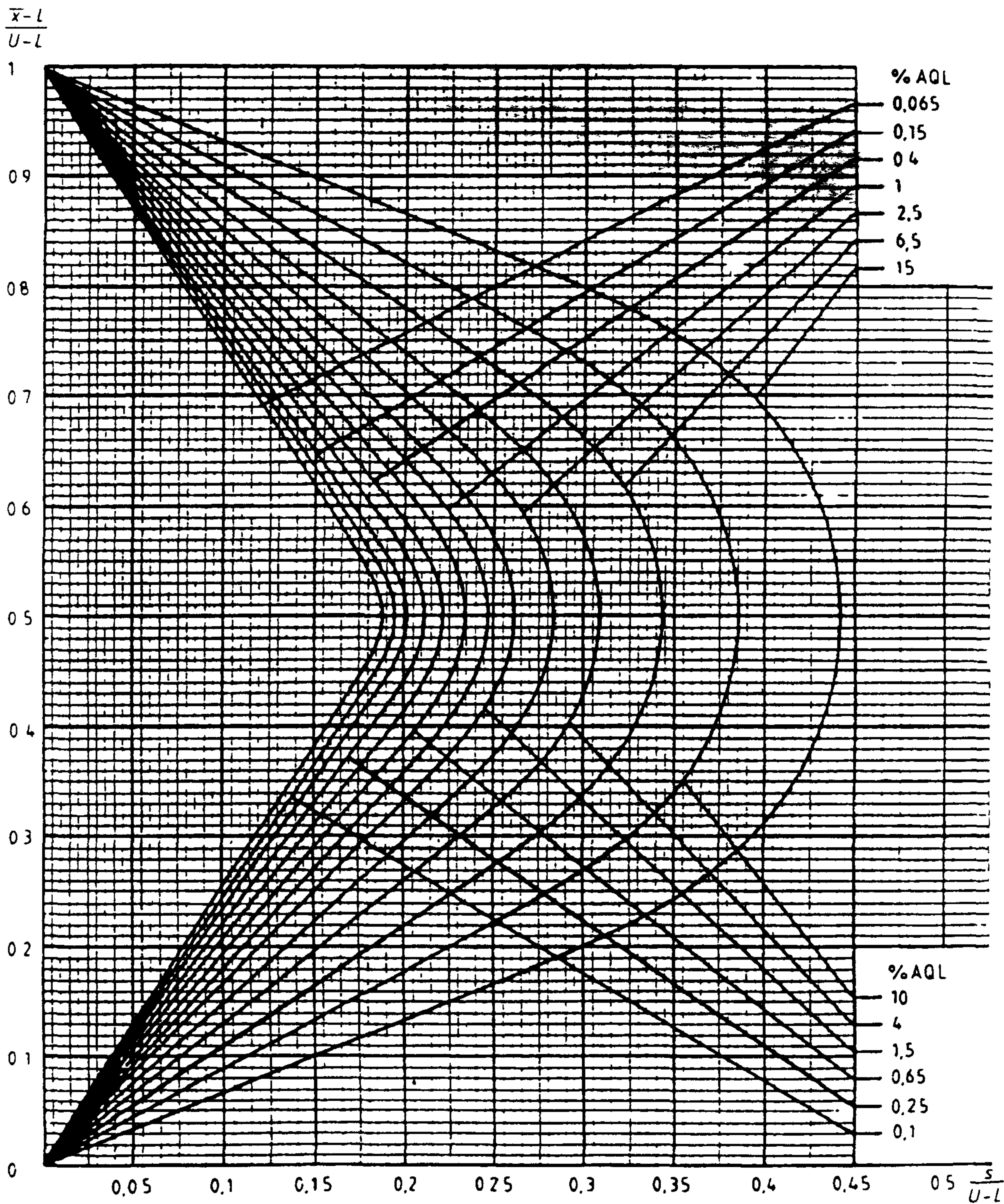
Диаграмма R-G — Кривые приемки для предельных значений с общим уровнем качества R-метод для кода объема выборки G (объем выборки — 15)
