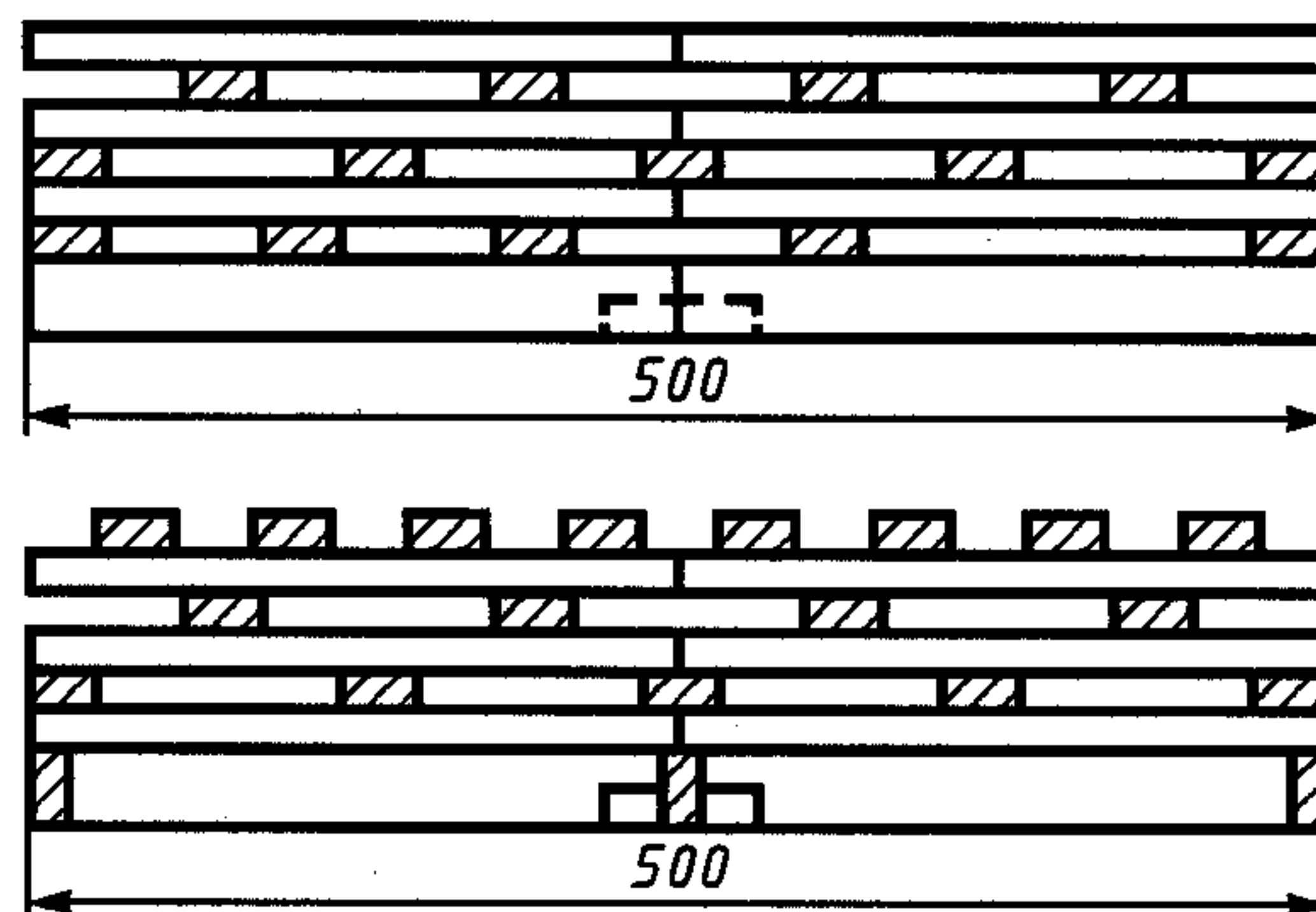
Рисунок Б.1 — Расположение буковых брусков для проведения испытаний
