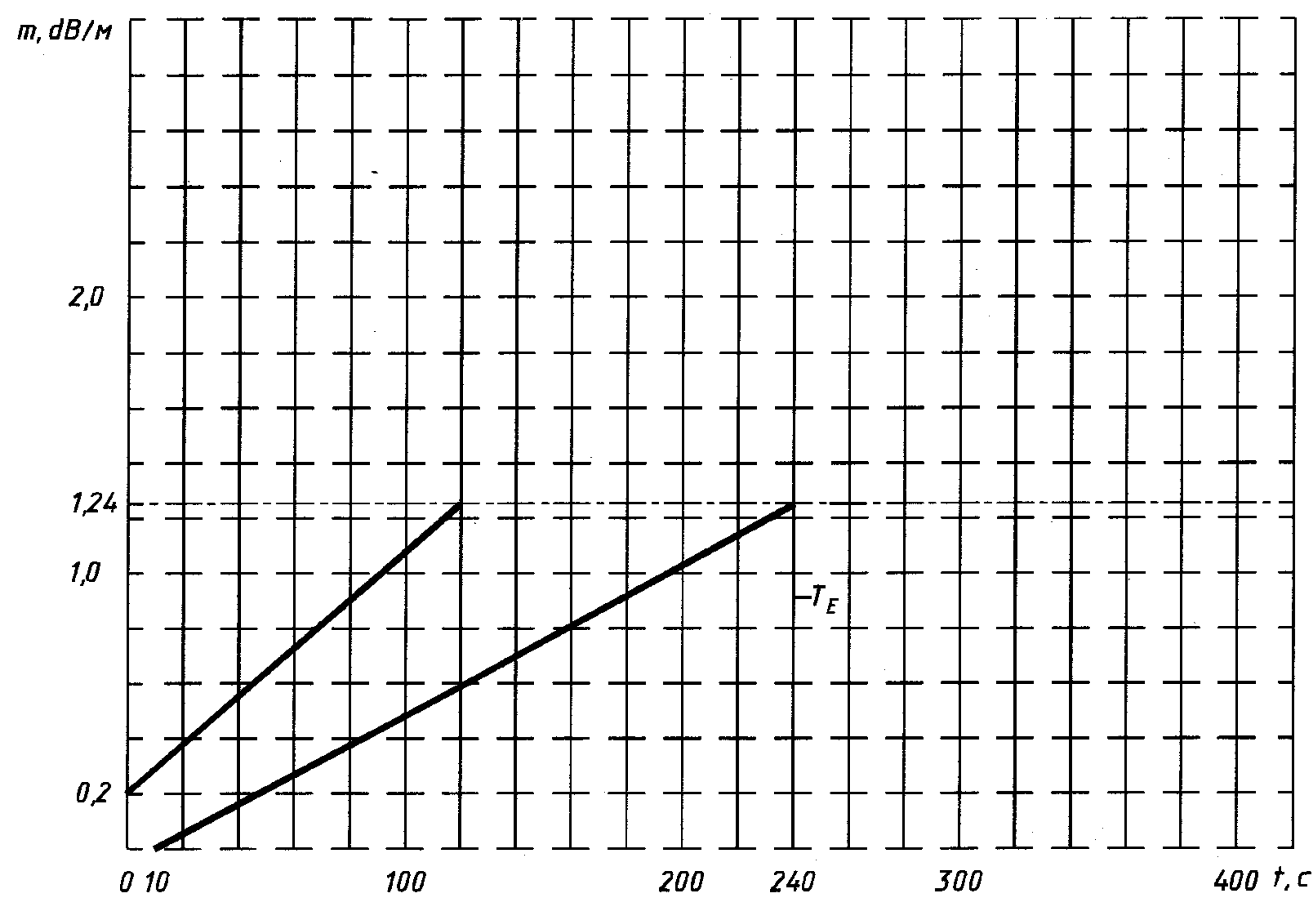
Рисунок Л.9 — Тестовый очаг пожара ТП-5. Зависимость оптической плотности среды от времени
