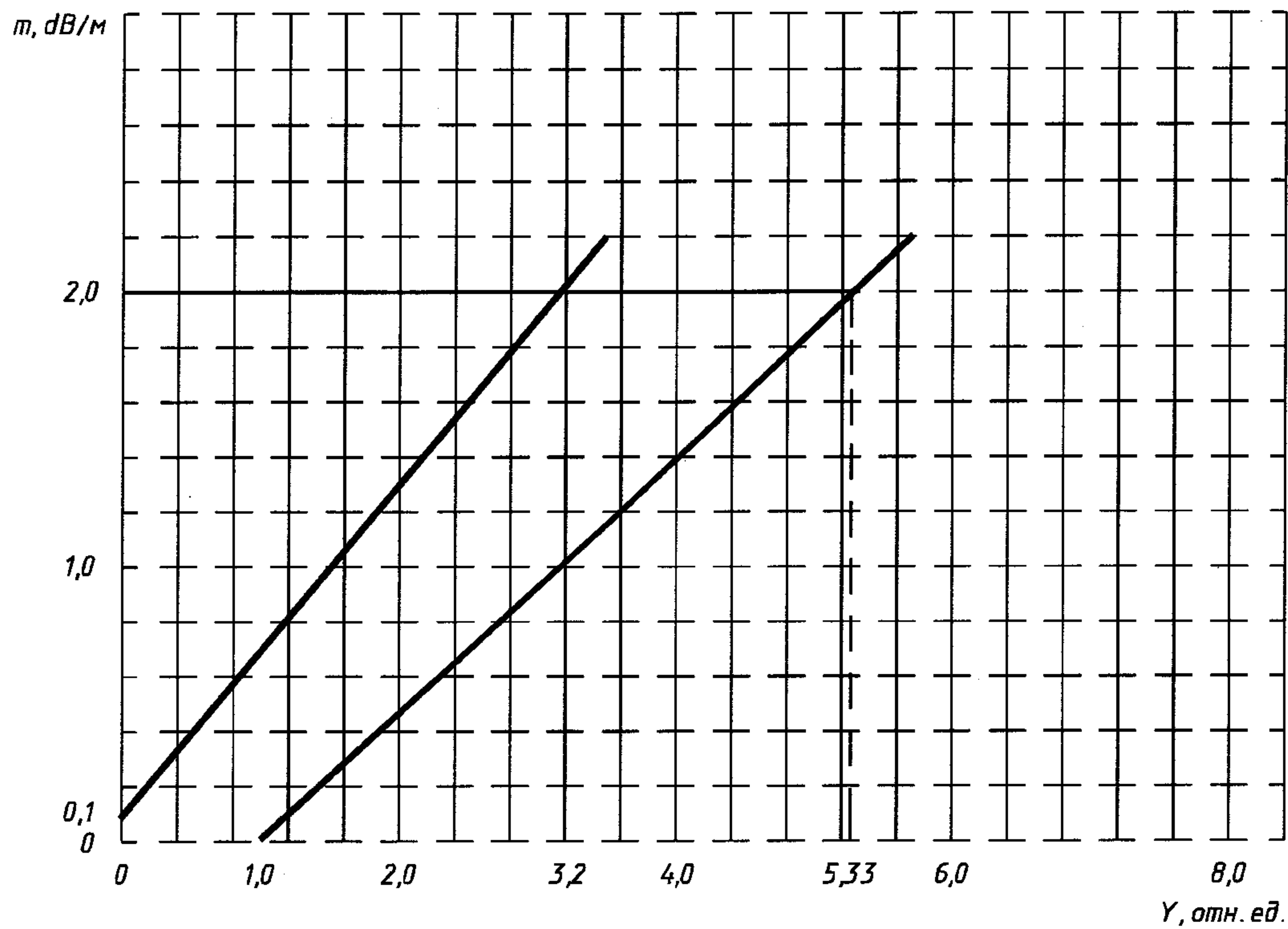
Рисунок Л.6 — Тестовый очаг пожара ТП-3. Зависимость оптической плотности среды от концентрации продуктов горения
