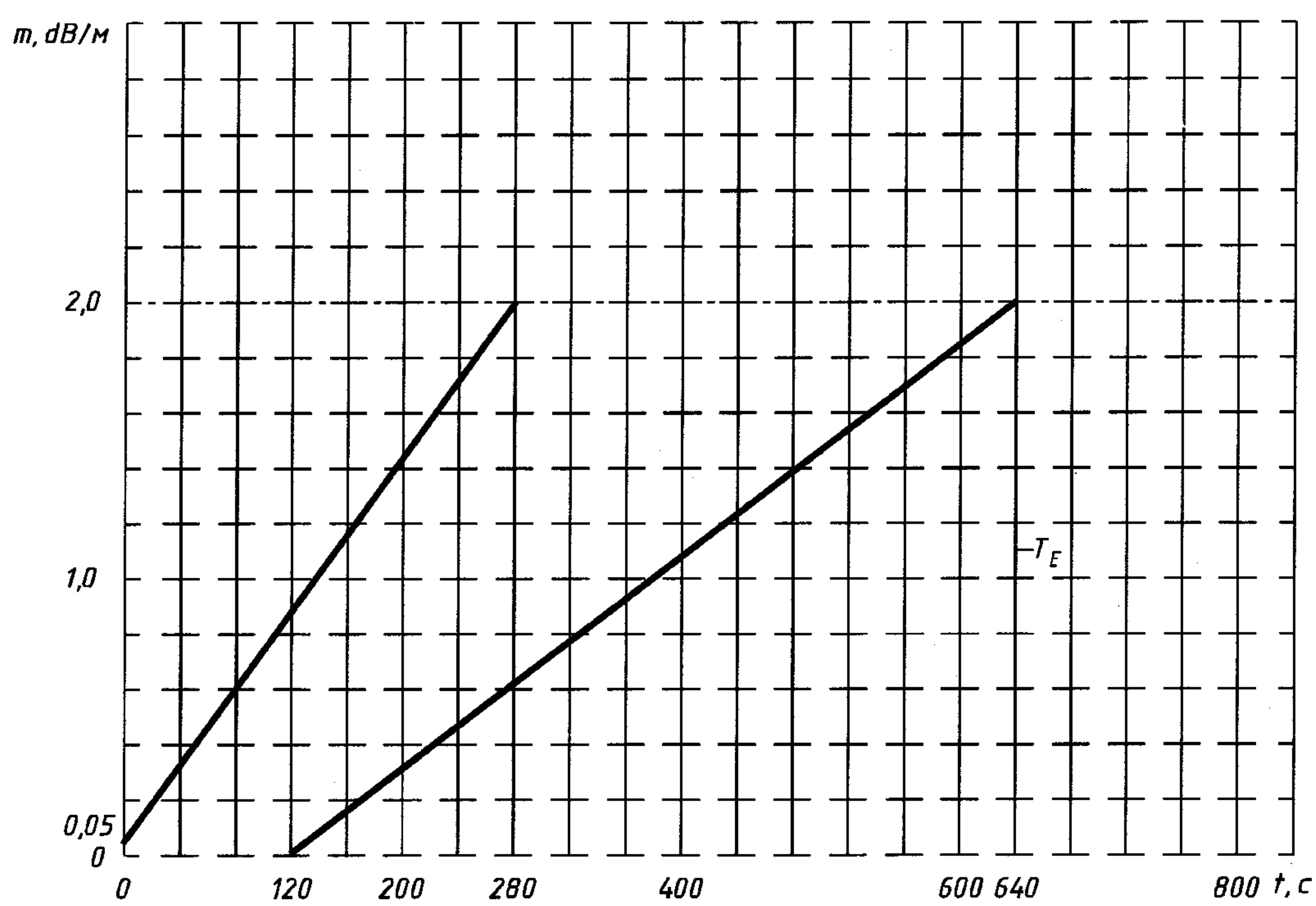
Рисунок Л.5 — Тестовый очаг пожара ТП-3. Зависимость оптической плотности среды от времени
