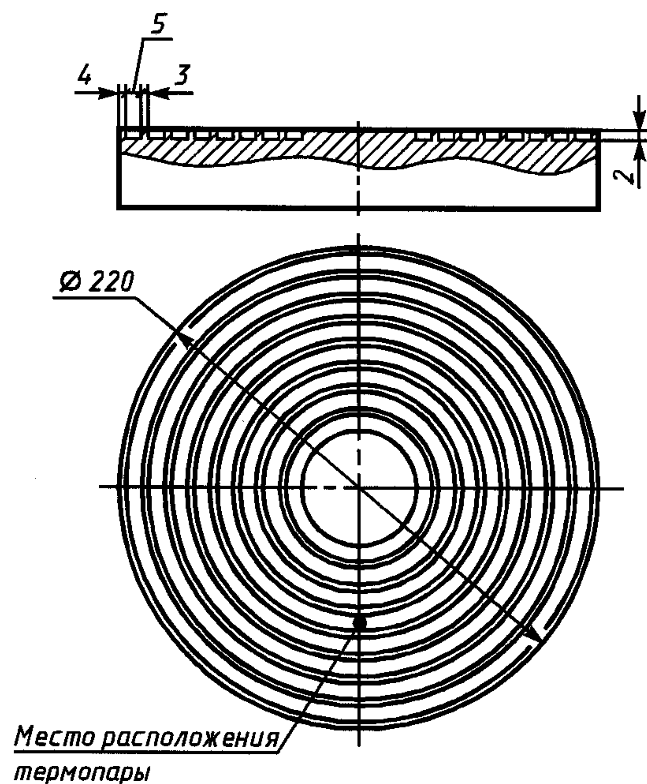
Рисунок В.1— Внешний вид рабочей поверхности электроплиты
