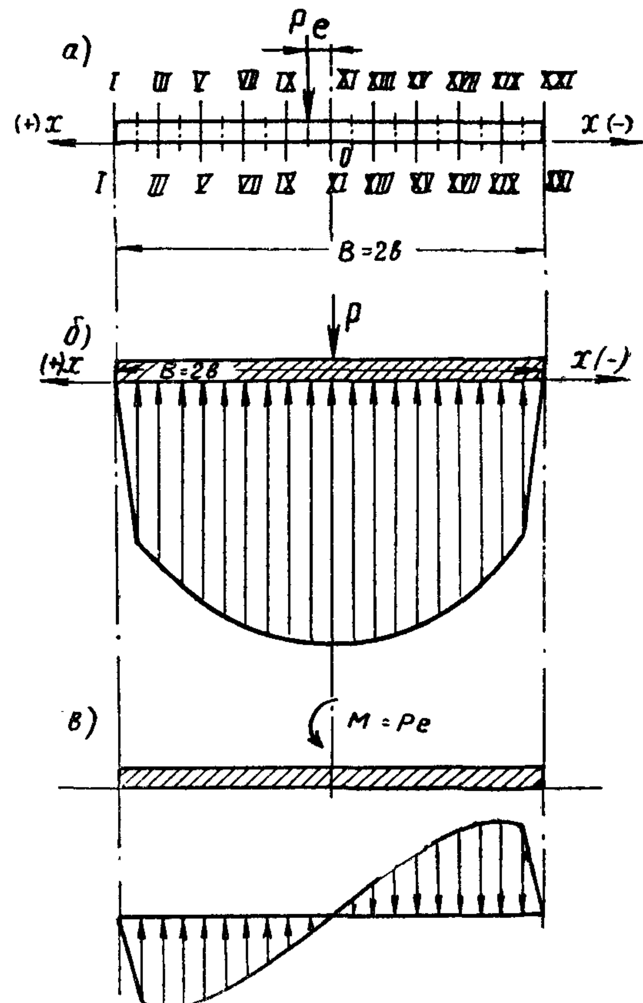
Рис. 6. К расчету фундаментной плиты а — расчетные сечения фундаментной плиты; б — эпюра контактных напряжений при действии только центральной вертикальной силы P 1 - \sigma_x = \bar{\sigma}_x \sigma_{\text{ср}} ; в — эпюра контактных напряжений при действии только момента
