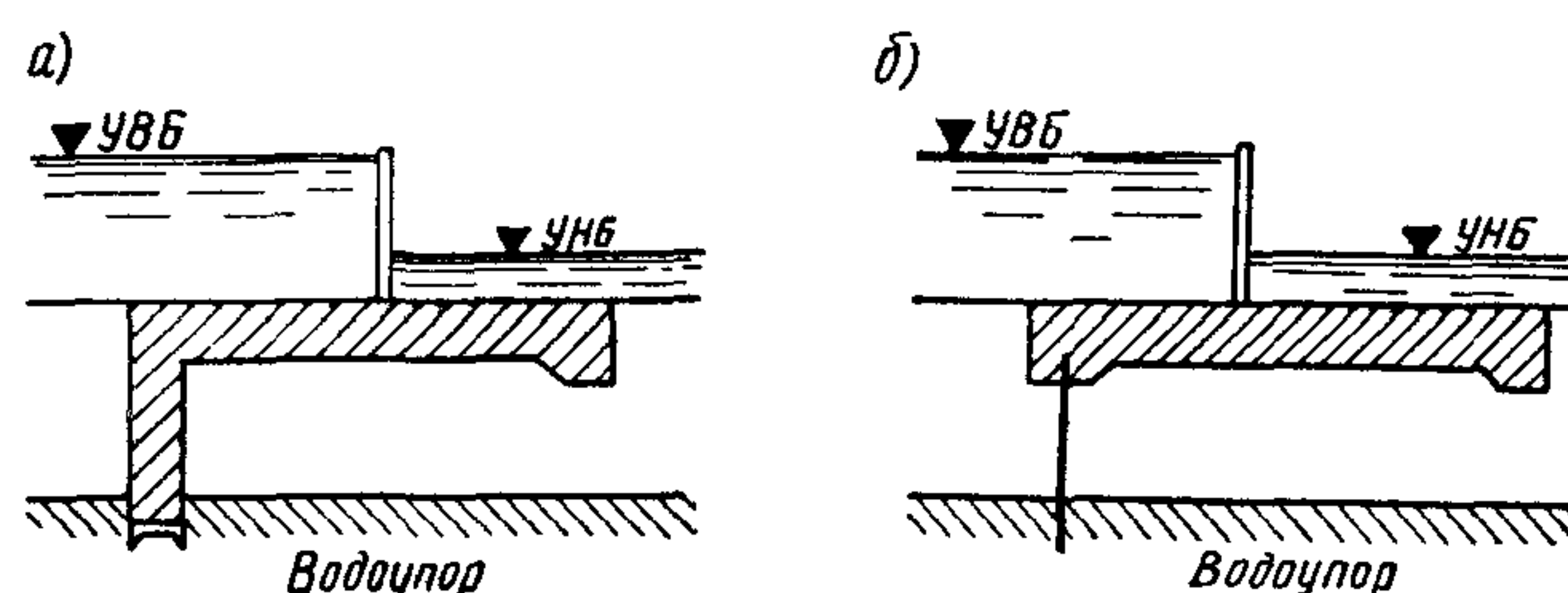
Рис. 4. Водопроницаемое основание до водоупора пересекается:
