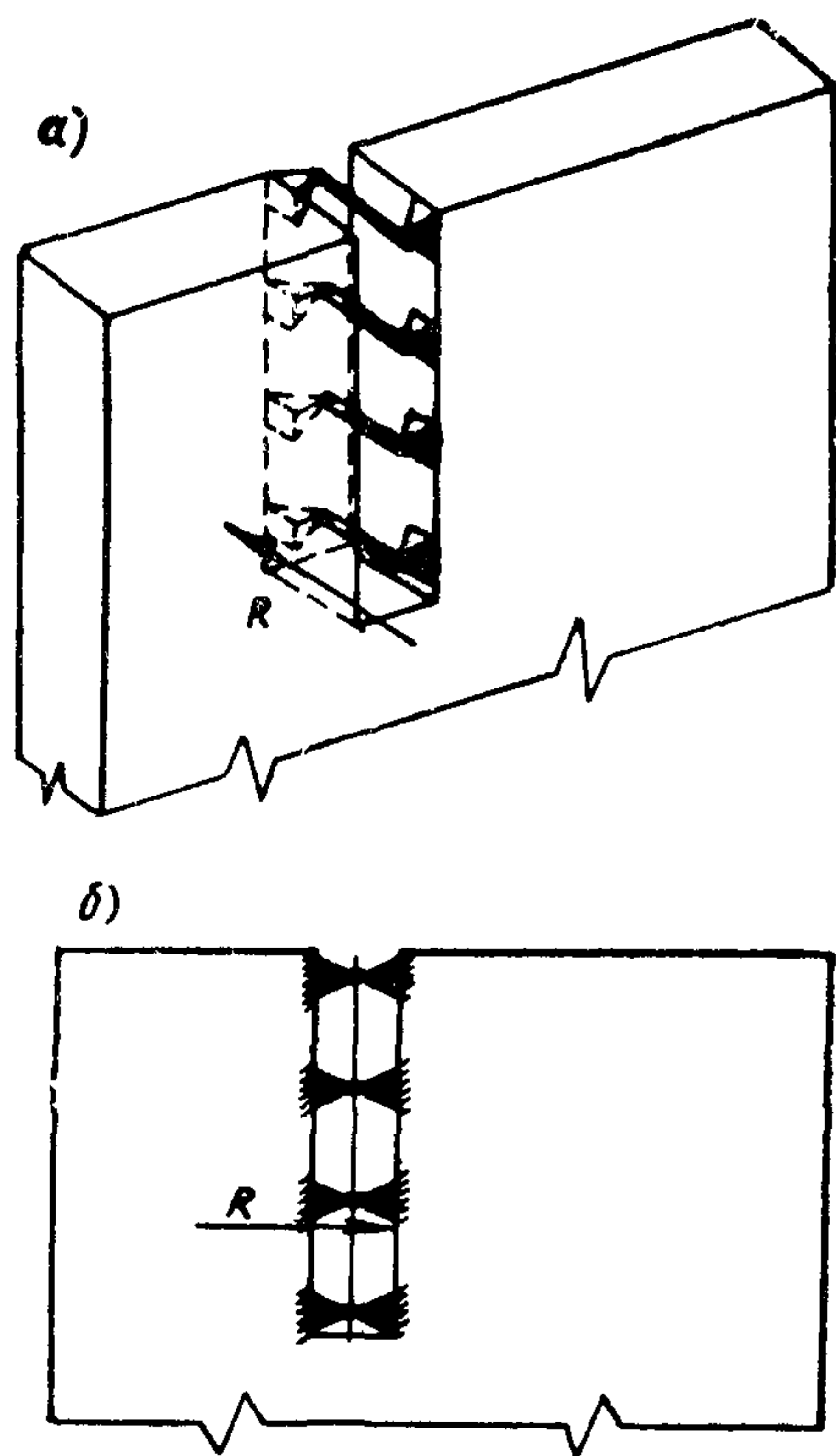
Рис. 5. Расчетная схема быка
