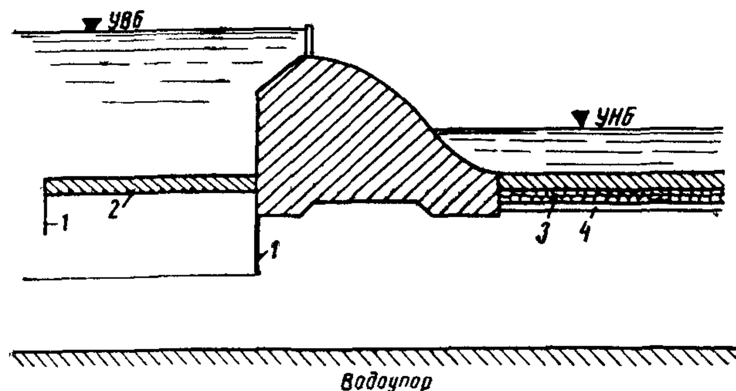
Рис. 1. Бездренажные фундаментная плита и понур 1 — шпунт; 2 — понур; 3 — дренаж; 4 — обратный фильтр
