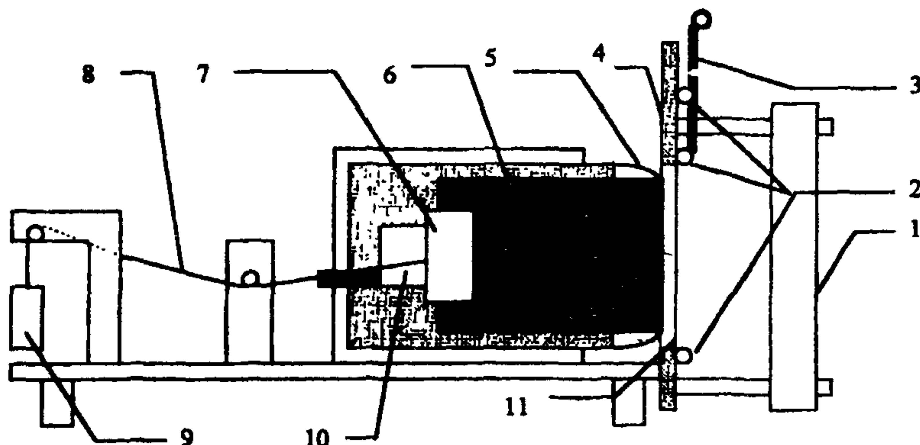
Рисунок 7. Схема установки для определения коэффициента теплопередачи текстильных материалов:
