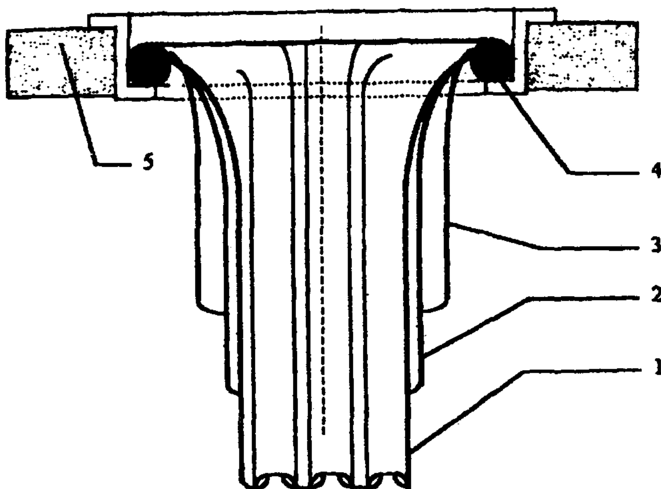
Рисунок 2. Конструкция спасательного рукава:
