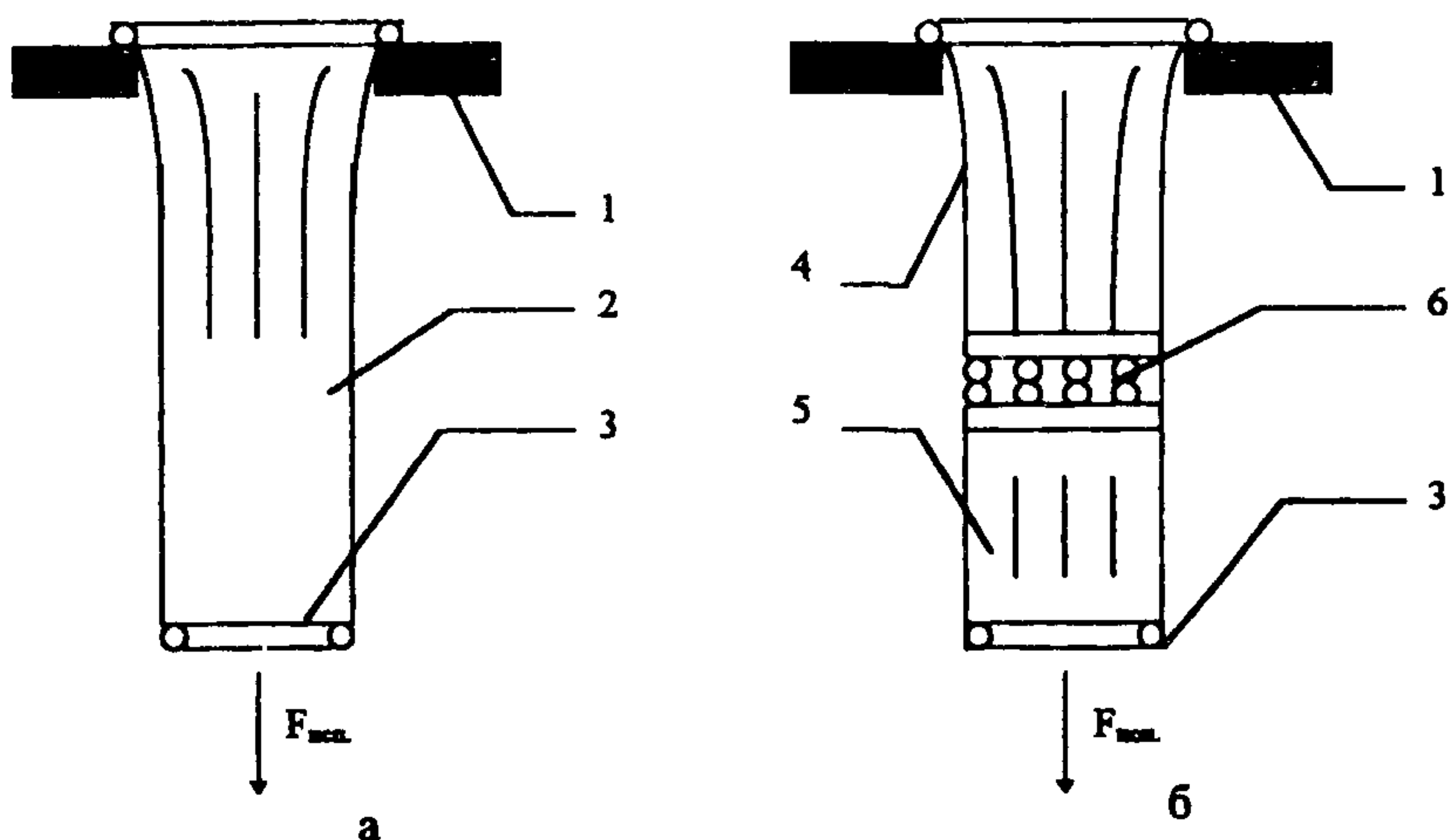
Рисунок 4. Схема испытания спасательного рукава на прочность:
