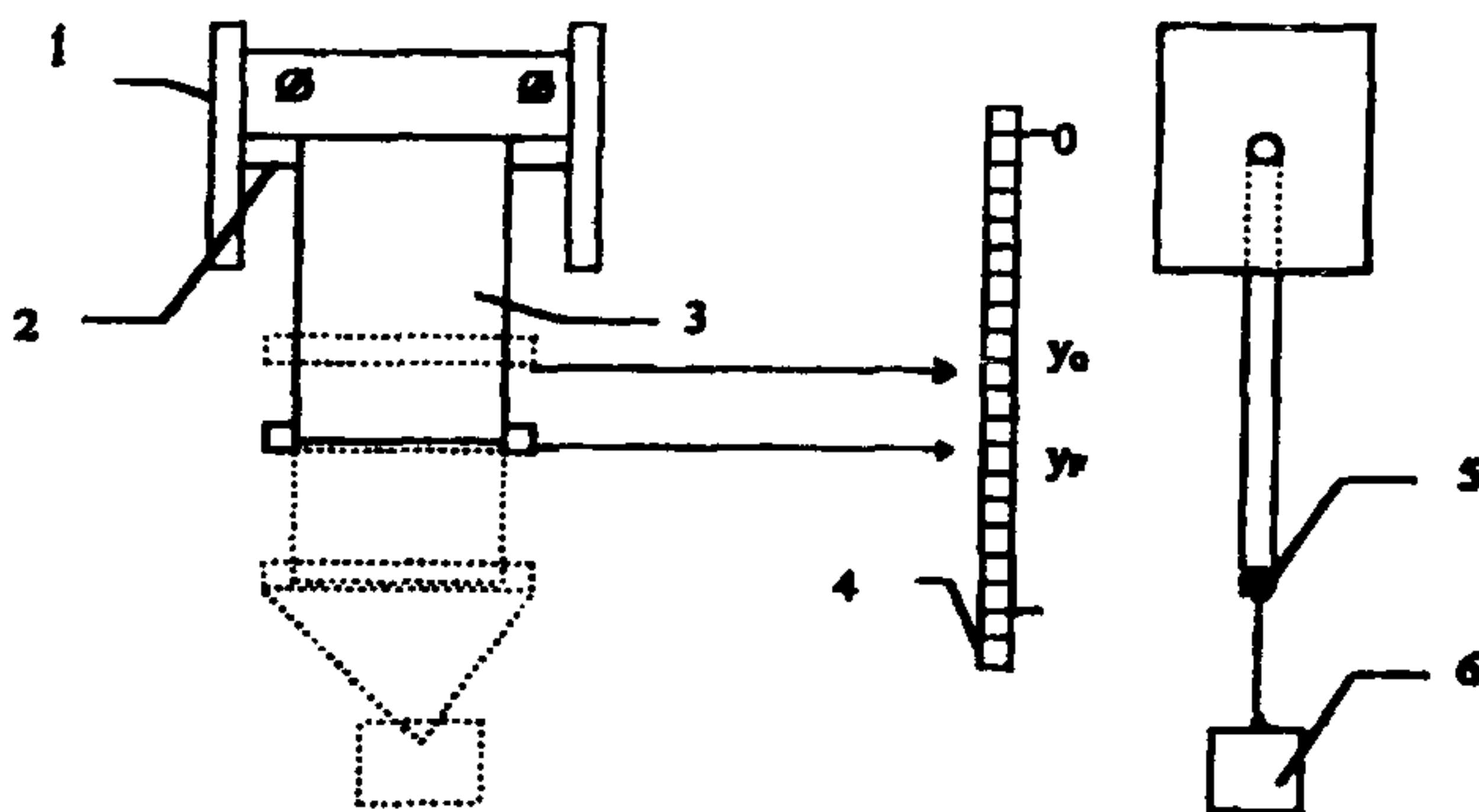
Рисунок 6. Установка для растяжения образцов эластичных рукавов:
