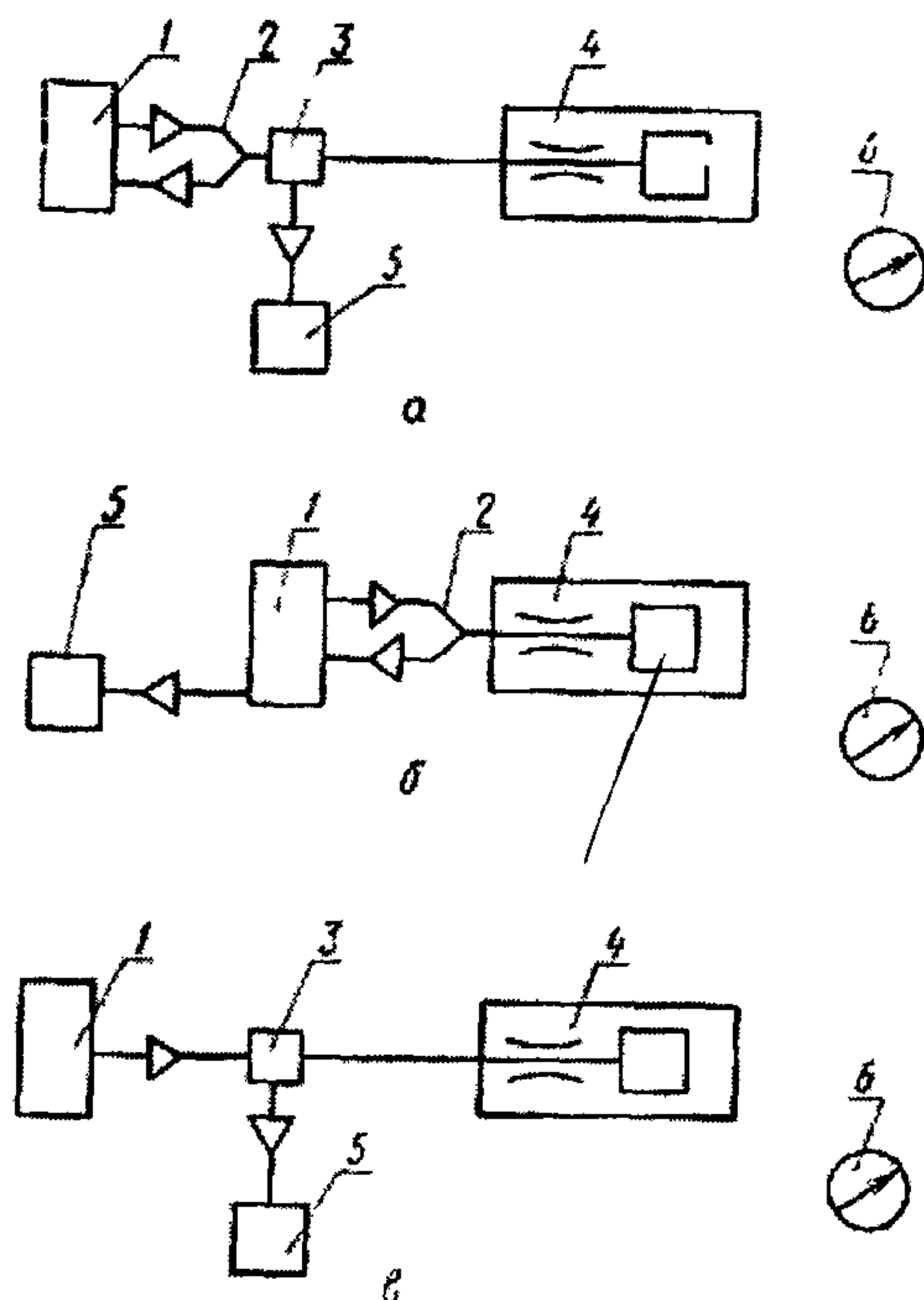
Рис. 2. Схемы проверки минутной вентиляции воздуха:
