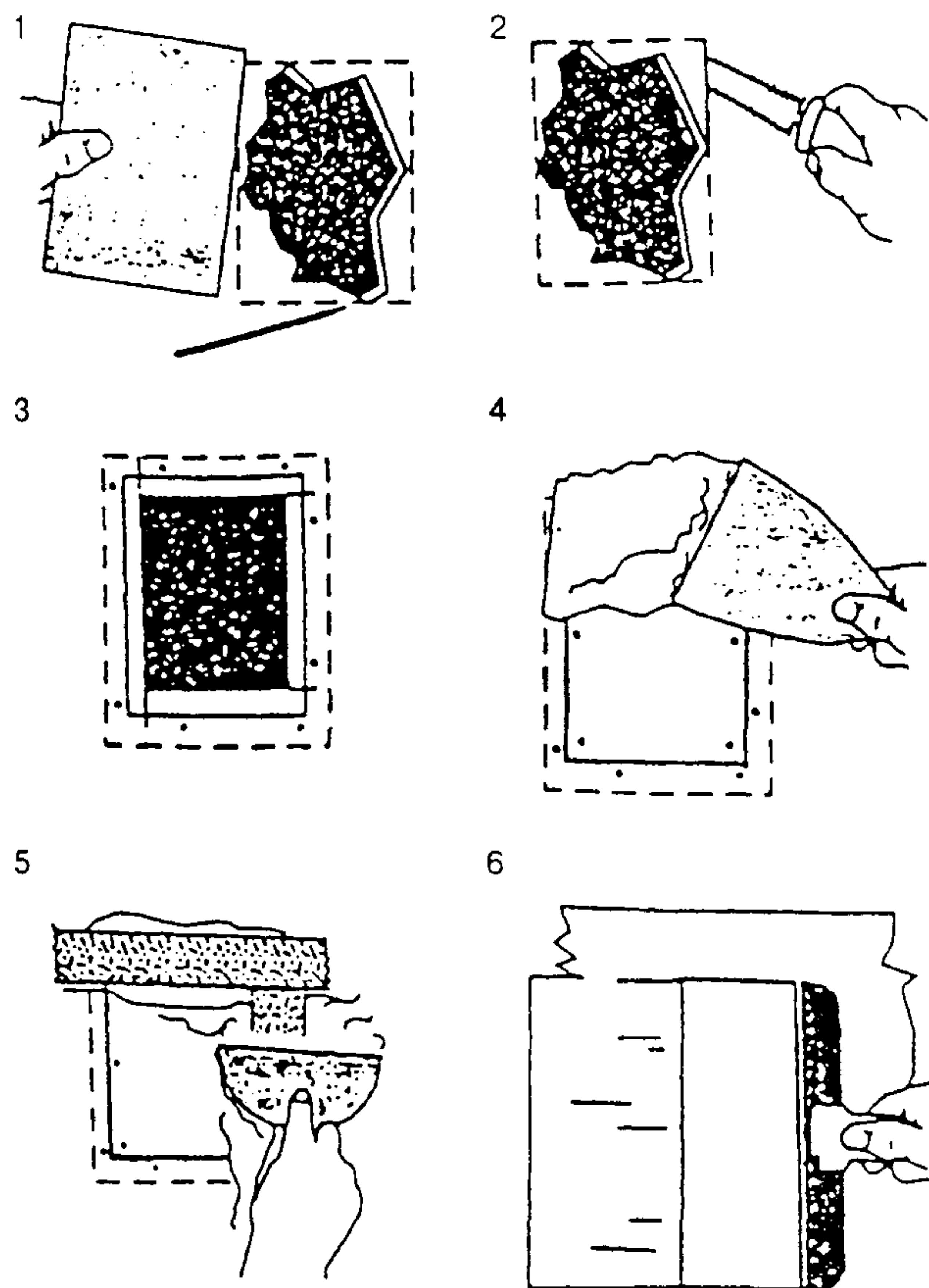
Рисунок 46 — Последовательность операций по заделке больших пробоин в ГКЛ
