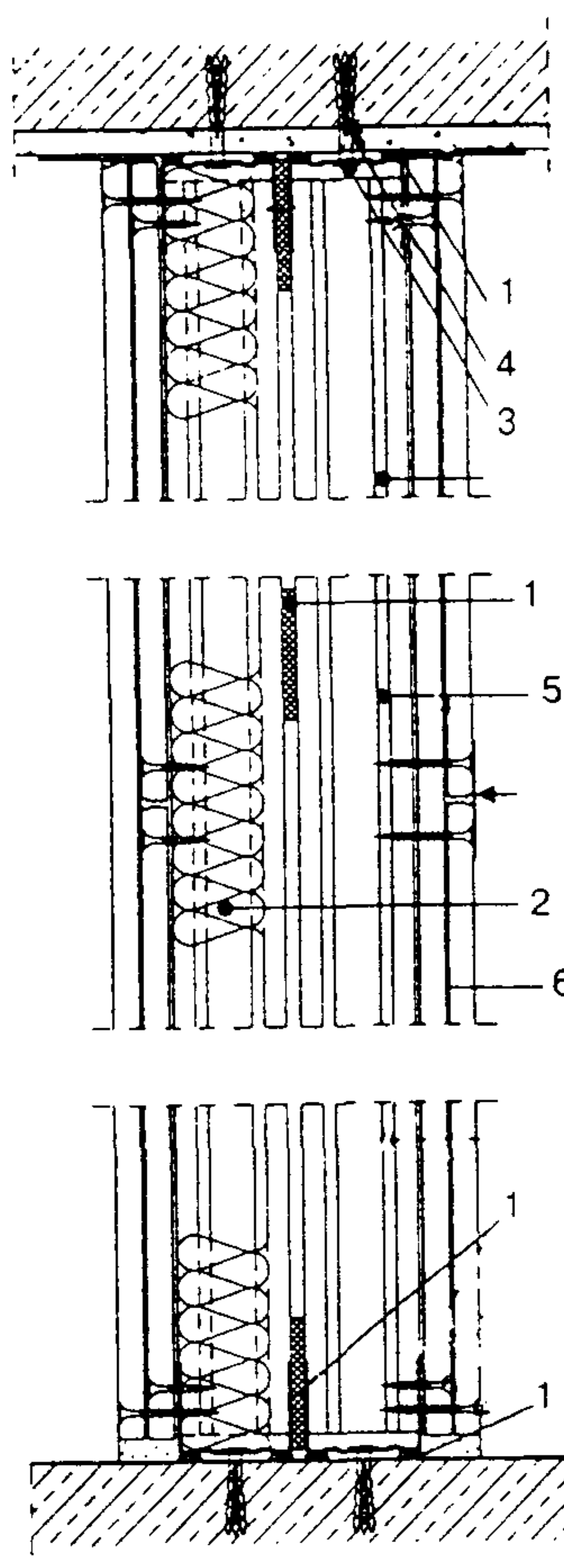
Вертикальный разрез
