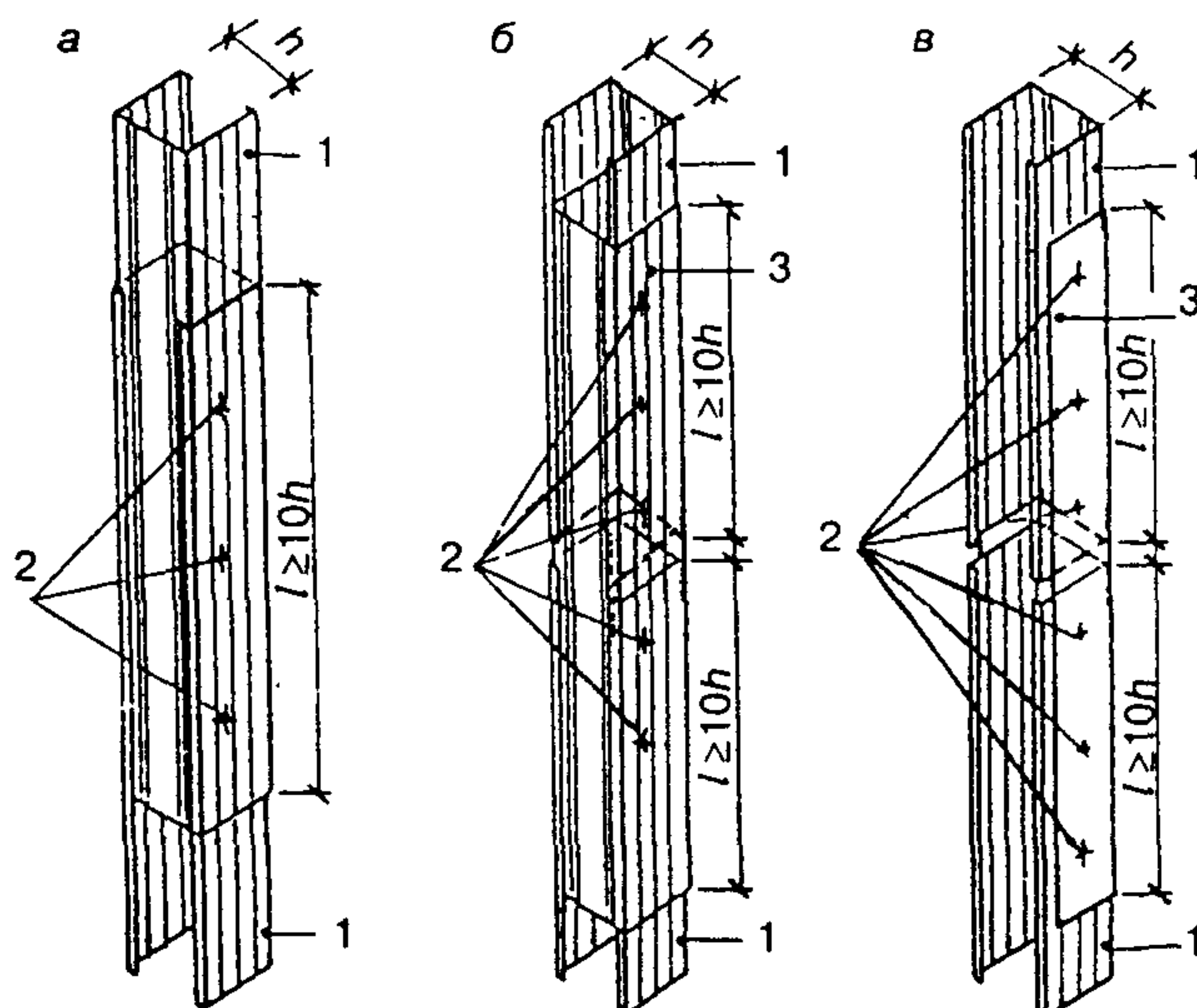
1 — стыкуемые профили; 2 — шурупы; 3 — дополнительный профиль
