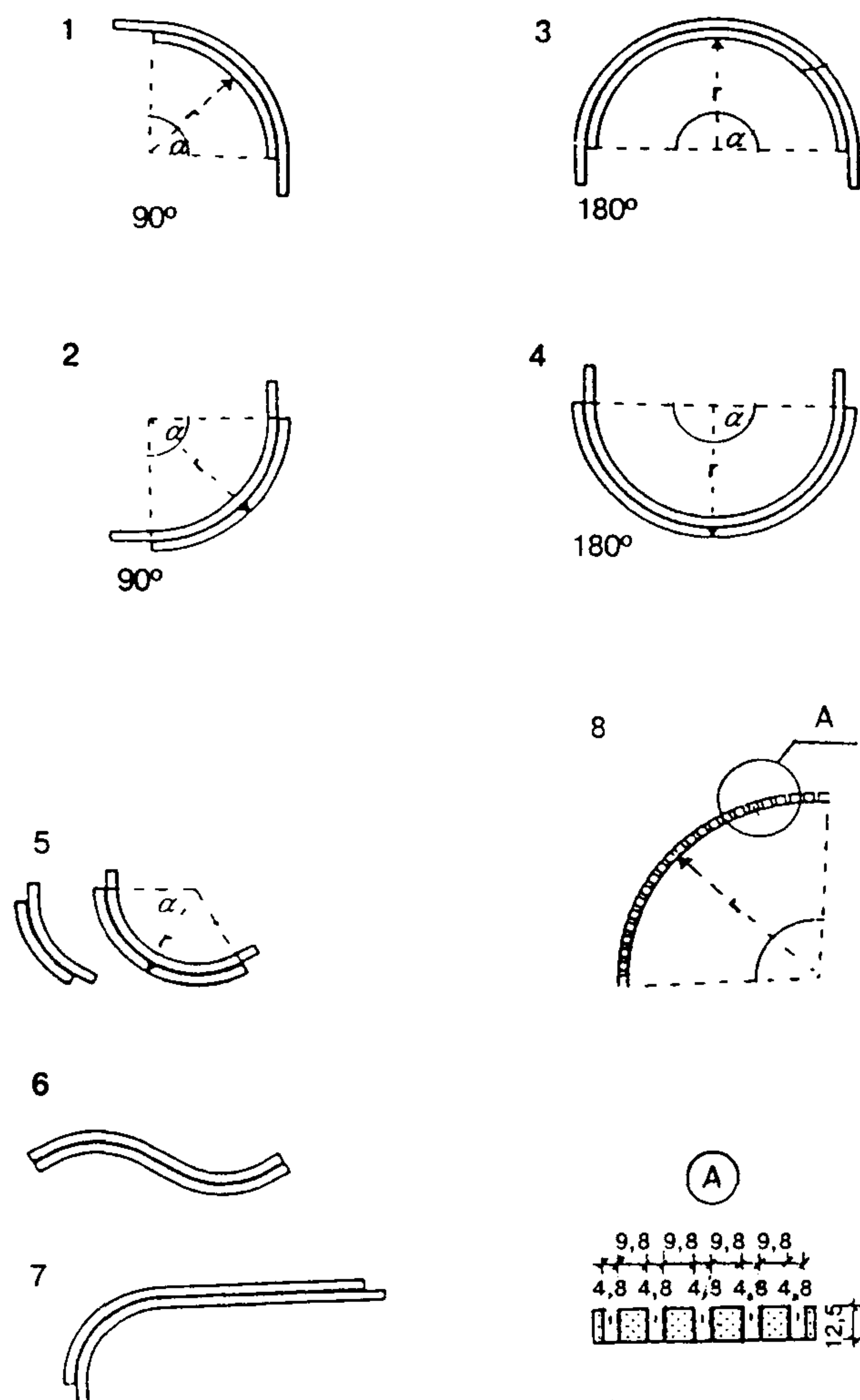
1, 2 — с углом 90°; 3, 4 — с углом 180°; 5 — с любым углом до 180°; 6 — S-образный; 7 — изогнутый по длине; 8 — криволинейный элемент со шлицевыми пазами
