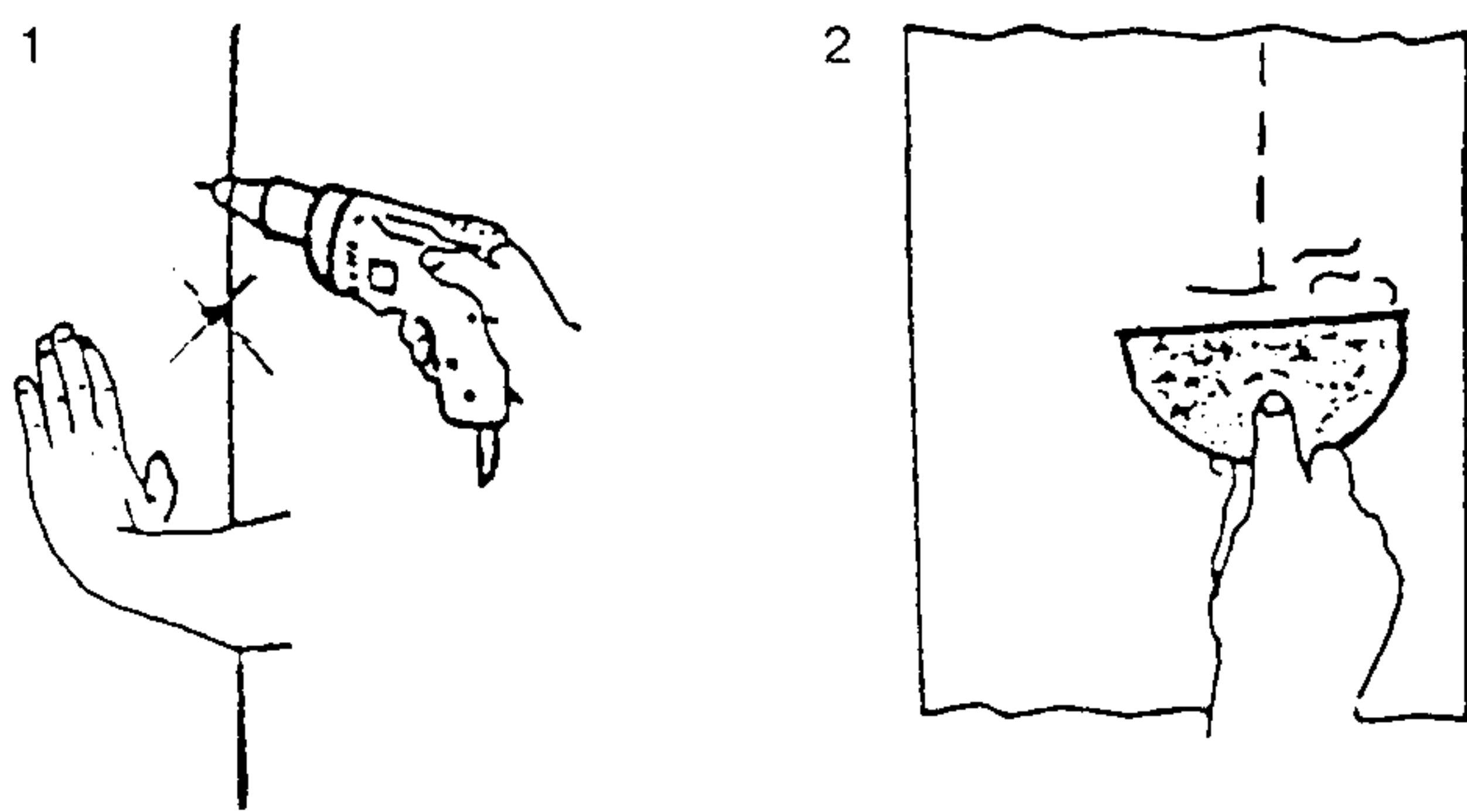
Рисунок 48 — Последовательность операций по замене крепежа ГКЛ
