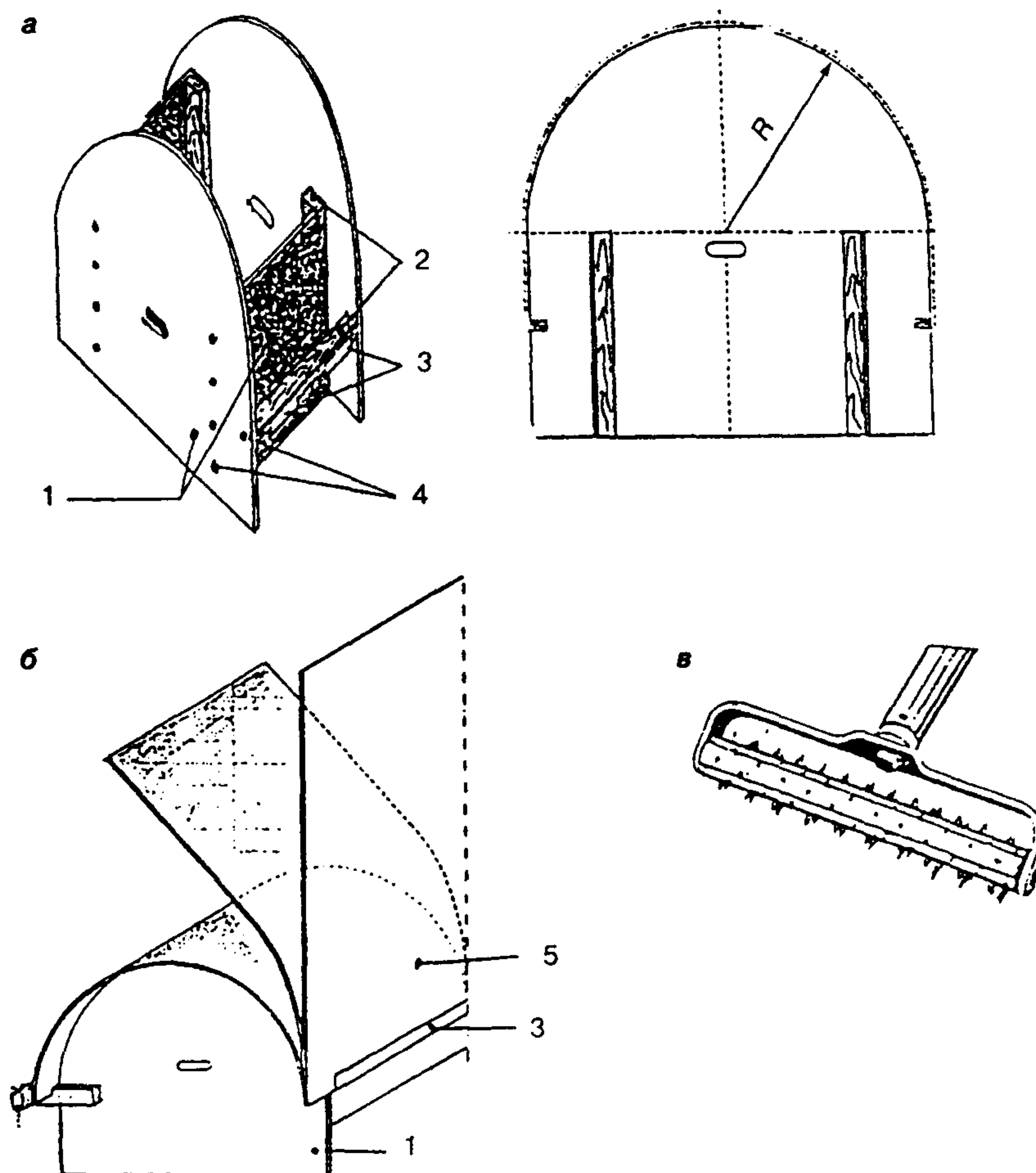
Рисунок 39 — Подготовка гипсокартонных листов
