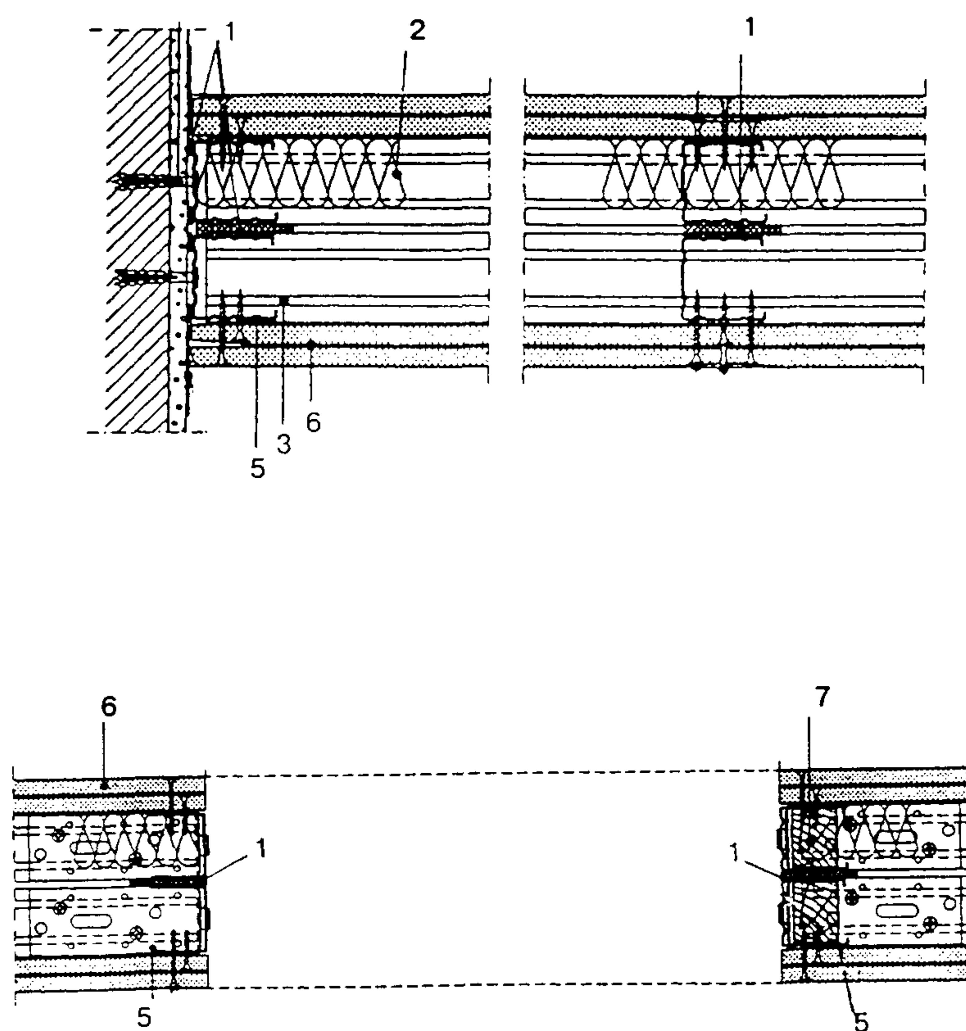
Горизонтальный разрез
