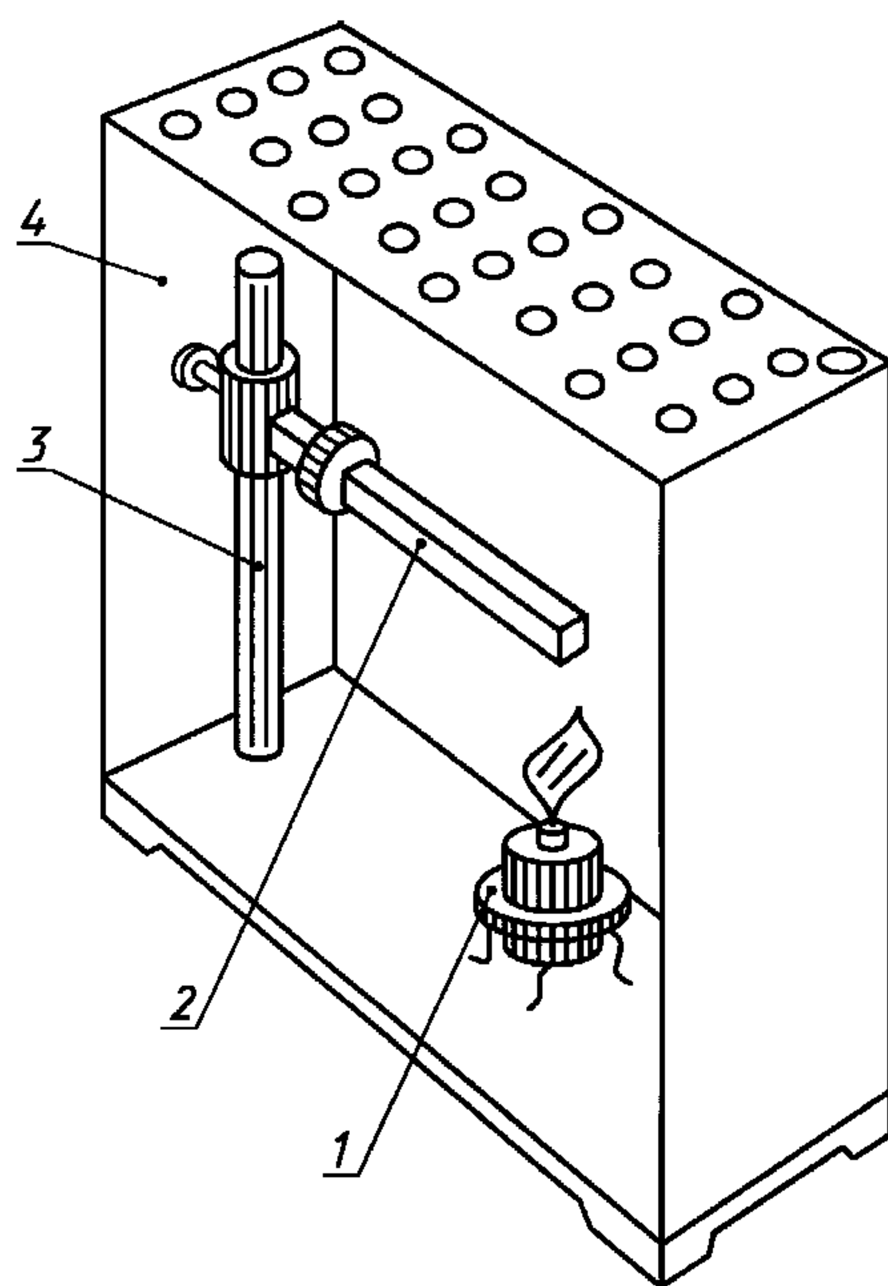
1 — горелка; 2 — образец; 3 — штатив; 4 — камера
