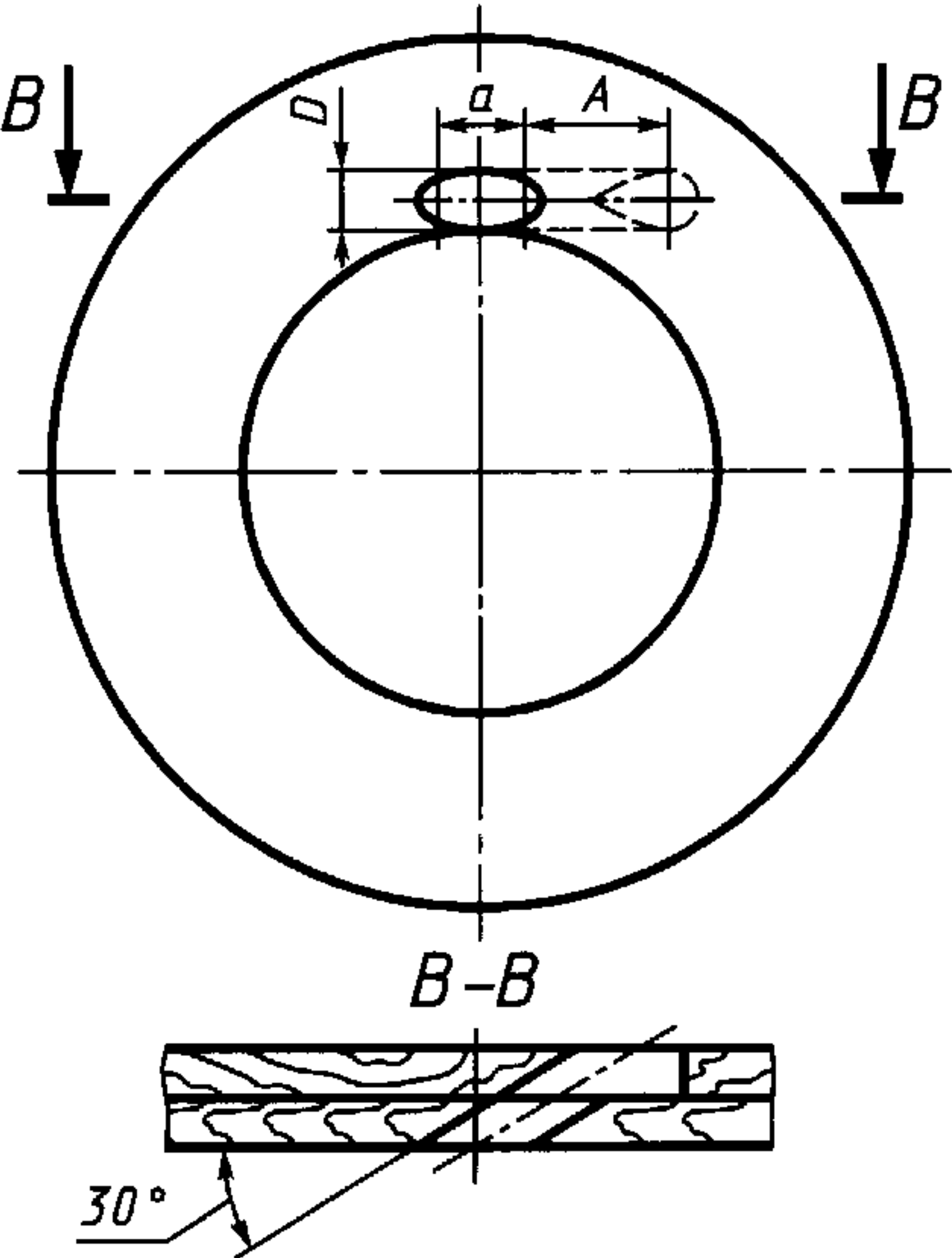
Выводное отверстие
