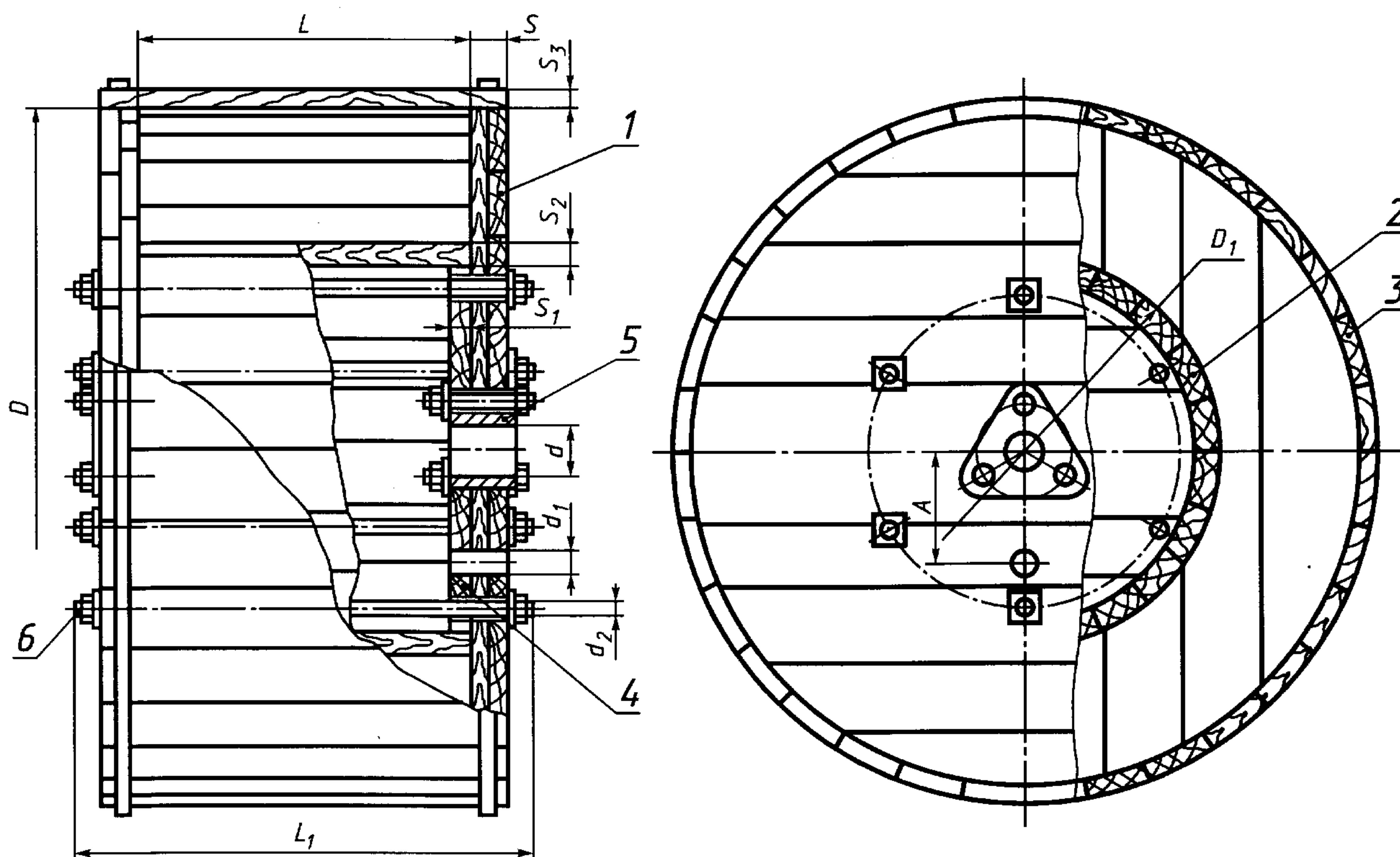
1 — щека; 2 — шейка; 3 — обшивка; 4 — круг шейки; 5 — втулка; 6 — шпилька
