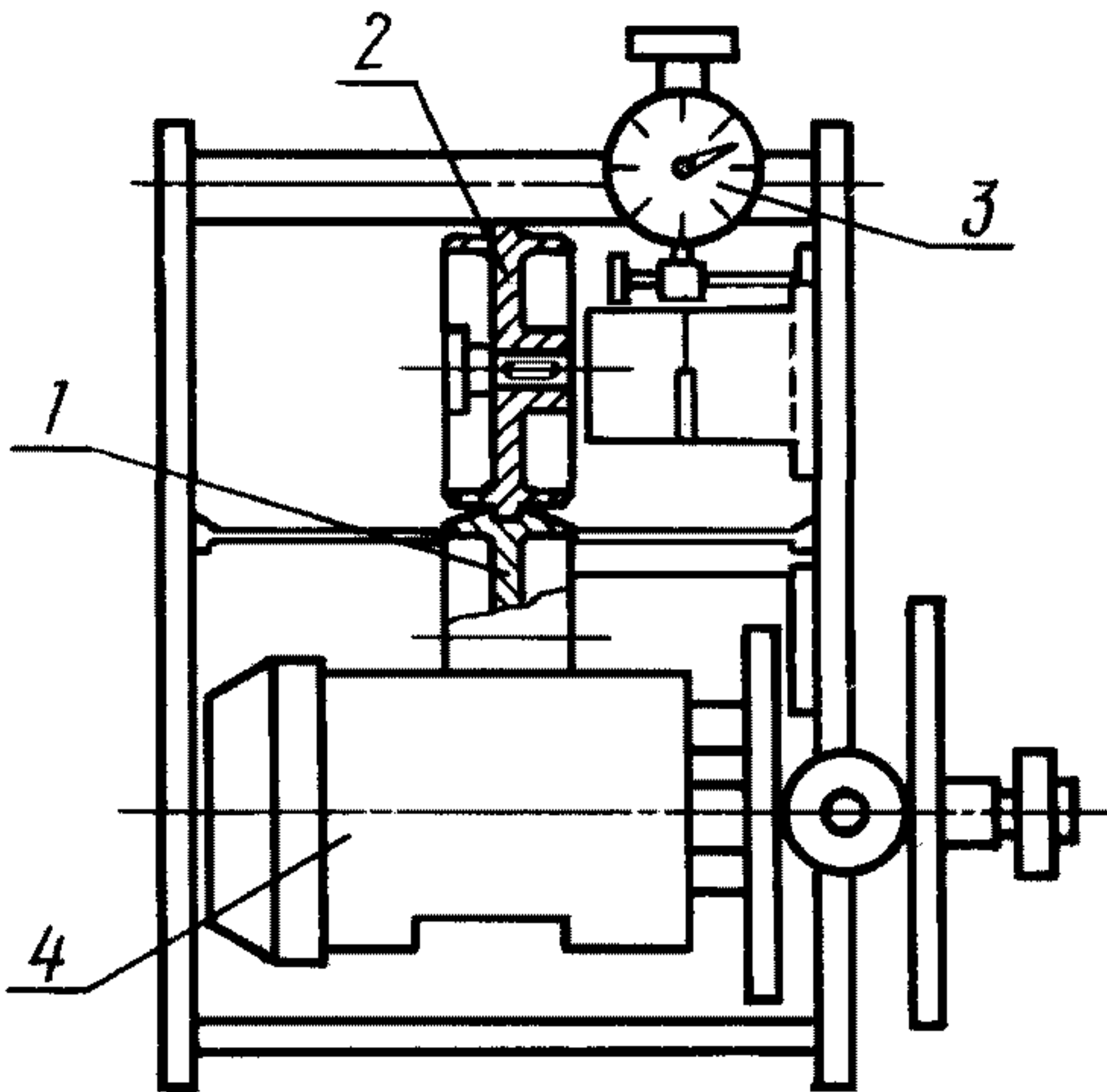
Устройство для рилевания
