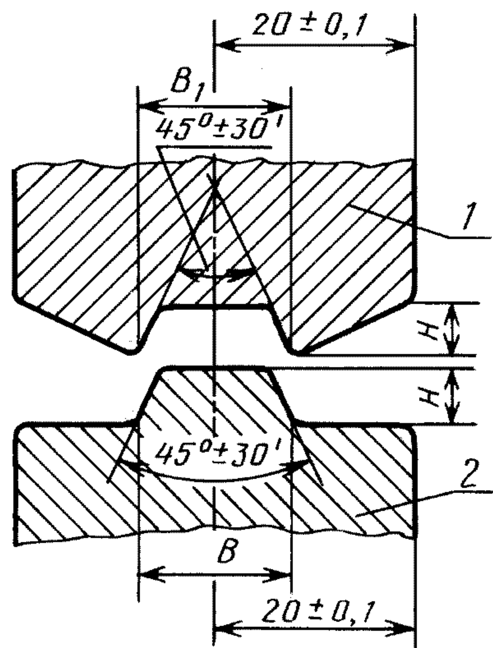
1 — муфта с выемкой; 2 — муфта с выступом
