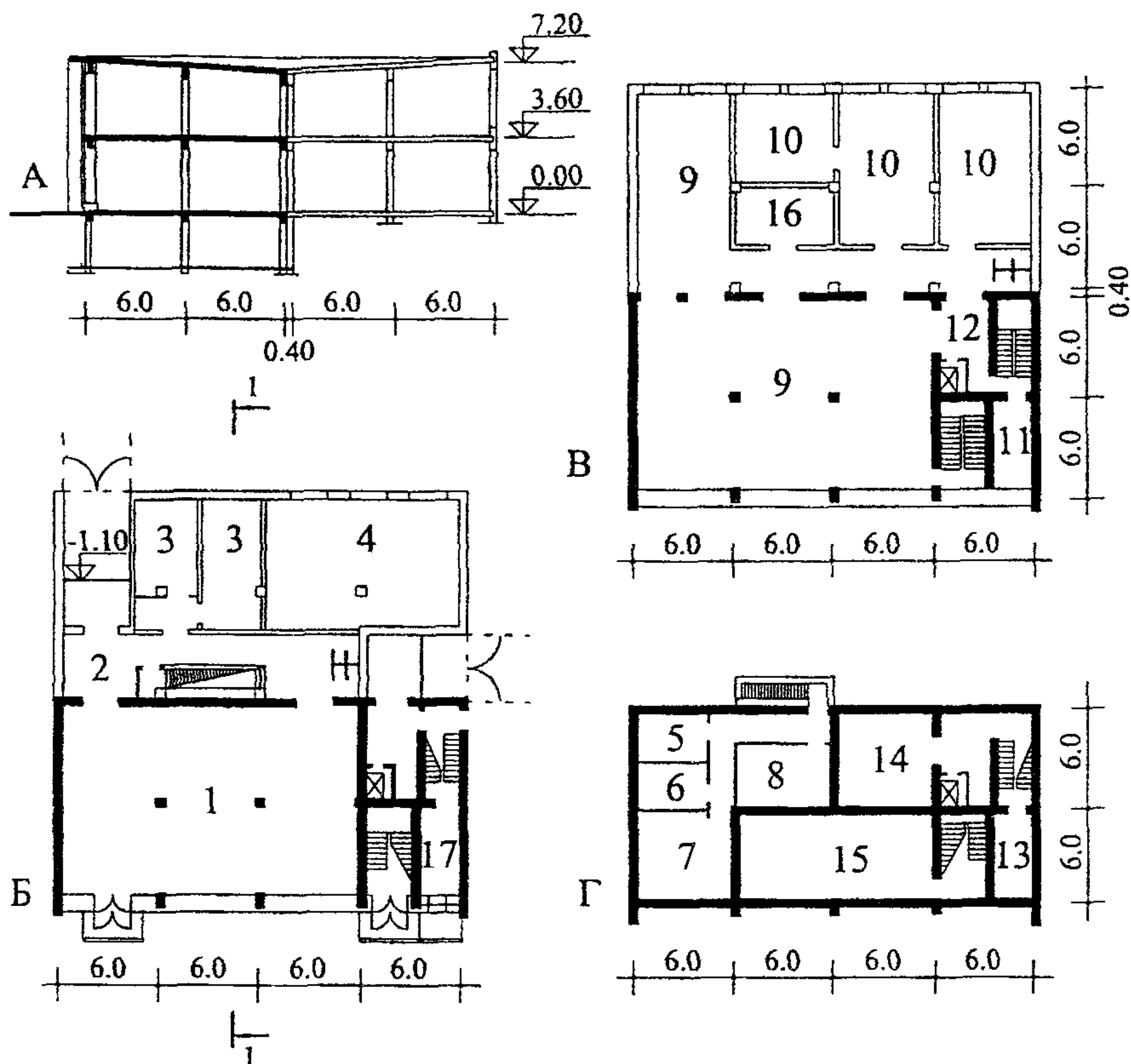
Рис. 13. ПРИМЕР РЕКОНСТРУКЦИИ ТИПОВОГО ПРОЕКТА 1Х-01-15
