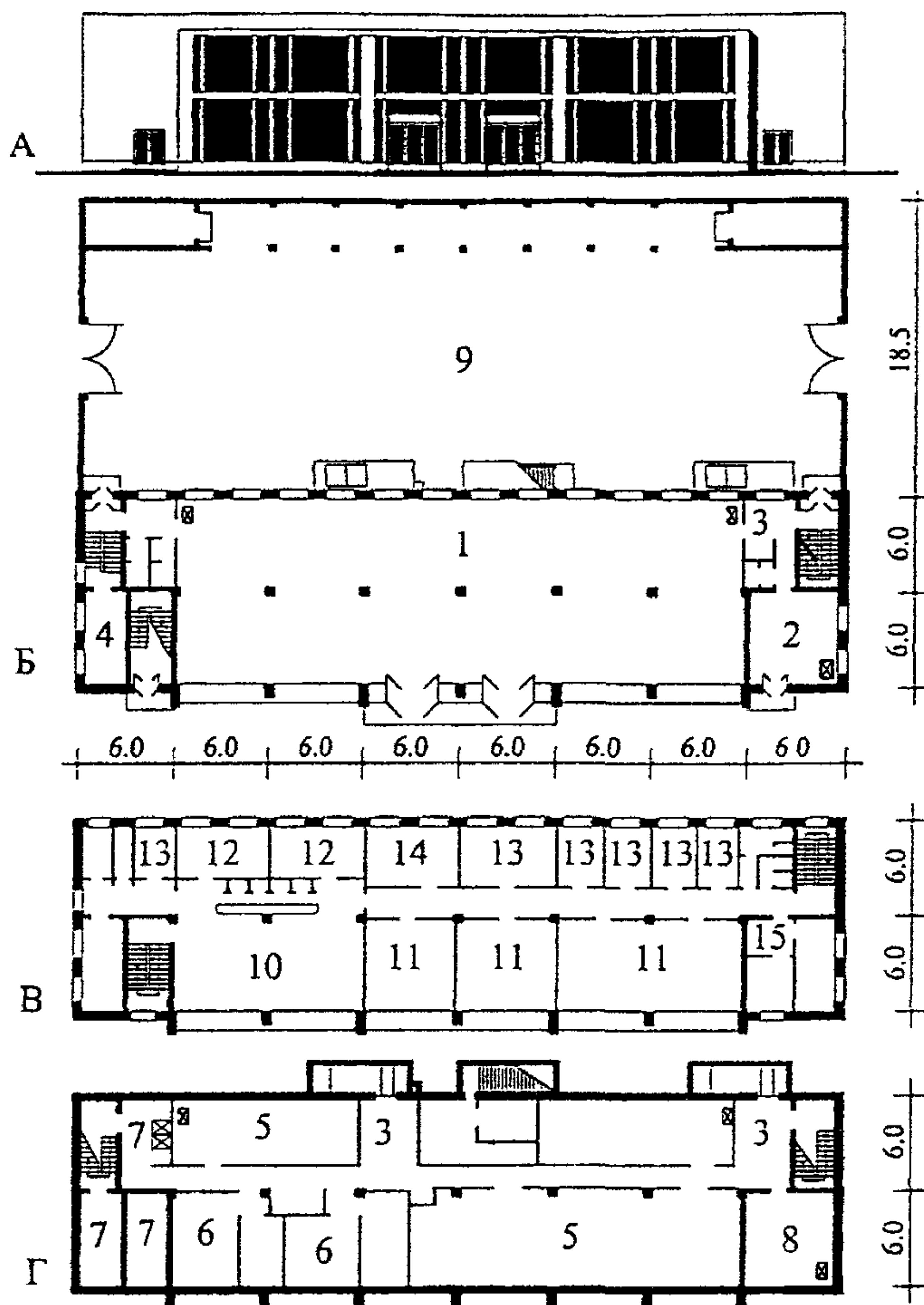
Рис. 2. ТИПОВОЙ ПРОЕКТ 1Х-01-18
