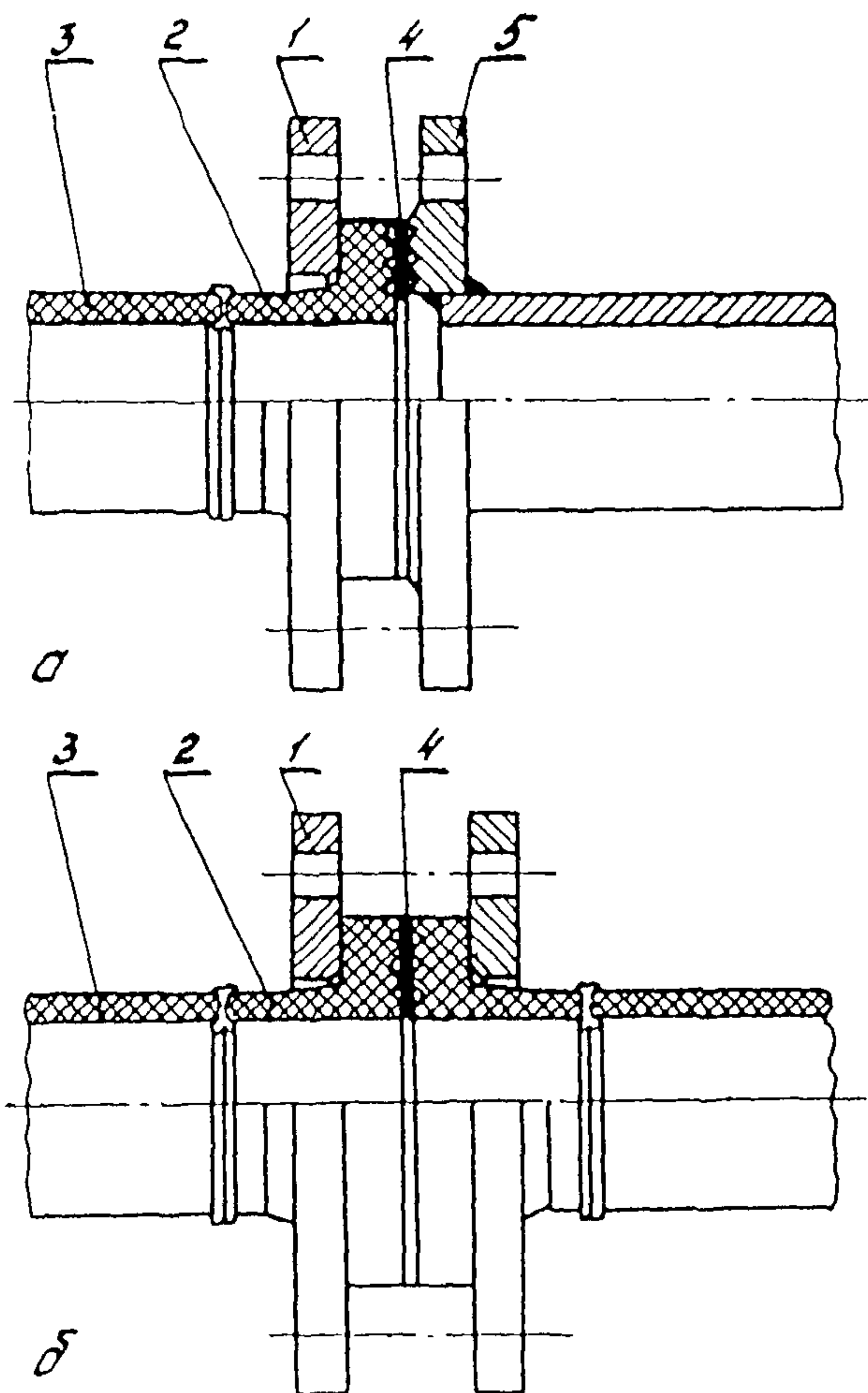
Рис.II. Фланцевые соединения ;
