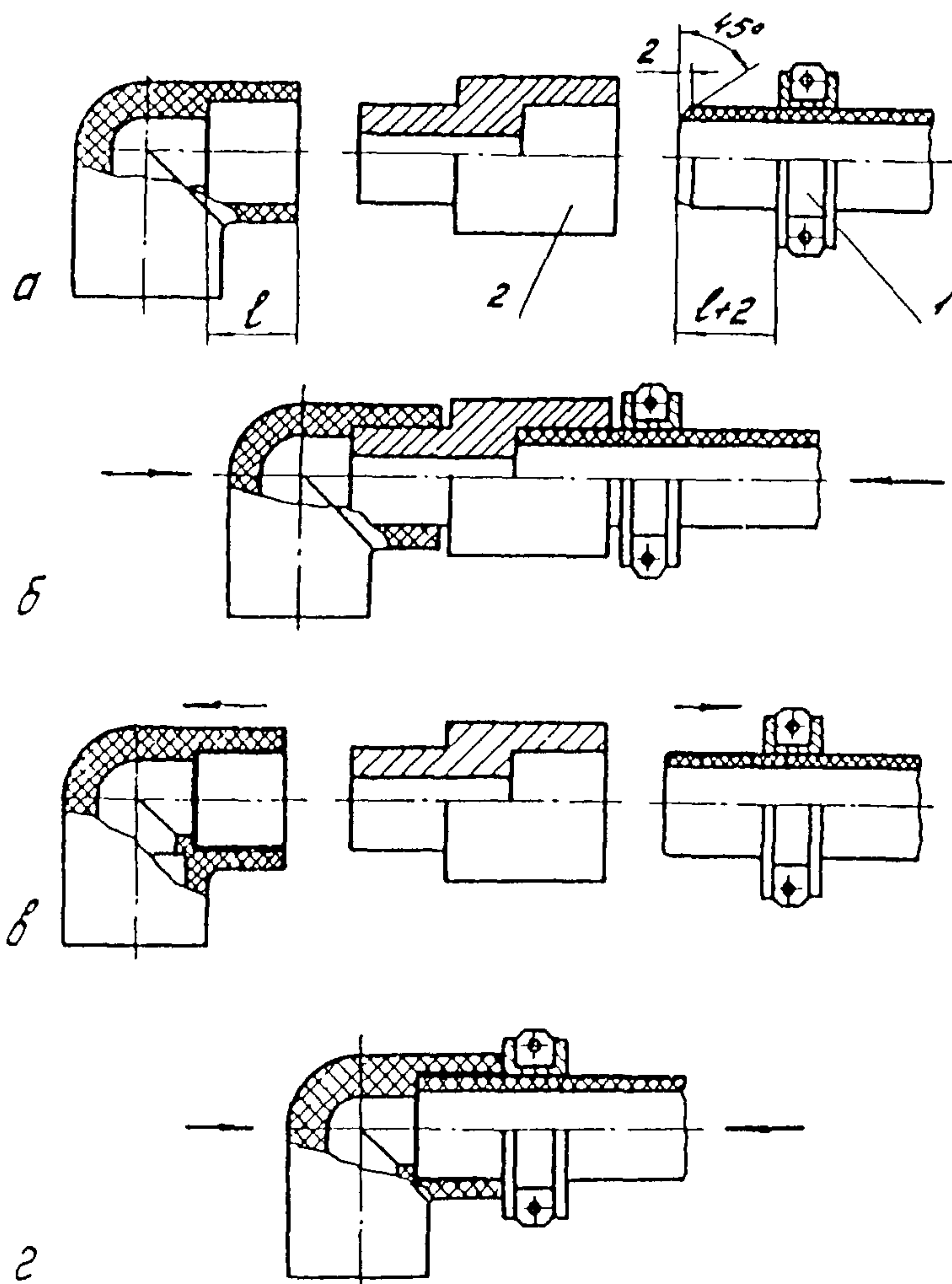
Рис. 9. Последовательность процесса контактной сварки в раструб труб и соединительных деталей из ПВД: а - центровки, закрепление в зажимах сварочного устройства концов свариваемых труб и деталей и установка ограничитель- ного хомута 1; б - установка дорна нагретого инструмента 2 в раструбе и гладкого конца трубы в гильзе; в - нагрев (оплавление) свариваемых концов, одновременно снятие их с дор- на и гильзы; г - соединение концов с выдержкой до затверде- вания сплавленного материала
