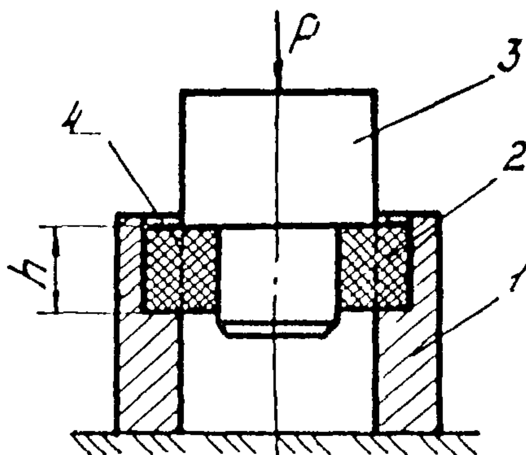
Рис.3. Схема испытания ра- трубного сварного соедине- ния на одвиг:
