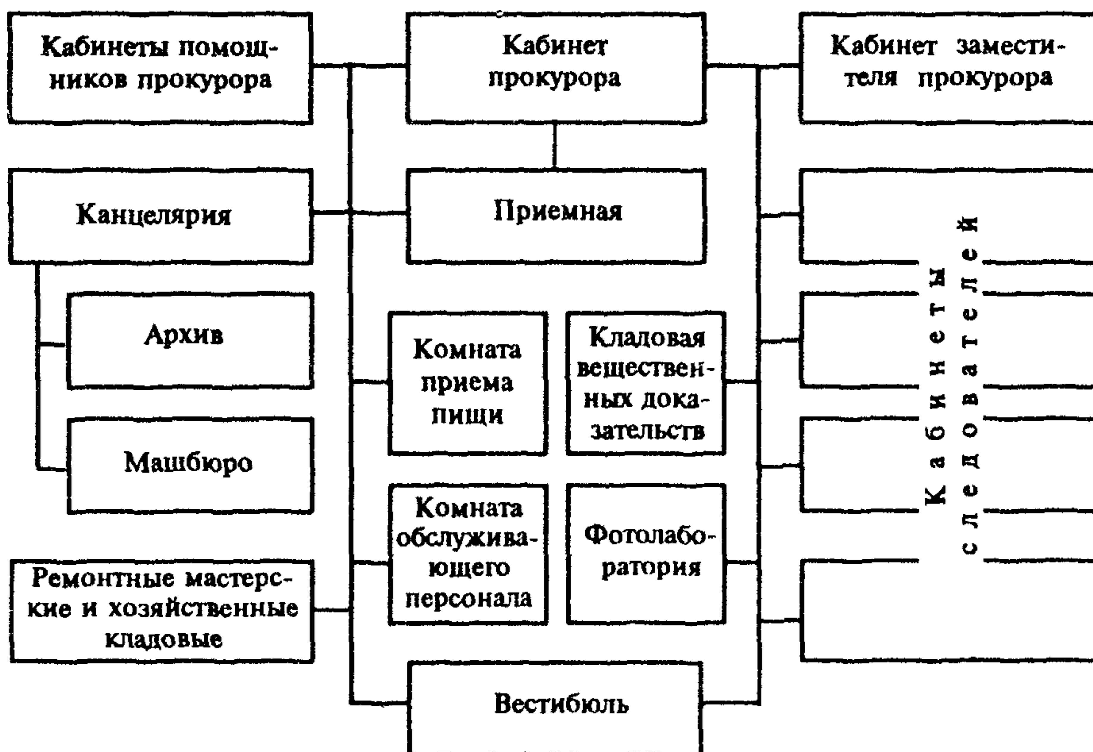
Рис. 3. Схема взаимосвязи помещений в зданиях районной и городской прокуратур
