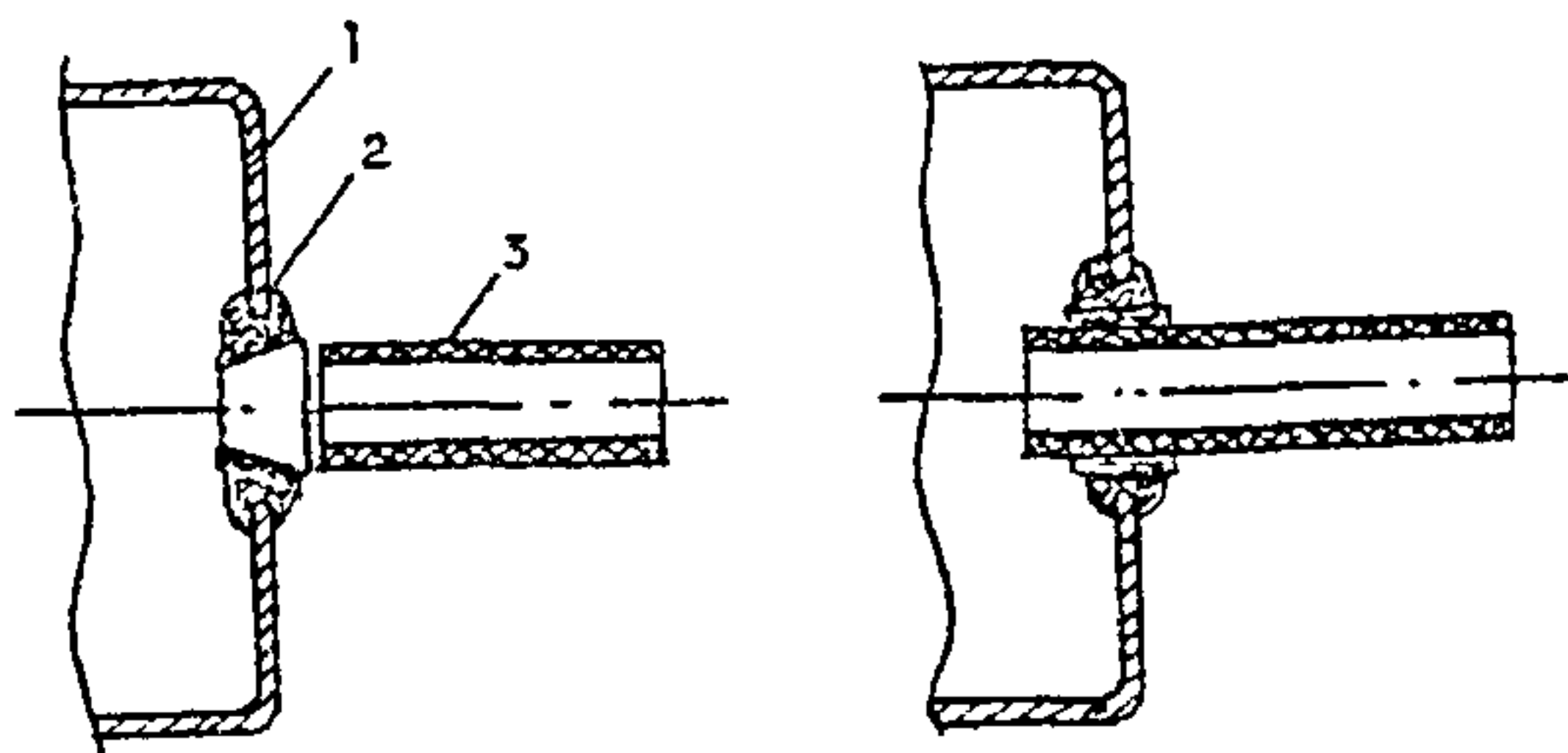
Рис.14. Схема устройства уплотненного ввода в коробку пластмассовых труб для электропроводок с использованием втулки:
