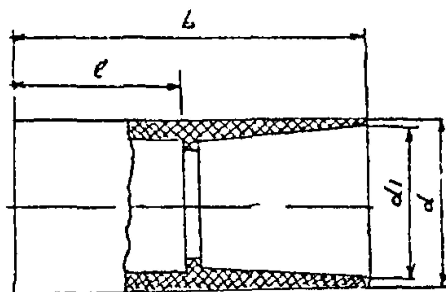
Рис.6. Схема соединительных муфт типа У276 УХЛЗ–У 297 УХЛЗ для использования с пластмассовыми трубами для электропроводок
