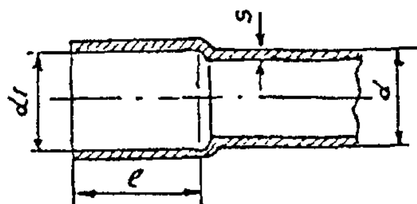
Рис.1 Схема раструба на пластмассовой трубе для электропроводок
