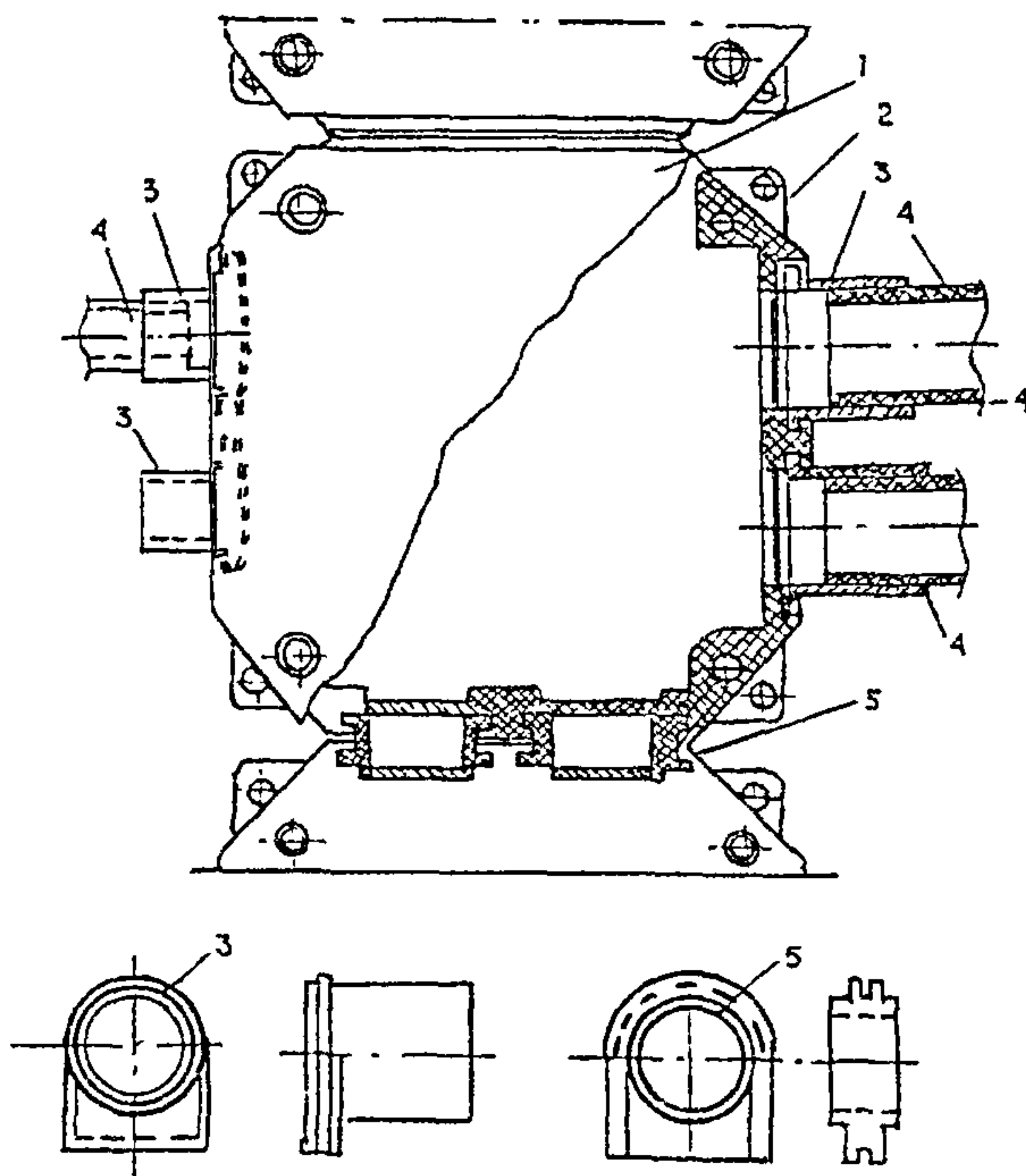
Рис.16. Схема ввода пластмассовых труб для электропроводок в распаечную пластмассовую коробку типа КРП-8:
