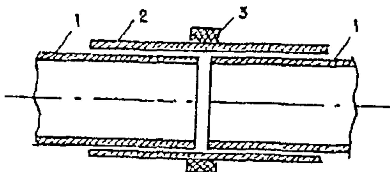
Рис.3. Схема компенсатора:
