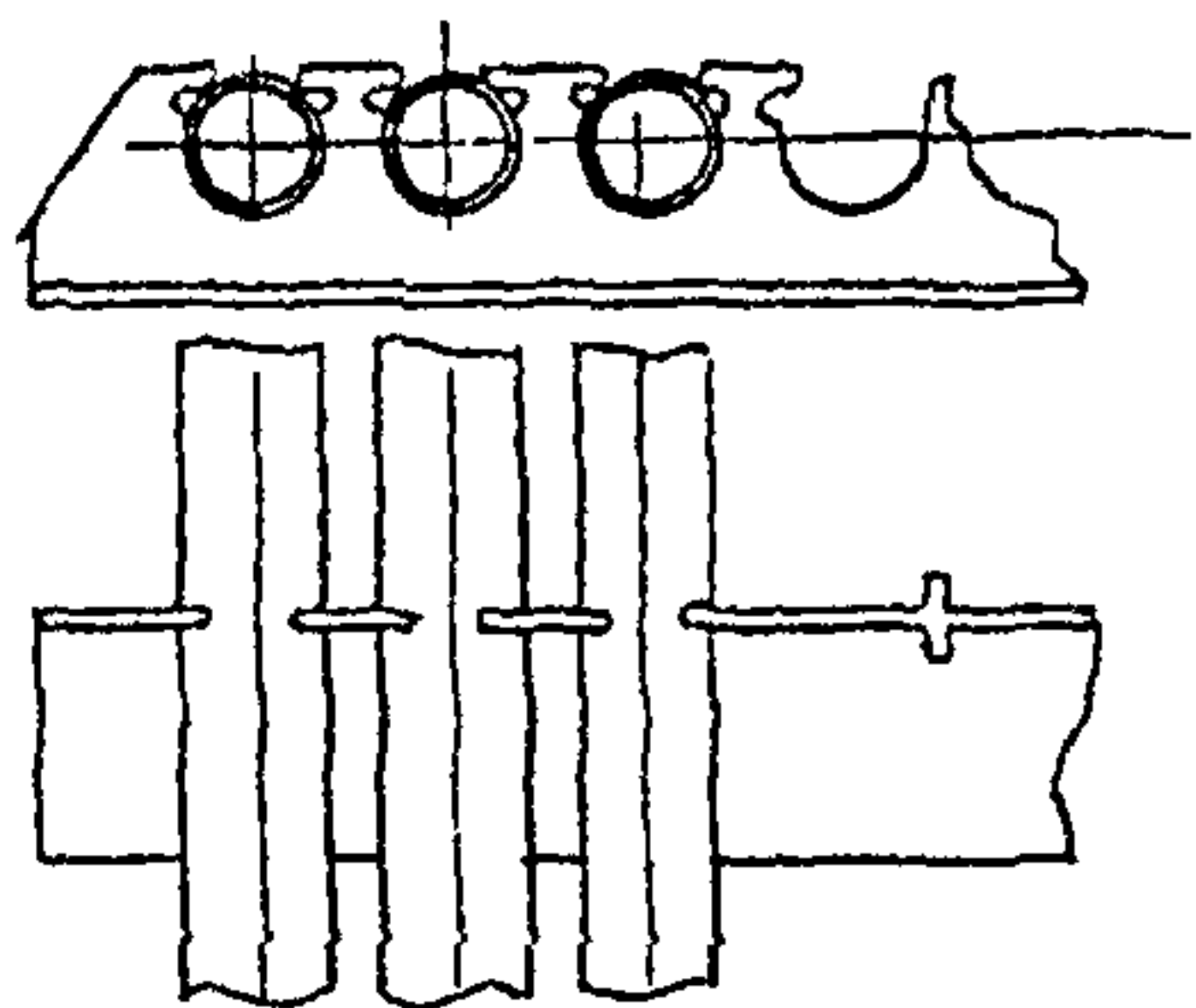
Рис. 12. Схема крепления пластмассовых труб для электропроводок в уголках из листовой стали с фасонными вырезами
