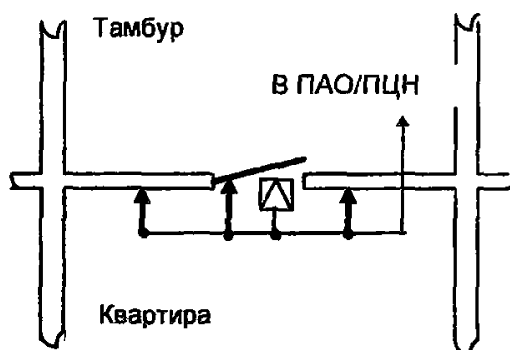
Рисунок 15 - Автономная (централизованная) охрана входной двери квартиры
