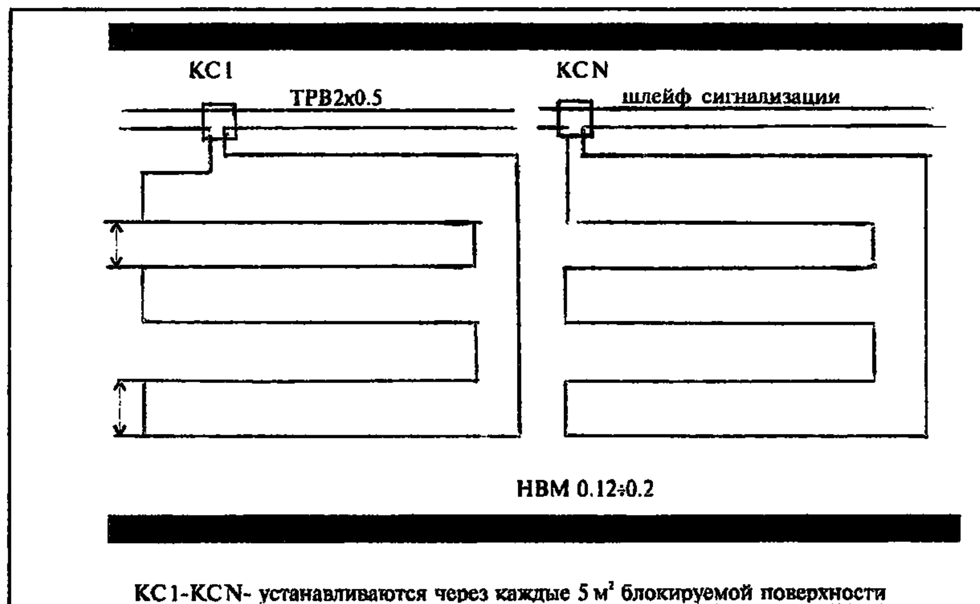
Рисунок 8 - Блокировка стен извещателем омическим типа “Провод”
