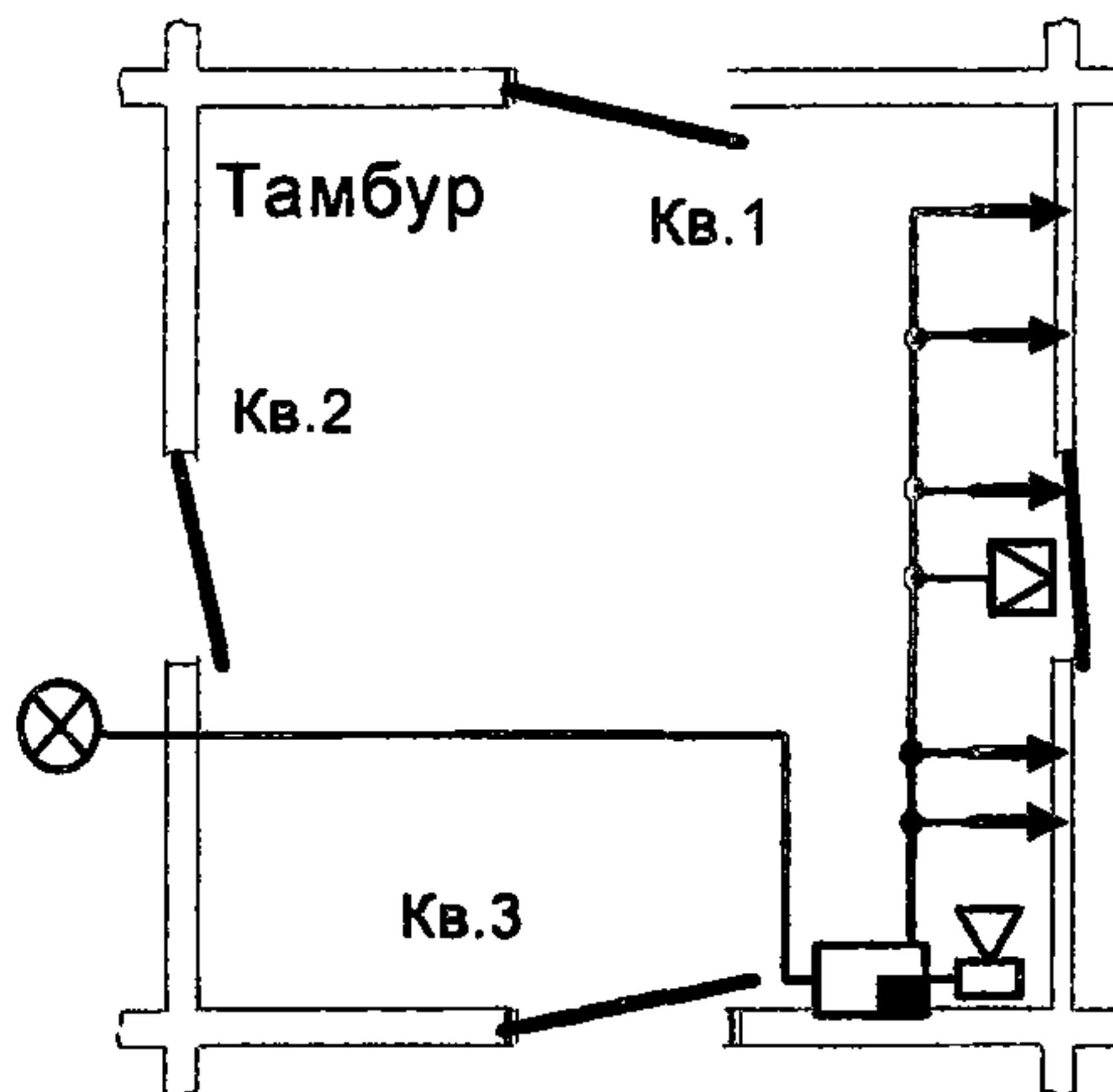
Рисунок 11 - Солидарная охрана двери квартирного тамбура
