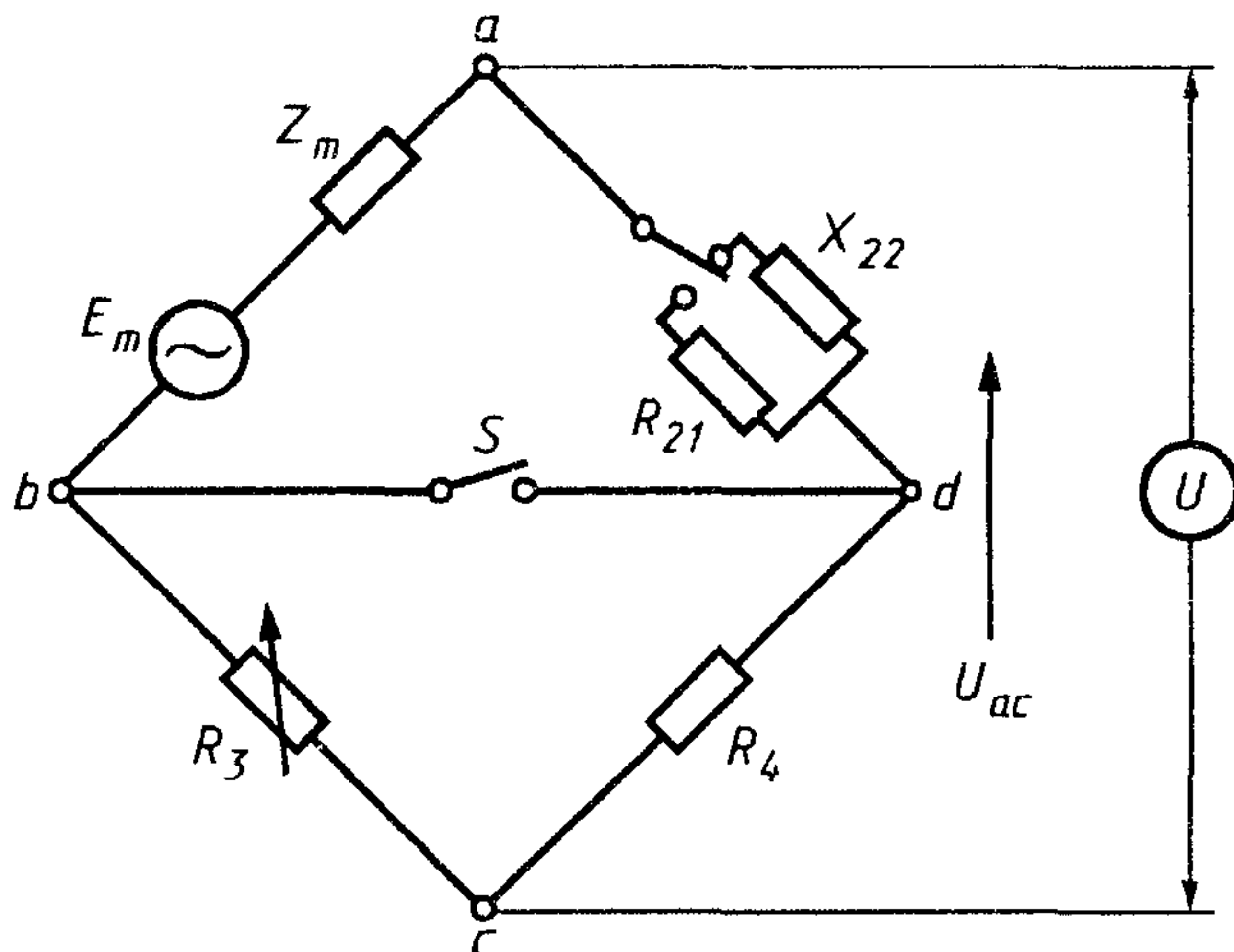
Рисунок J.1 — Мостовая схема
