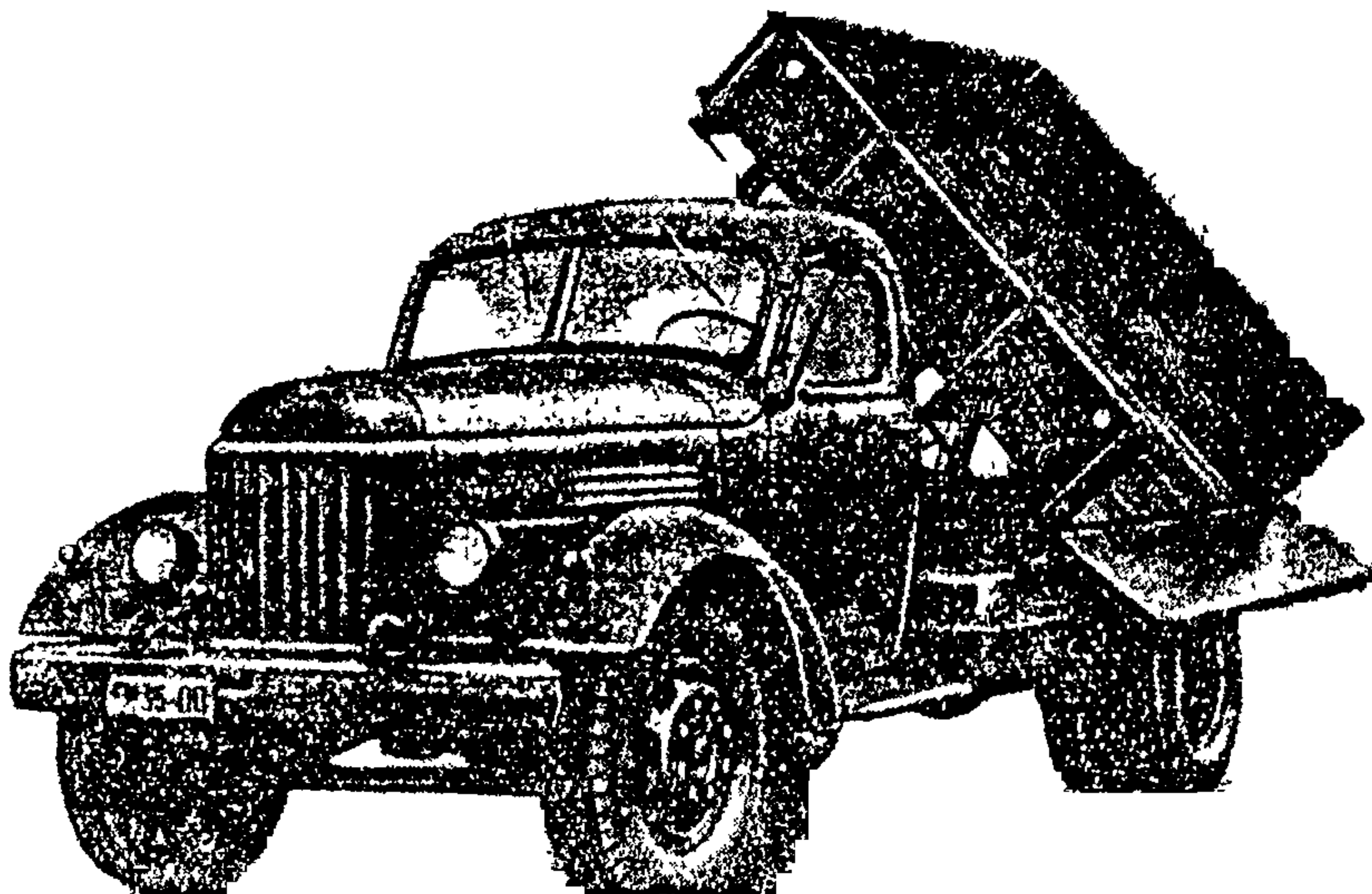
Автомобиль КАЗ-600АВ
