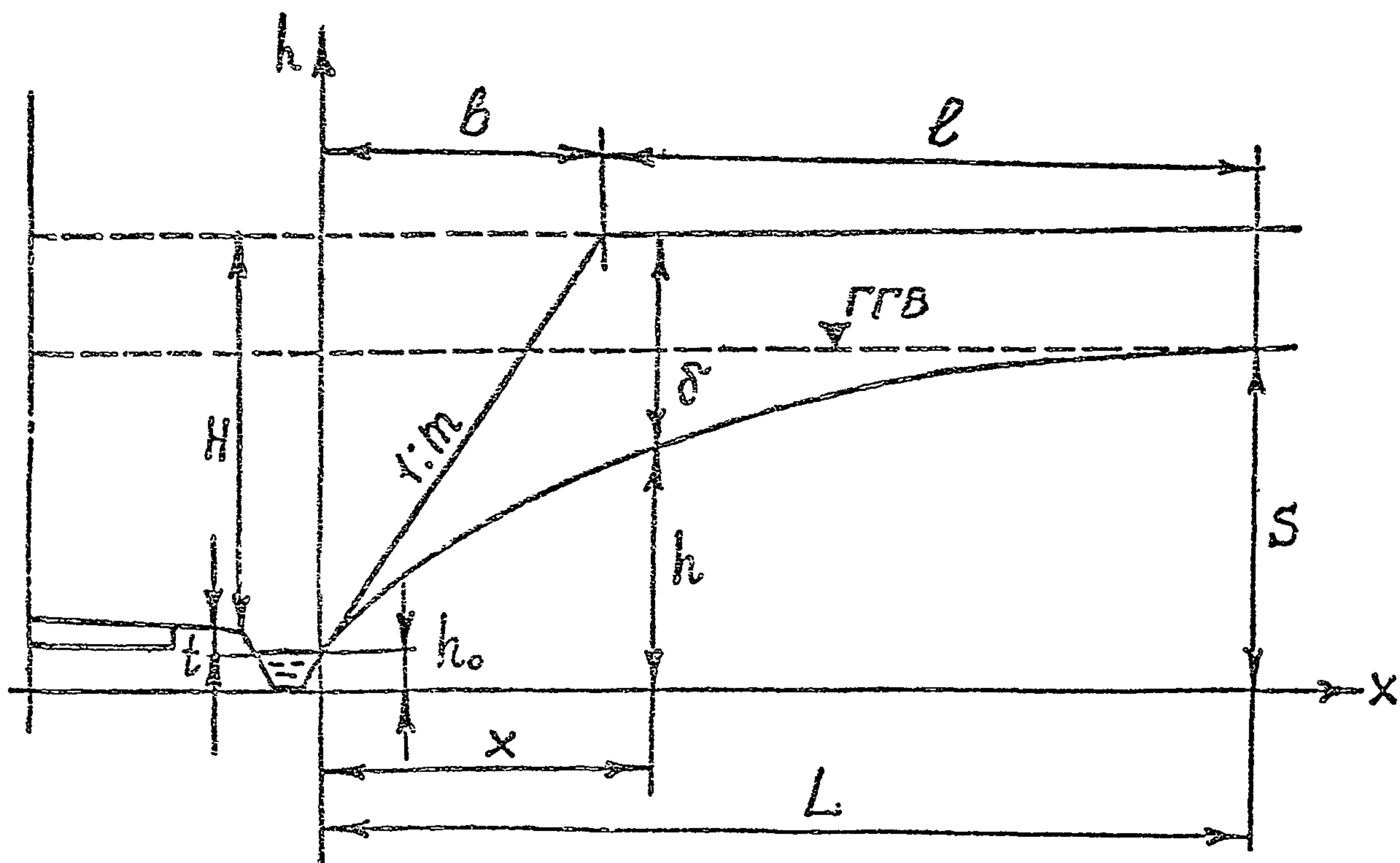
Рис.6.2. Влияние выемки на изменение уровня грунтовых вод.
