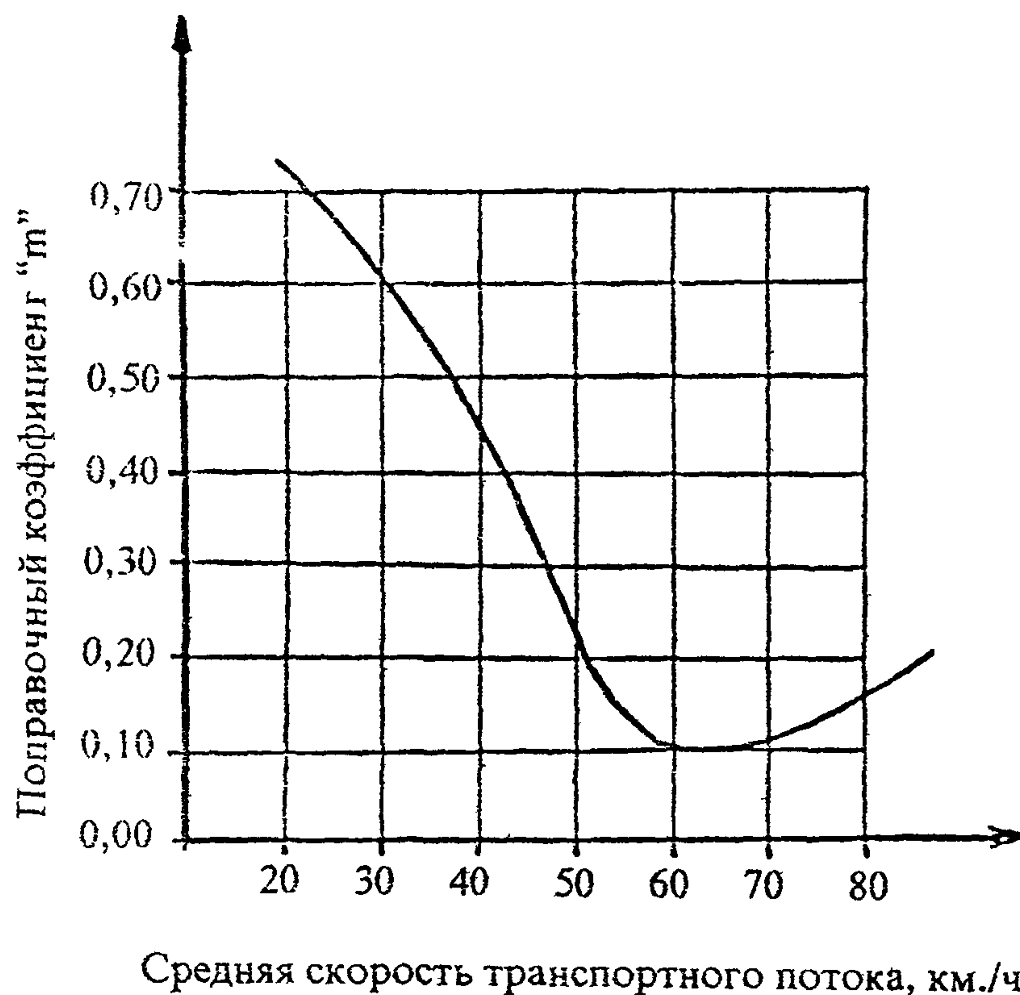
Рис.4.3.1. Зависимость коэффициента "m", учитывающего дорожные и автотранспортные условия движения от средней скорости транспортного потока.
