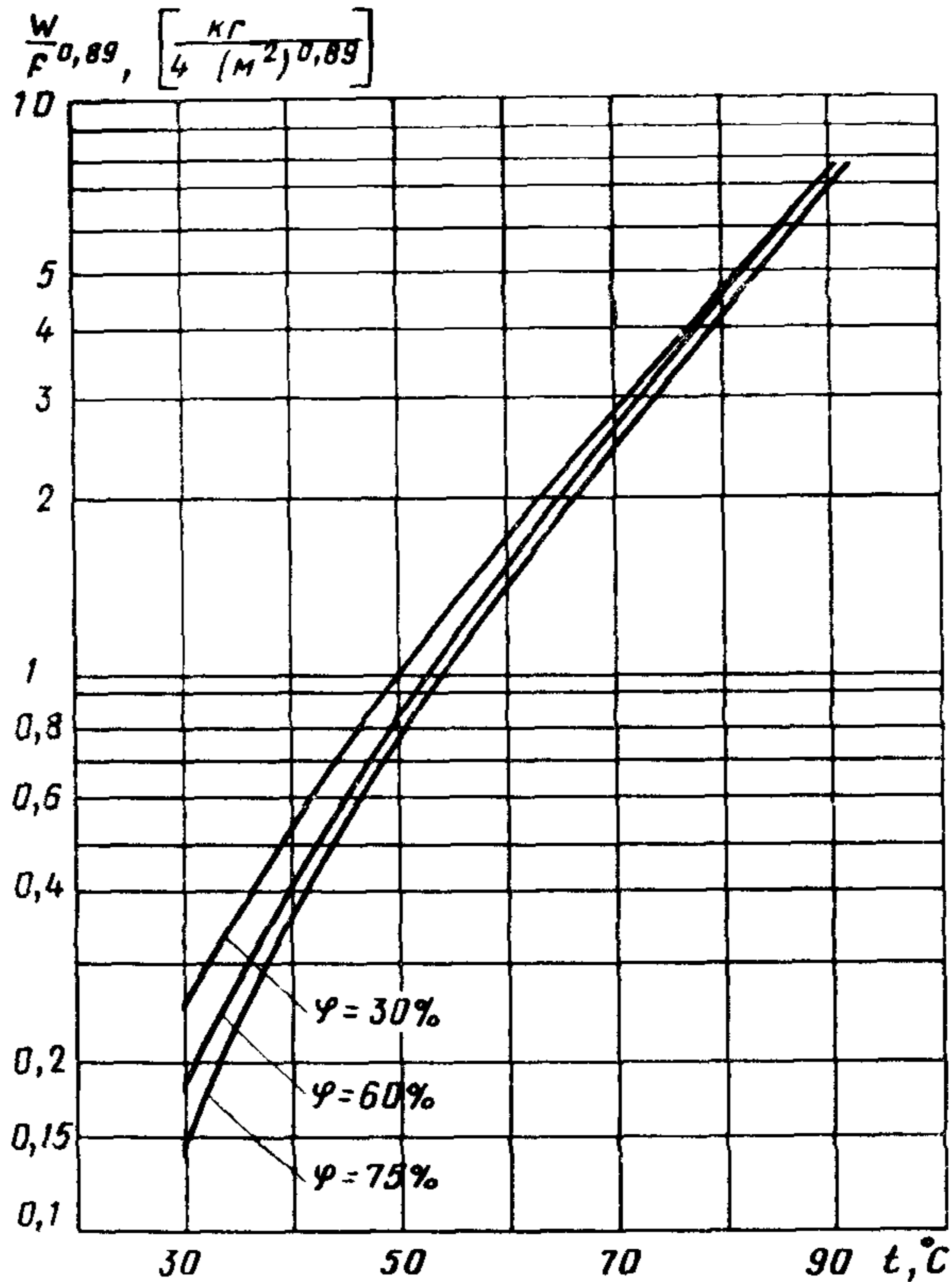
Рис. 4. Влаговыделения с открытой водной поверхности технологического оборудования в зависимости от относительной влажности внутреннего воздуха \varphi , % и температуры воды t , °C, для t_{\text{в}} = 16^{\circ}\text{C} , P_{\delta} = 1,01 \cdot 10^5 \text{ Па}
