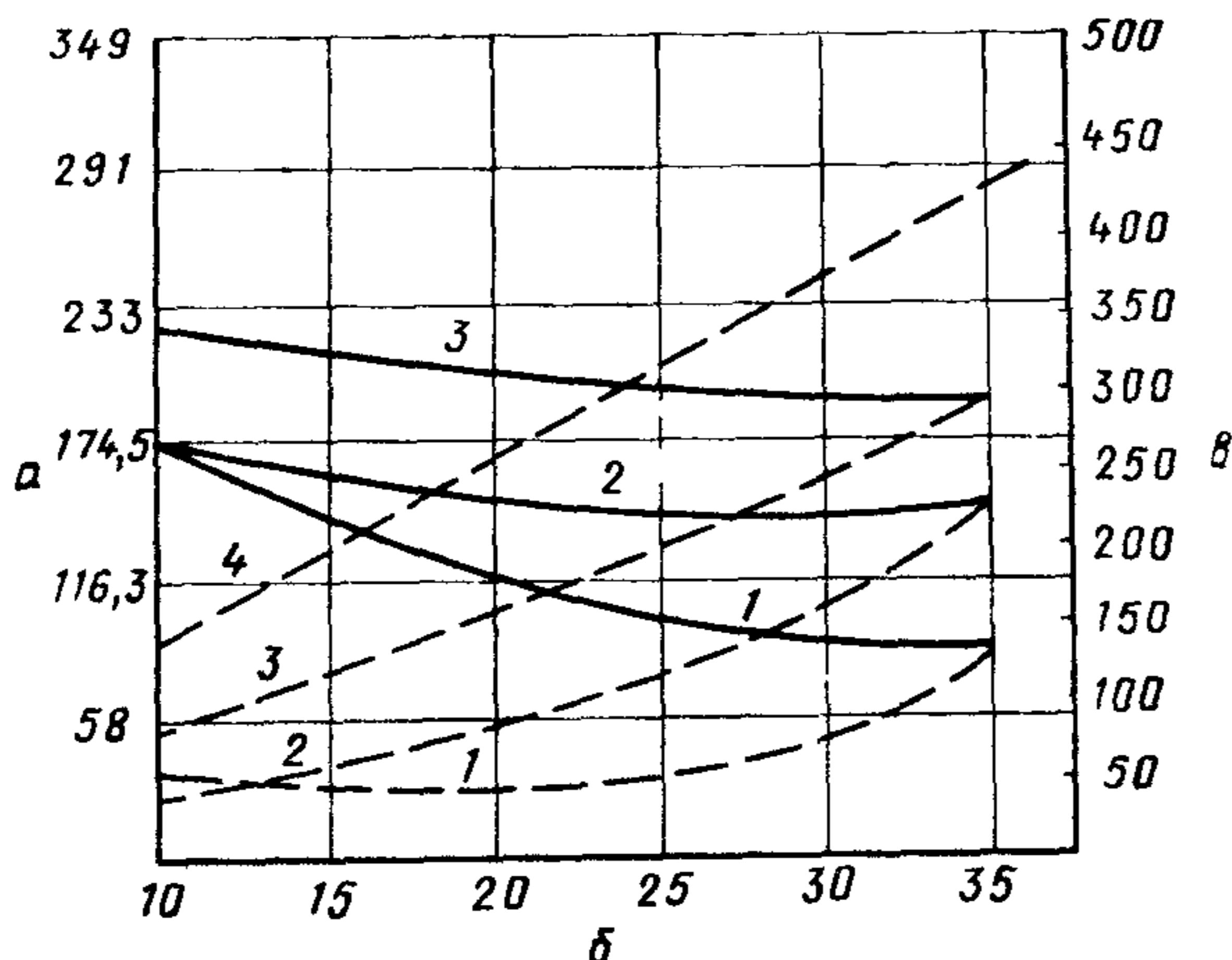
Рис. 3. Зависимость количества тепла и влаги, выделяемых человеком, от температуры воздуха в помещении и характера работы a – тепловыделение, Вт; б – температура воздуха, °С; в – влаговыделение, г/ч — — полное количество тепла, - - - - тепло, идущее на испарение влаги; 1 – человек в покое; 2 – легкая работа в учреждении; 3 – физическая работа; 4 – тяжелая физическая работа
