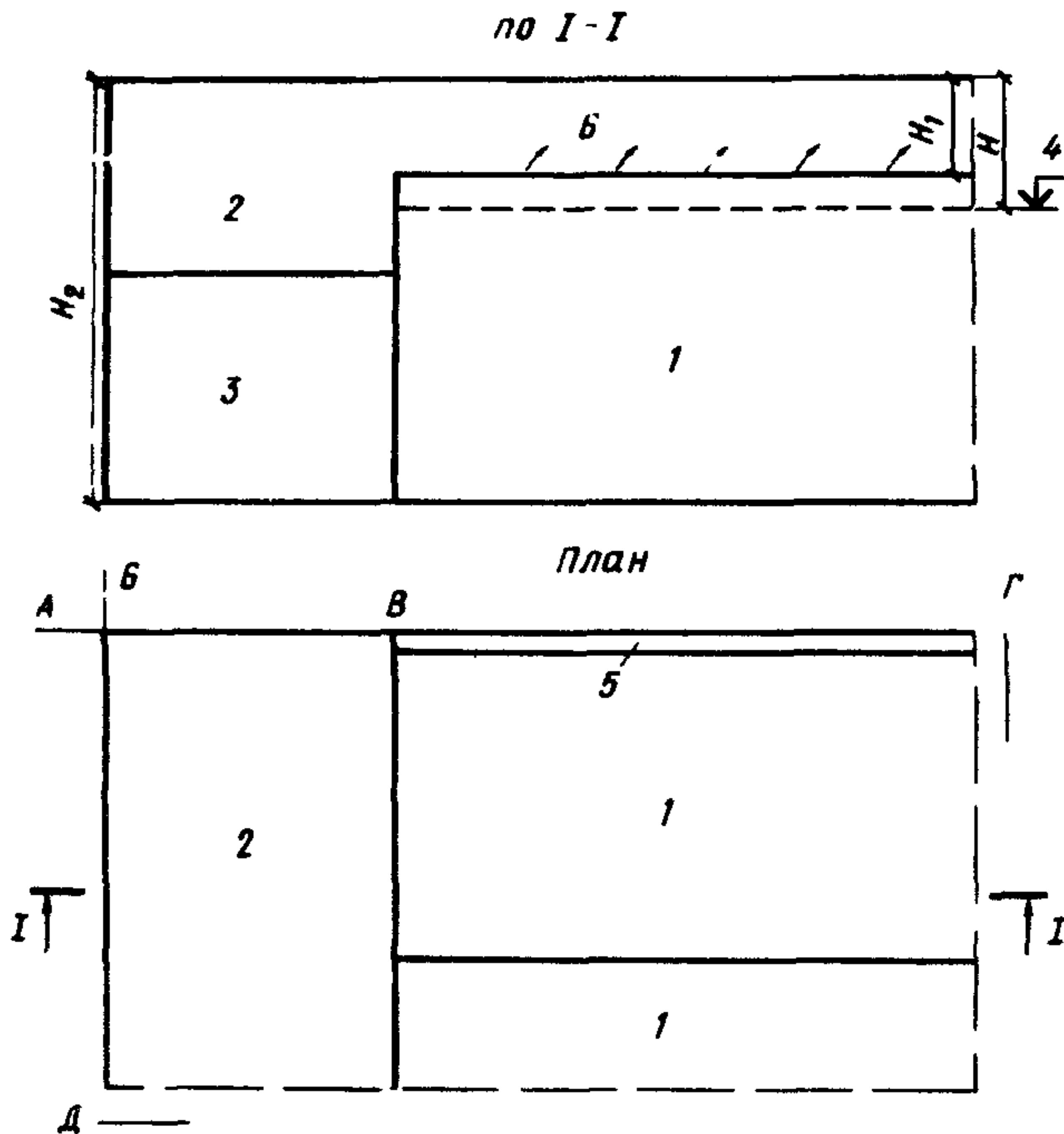
Рис. 1. Фрагменты схем сечения картофелехранилища H – высота верхней зоны; 1 – секция хранения; 2 – венткамера в общем объеме верхней зоны; 3 – технологический проезд; 4 – уровень верха насыпи; 5 – вентилируемая прослойка; 6 – выход воздуха из прослойки
