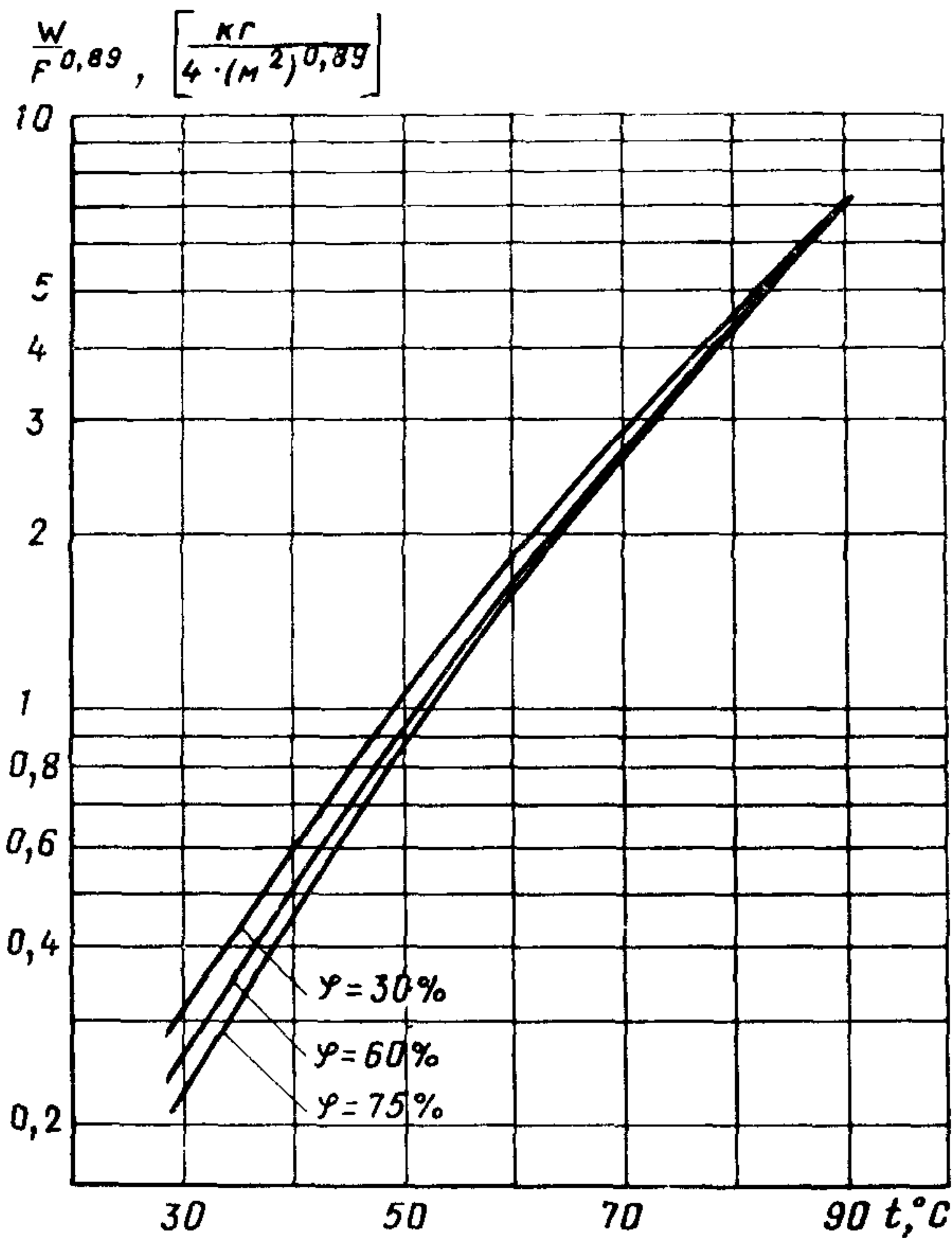
Рис. 5. Влаговыделения с открытой водной поверхностью технологического оборудования в зависимости от относительной влажности внутреннего воздуха \varphi , %, и температура воды t , ^{\circ}\text{C} , для t_{\text{в}} = 22^{\circ}\text{C} и P_{\delta} = 1,01 \cdot 10^5 \text{ Па}
