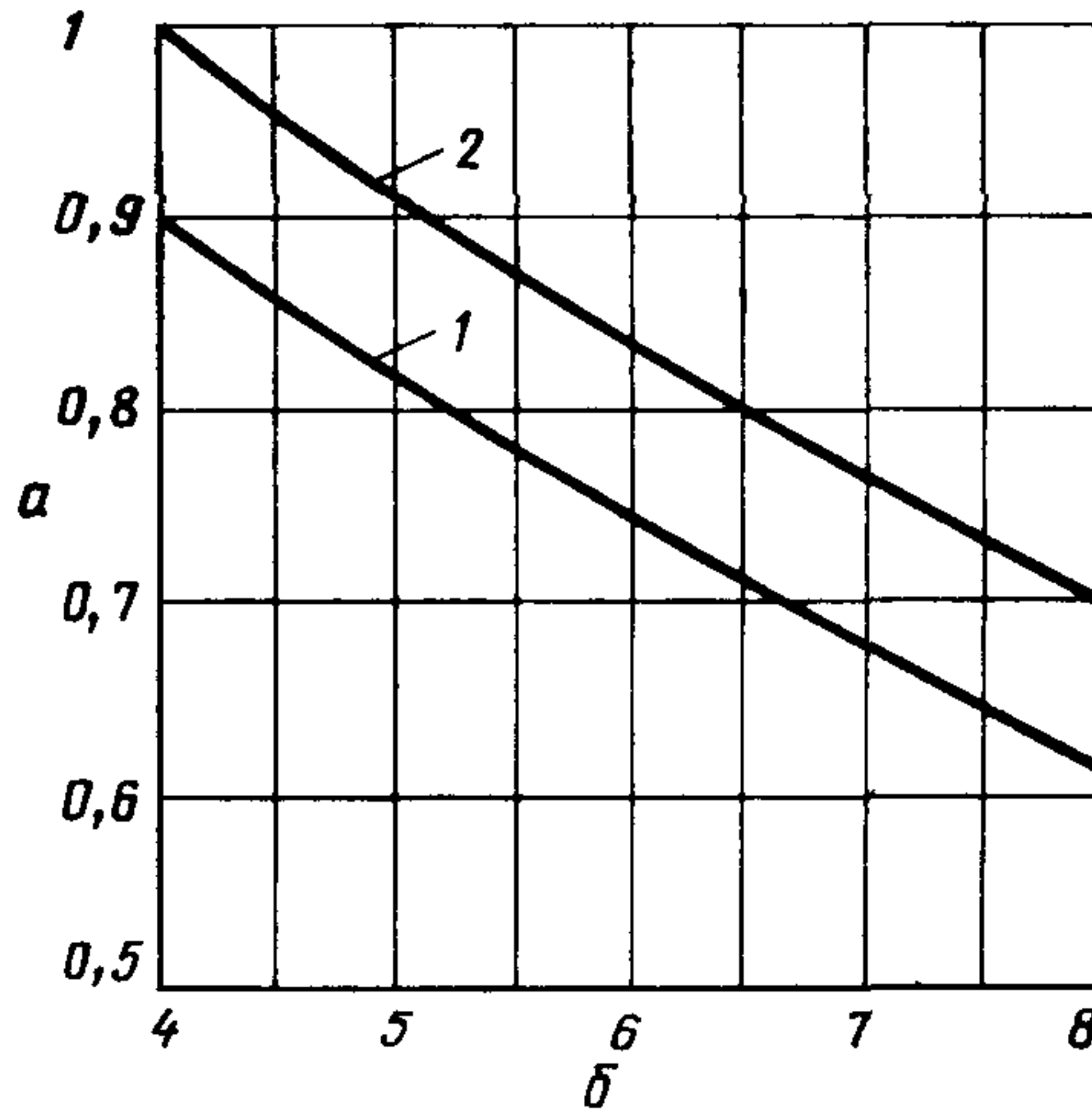
Рис. 2 Средние значения температурного градиента \Delta , ^{\circ}\text{C}/\text{м} , в зависимости от высоты помещения и теплонапряженности q , \text{Вт}/\text{м}^3 a – температурный градиент \Delta , ^{\circ}\text{C}/\text{м} ; b – высота помещения, м; 1 – до 23 \text{ Вт}/\text{м}^3 ; 2 – до 46 \text{ Вт}/\text{м}^3
