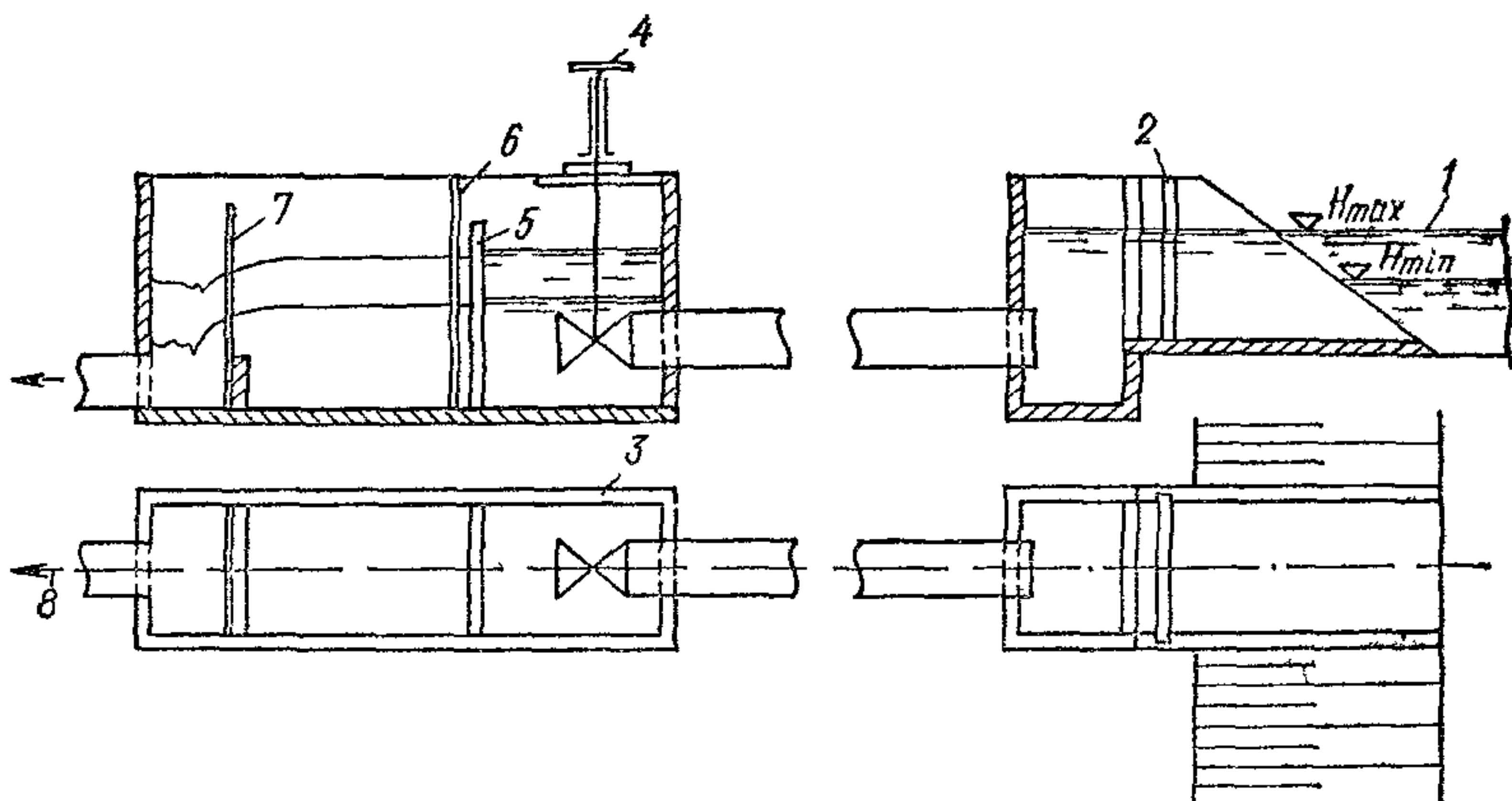
Рис. 51. Схема входного узла с водосливом
