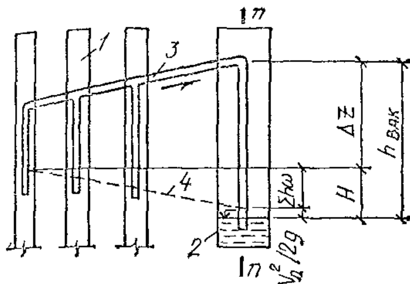
Рис. 94. Схема сифонного водовода 1 — скважины; 2 — приемный или сборный резервуар; 3 — сифонный трубопровод; 4 — пьезометрическая линия
