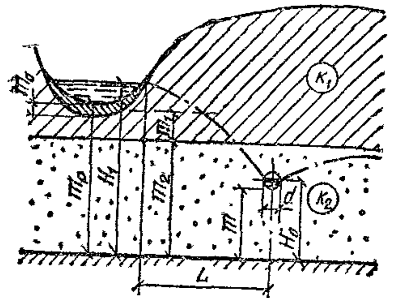
Рис. 24. Схема к расчету горизонтального водозабора в двухслойном полуограниченном водоносном пласте
