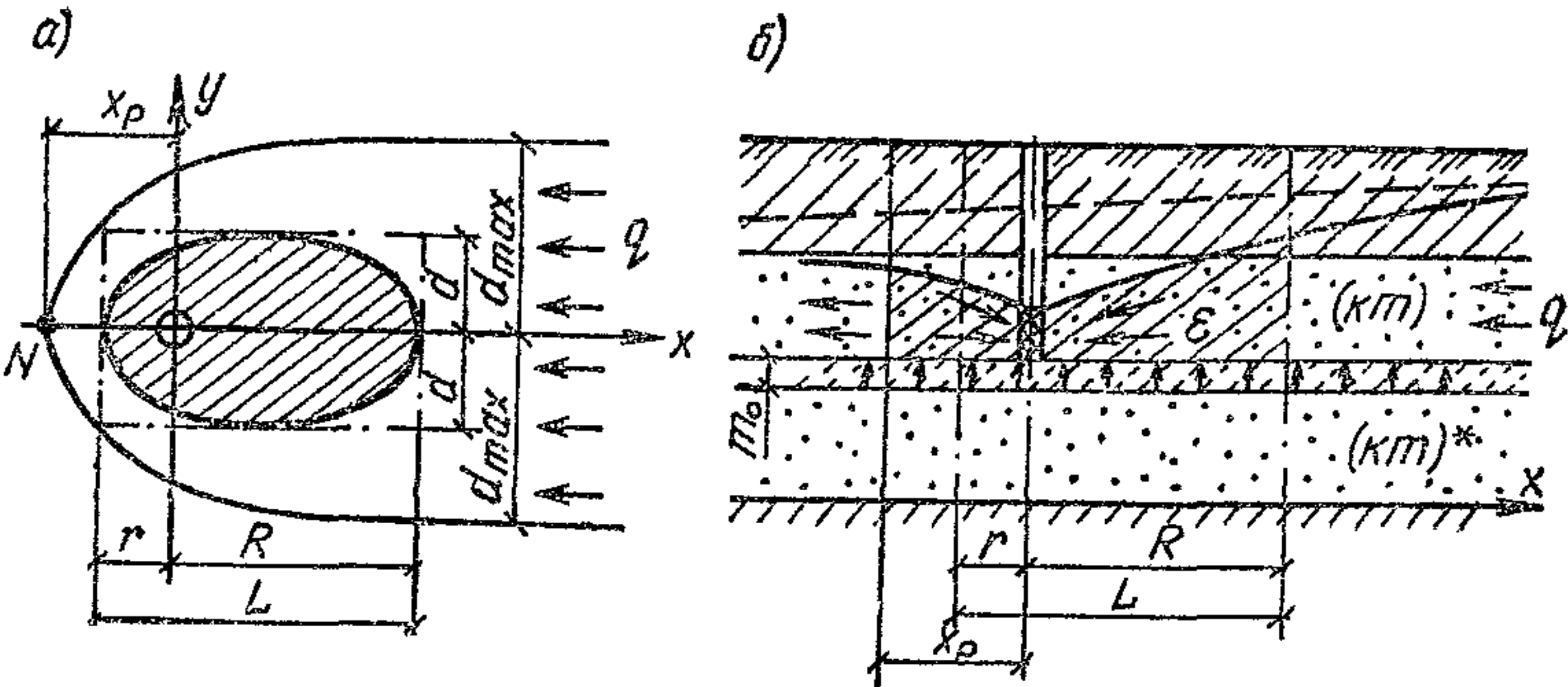
Рис. 86. Схемы фильтрации в водозаборе в условиях дополнительного питания пласта
