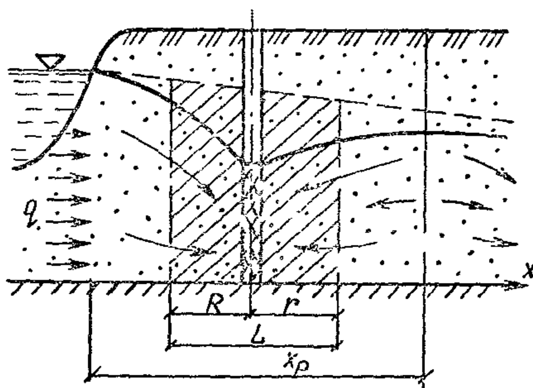
Рис 72. Схема фильтрации к береговому сосредоточенному водозабору при естественном потоке, направленном от реки
