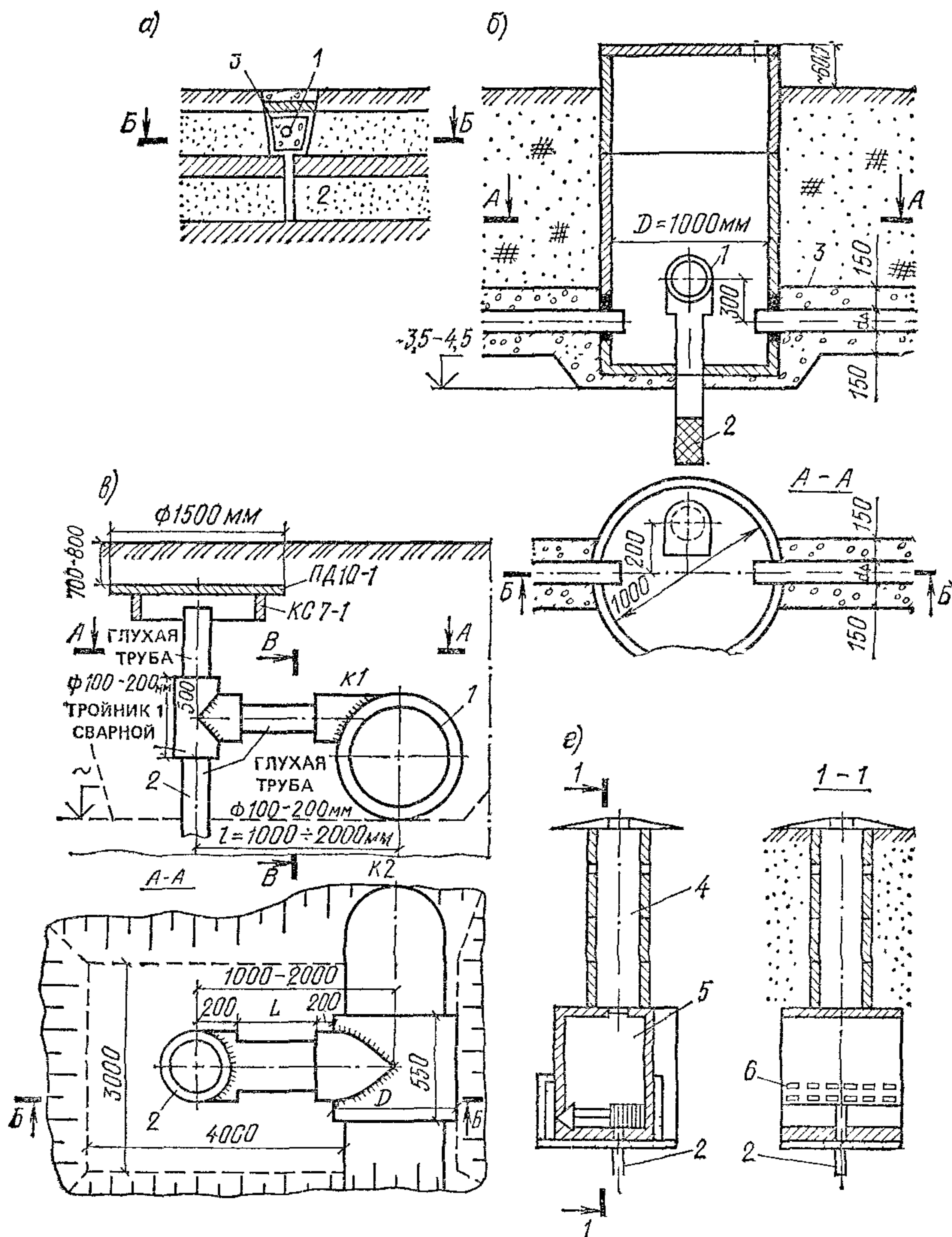
Рис. 20. Комбинированный горизонтальный водозабор с вертикальными скважинами-усилителями
