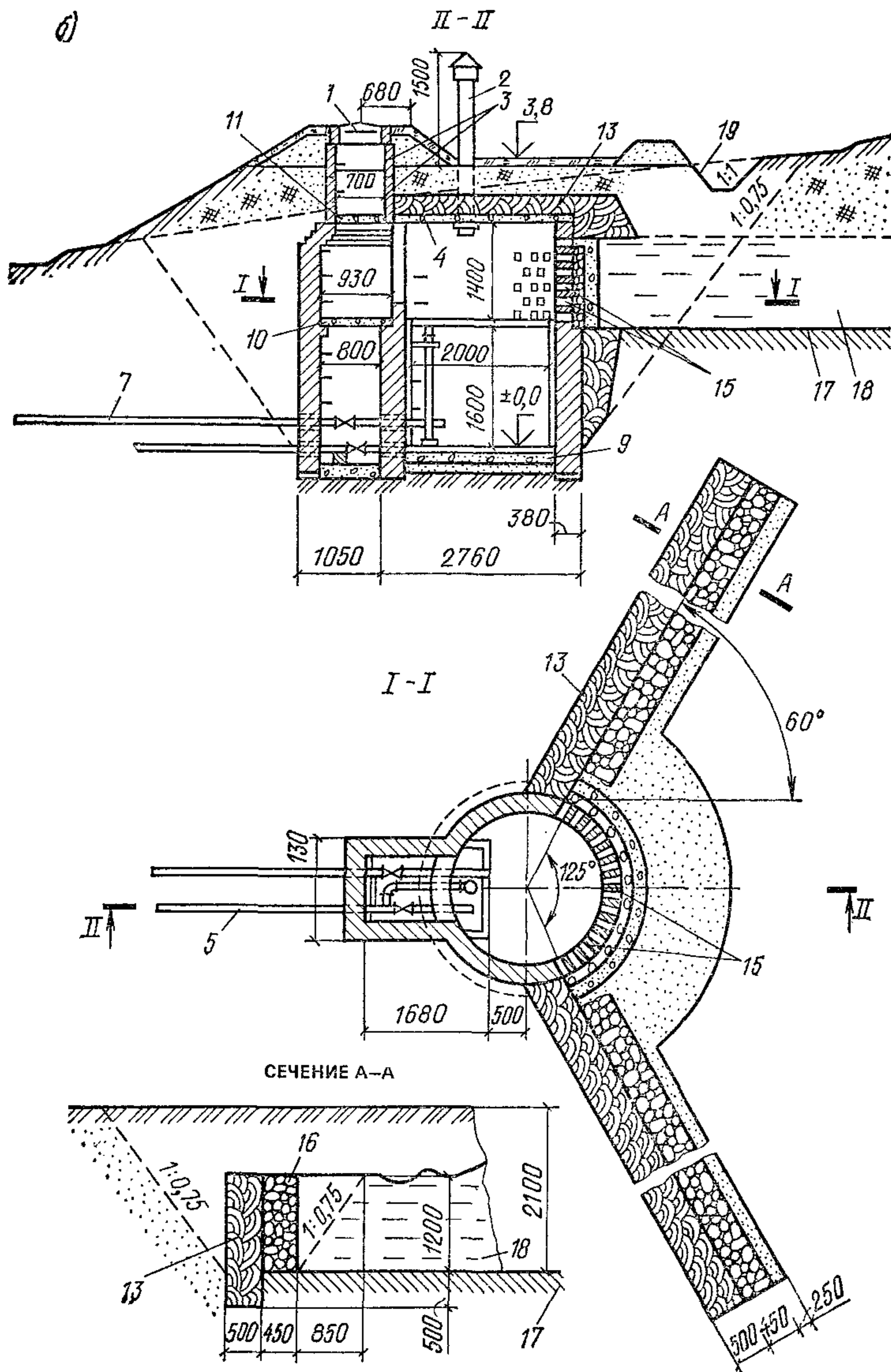
Рис 44. Кирпичная каптажная камера
