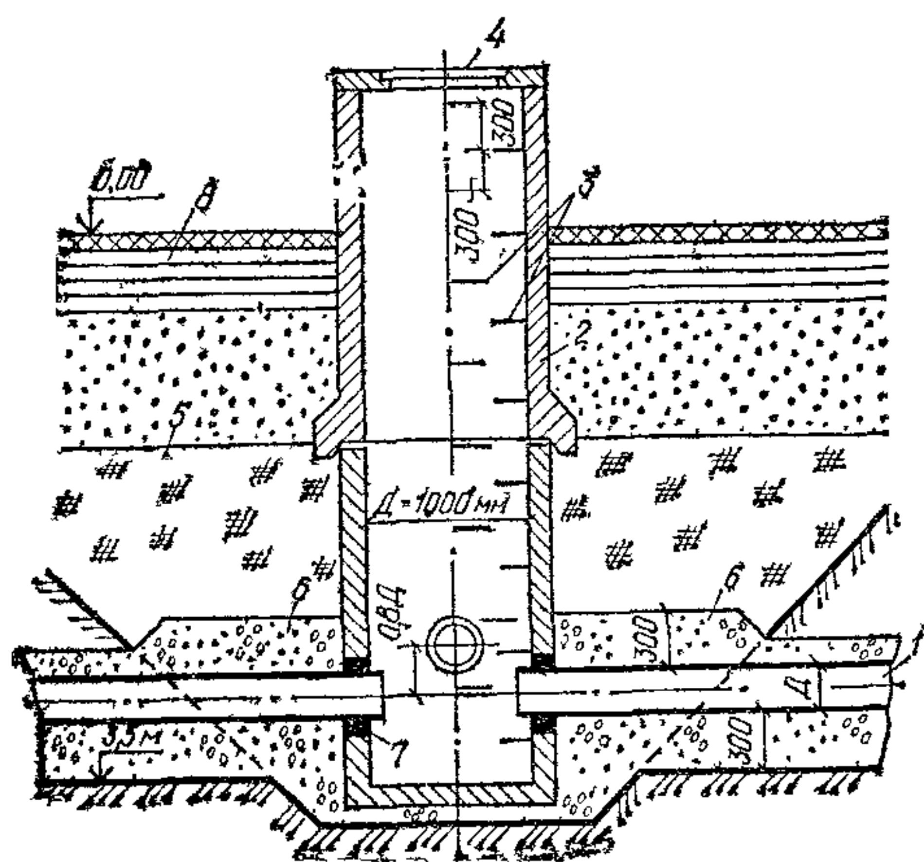
Рис. 21. Смотровой колодец (типовой проект Гипроводхоза)
