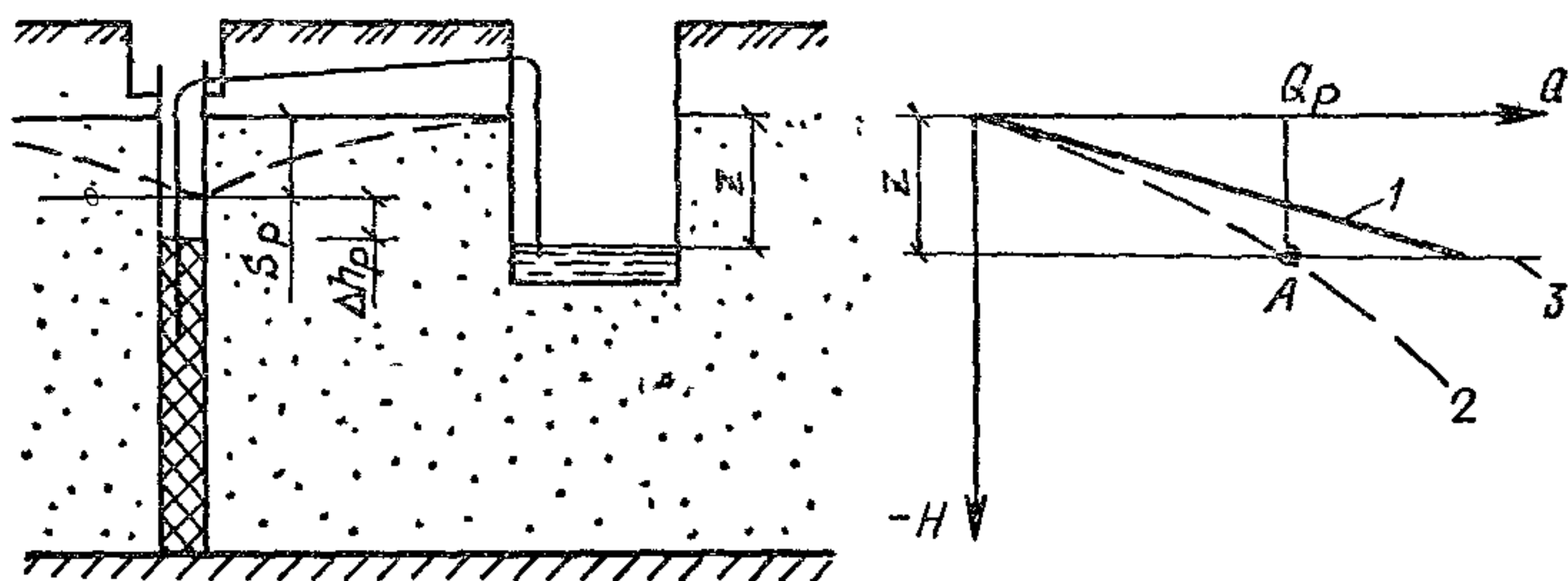
Рис. 104. Схема и расчету скважин при сифонном водоотборе Q_p — координаты точки A на оси Q ; S_p — расчетное понижение уровня воды в скважине; \Delta h_p — расчетные потери напора в водоводе; z — разность между уровнем грунтовых вод и отметкой воды в резервуаре; 1 — характеристика Q-H скважины; 2 — характеристика Q-H скважины и водовода; 3 — линия отметки воды в резервуаре
