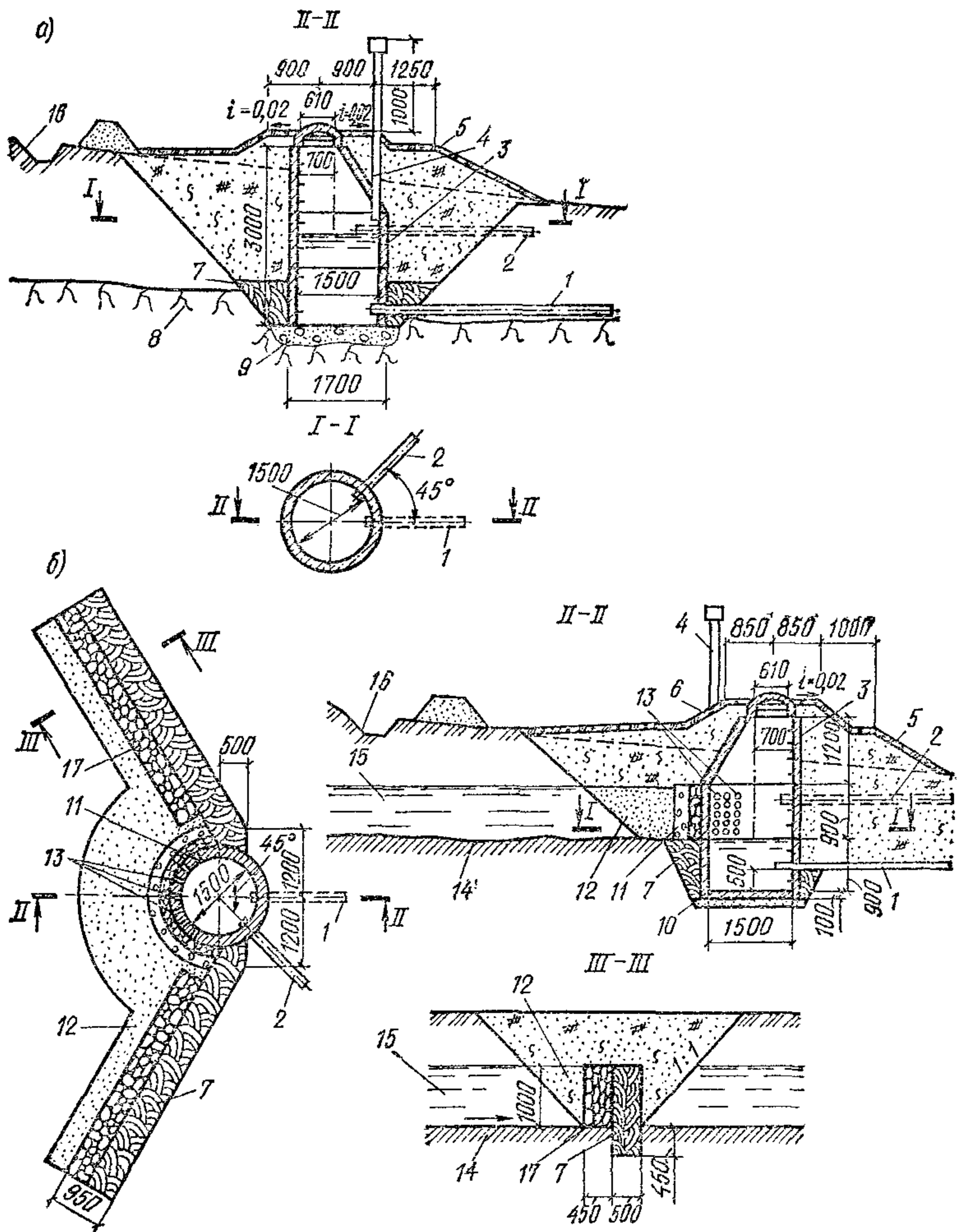
Рис. 43. Железобетонная каптажная камера
