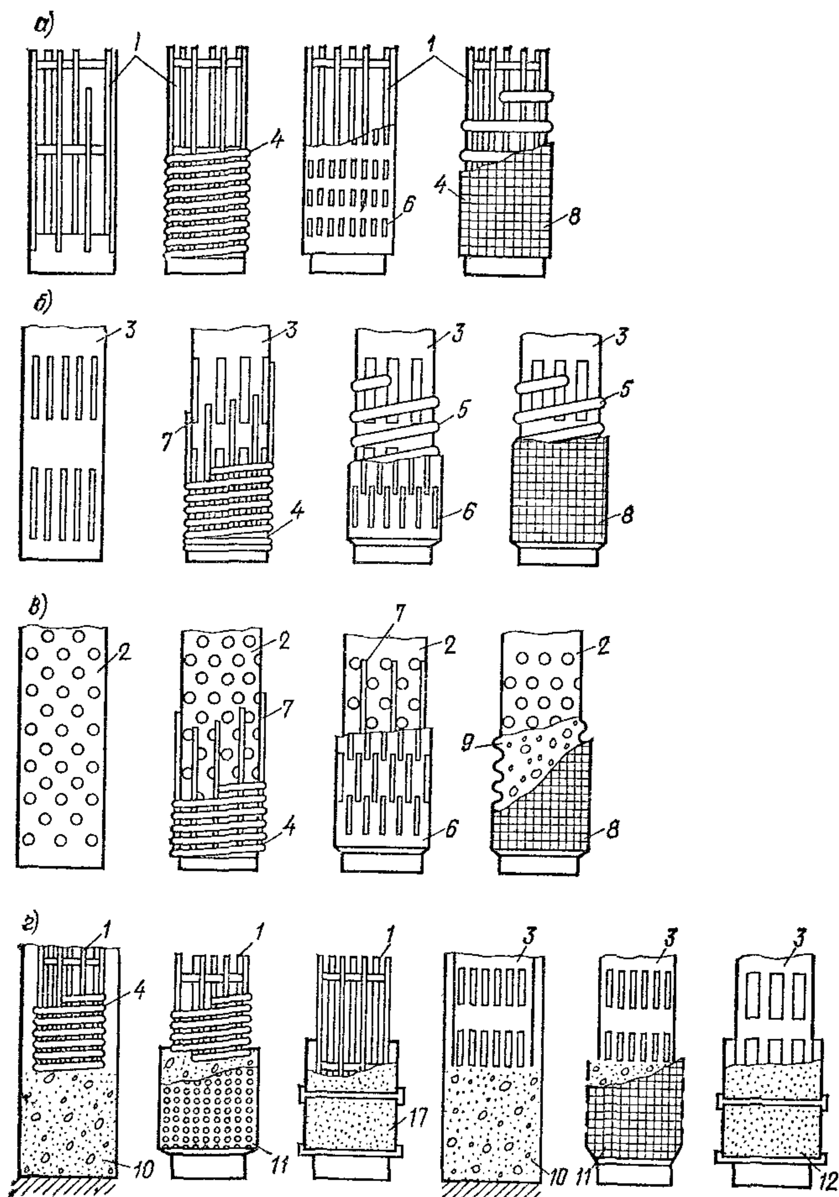
Рис. 9. Основные схемы конструкций фильтров водозаборных скважин а — на основе стержневых каркасов; б — на основе трубчатых каркасов со щелевой перфорацией; в — на основе трубчатых каркасов с круглой перфорацией; г — гравийные фильтры; 1 — стержневой каркас на опорных кольцах; 2 — трубчатый каркас с круглой перфорацией; 3 — щелевой трубчатый каркас; 4 — проволоочная обмотка из нержавеющей стали; 5 — опорная проволоочная спираль; 6 — лист, штампованный из нержавеющей стали; 7 — опорные проволоочные стержни под проволоочную обмотку и лист; 8 — сетка из нержавеющей стали или латуни; 9 — сетка подкладная, синтетическая; 10 — рыхлая обсыпка; 11 — гравийная обсыпка в кожухе; 12 — гравийный блок
