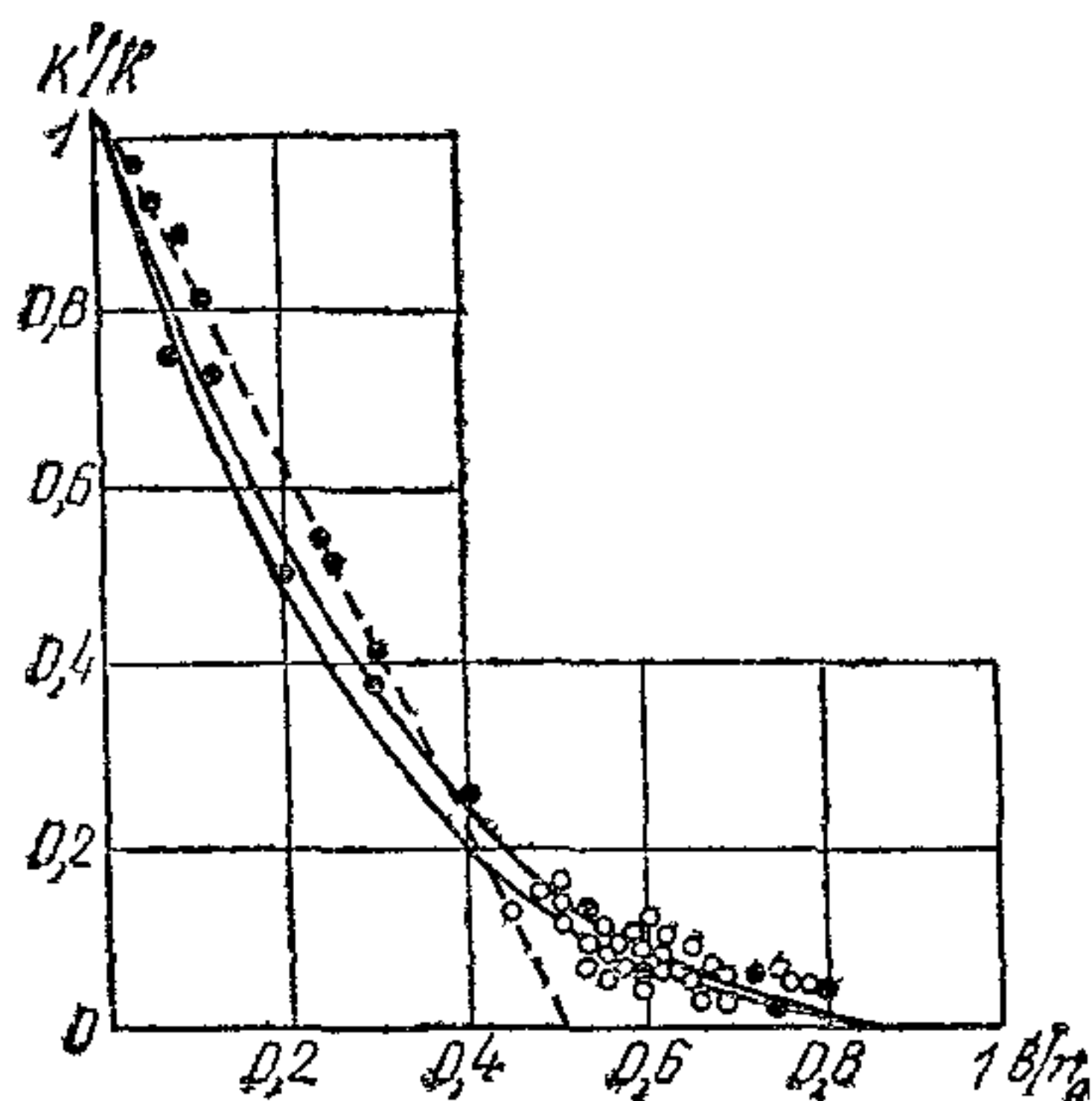
Рис. 59. Графики роста сопротивления скважин
