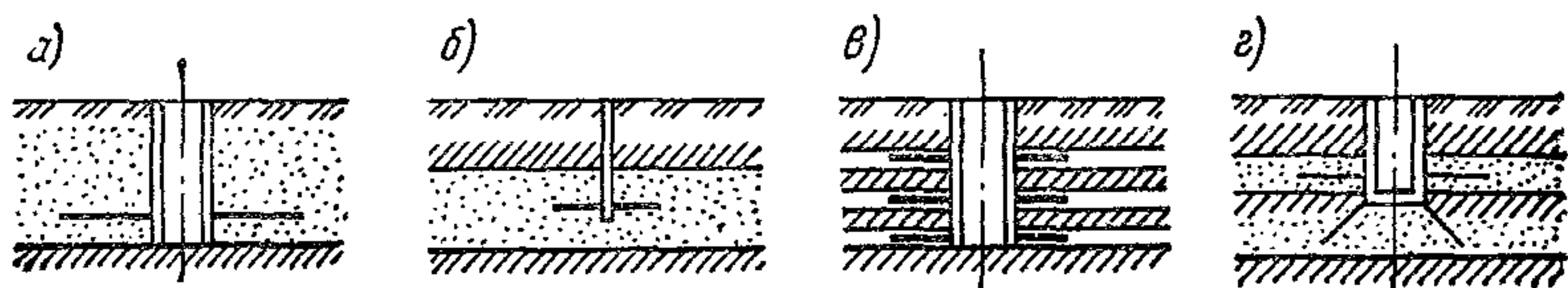
Рис. 36. Схемы лучевых водозаборов в разрезе
