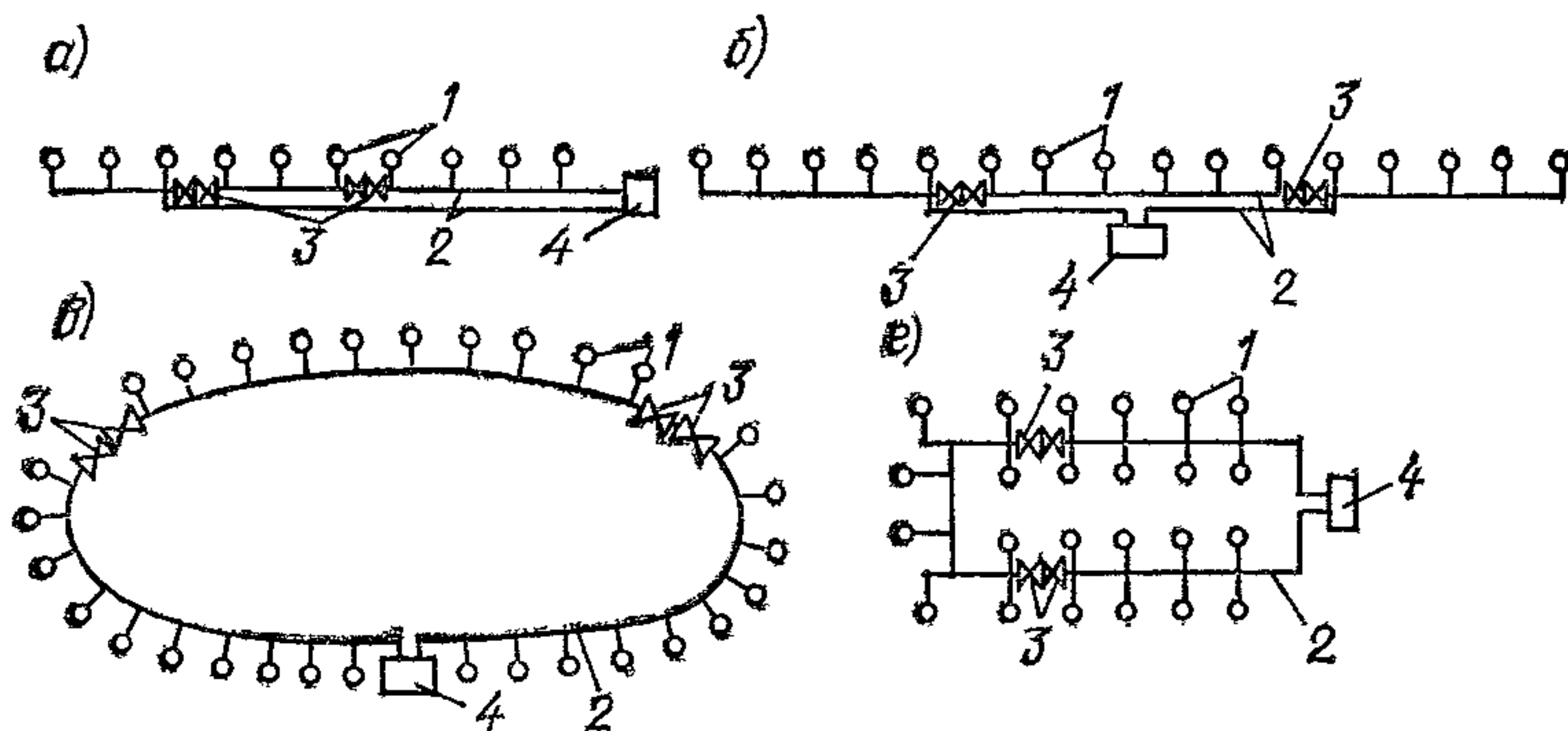
Рис. 91. Схемы кольцевых сборных водоводов
