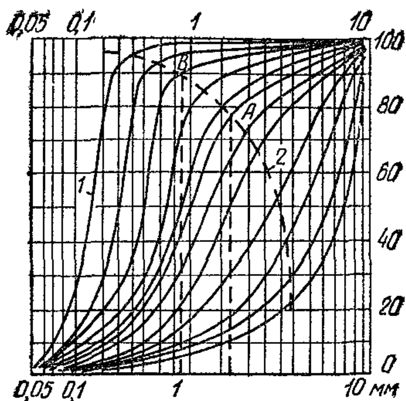
Рис. 11. График для определения состава гравийной обсыпки
