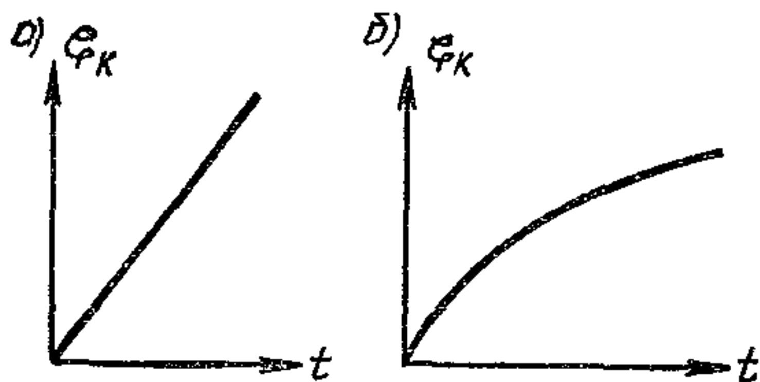
Рис. 59. Графики роста сопротивления скважин
