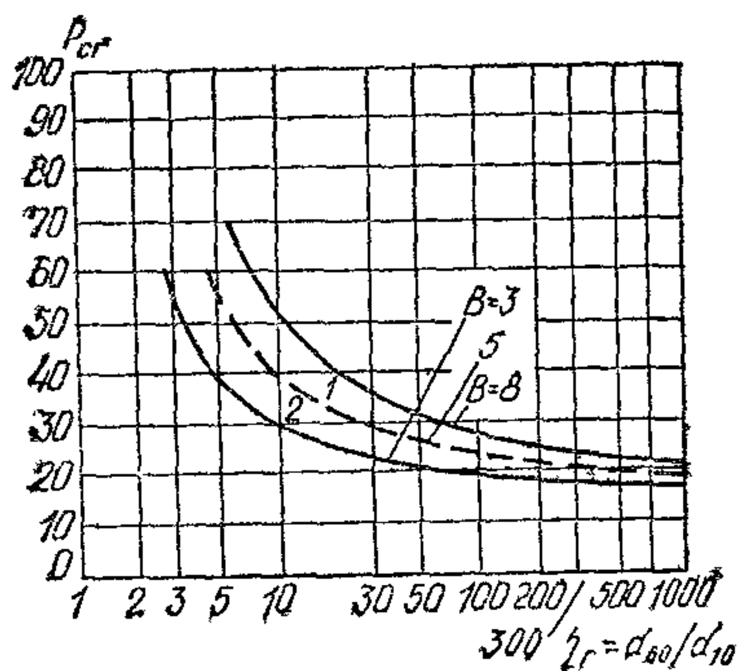
Рис. 31. График P_{ср}^{расч} = f(\eta) для определения расчетных размеров сводообразующих частиц грунта d_{ср} 1 — область выбора расчетных значений d_{ср} для фильтров из щебеночного материала; 2 — область выбора расчетных значений d_{ср} для фильтров из песчано-гравийно-галечникового грунта
