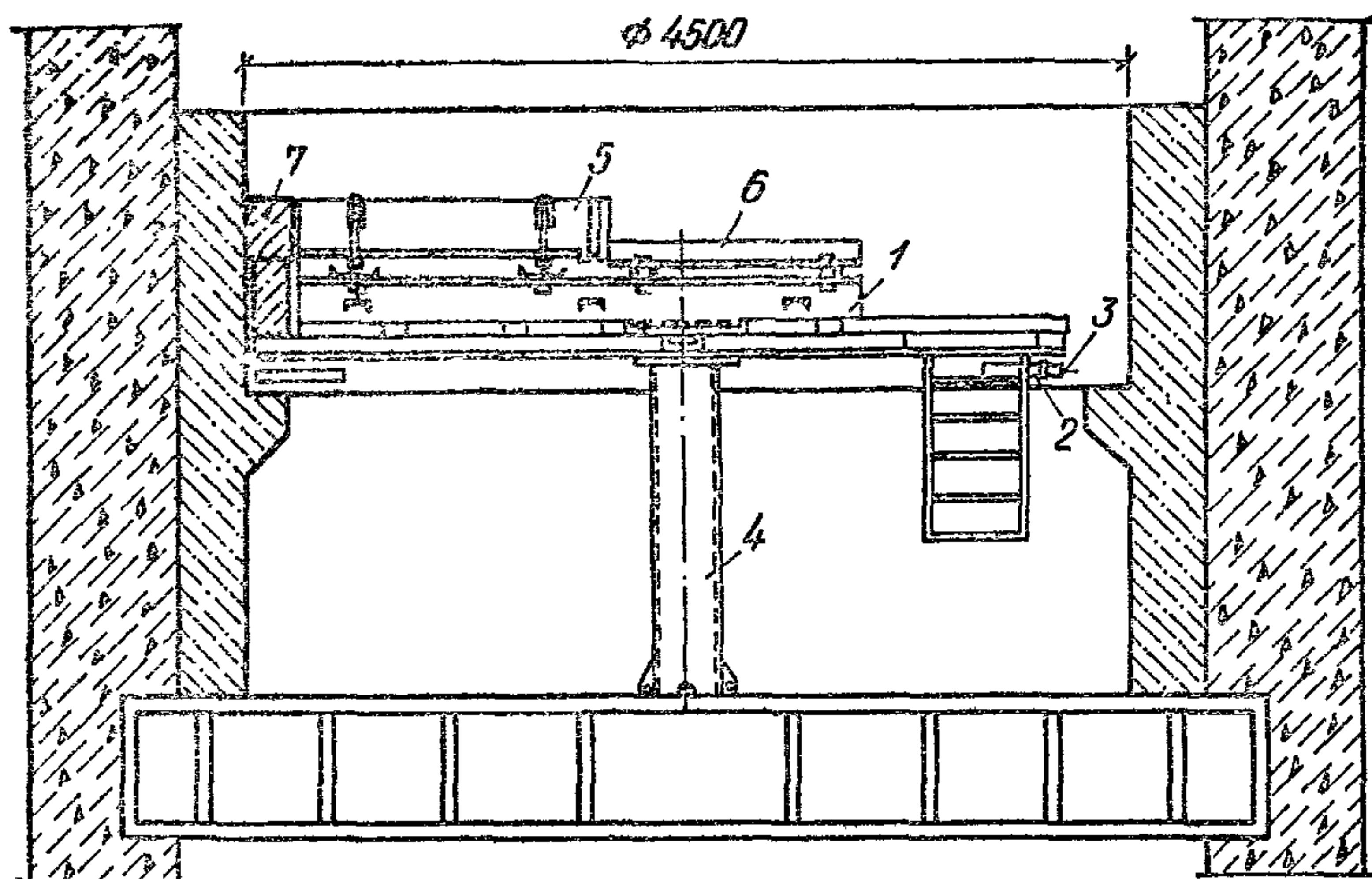
Рис. 41. Рабочая площадка лучевого водозабора
