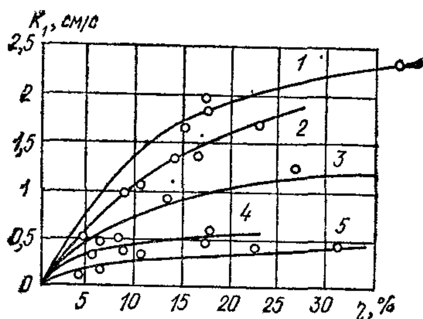
Рис. 10. Изменение проницаемости различных фильтров от скважности 1 — каркасно-стержневого; 2 — проволочного на трубчатом каркасе; 3 — с мостообразными отверстиями; 4 — с водоприемной поверхностью из штампованного листа; 5 — с сеткой галунного плетения
