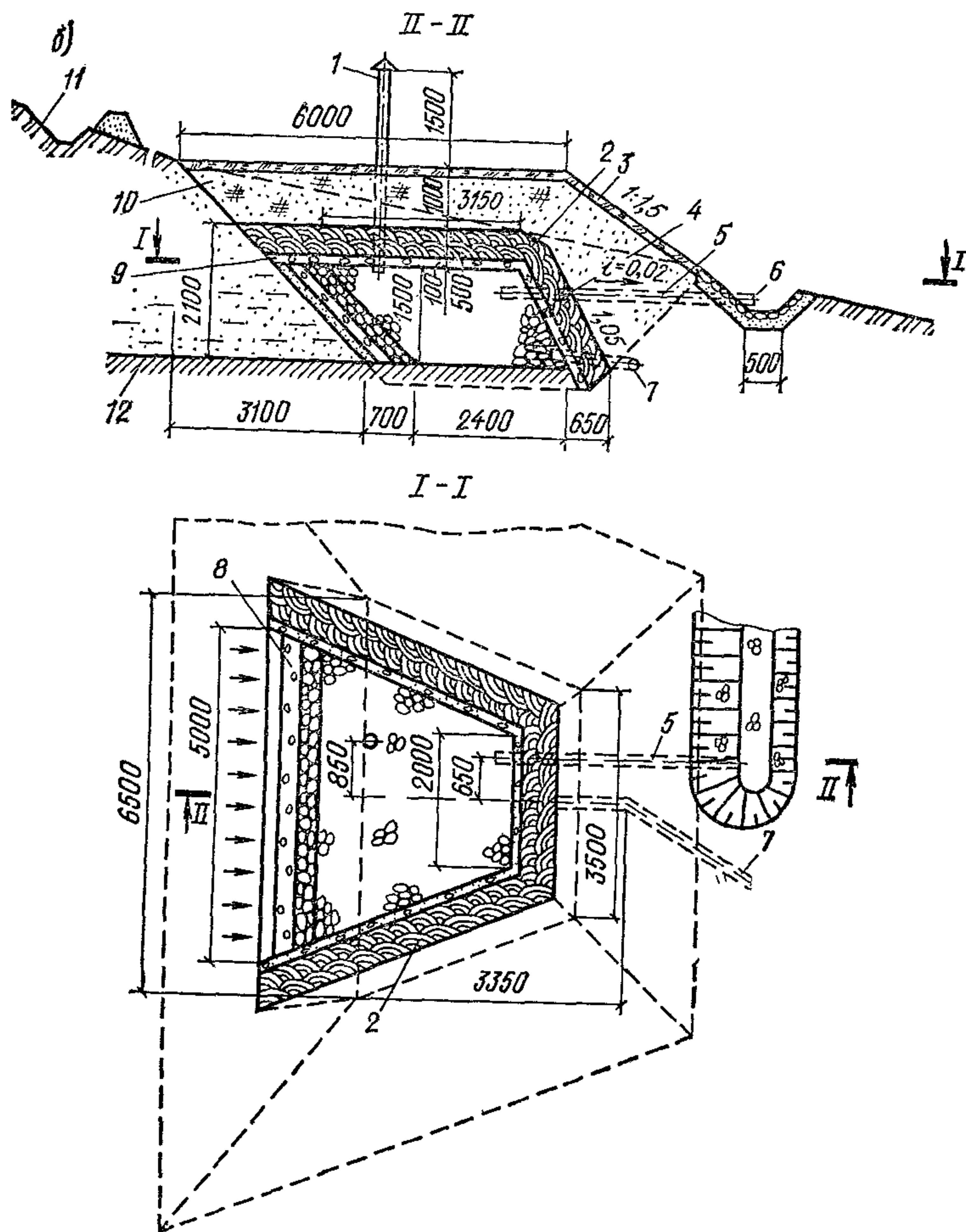
Рис. 45. Глиняно-каменная каптажная камера
