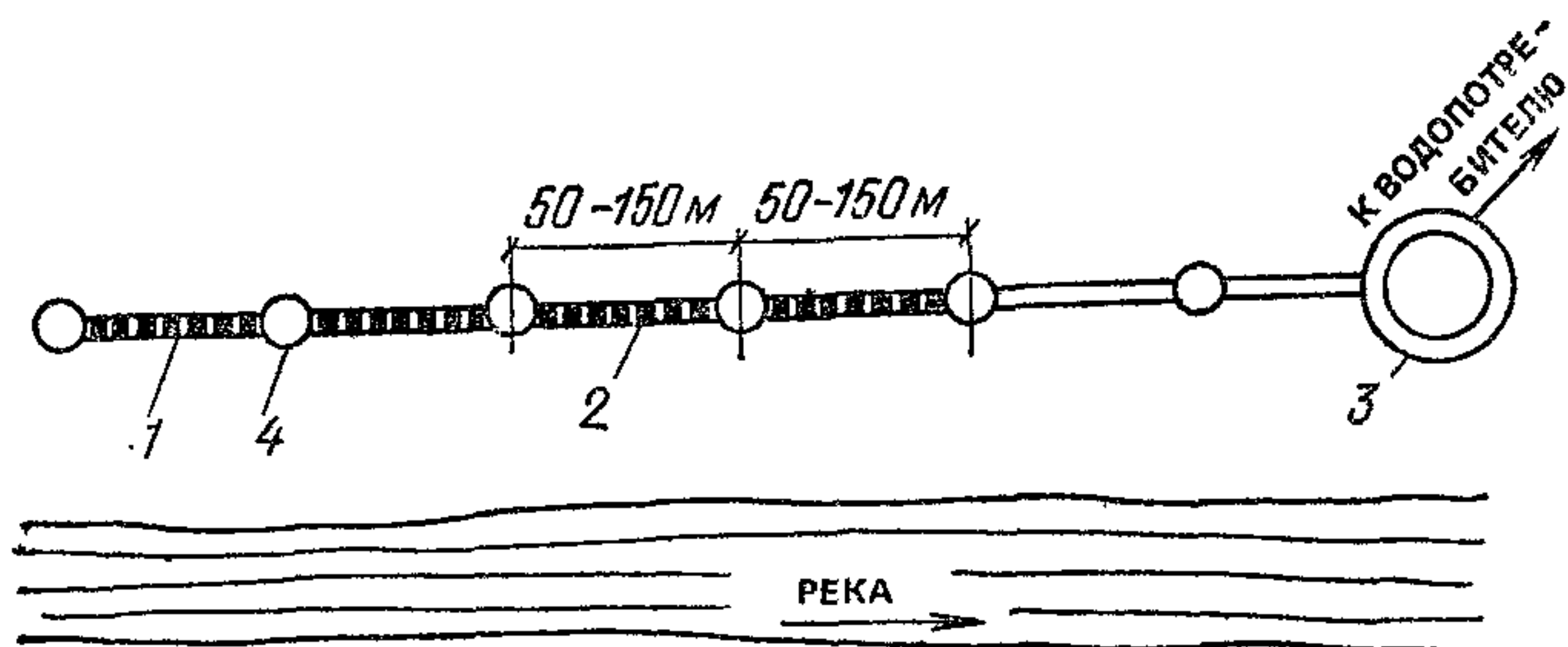
Рис. 14. Схема горизонтального водозабора
