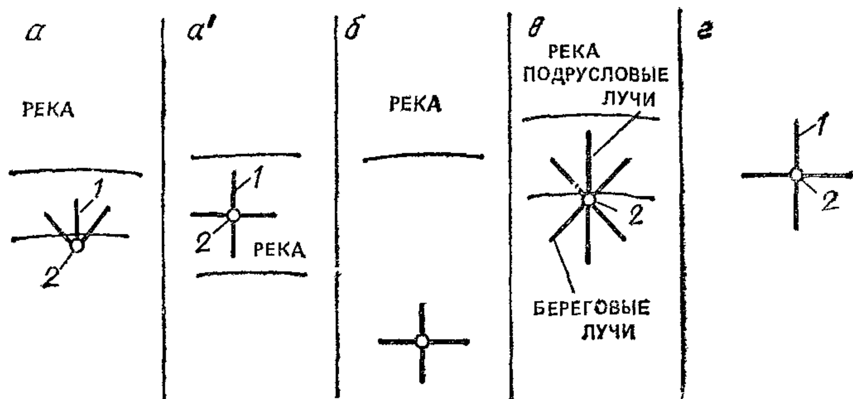
Рис. 35. Схемы лучевых водозаборов в плане
