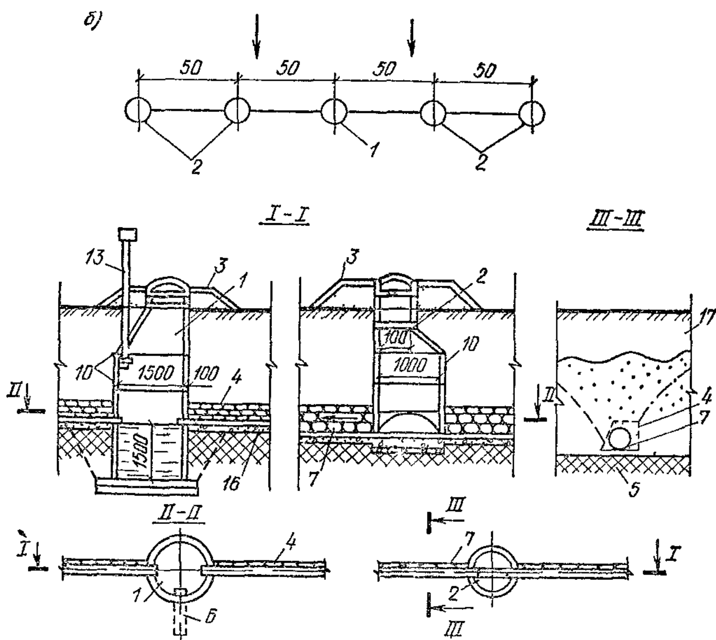
Рис. 17. Горизонтальные водозаборы трубчатого типа
