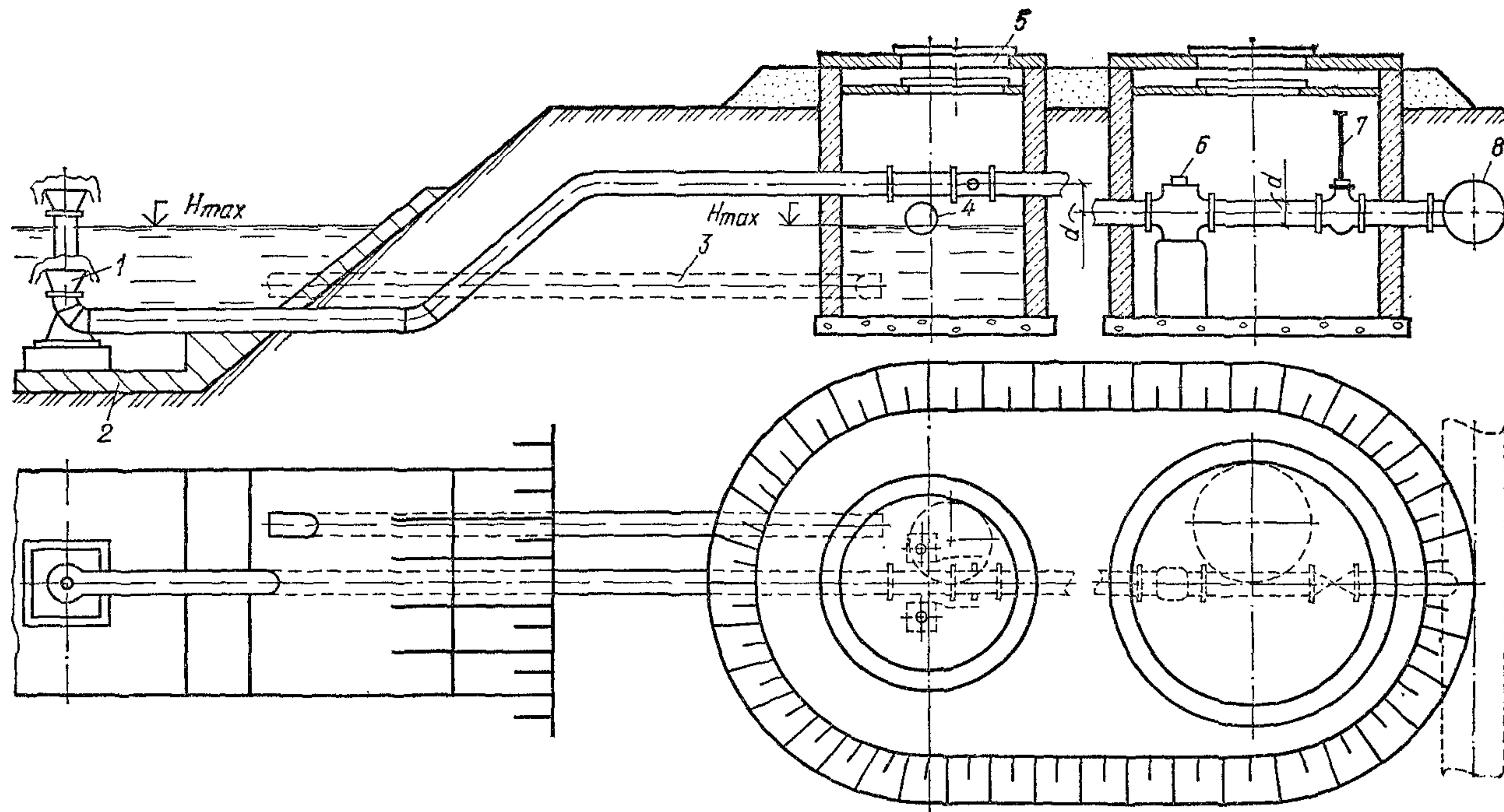
Рис. 50. Схема входного узла (закрытая распределительная сеть) 1 — водовыпускное устройство; 2 — водослив, 3 — труба, связывающая «мокрый колодец с бассейном»; 4 — ограничитель уровня дроссельно поплавкового типа; 5 — люки, 6 — водомер; 7 — задвижка; 8 — распределительный трубопровод
