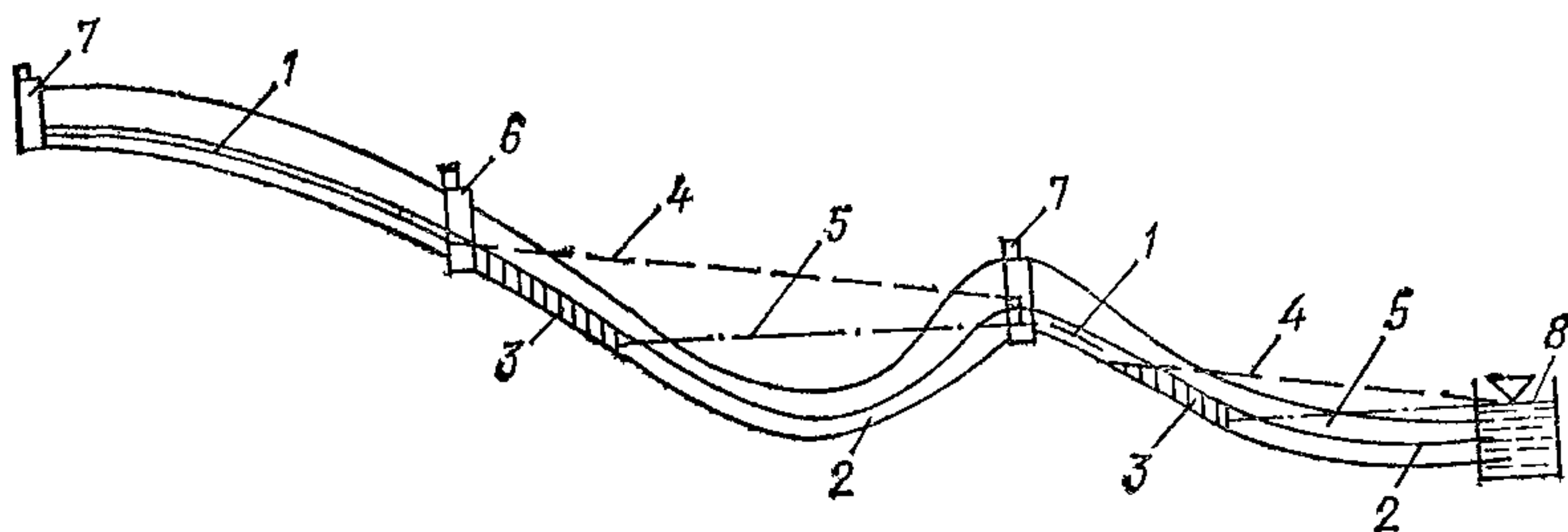
Рис. 93. Схема самотечно-напорного водовода
