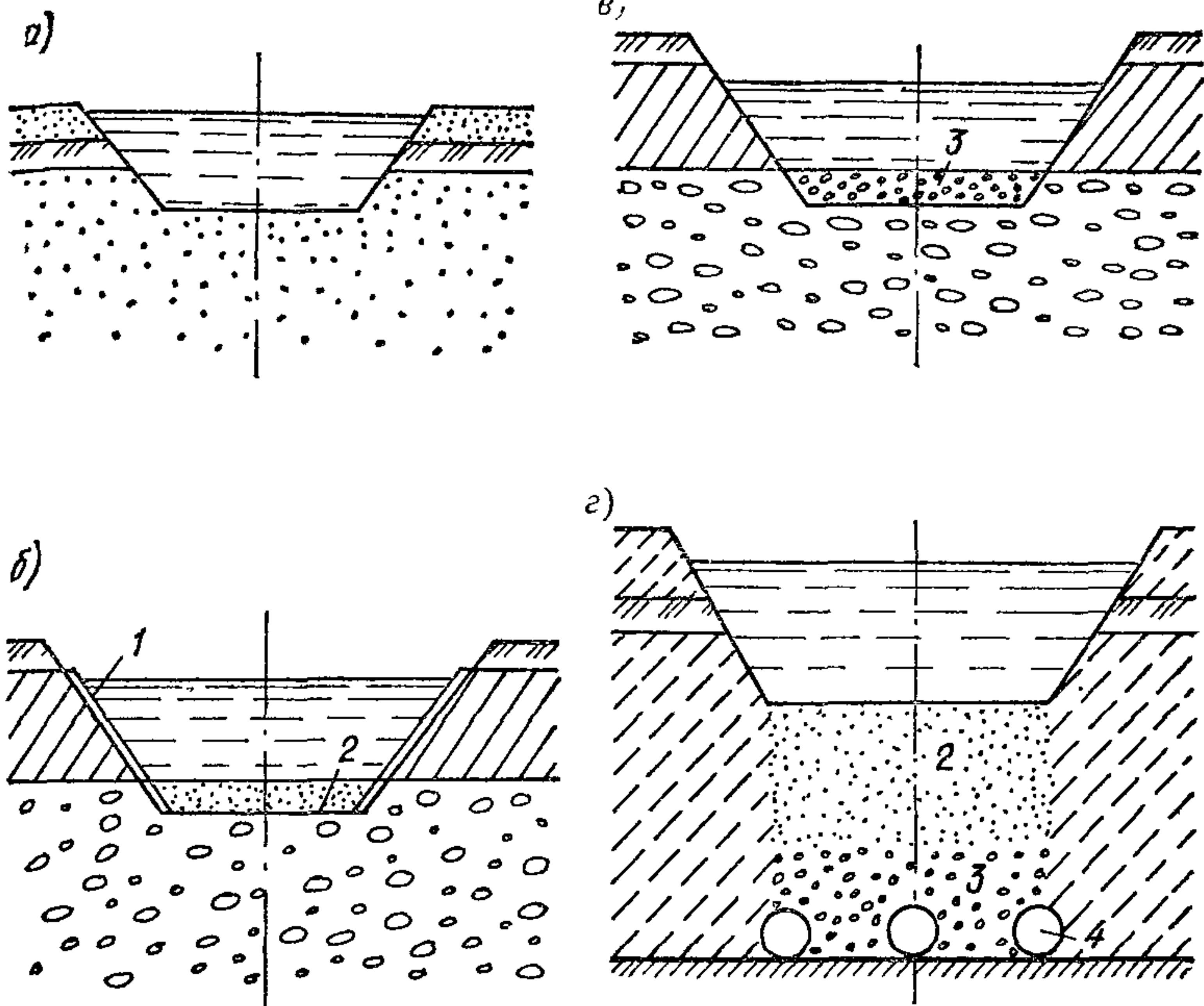
Рис. 48. Схемы инфильтрационных бассейнов
