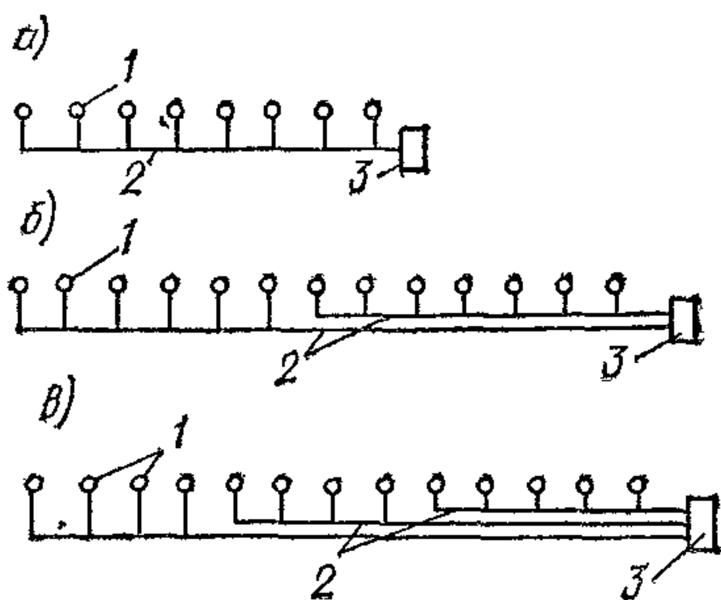
Рис. 88. Схемы линейных (тупиковых) сборных водоводов при линейном расположении водозаборных сооружений и концевом расположении сборного узла
