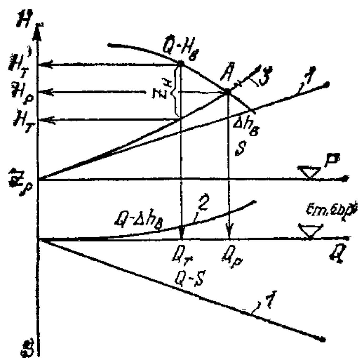
Рис. 100 Графоаналитический метод расчета системы «скважина — насос — водовод — резервуар»
