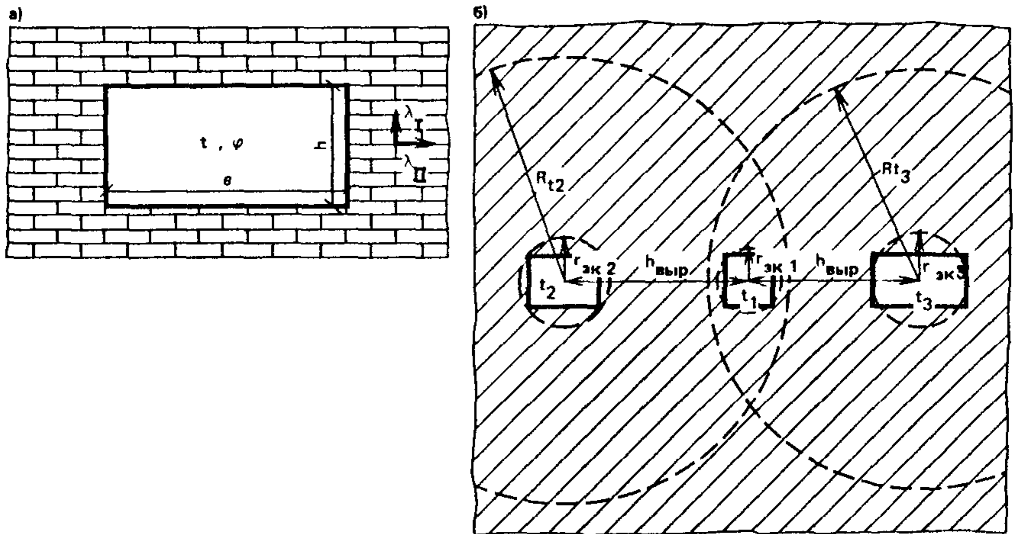
Рис. 6. Расчетные схемы к определению k_{\tau}
