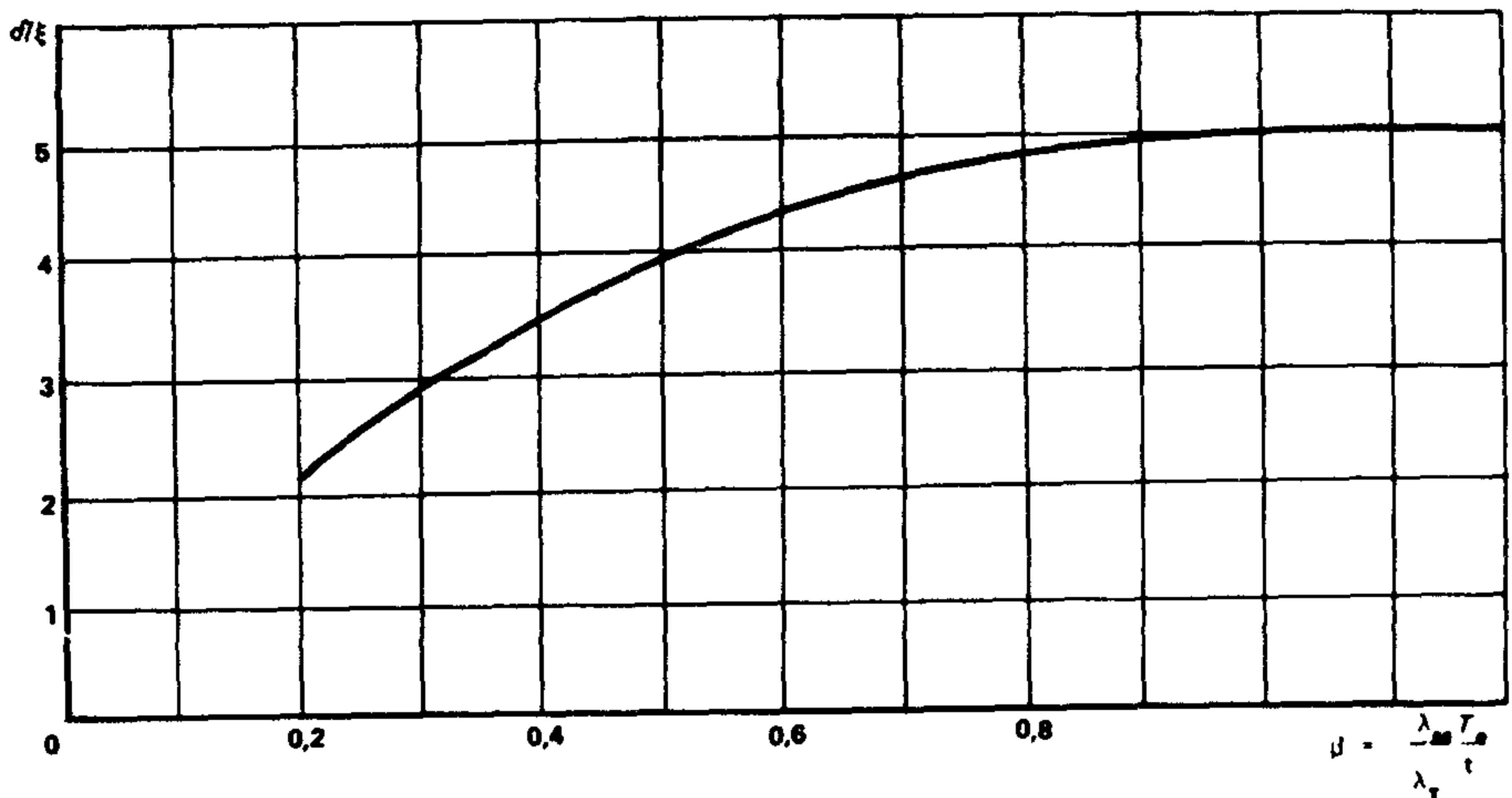
Рис. 11. График для определения отношения \delta/\xi в зависимости от параметра (-\lambda_{пм}/\lambda_{пт} T_e/t_{ср})
