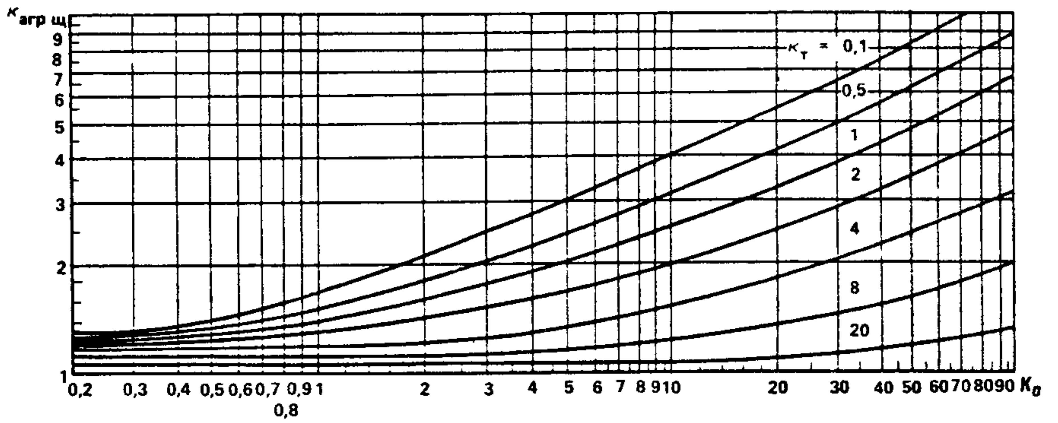
Рис. 9. Номограмма для определения коэффициента k_{agr щ}
