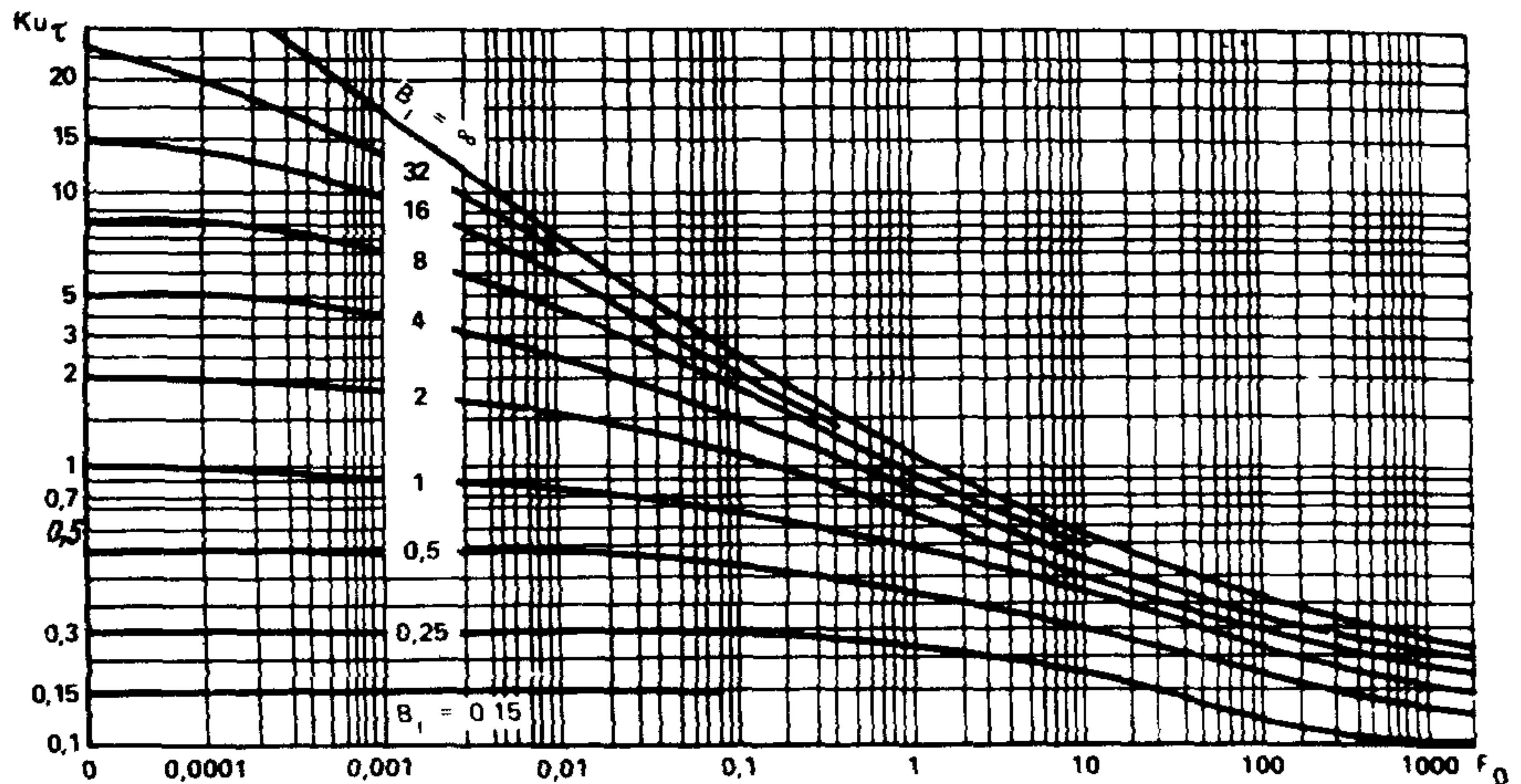
Рис. 4. Номограмма для определения коэффициента нестационарного теплообмена
