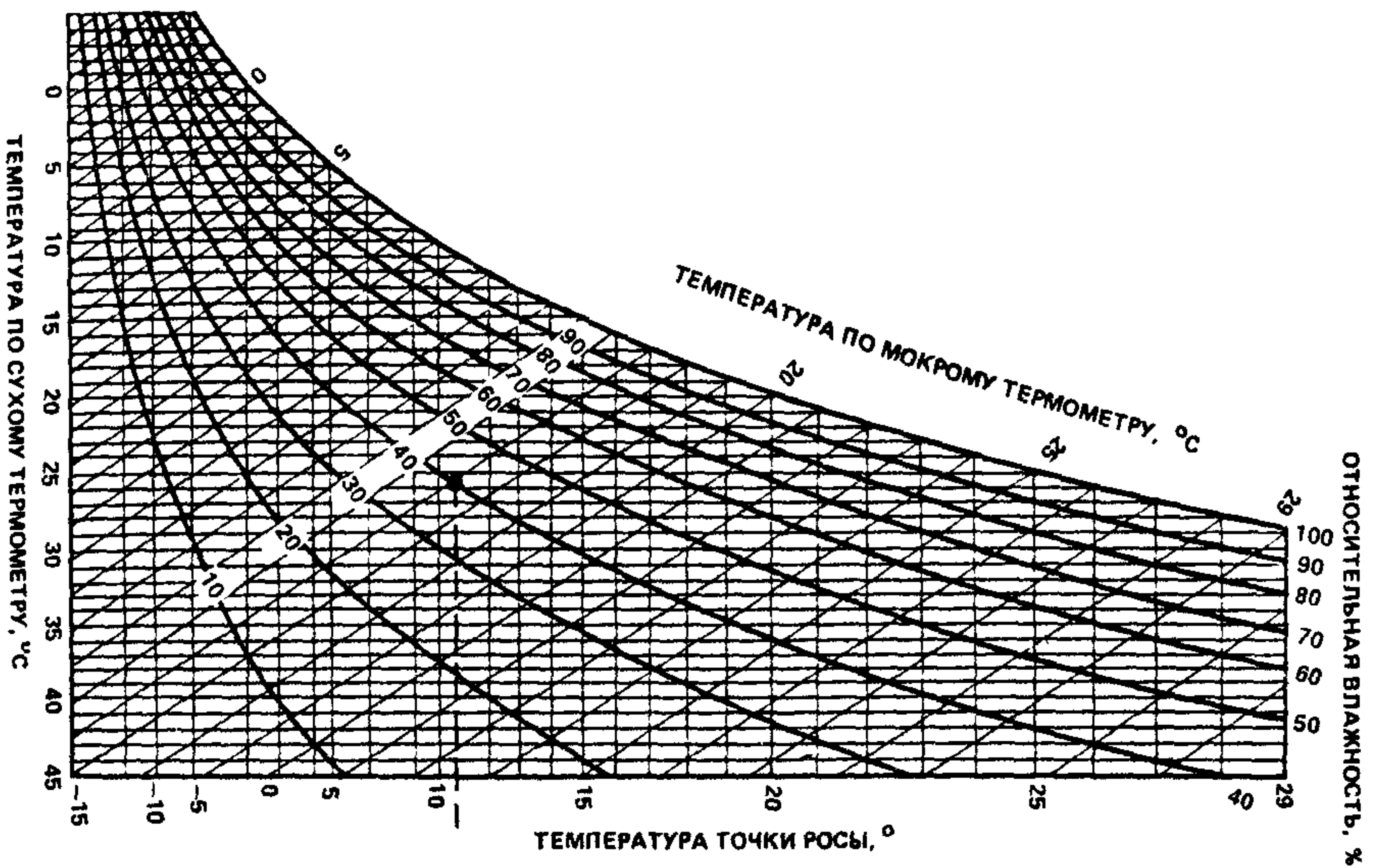
Психрометрическая диаграмма
