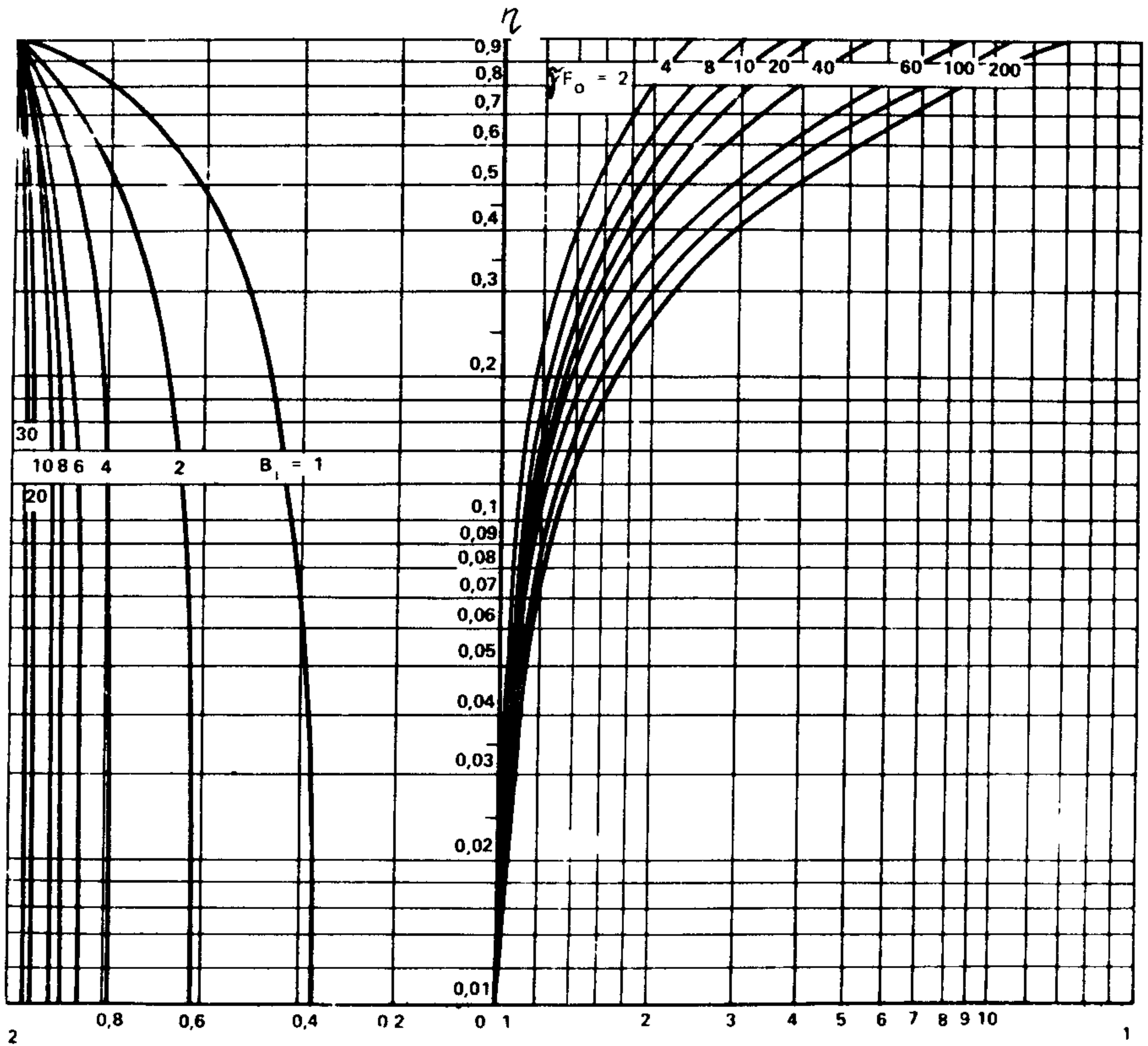
Рис. 10. Номограмма для вычисления параметров \zeta_1 и \zeta_2
