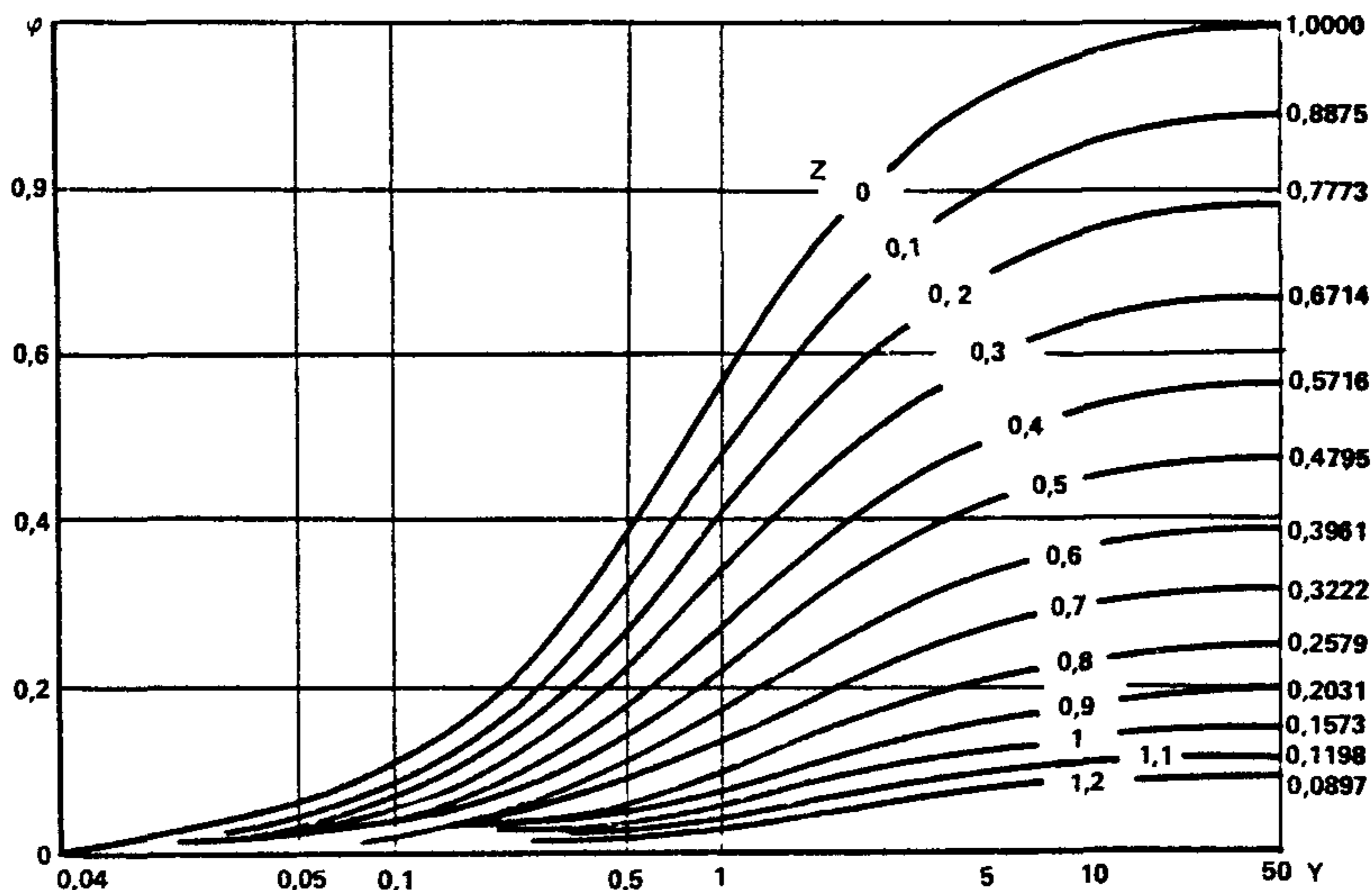
Рис. 12. График для определения значения функции \varphi(Z, Y) .
