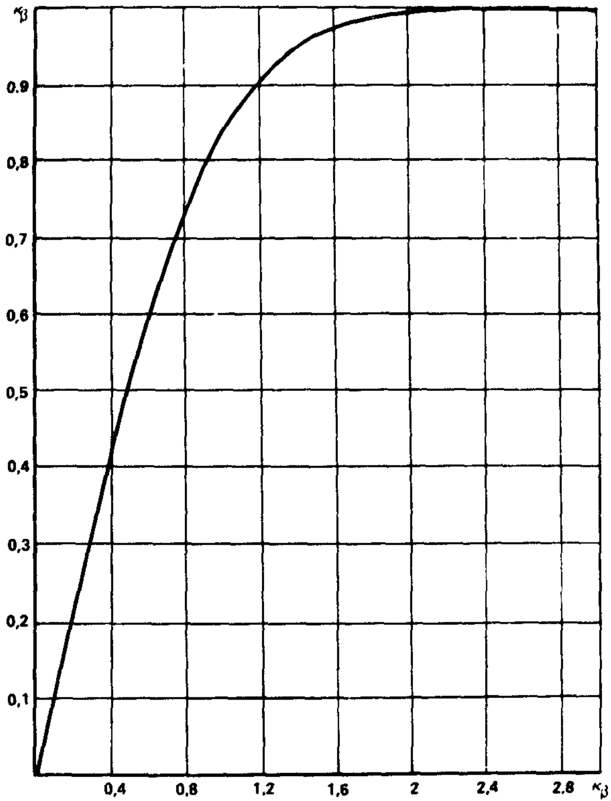
Рис. 8. График зависимости интеграла вероятности, erf, от параметра k_\beta
