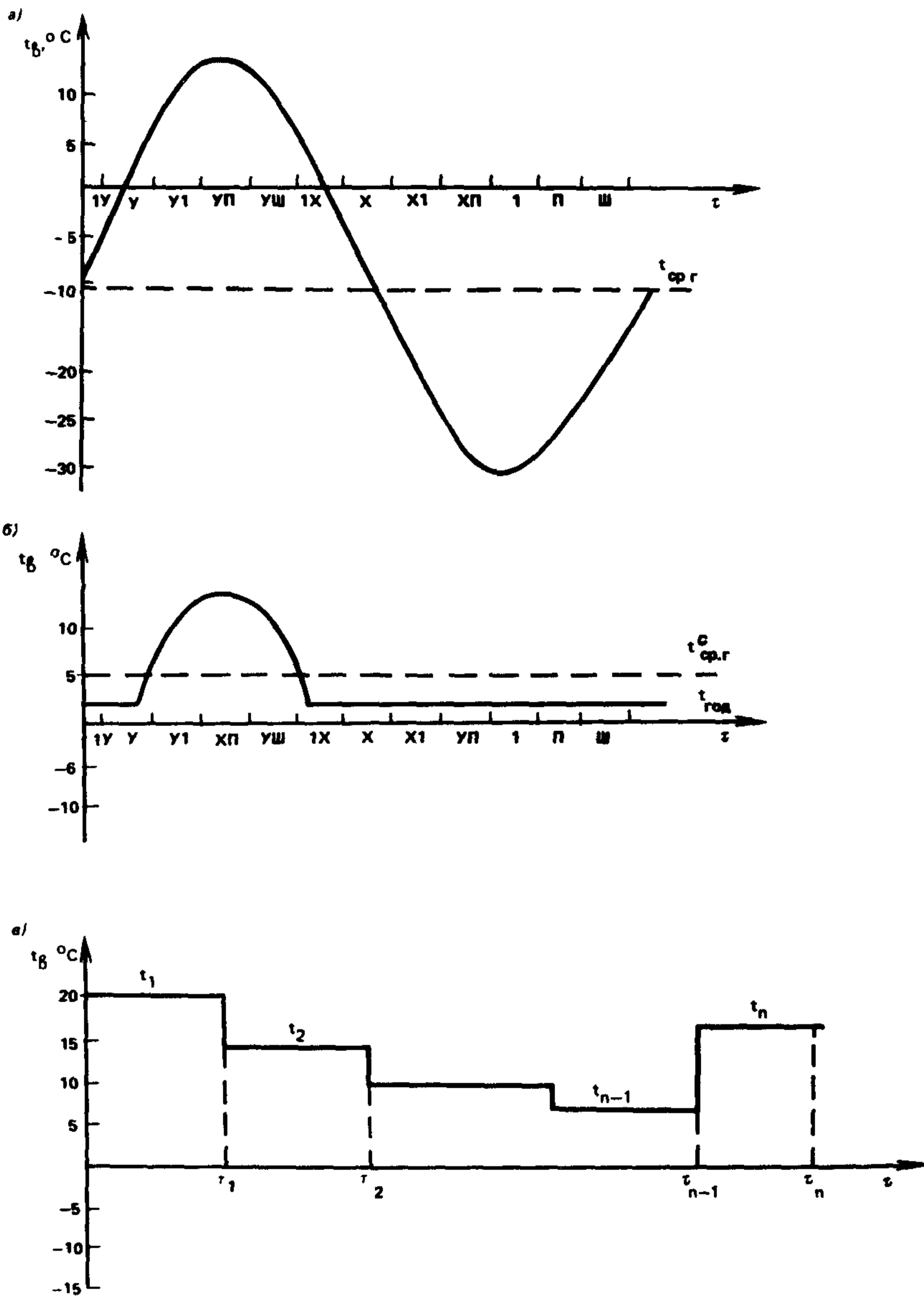
Рис 1. Характер изменения температуры воздуха, поступающего в ПС а — гармонический закон (изменение температуры атмосферного воздуха); б — изменение температуры воздуха при его подогреве до положительной температуры в зимнее время, в — ступенчатый закон изменения температуры воздуха
