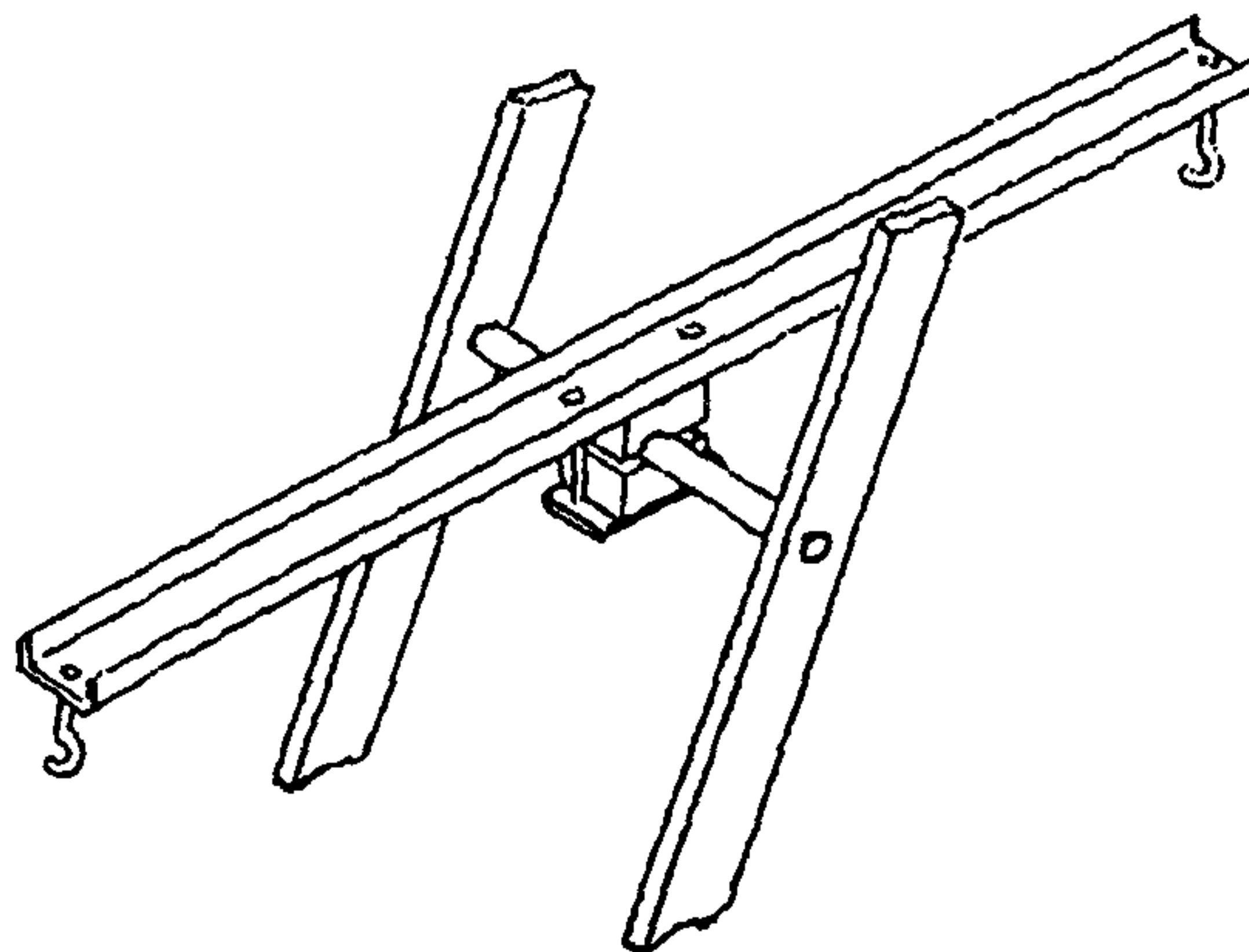
Рис. 7. Приспособление для испытания ступеньки лестницы на кручение
