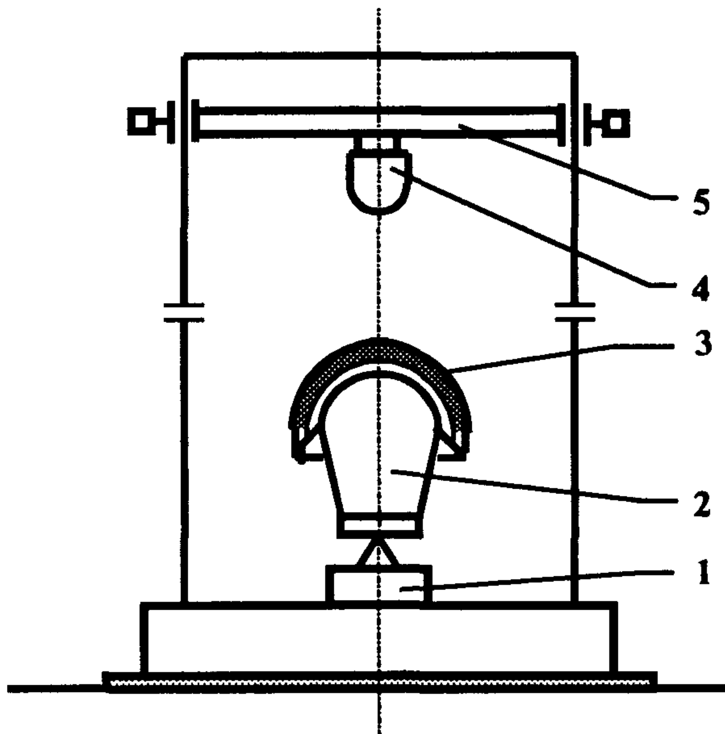
Рис. 1. Принципиальная схема стенда ударного:
