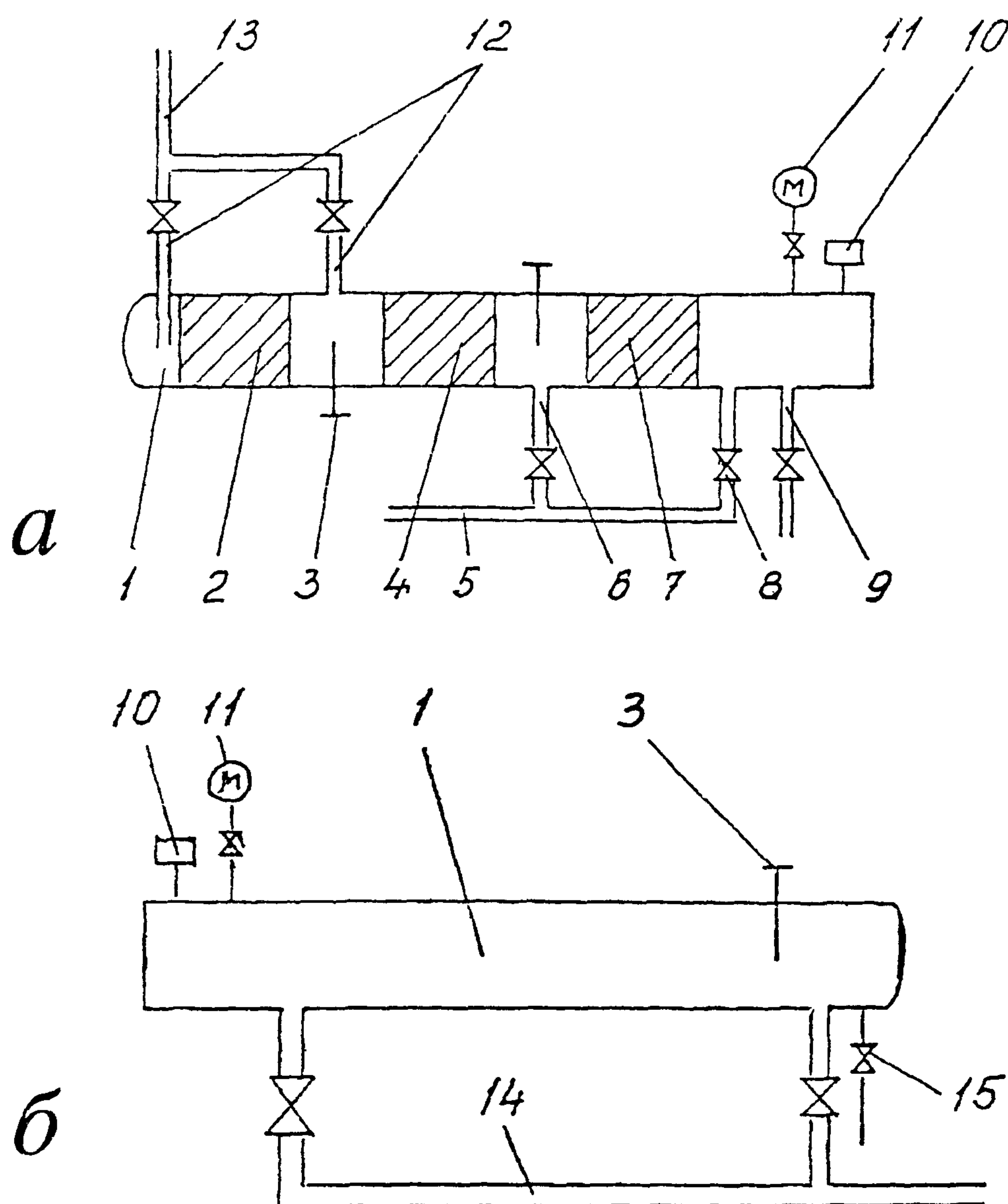
Рис. 8 Принципиальная схема камеры пуска и камеры приема поршней при промывке и удалении воды после испытания:
