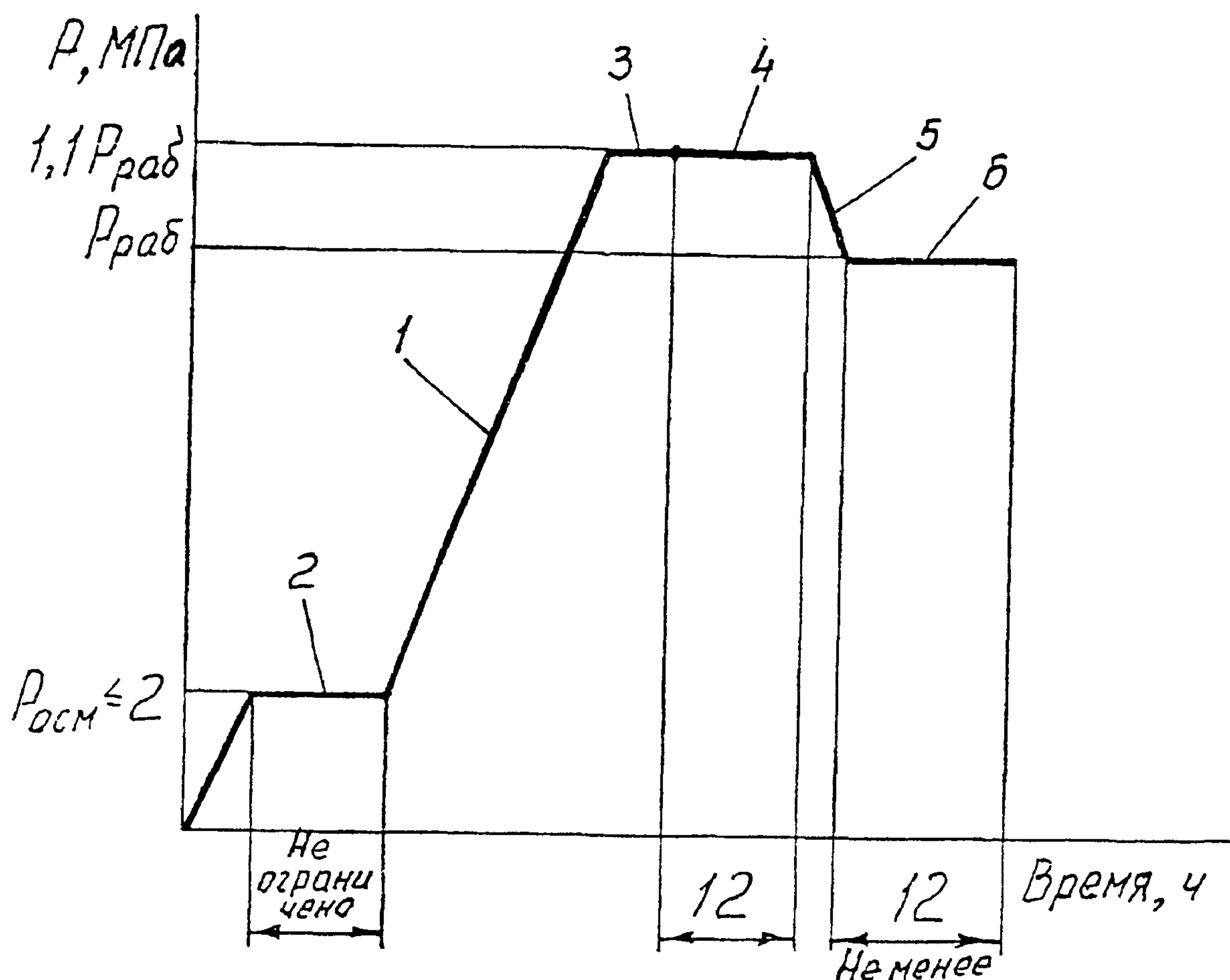
Рис. 7 График изменения давления в газопроводе при пневматическом испытании:
