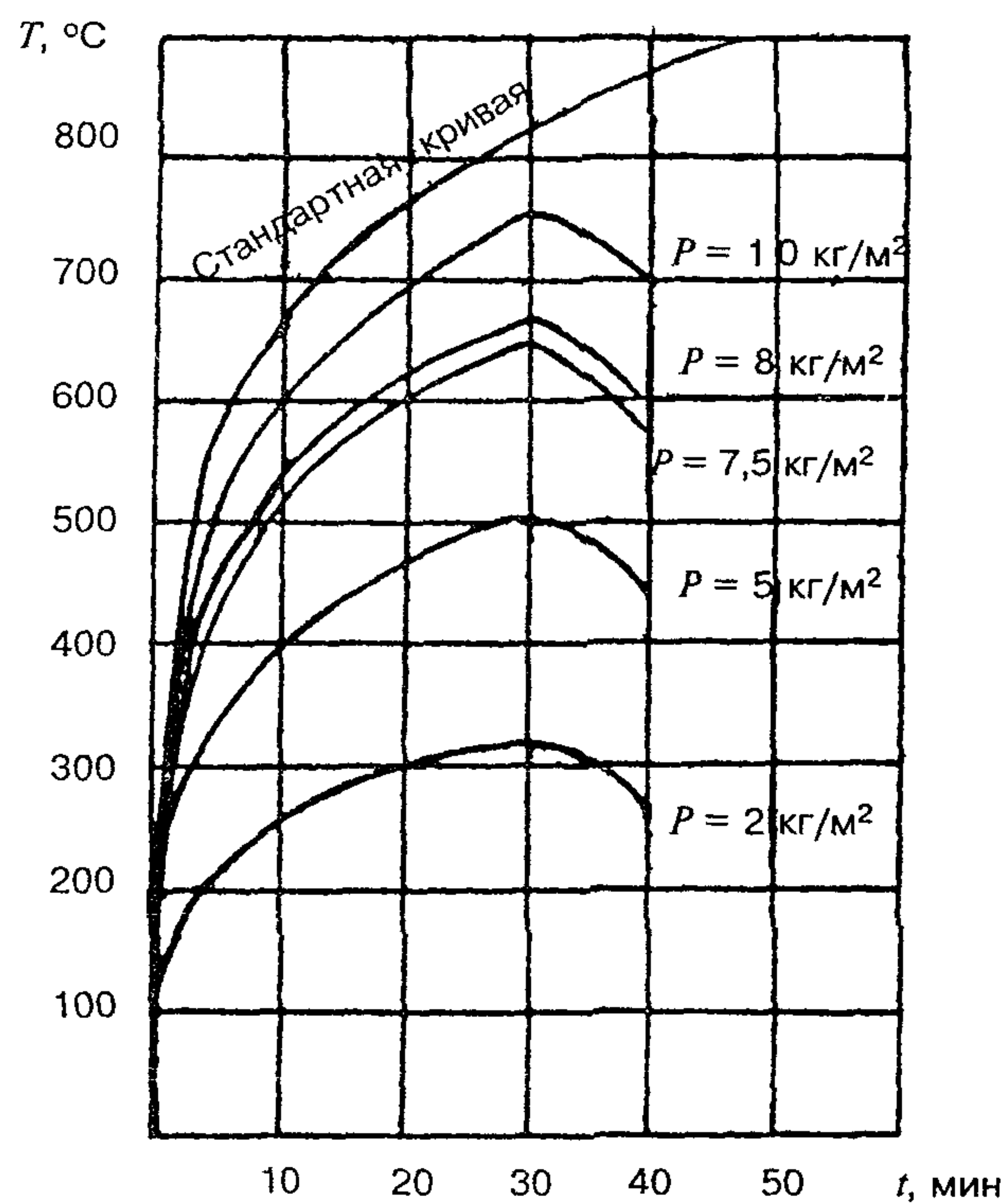
Рис. 4. Температурные режимы ПРН
