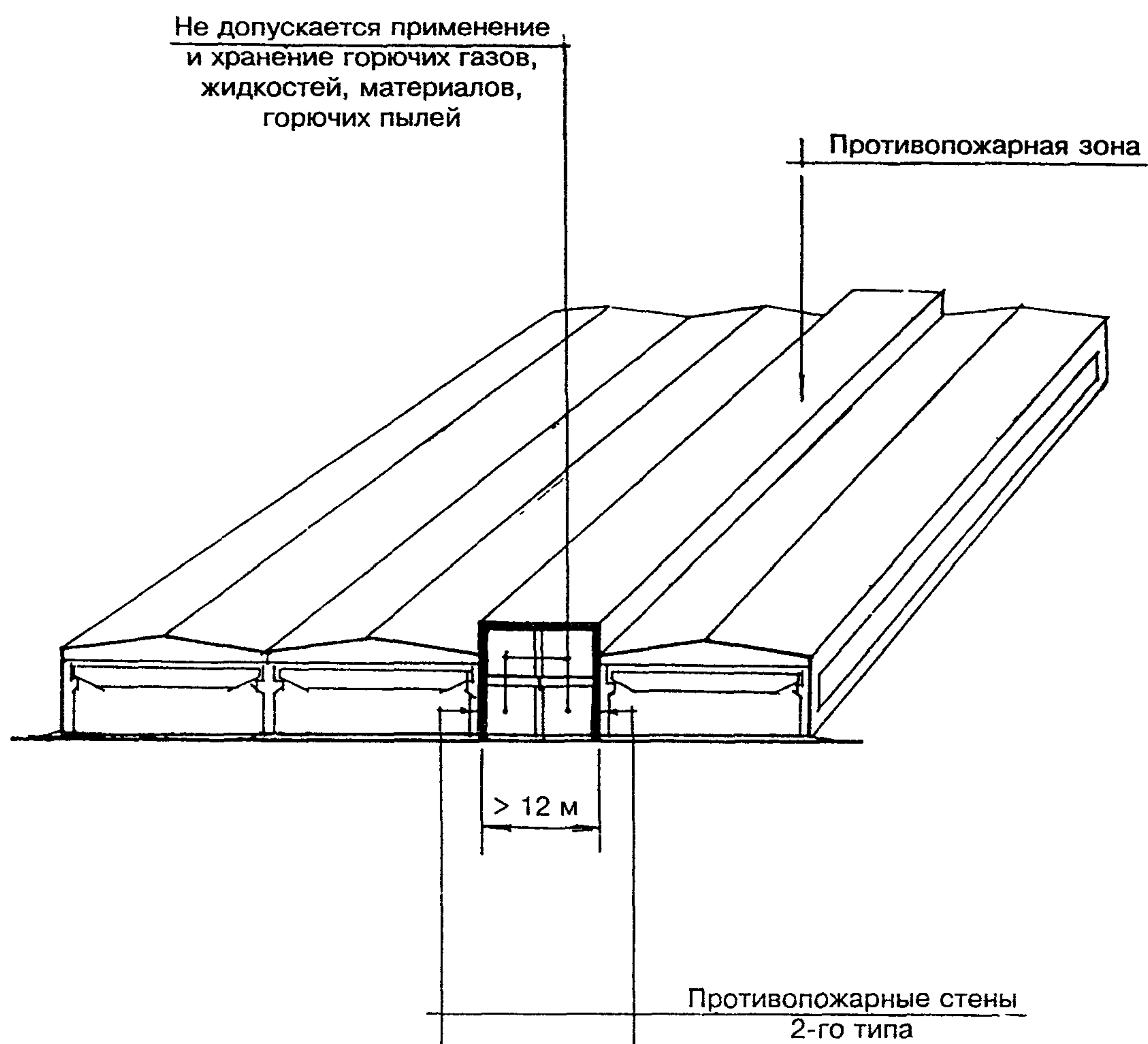
Рис. 9. Противопожарная зона
