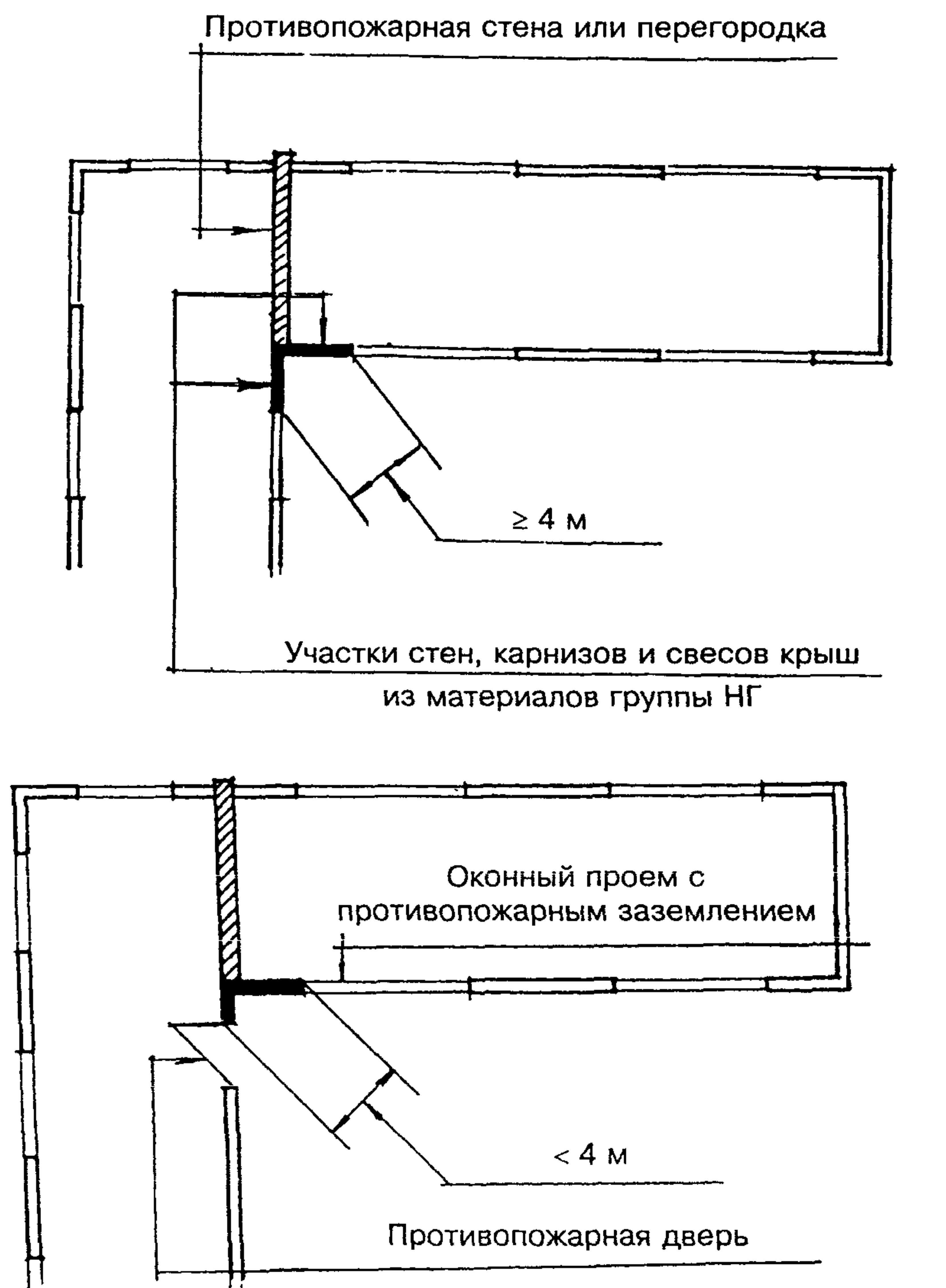
Рис. 6. Участок стены в местах примыкания частей зданий под углом, разделенных противопожарными стенами
