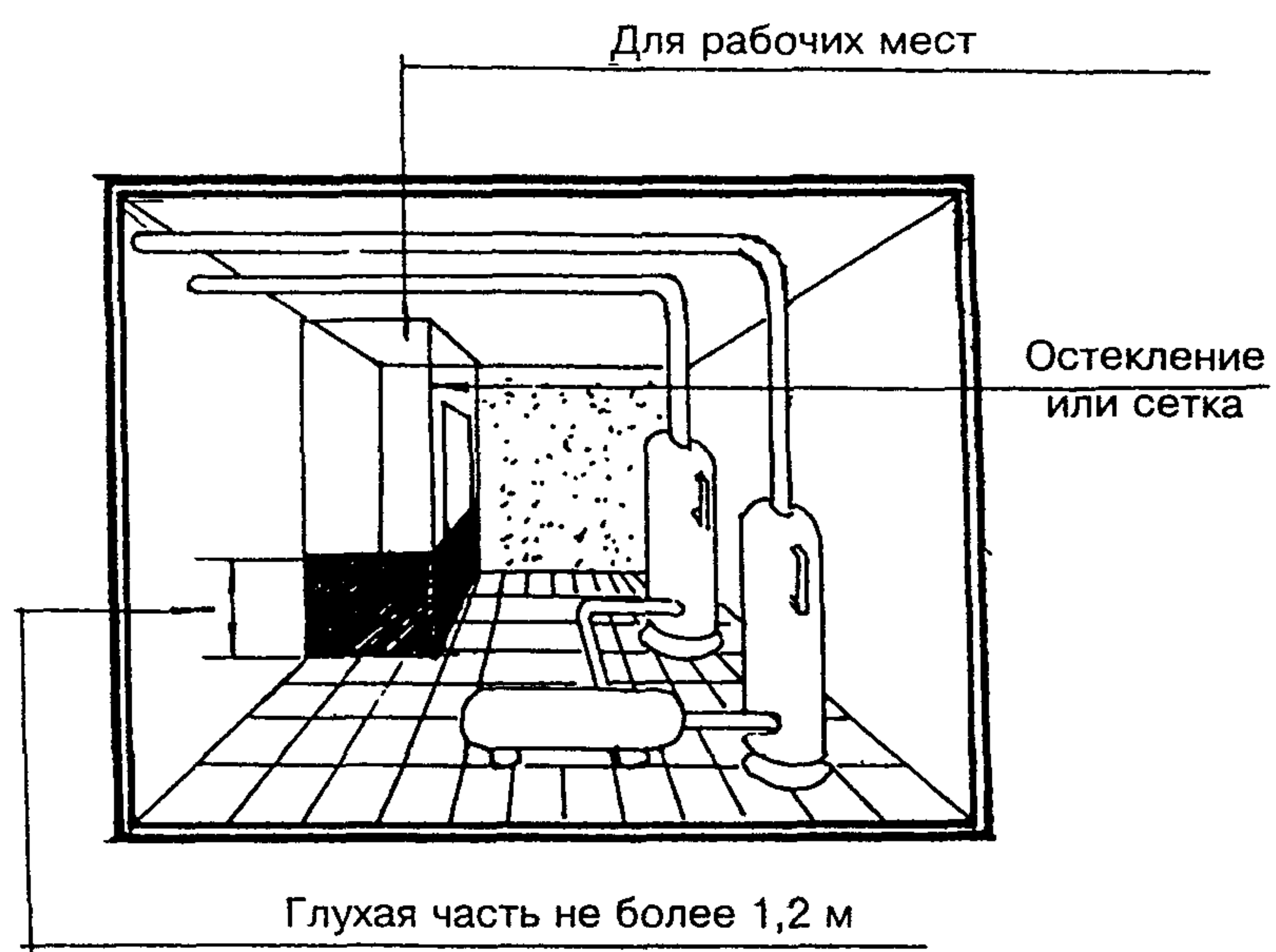
Рис. 7. Выгораживание рабочих мест
