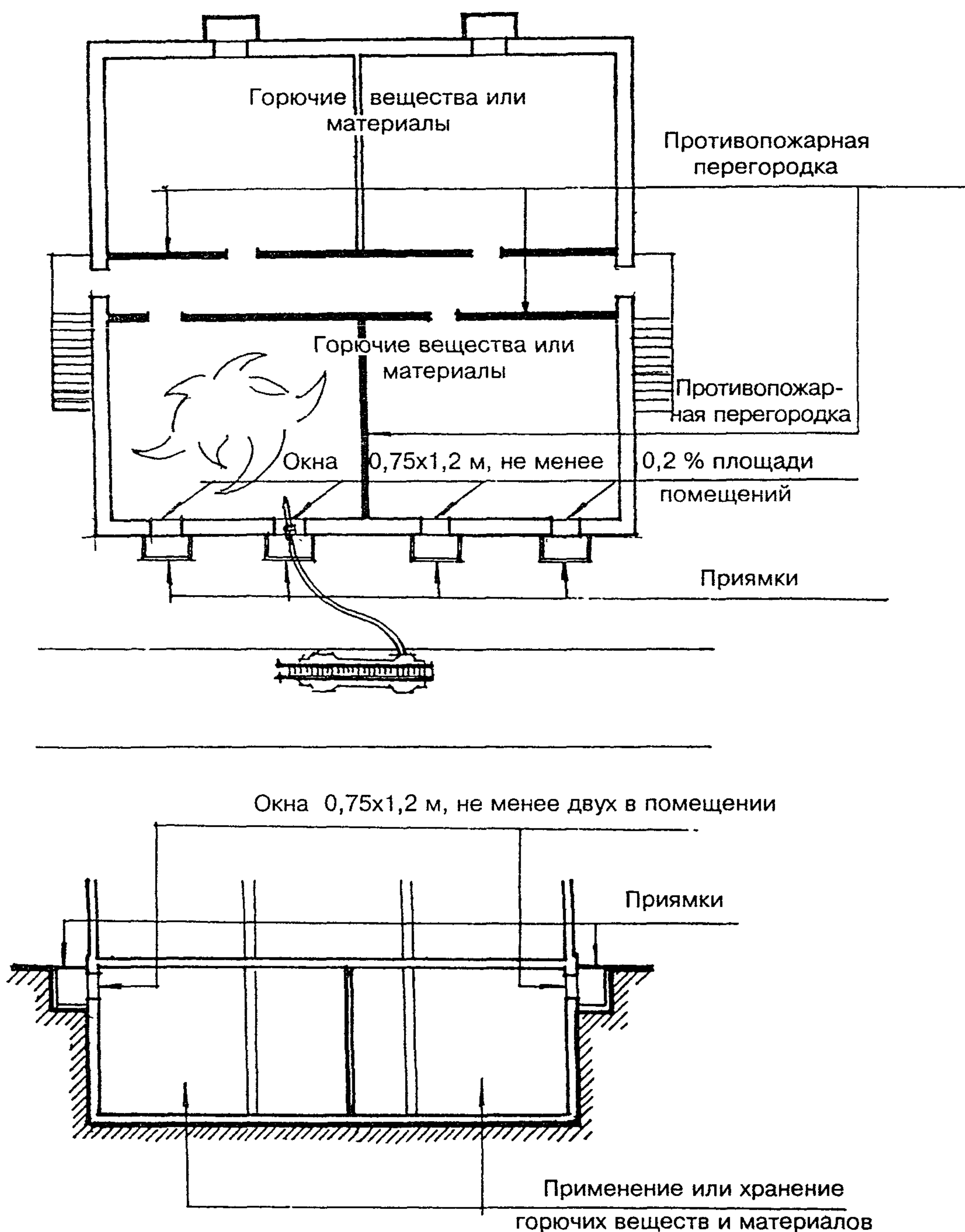
Рис. 2. Устройство окон с приямками в подвальных этажах
