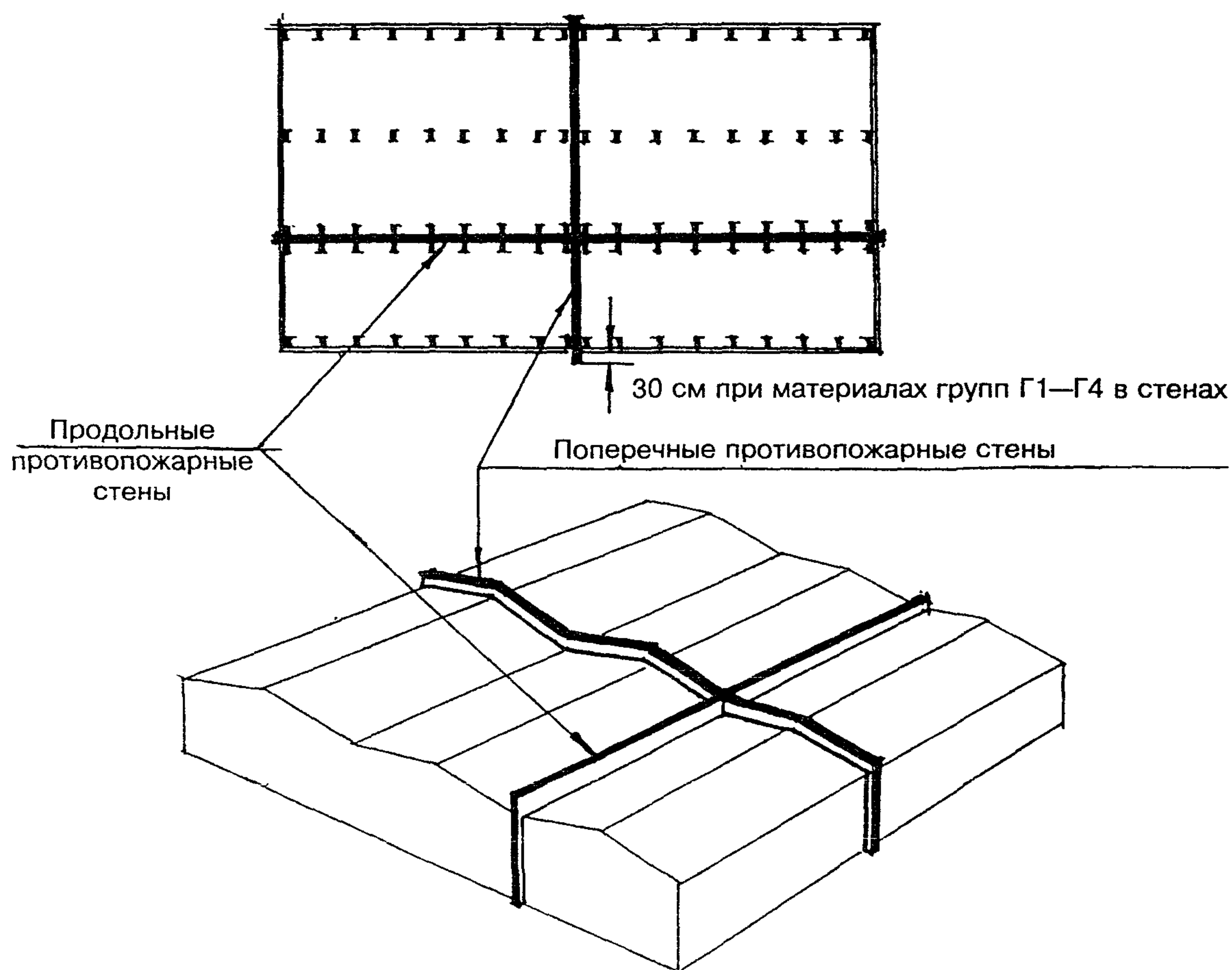
Рис. 4. Разделение зданий на пожарные отсеки противопожарными стенами
