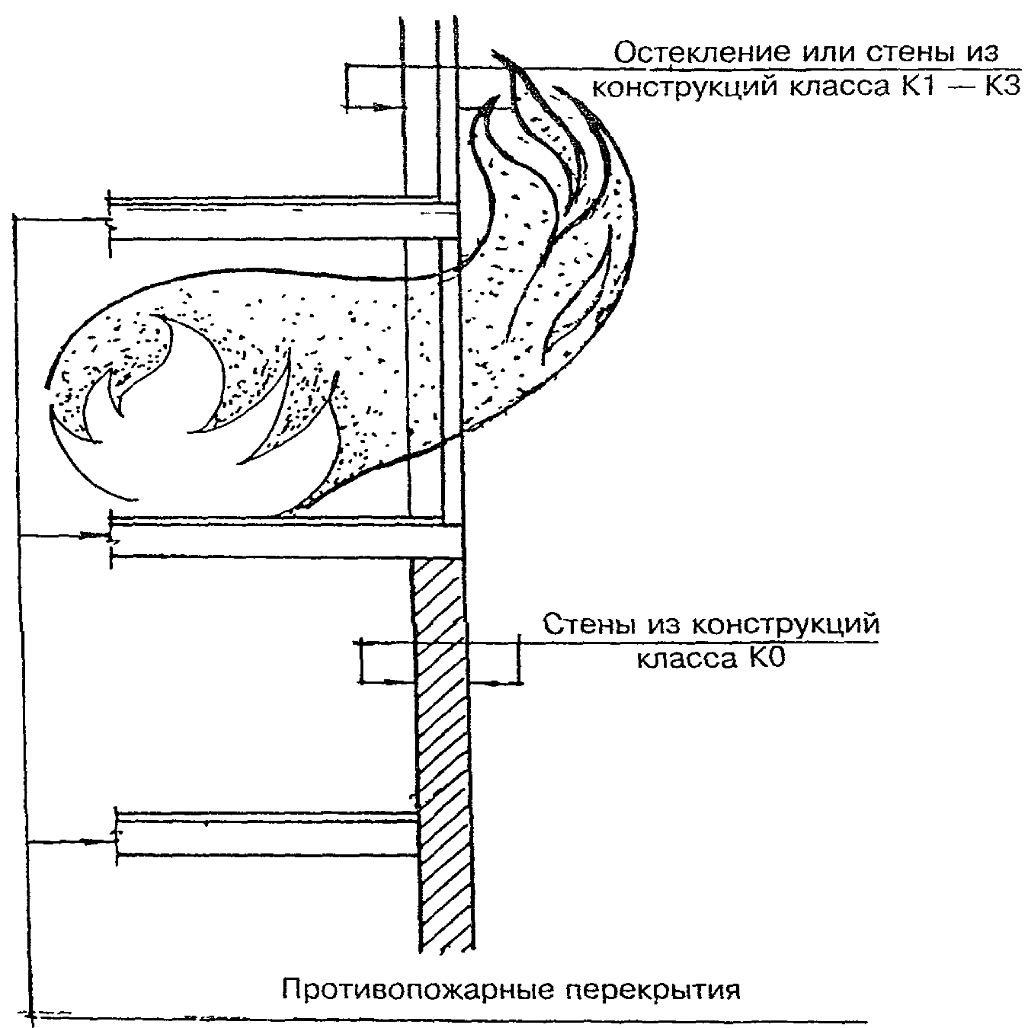
Рис. 8. Примыкание противопожарного перекрытия к наружной стене
