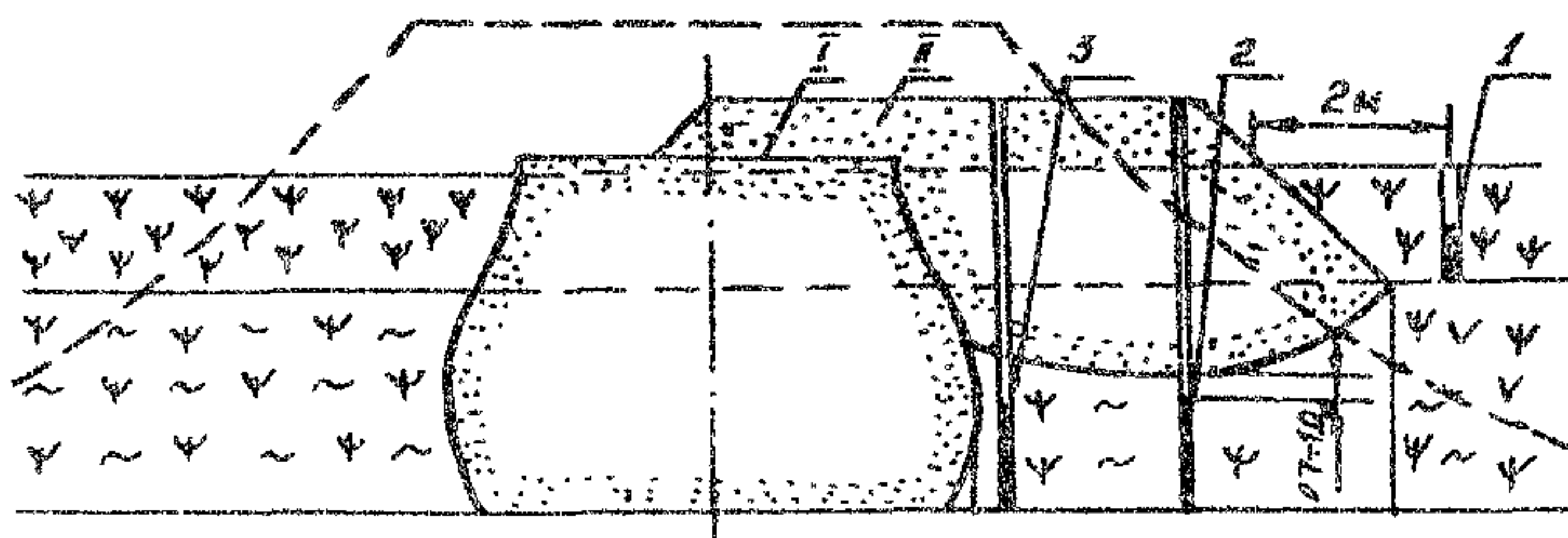
Рис. 28. Схема расположения скважинных зарядов при посадке на дно болота откосного участка широкой насыпи: I—ядро насыпи; II—откосный участок; 1—вспомогательный заряд; 2, 3—основные заряды
