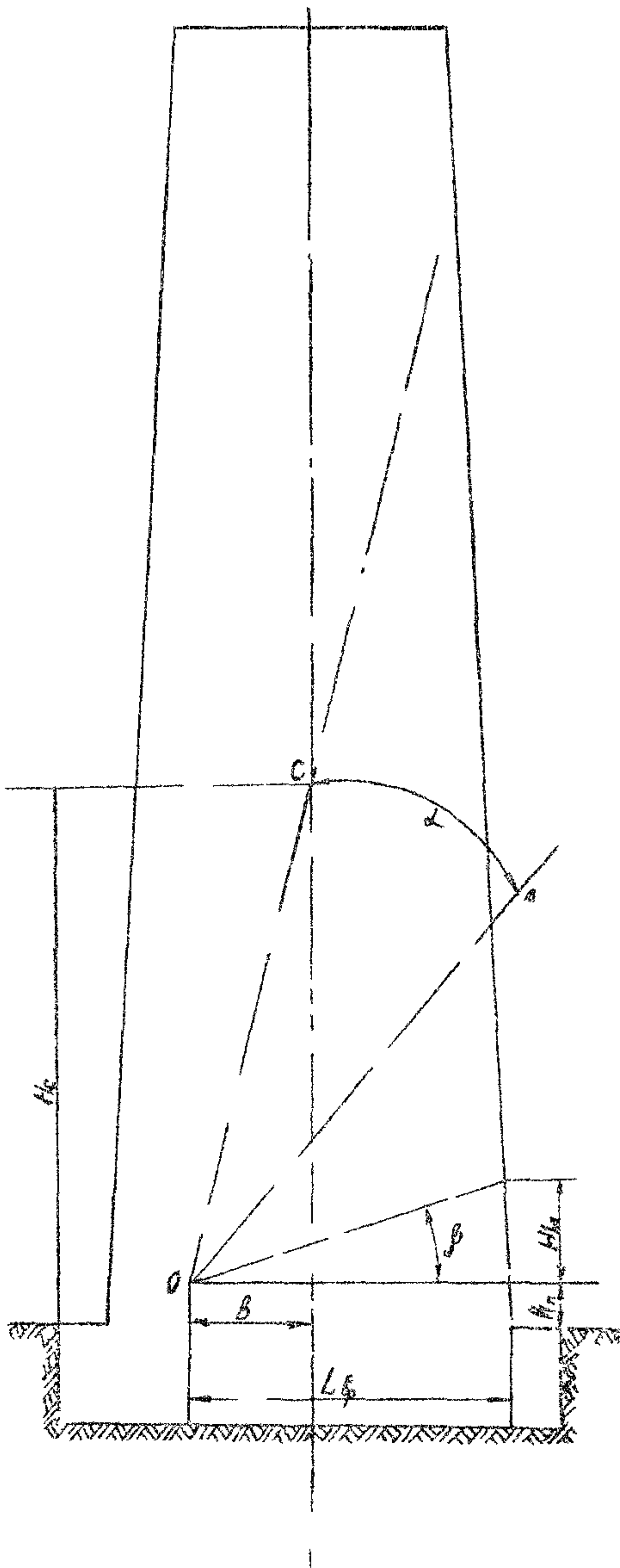
Рис 31 Схема для расчета опрокидывания грубы в заданном направлении
