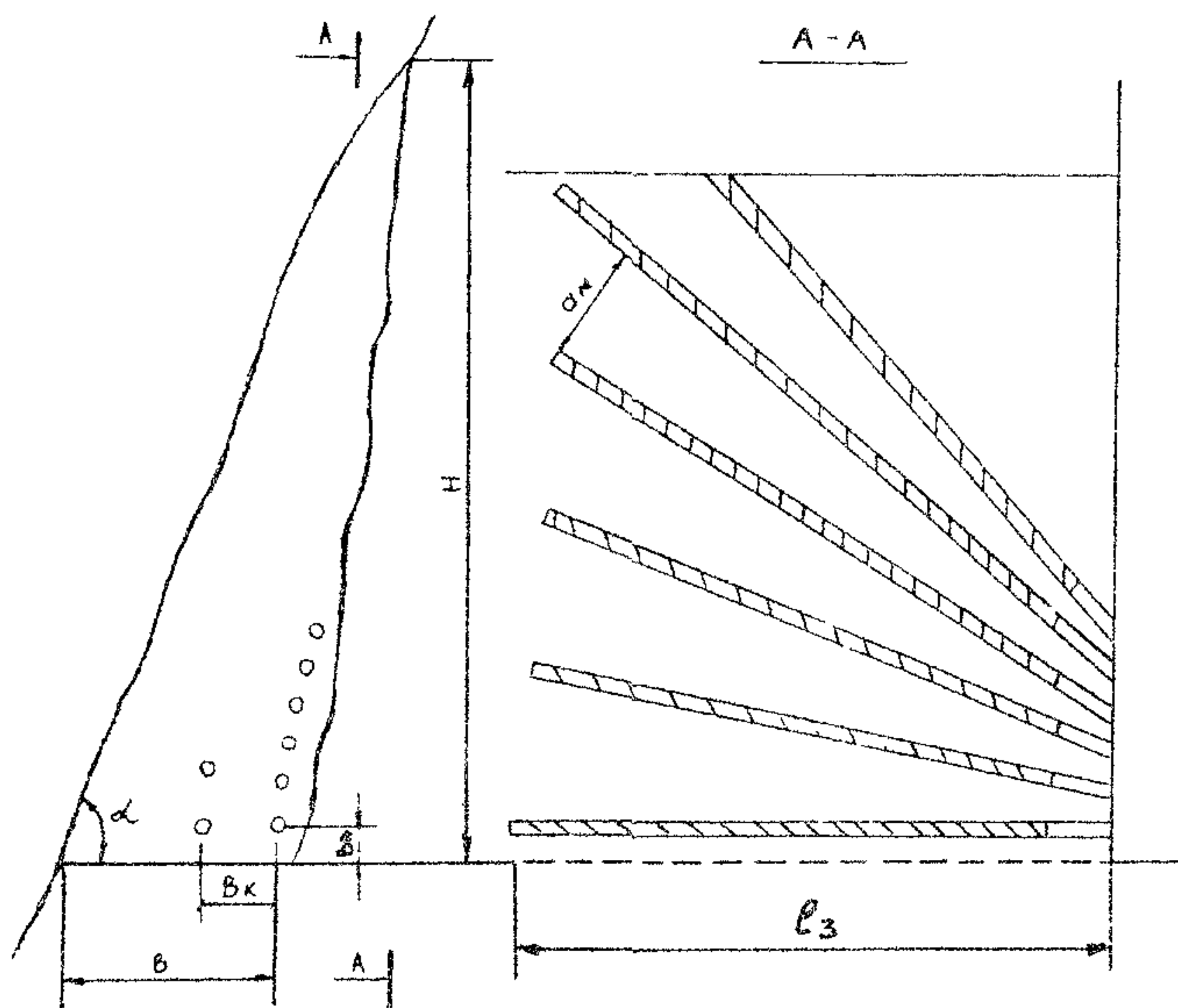
Рис. 20. Схема взрыва на обрушение веерными скважинами
