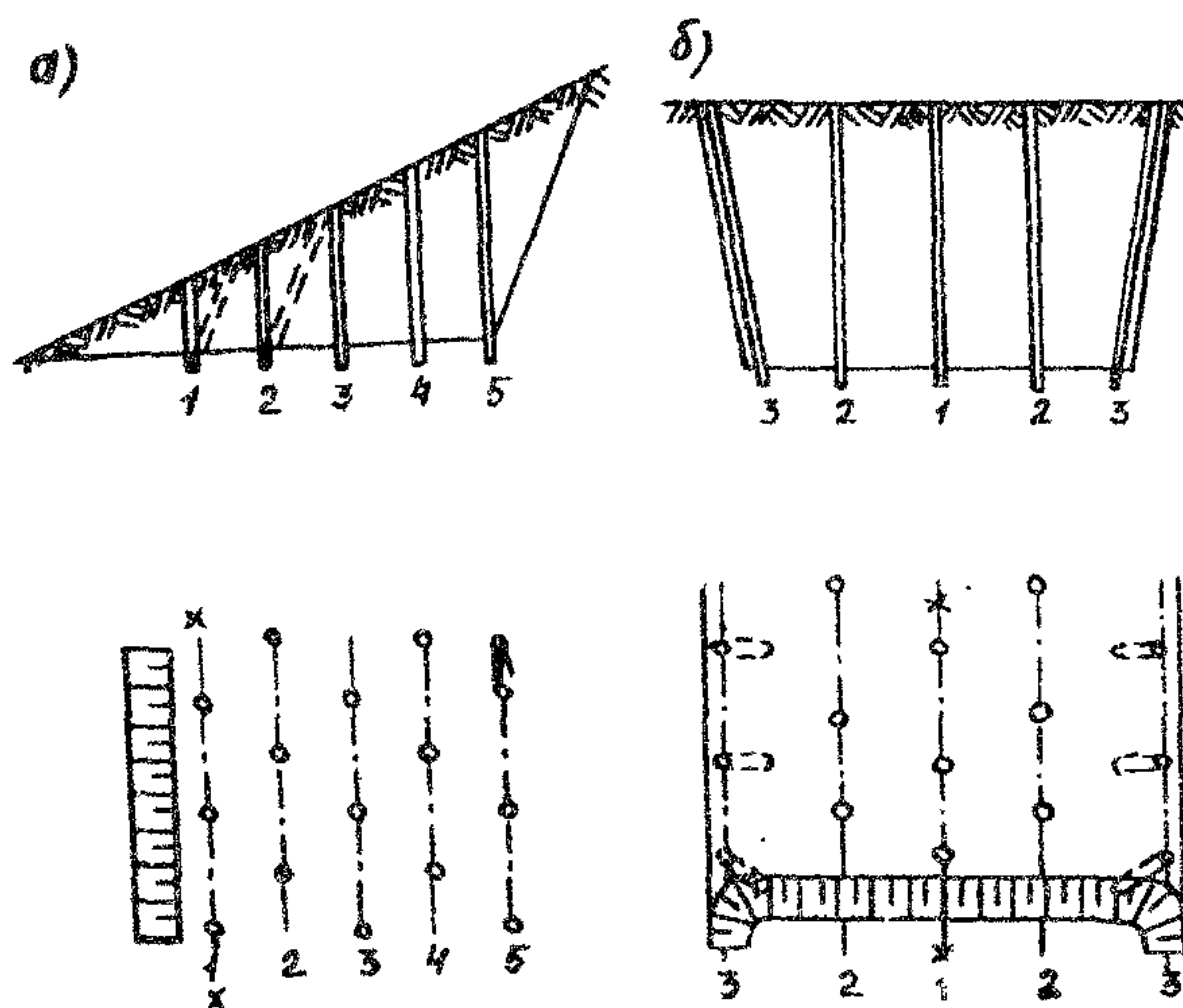
Рис. 5. Продольно-порядные схемы КЗВ: а—для выемки на косогоре; б—для выемки на равнинном участке; 1, 2, 3, 4, 5—очередность взрывания рядов скважин
