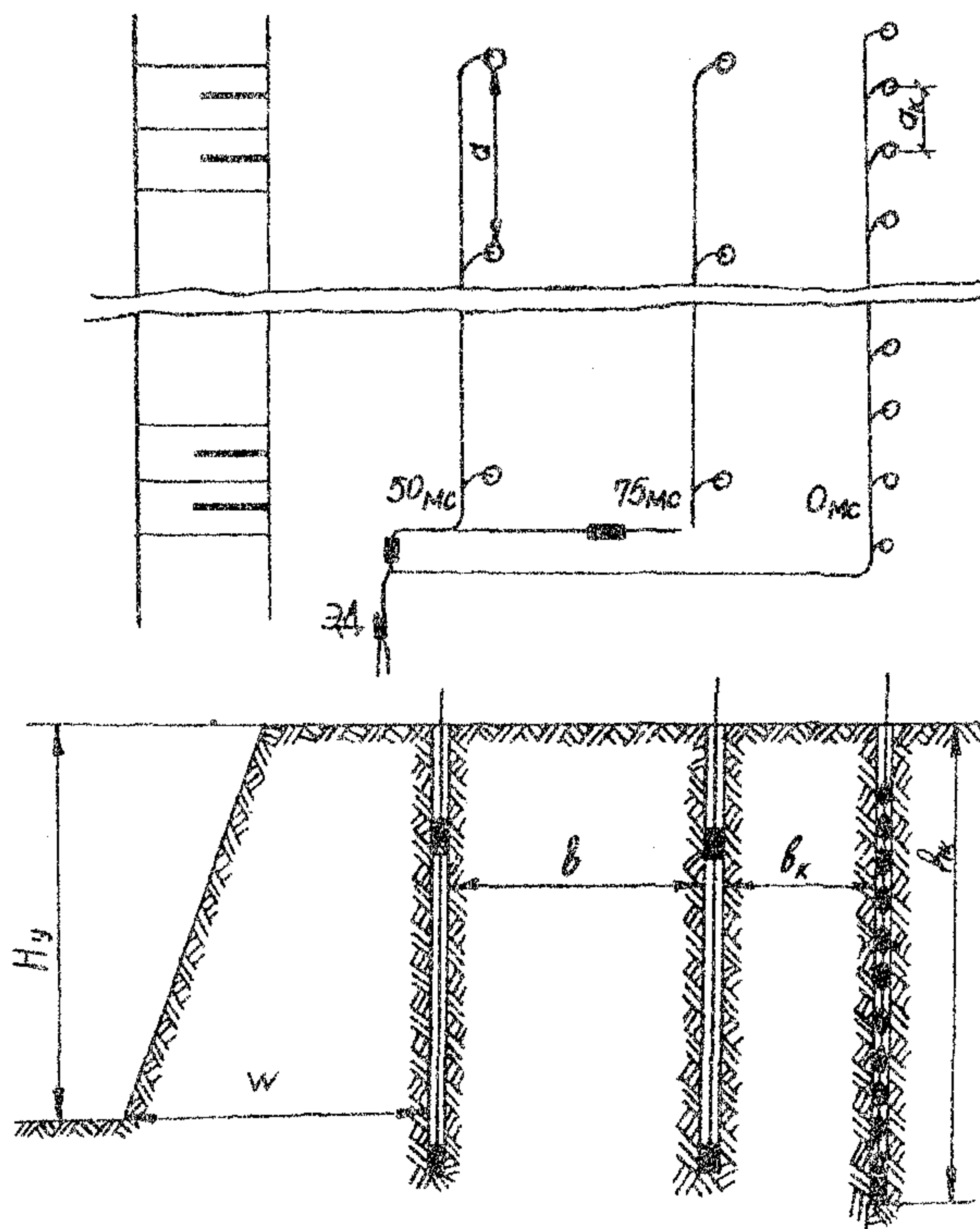
Рис. 32. Схема контурного взрывания методом предварительного щелеобразования. 0 мс, 50 мс, 75 мс—интервалы замедления
