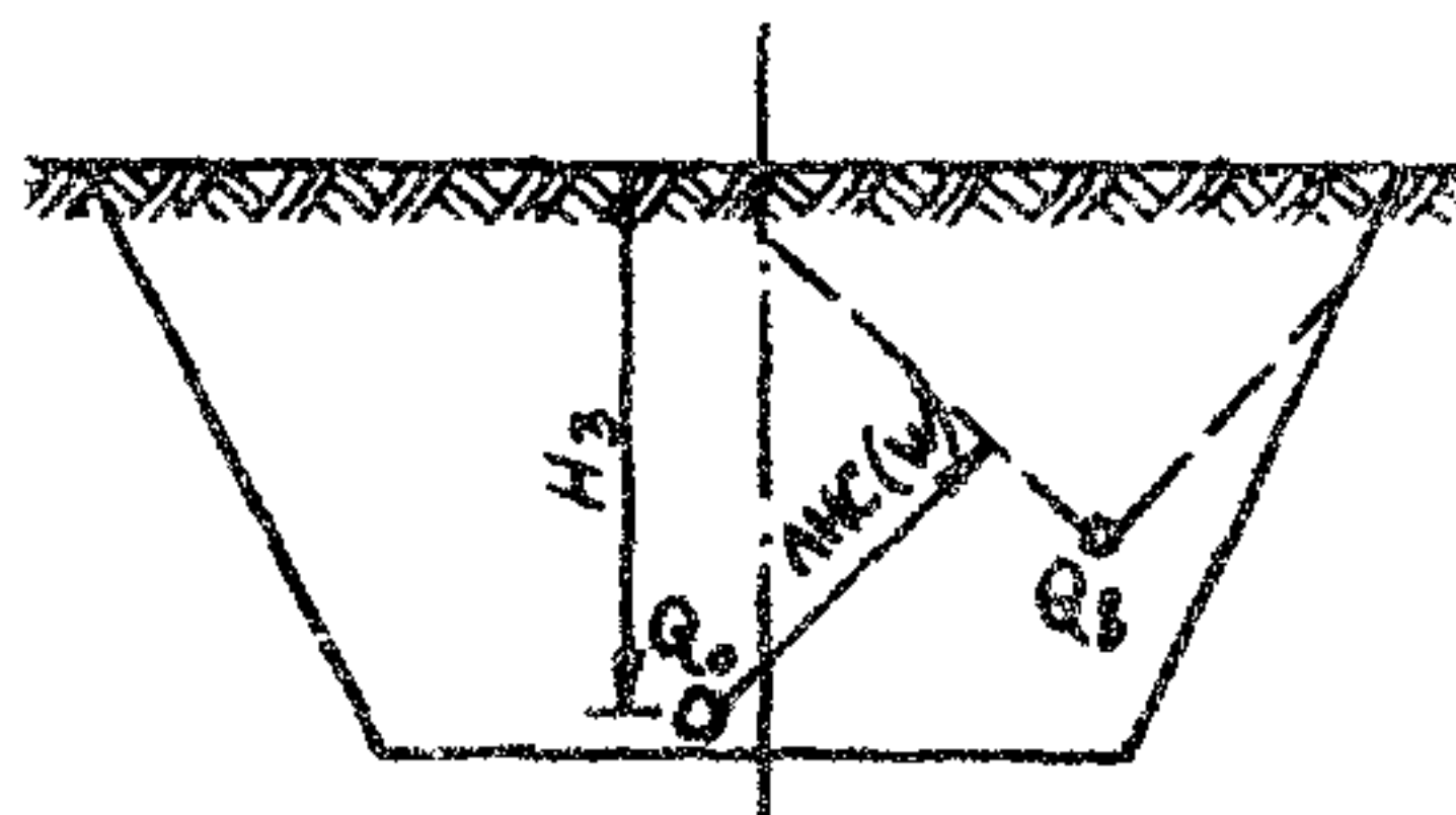
Рис. 12. Схема расположения основного Q_0 и вспомогательного Q_в ряда зарядов в поперечном профиле выемки при направленном выбросе
