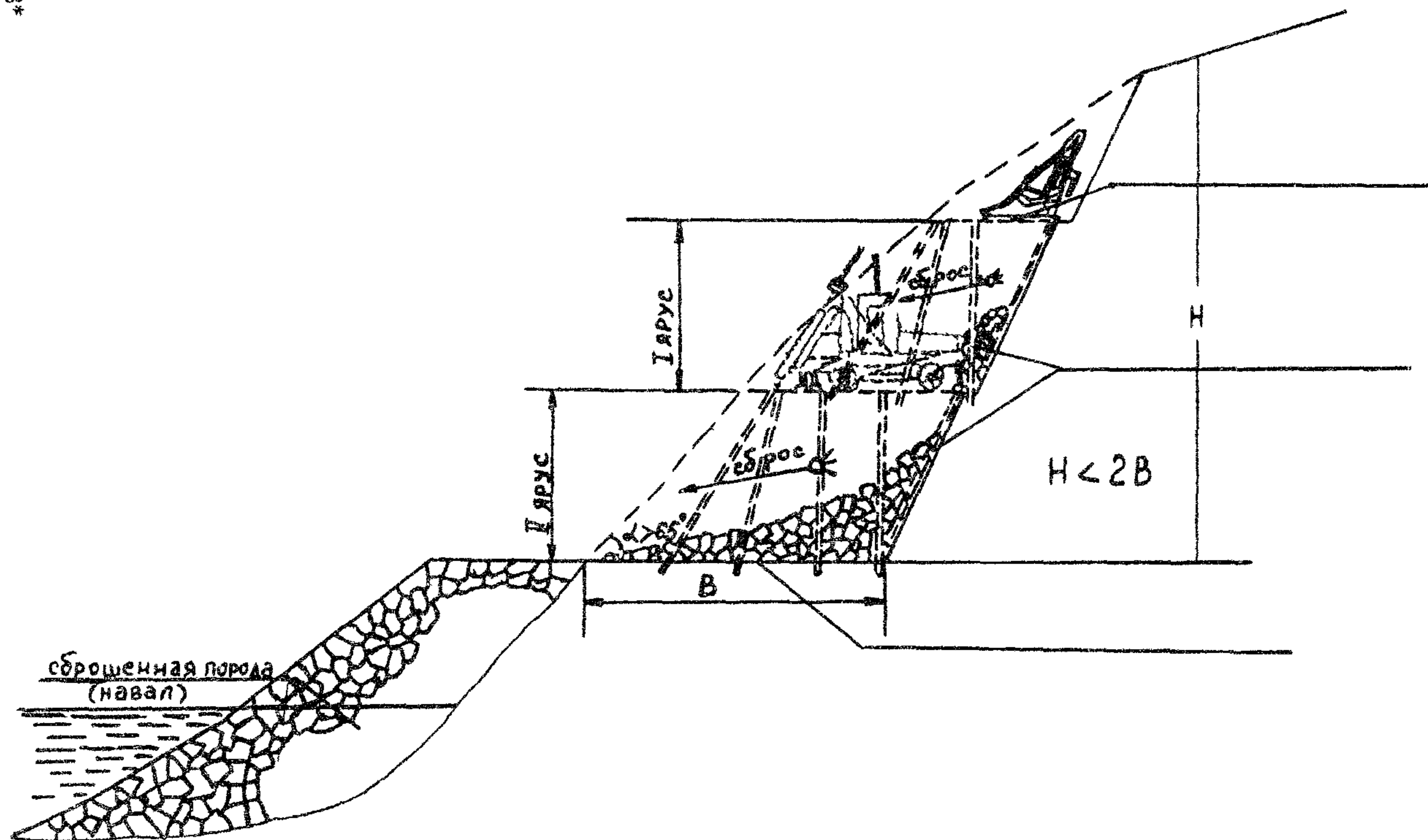
Рис 13 Схема взрыва на сброс
