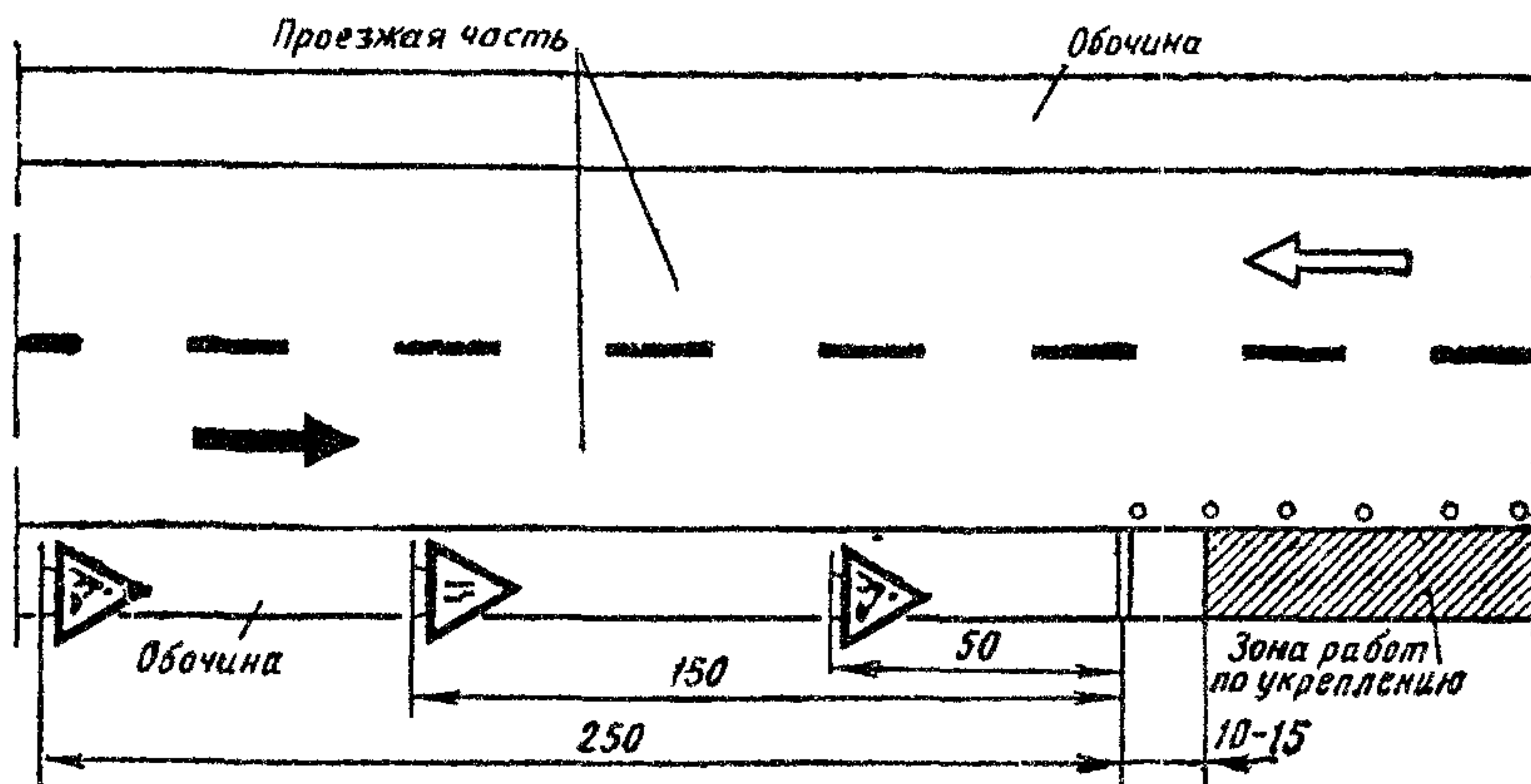
Рис. 4.1. Схема ограждения участка работы по укреплению обочины
