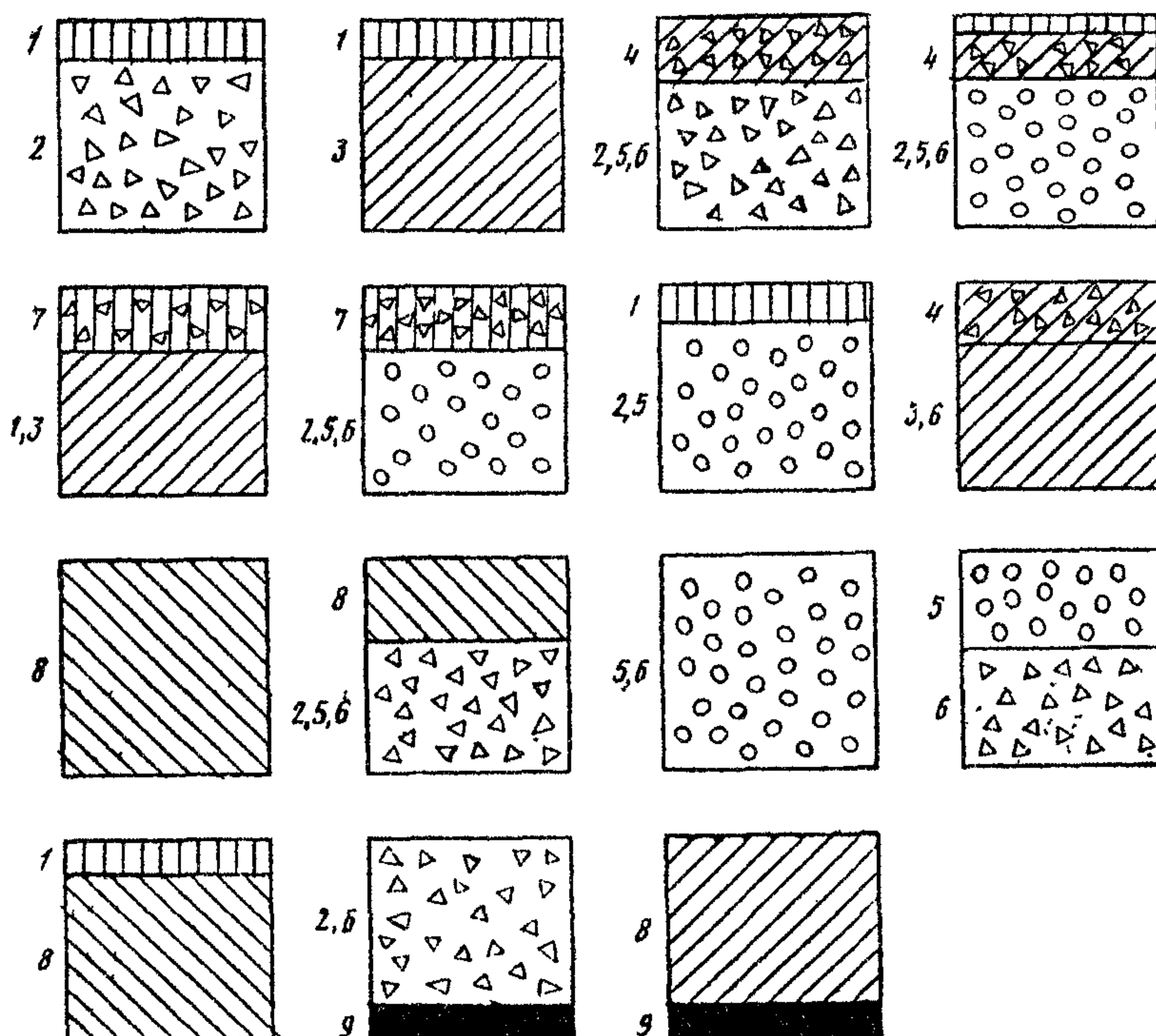
Рис 3.1. Материалы слоев укрепления обочин
