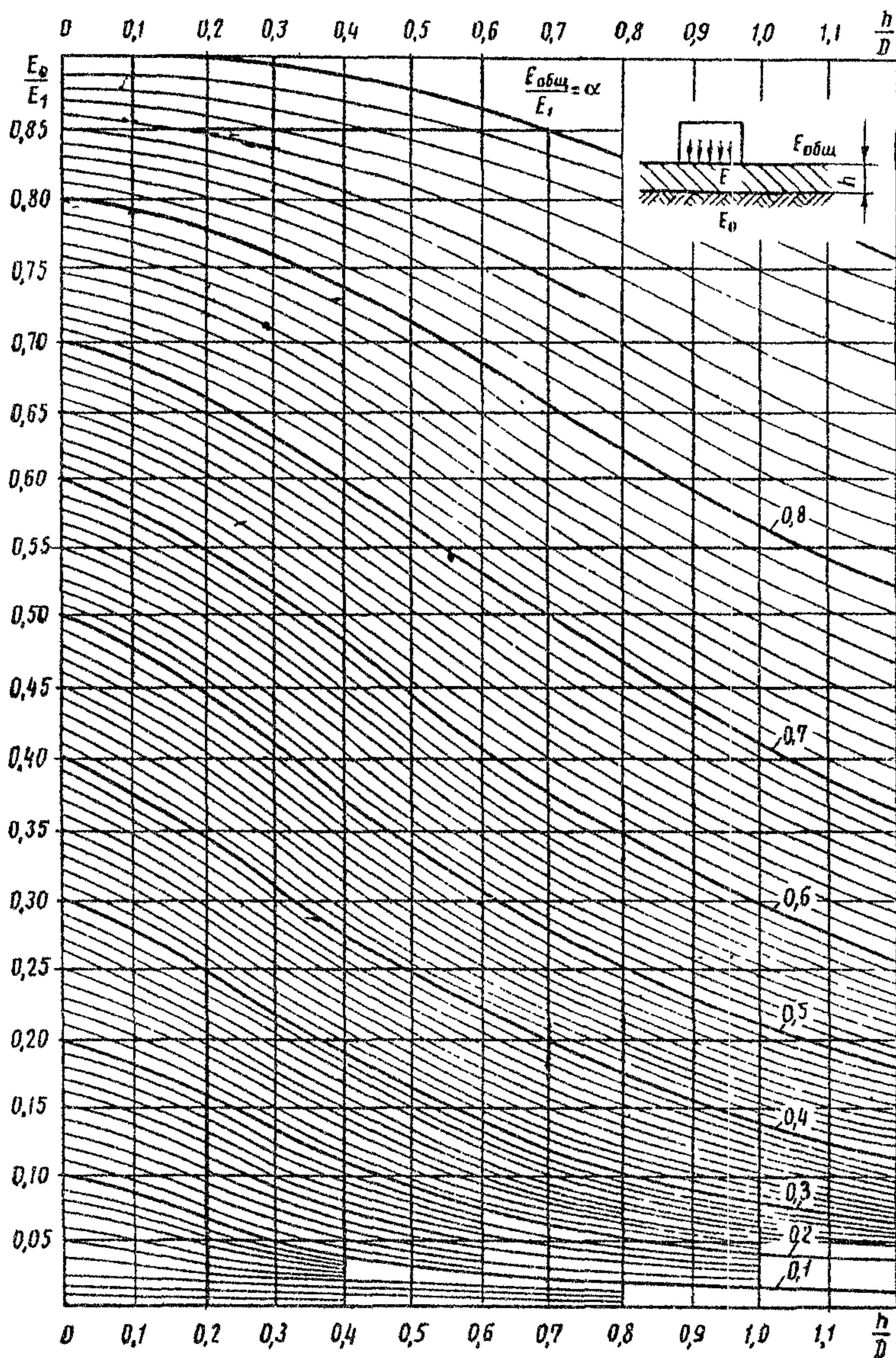
Рис. 2.2. Номограмма для расчета слоев укрепления обочин: E_0 — модуль упругости грунта; E_1 — то же слоя укрепления; E_{\text{общ}} — то же, конструкции укрепления, получаемый в результате расчета. h — толщина слоя укрепления; D — диаметр штампа, равный 33 см
