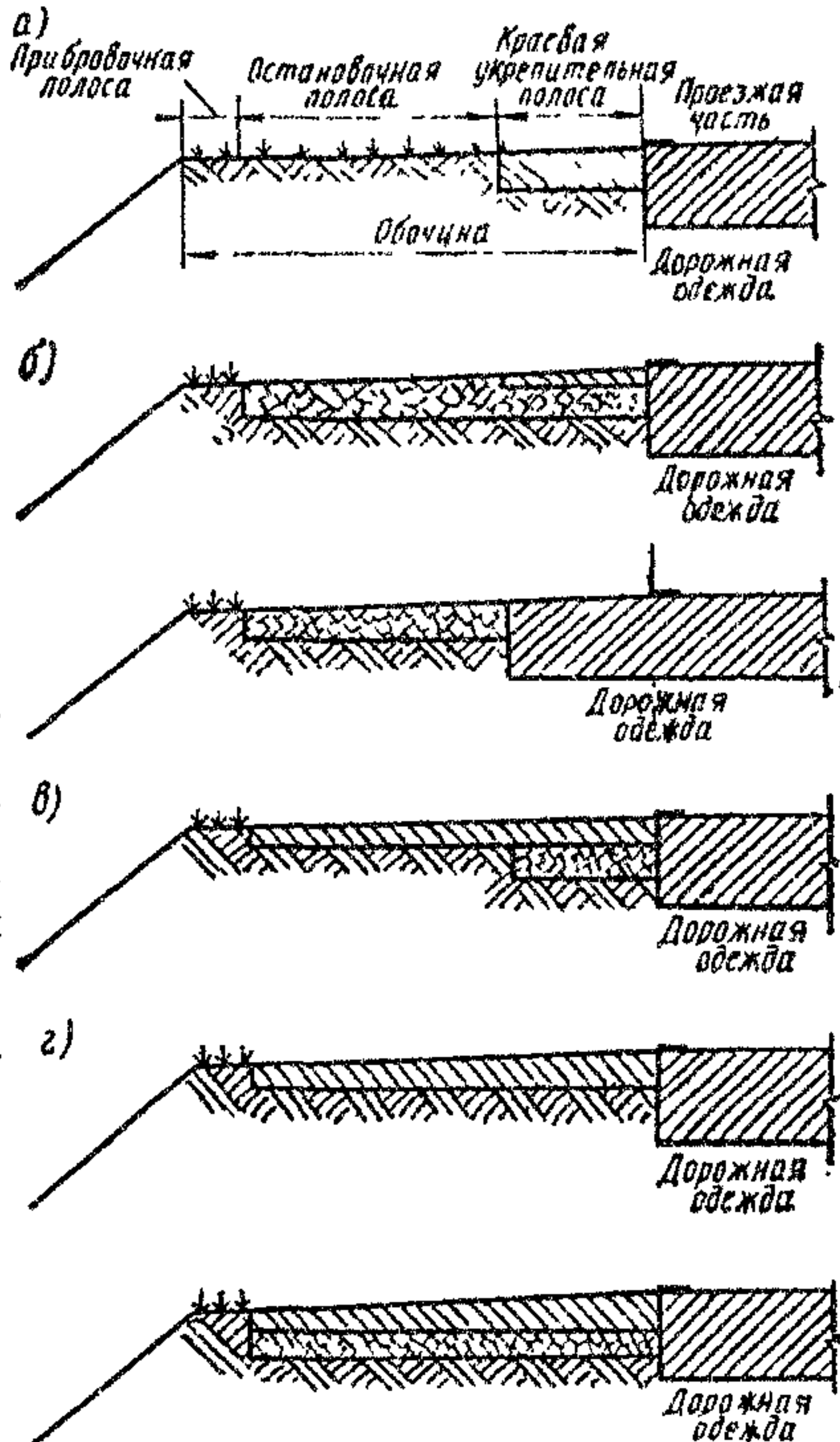
Рис. 1.2. Конструкции укрепления обочин:
