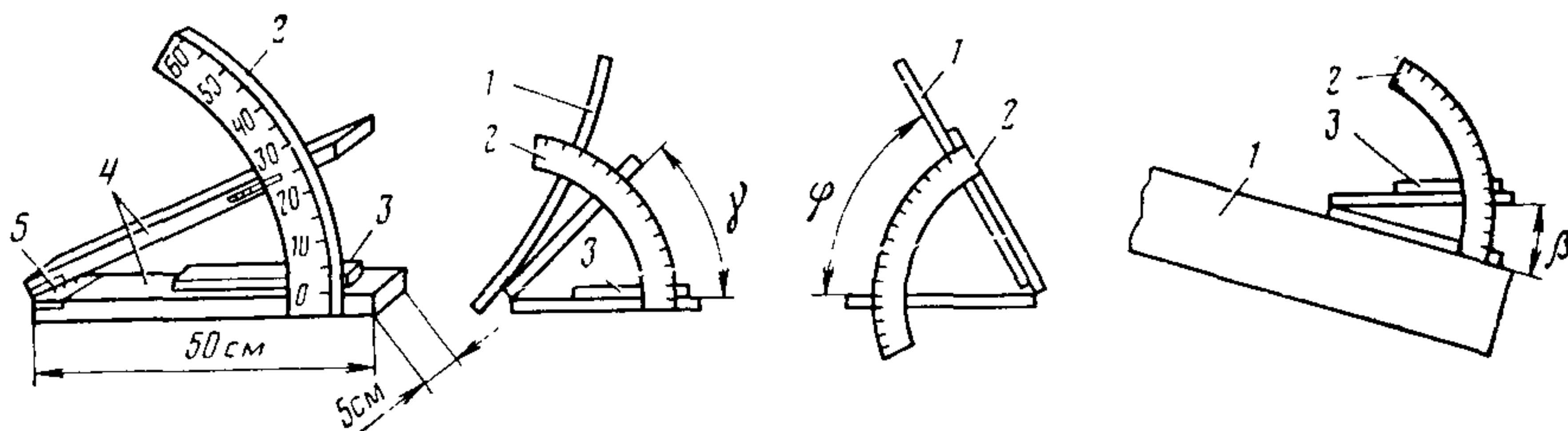
Рис. 3.1. Угломер и его установка при замере углов захвата \varphi , резанья \gamma и наклона \beta :
