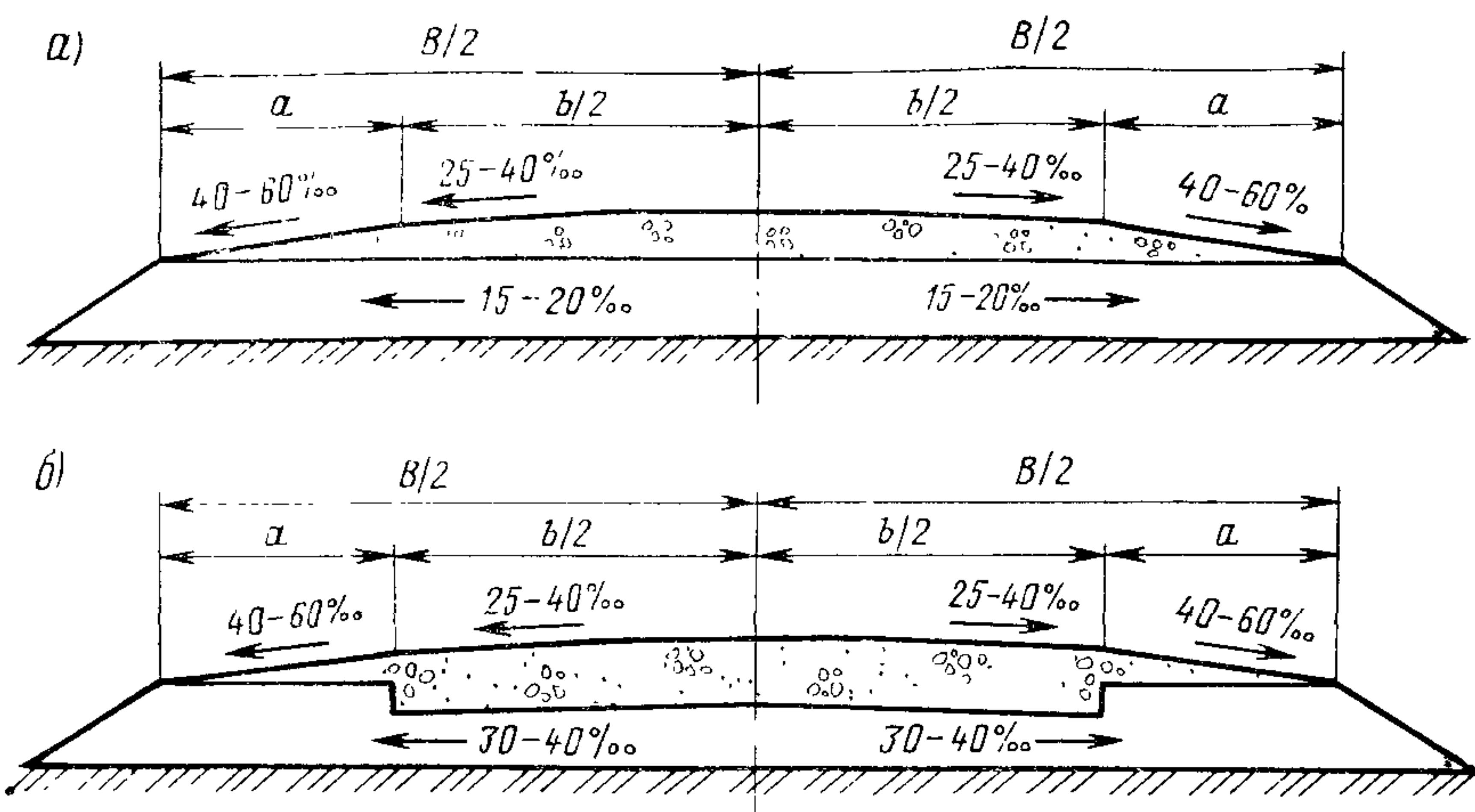
Рис. 1.1. Поперечные профили:
