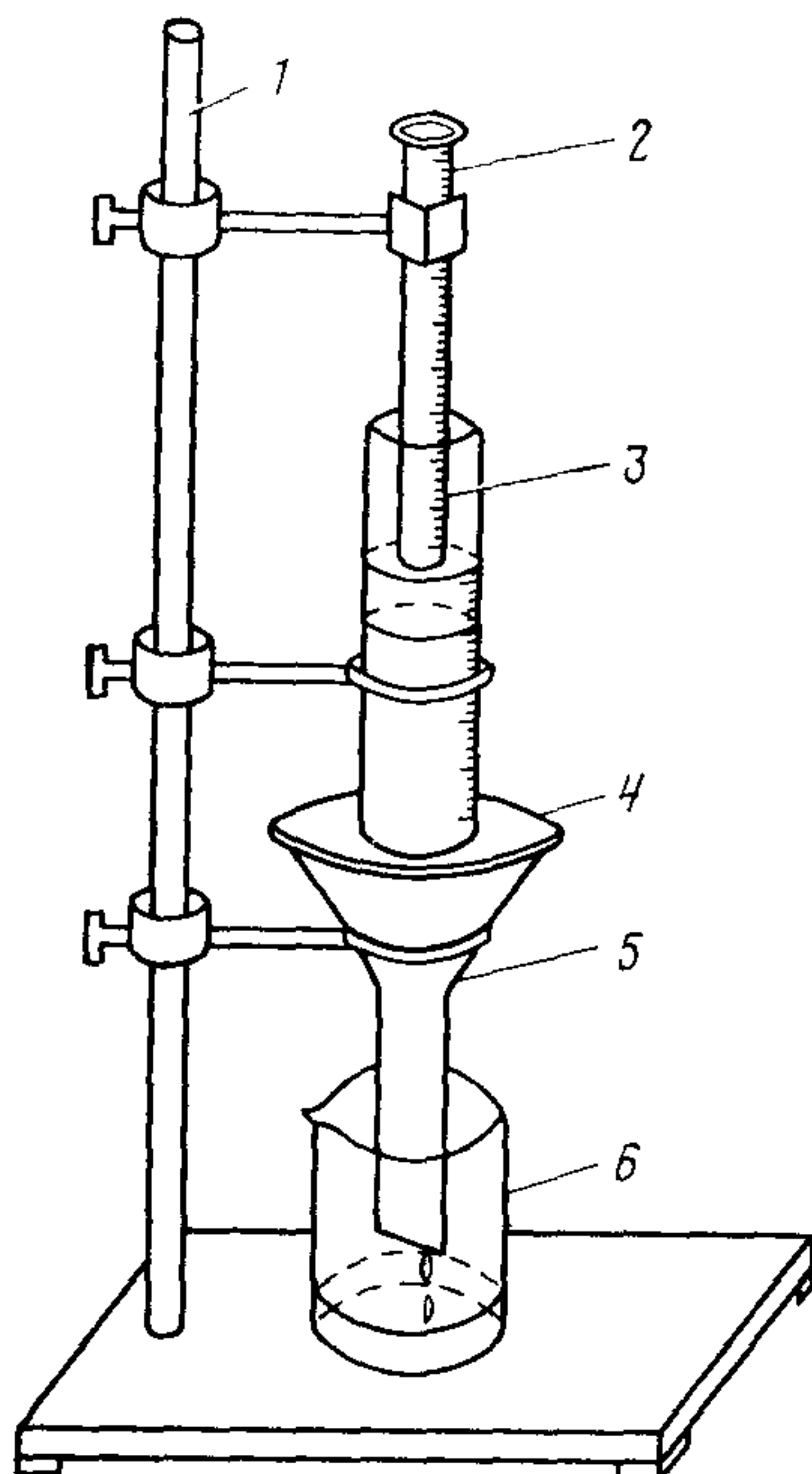
Рис. 1. Прибор для определения водостойкости лигносульфонатов технических
