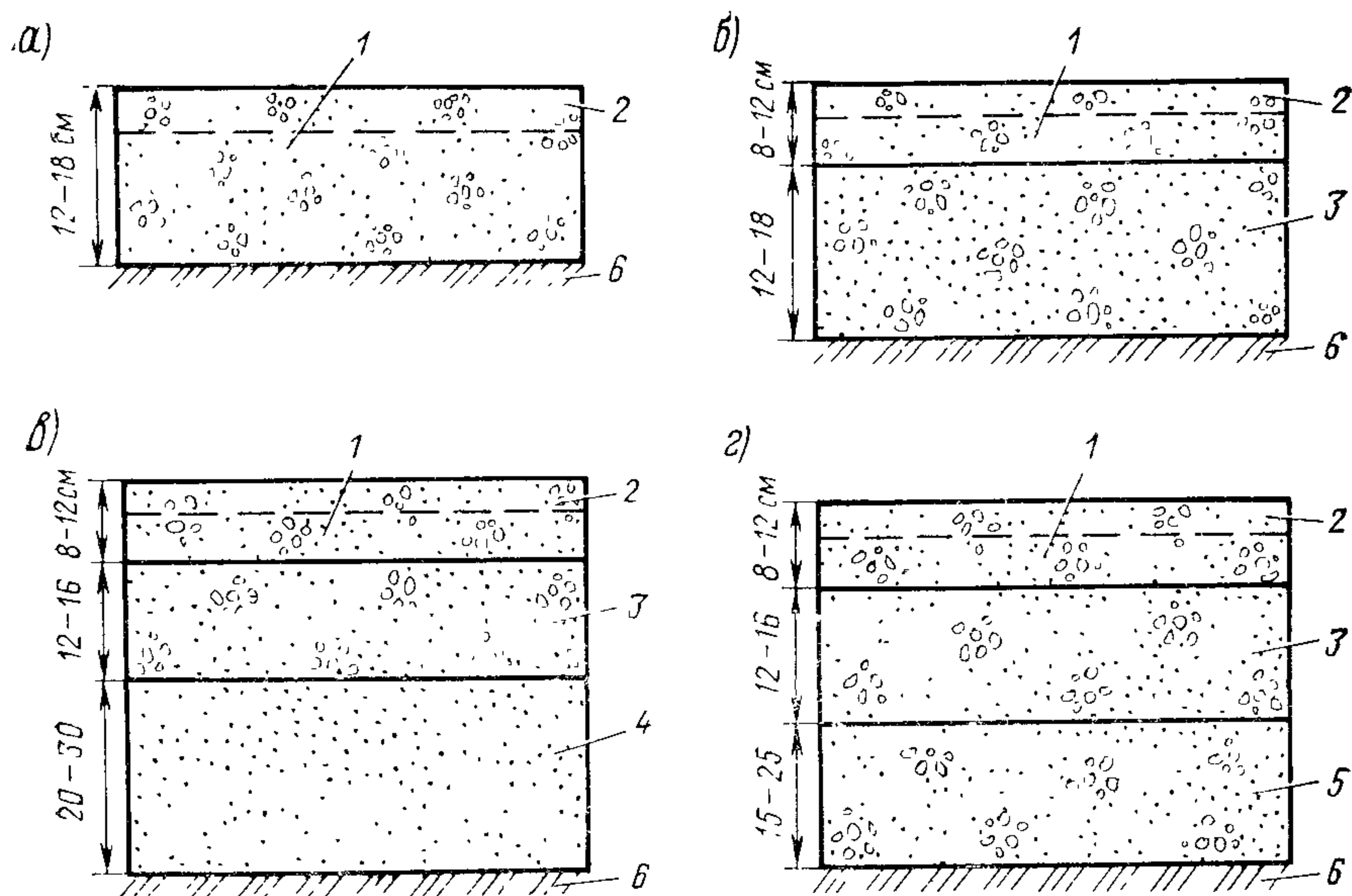
Рис. 1.2. Примеры конструкций дорожных одежд с гравийными покрытиями: a — однослойным; b — двухслойным; в — двухслойным на дополнительном песчаном слое; г — трехслойным; 1 — песчано-гравийно-щебеночная смесь (см. табл. 2.1, смесь № 3 и 5); 2 — слой из песчано-гравийно-щебеночной смеси, обработанной обеспыливающими материалами (4—6 см); 3 — песчано-гравийная смесь (см. табл. 2.1, смесь № 1, 2, 4, 6, 7); 4 — песок; 5 — гравийная смесь (см. табл. 2.3, смесь № 1 и 2); 6 — грунт земляного полотна
