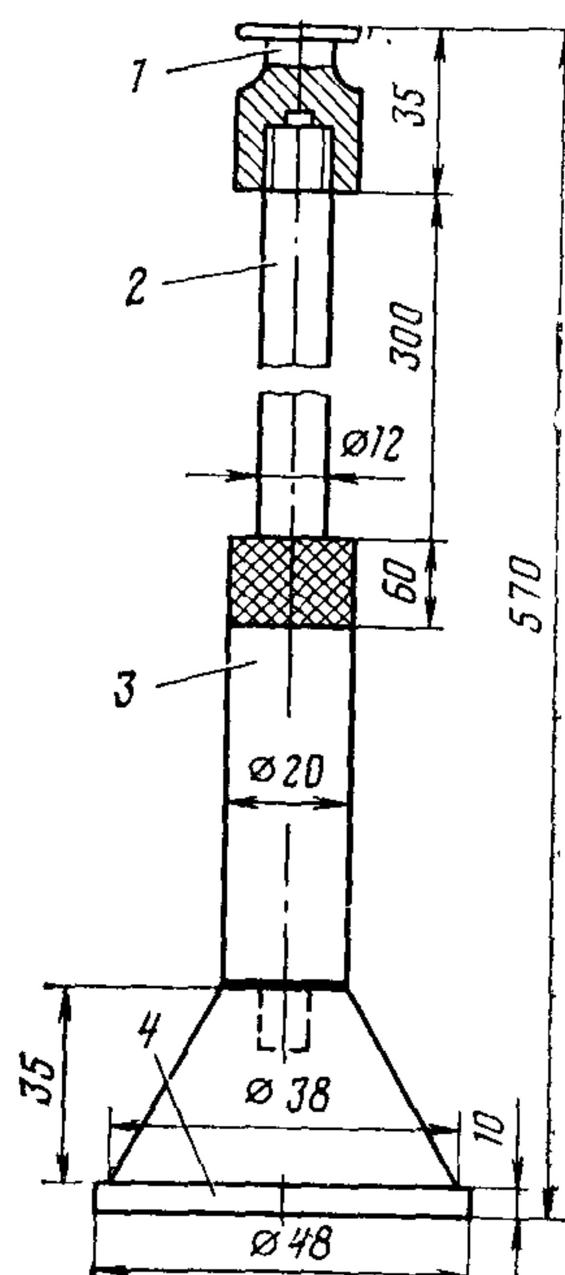
Рис. 2. Уплотнитель:
