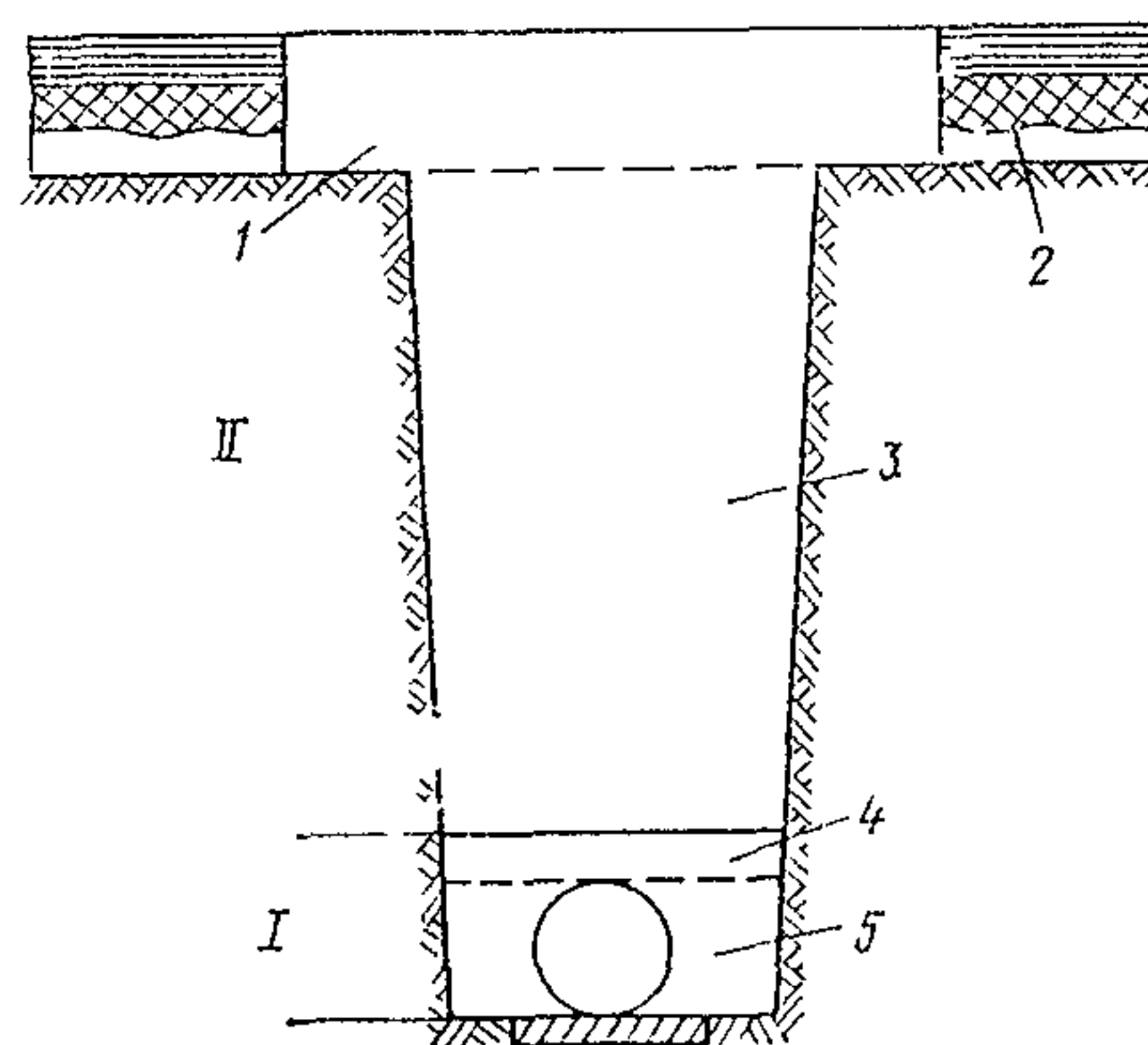
Рис 4 6. Схема засыпки и уплотнения грунта в траншее:
