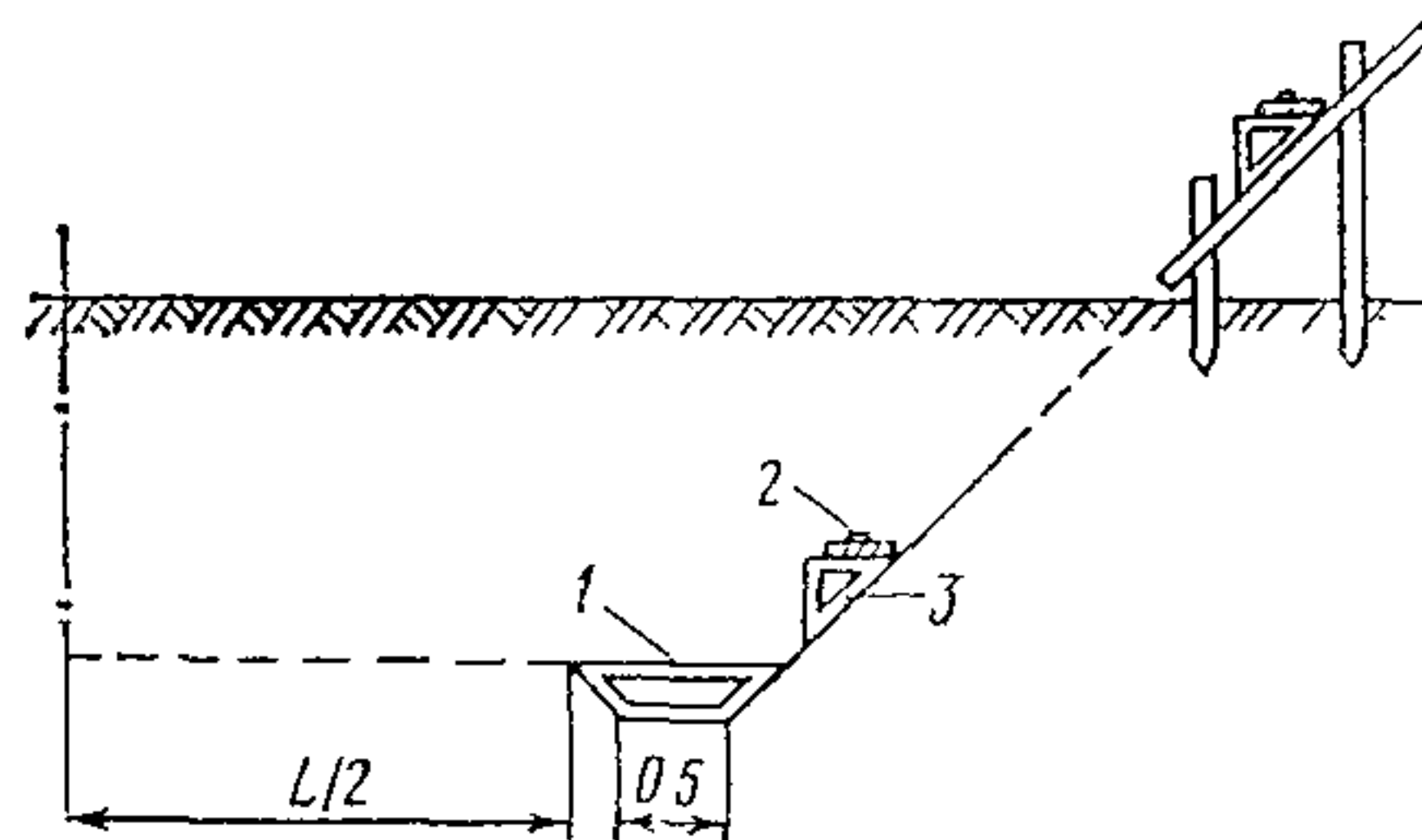
Рис. 3.10. Разбивка выемки 1—шаблон, 2—уровень, 3—лекало
