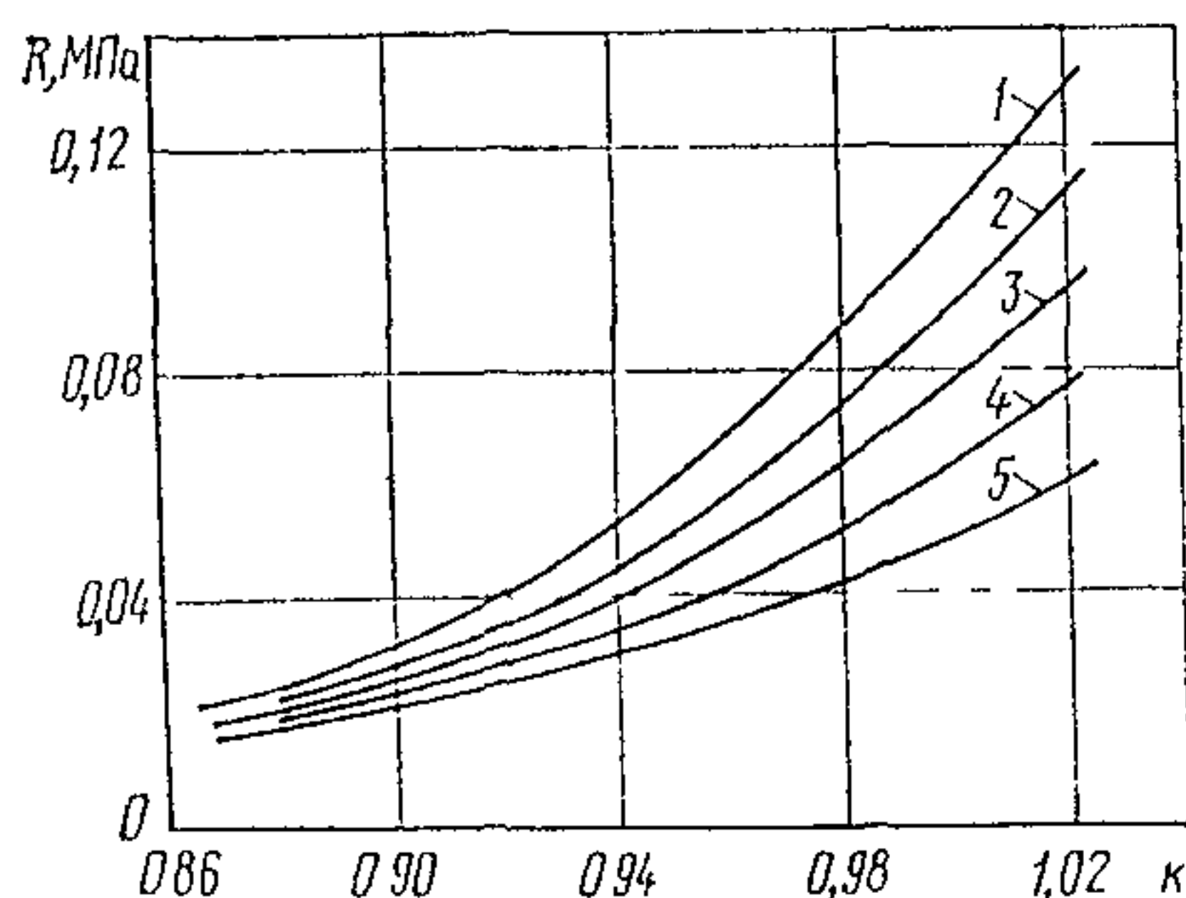
Рис 7 Номограмма для определения коэффициента уплотнения песчаных грунтов средней крупности и крупных по результатам пенетрационных испытаний
