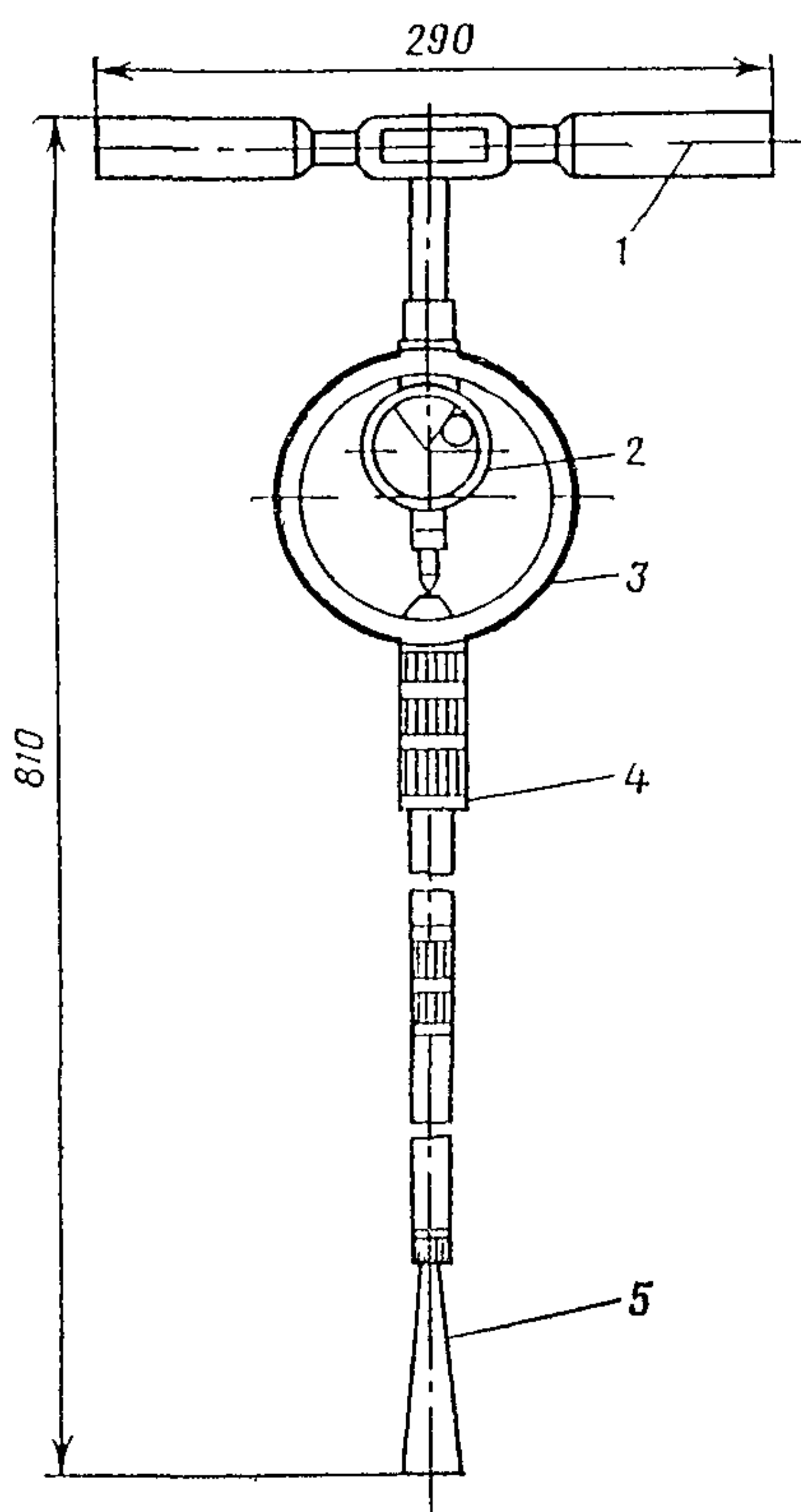
Рис 1. Плотномер пенетрационный статического действия СП
