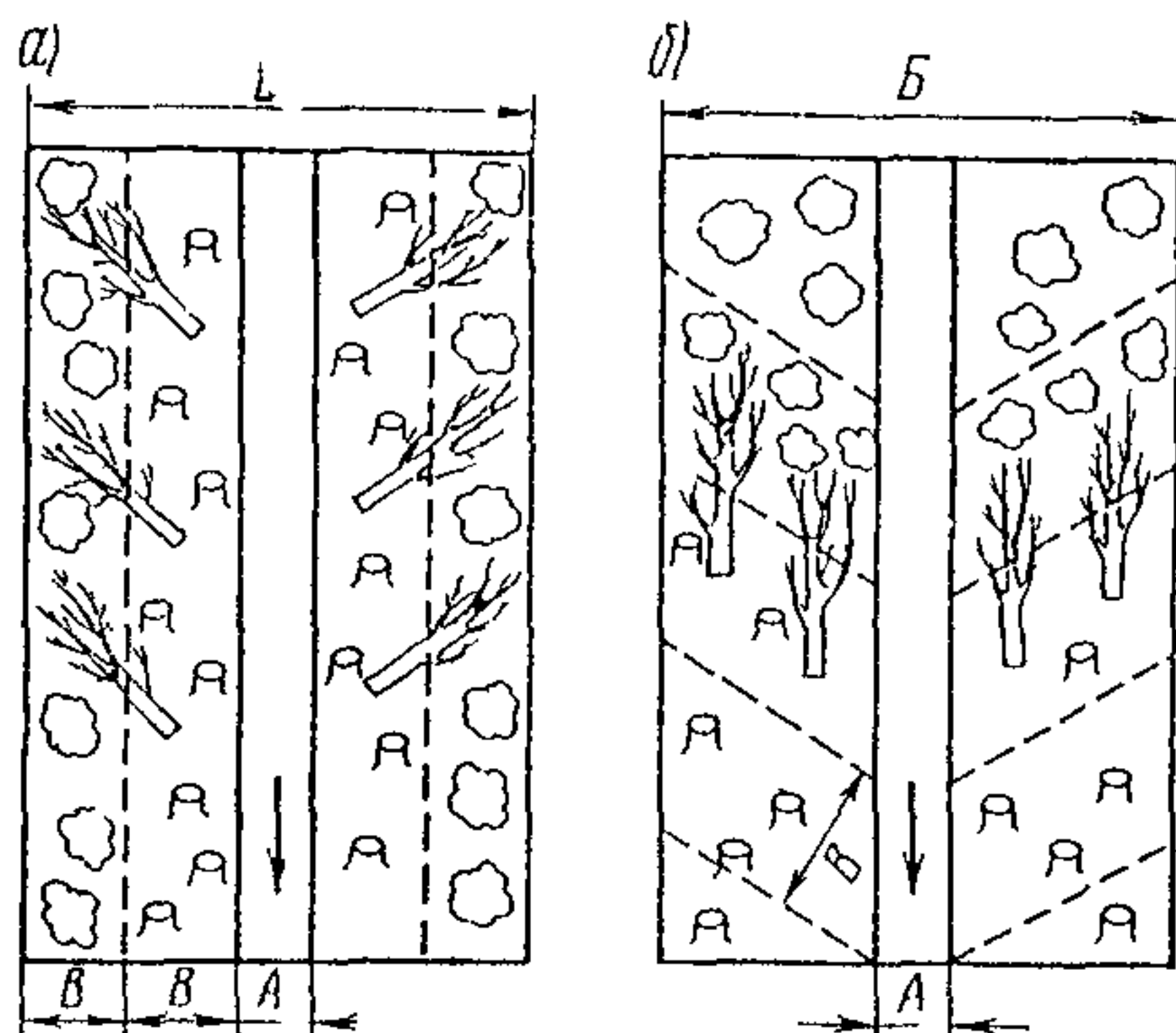
Рис 25 Направление валки деревьев при различных вариантах греблевки а—при разработке продольными лентами б—при разработке лентами, расположенными под углом к волоку А—ширина греблевого волока (5 м) В—ширина пасеки В — ширина ленты 5—7 м
