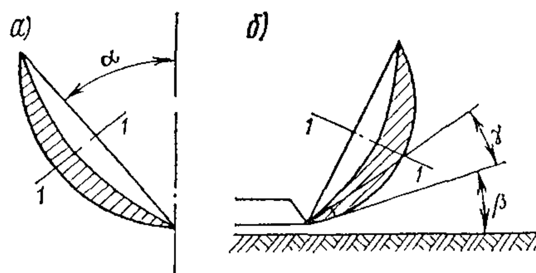
Рис. 3.6. Углы установки дискового плуга грейдер-элеватора:
