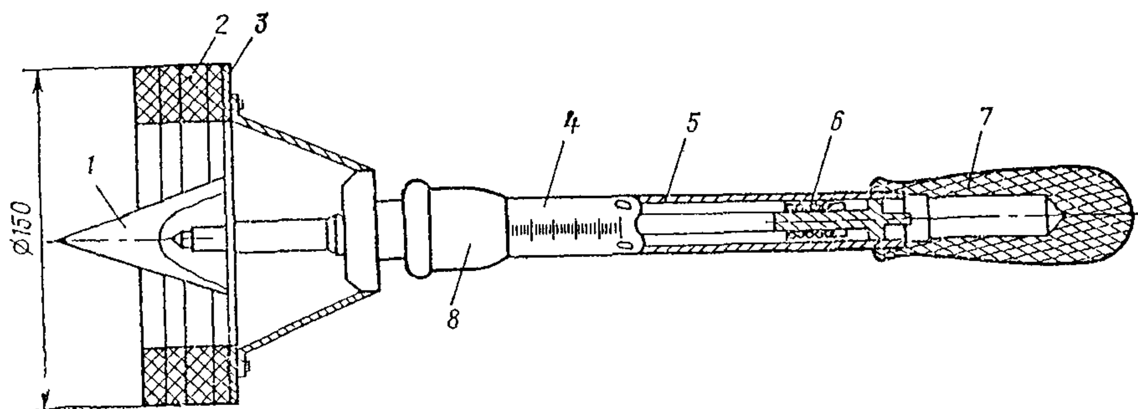
Рис. 4. Пенетромтр:
