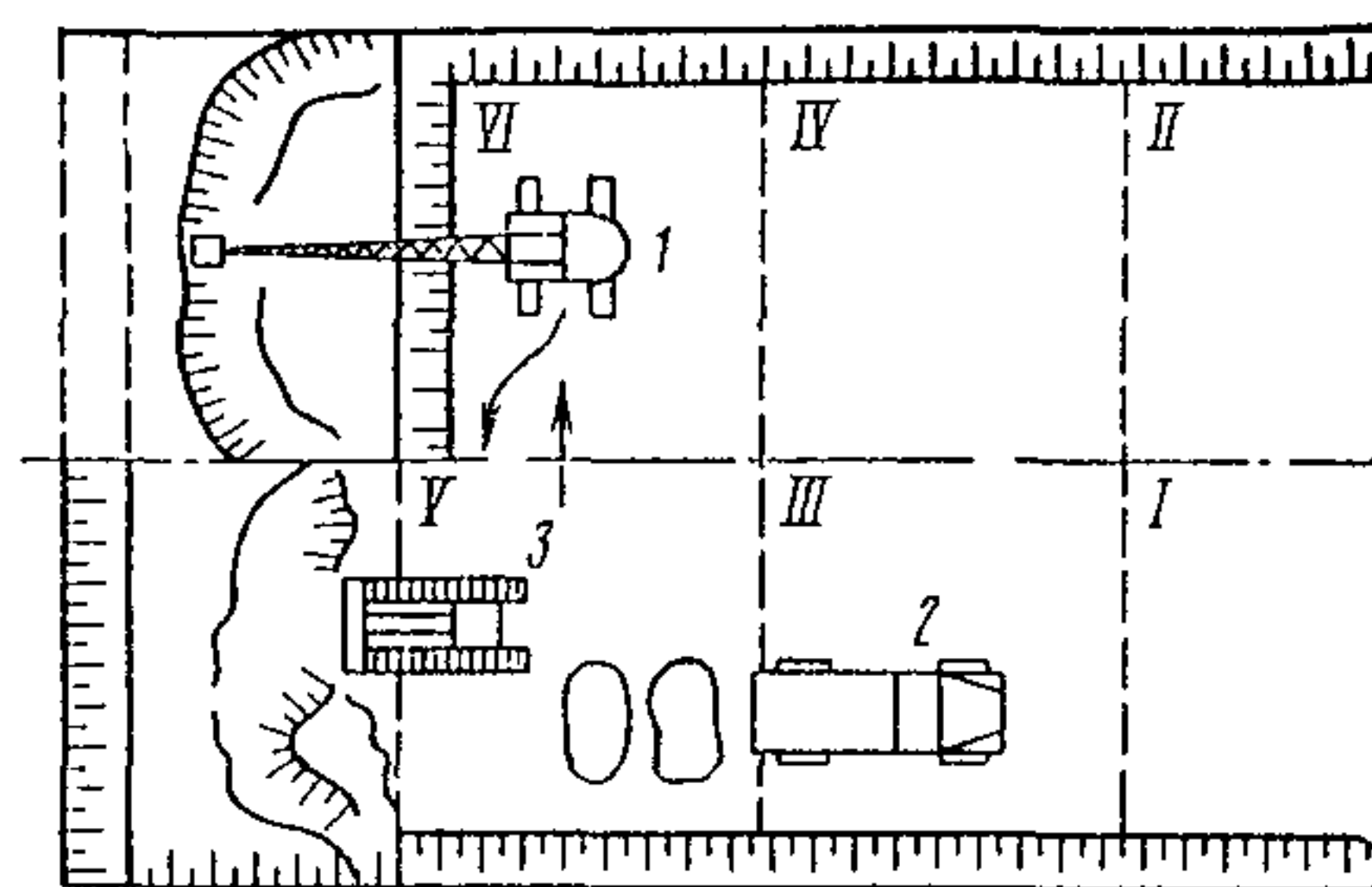
Рис. 12.3. Схема выторфовывания поперечными проходами с перемещением экскаватора на насыпи:
