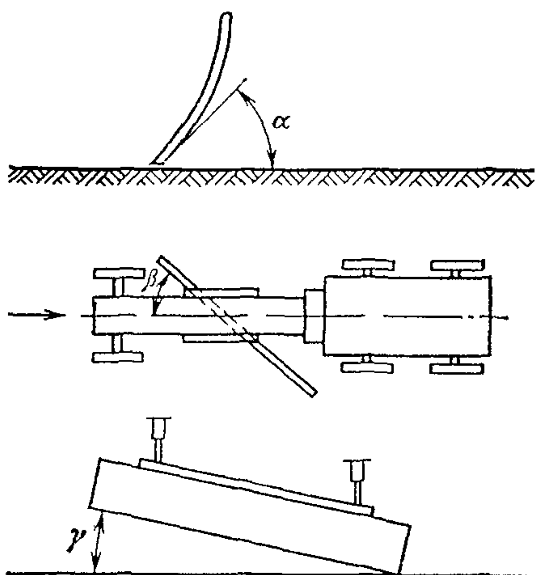
Рис 3 5 Углы установки ножа грей- дера (автогрейдера) \alpha —резания — \alpha , \beta —захвата — \beta , \gamma —накло- на — \gamma
