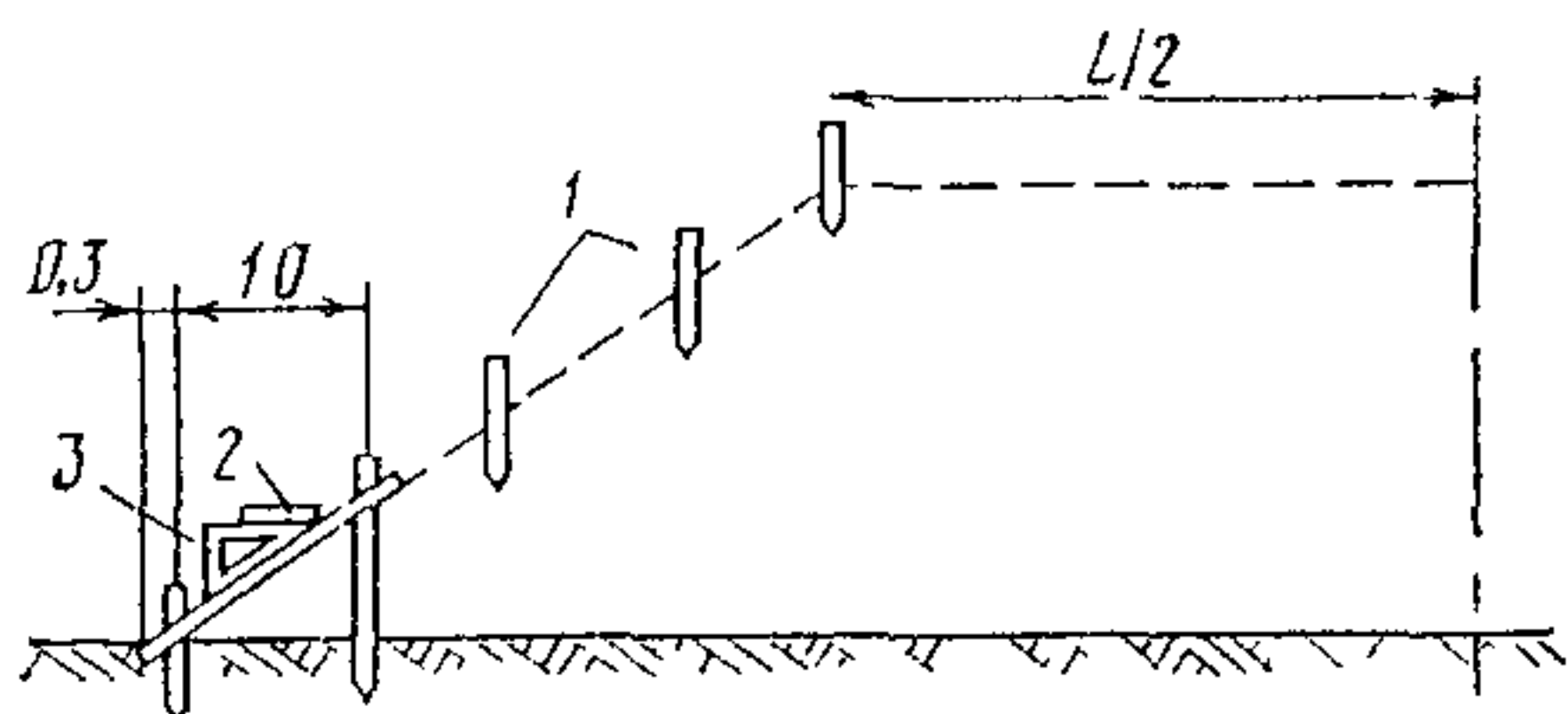
Рис. 3.9. Разбивка насыпи высотой более 1 м в горизонтальной местности
