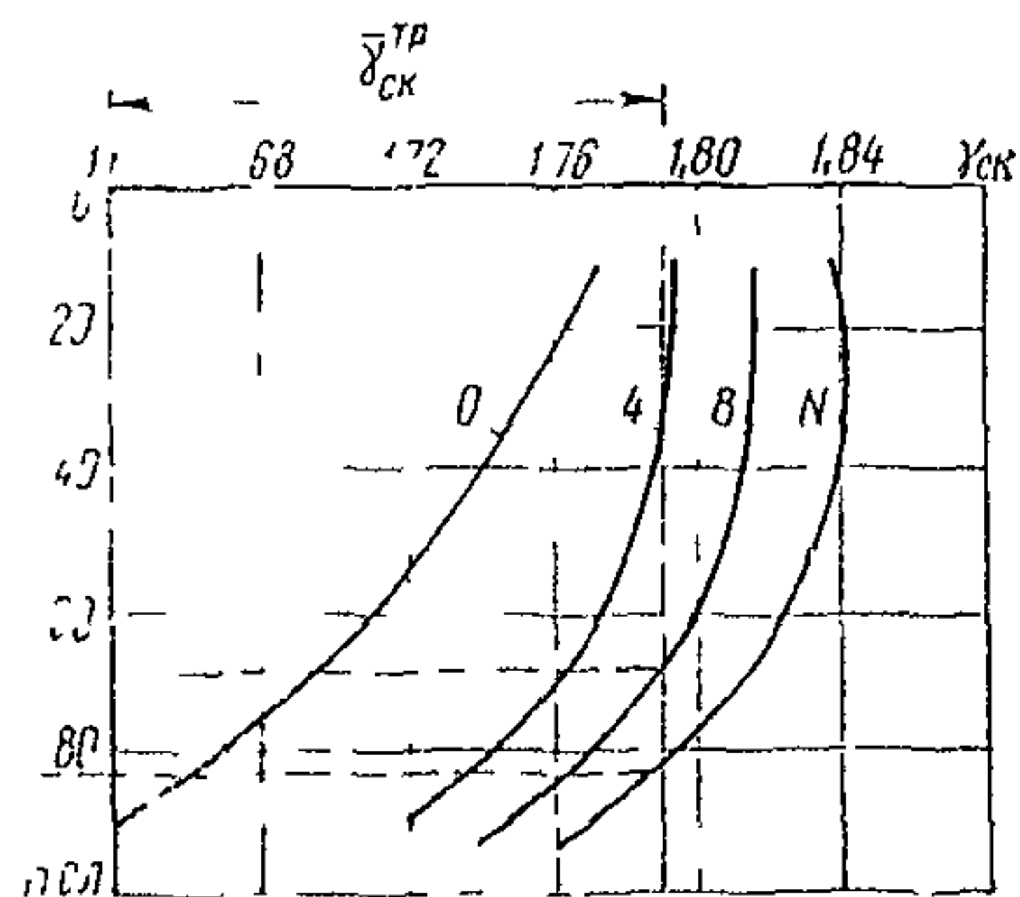
Рис 3 Зависимость плотности сухого грунта по толщине пробного слоя от количества проходов катка по одному следу \bar{\gamma}_{ск} = f(H_{сл}, N) . Цифры на кривых обозначают количество проходов по одному следу, h_{min} , h_{max} — минимальная и максимальная зоны по толщине пробного слоя, в пределах которых достигается требуемое среднеарифметическое значение плотности сухого грунта \bar{\gamma}_{ск}^{тр} при различном количестве проходов катка по одному следу
