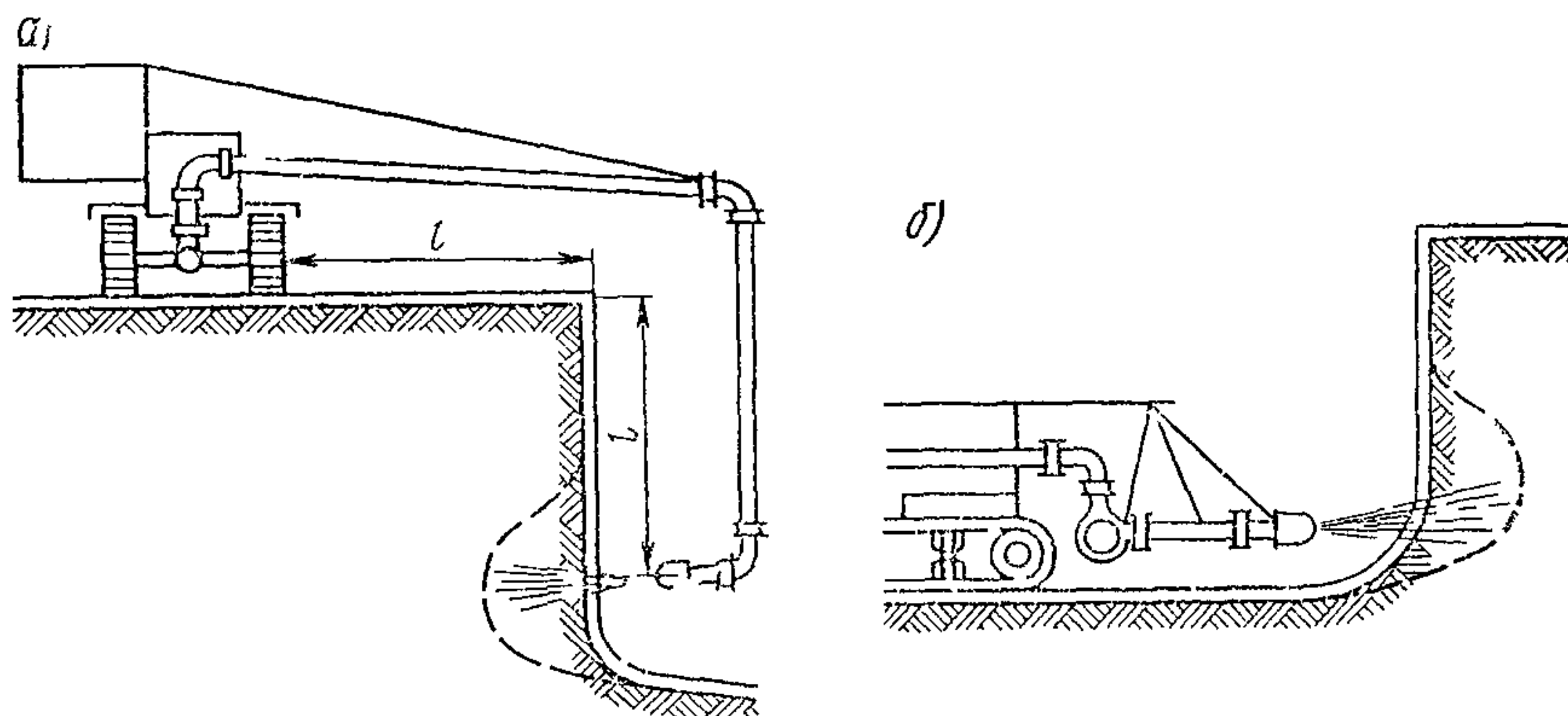
Рис 7.2 Схема установки гидромонитора а—перемещение по верху забоя б—перемещение по подонку забоя
