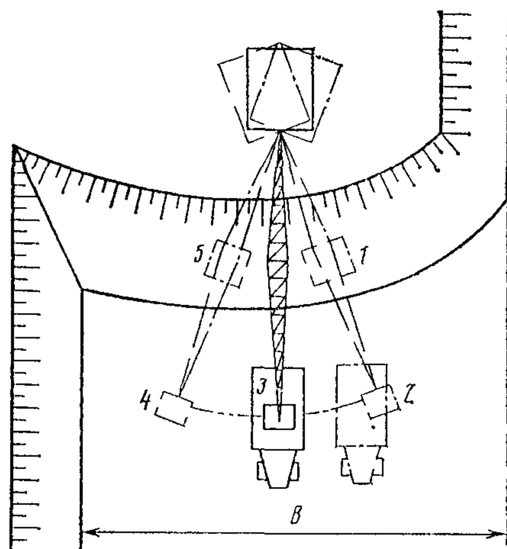
Рис. 3.14. Схема работы экскаватора с оборудованием драглайн при загрузке автомобилей-самосвалов грунтом челночным способом:
