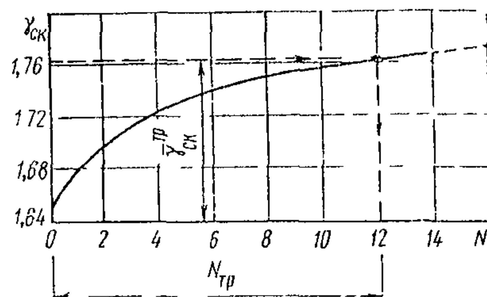
Рис 2 График зависимости плотности сухого грунта от количества проходов катка по одному следу \bar{\gamma}_{ск} = f(N)
