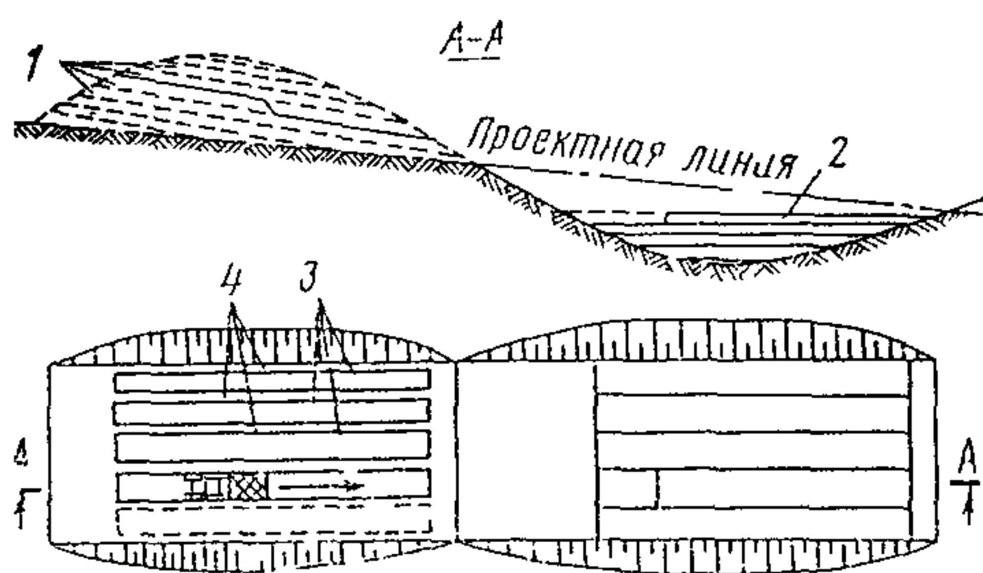
Рис 3 11 Траншейно-ярусная схема разработки грунта.
