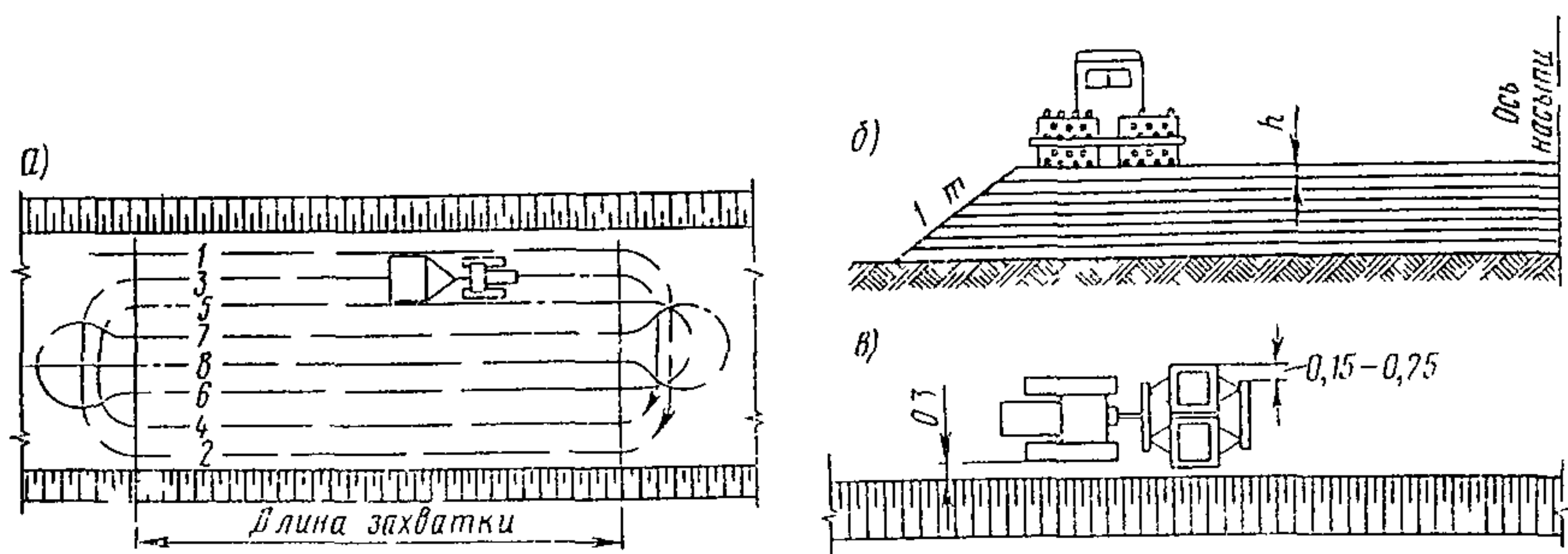
Рис 41 Схема работы прицепных кулачковых катков
