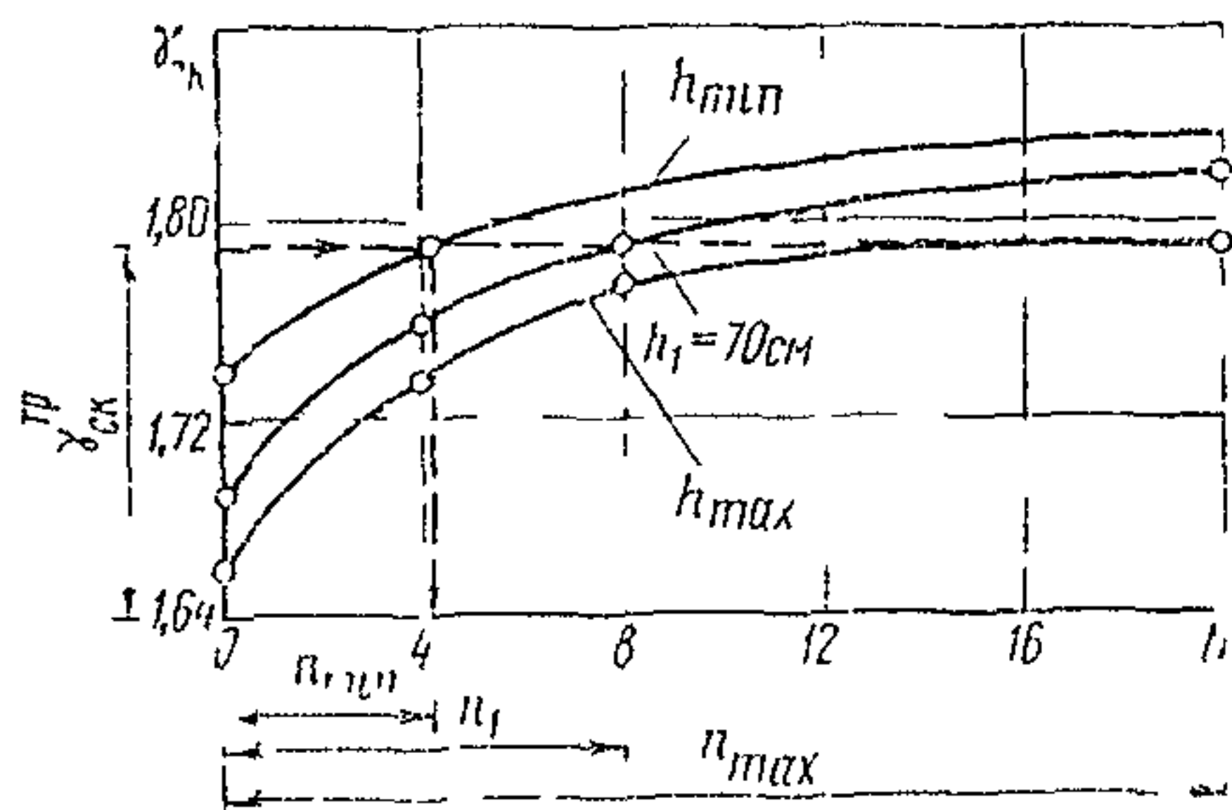
Рис 4 Зависимость плотности сухого грунта от количества проходов катка по одному следу \bar{\gamma}_{ск} = f(N) , для различных значений толщины слоя грунта в интервале (h_{min} - h_{max})
