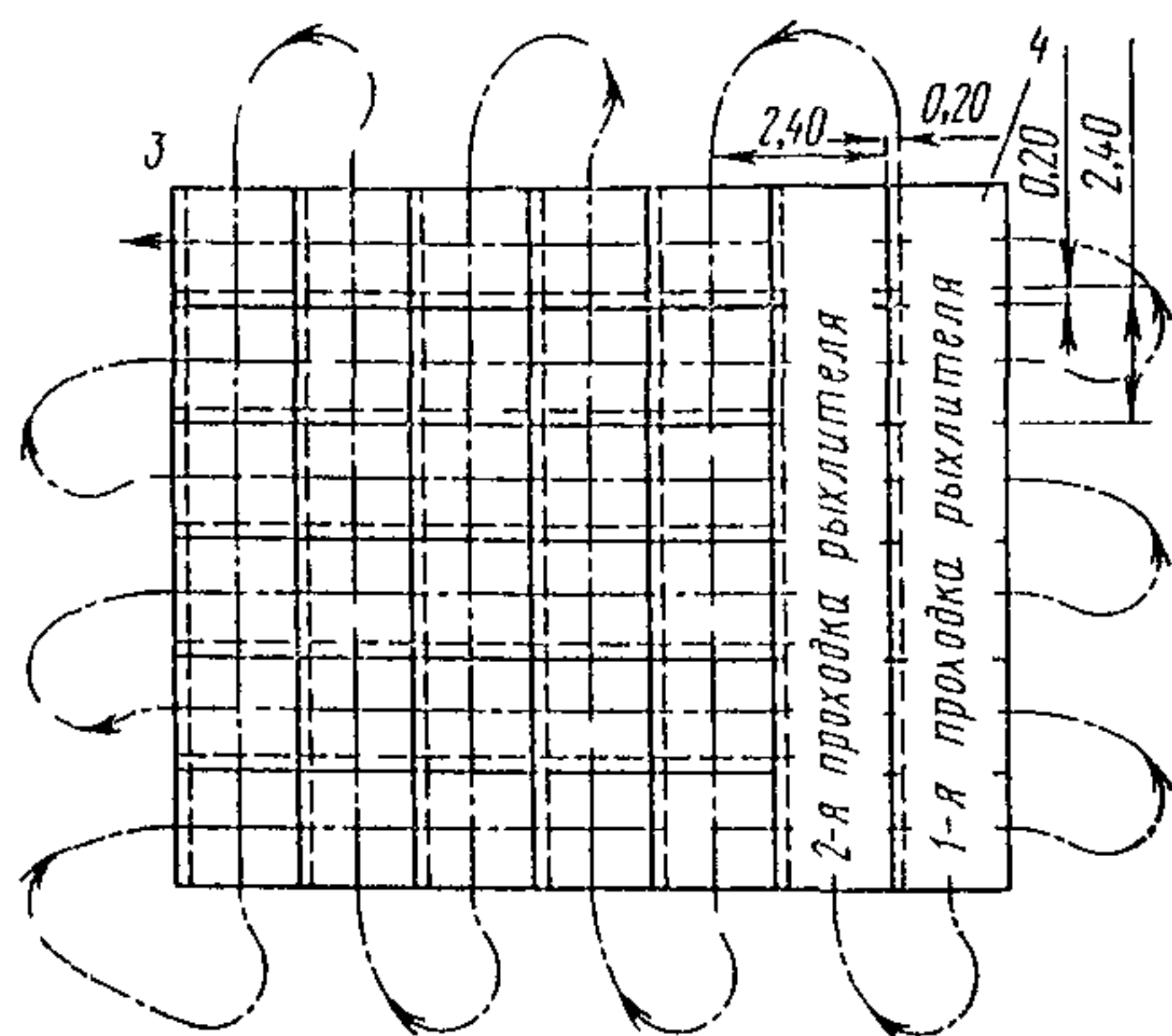
Рис. 9.1. Схема вспахивания грунта при помощи рыхлителя.
