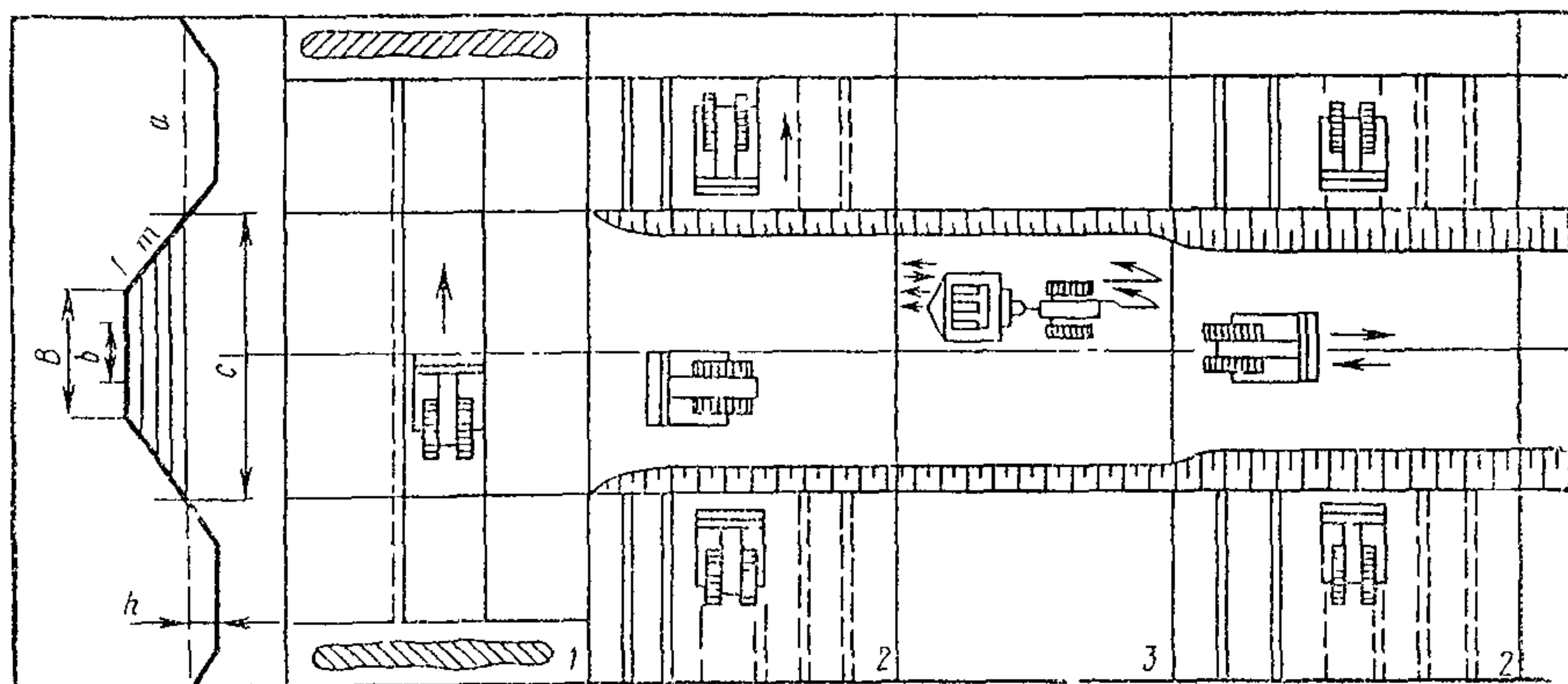
Рис. 3.7. Технологическая схема возведения насыпи 1—снятие плодородного слоя почвы с укладкой в боковые валы, 2—отсыпка отдельных выравниванием его в насыпи, 3—последовательное уплотнение грунта в насыпи; 4—планировка на- дозером
