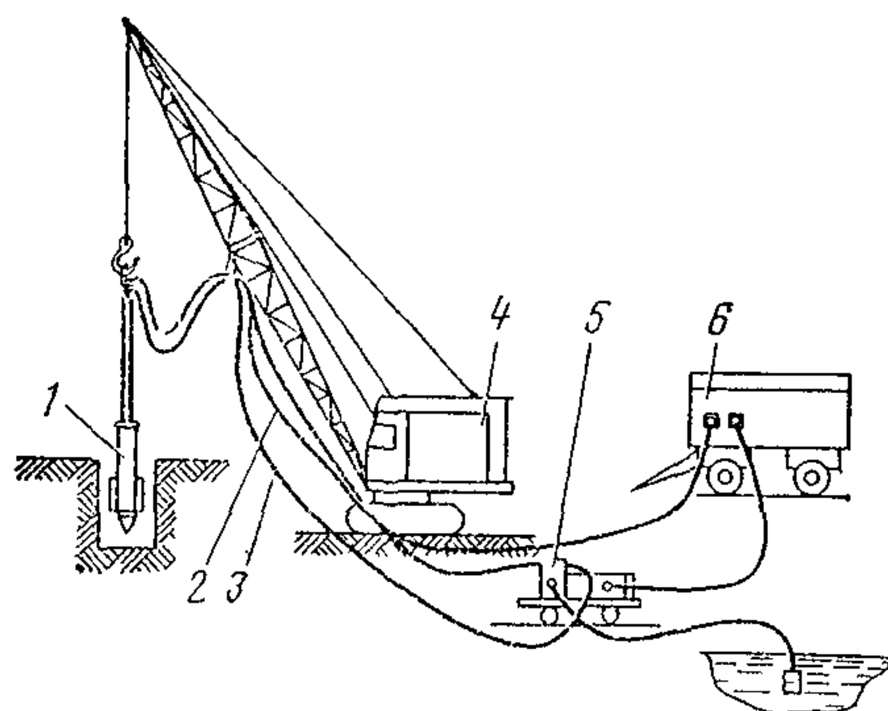
Рис 48 Схема гидровибрационной установки для уплотнения песчаных грунтов
