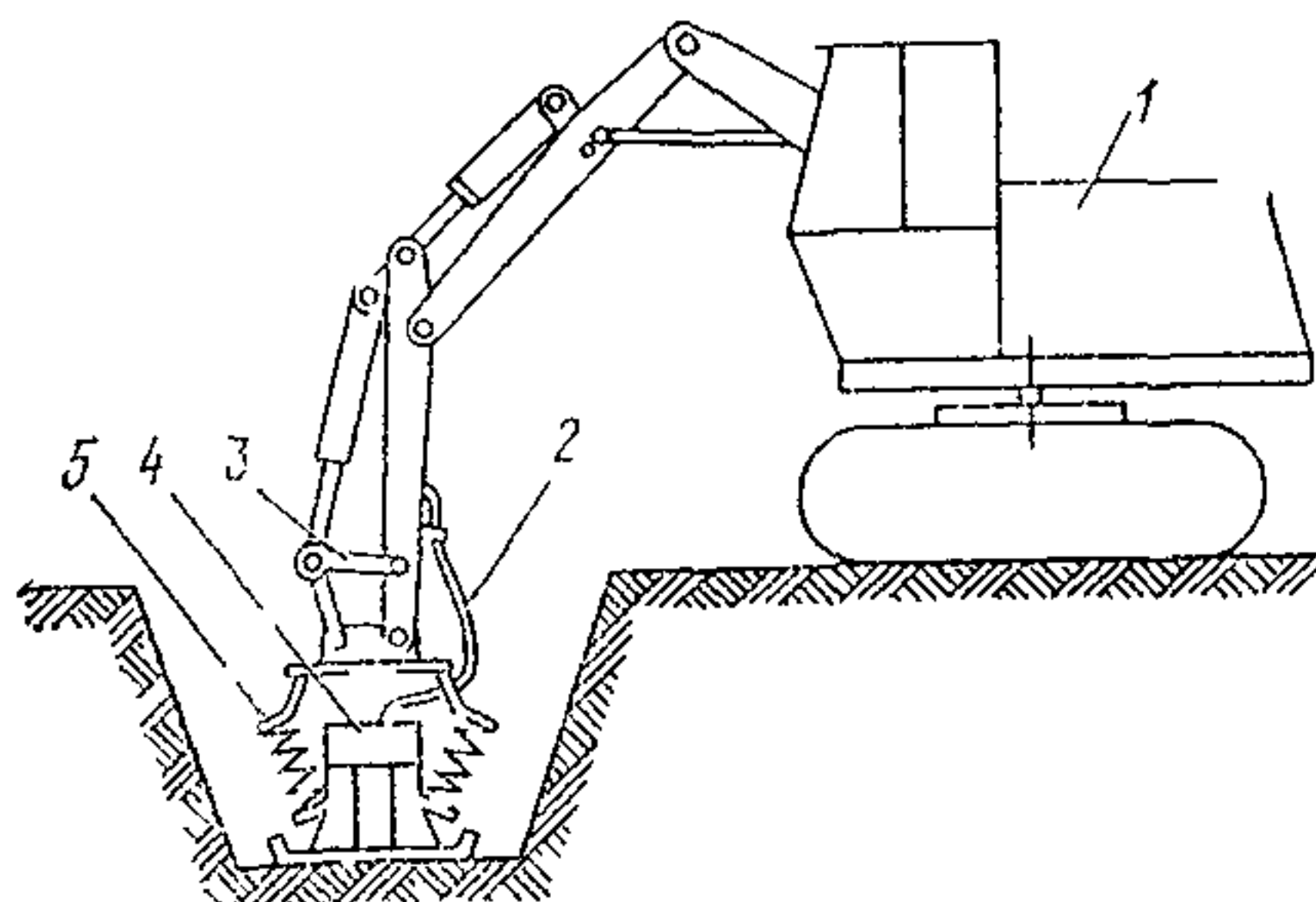
Рис 47 Уплотнение грунта обратной засыпки траншей
