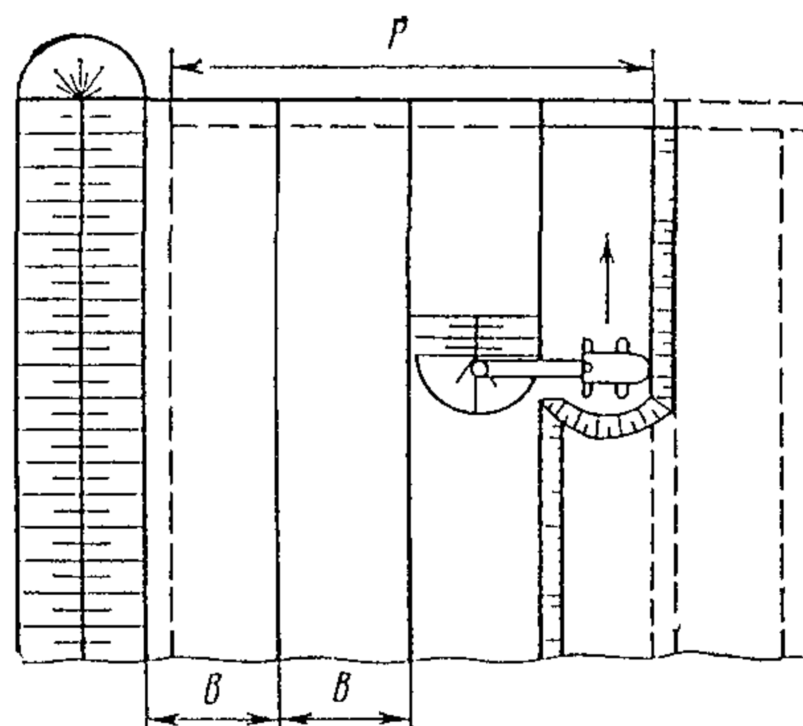
Рис. 9.2. Схема предохранения грунта от промерзания методом перелопачивания:
