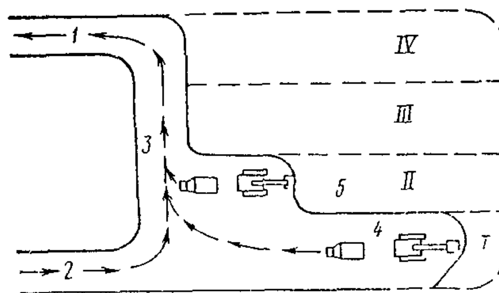
Рис 3.13 Схема продольной разработки выемки
