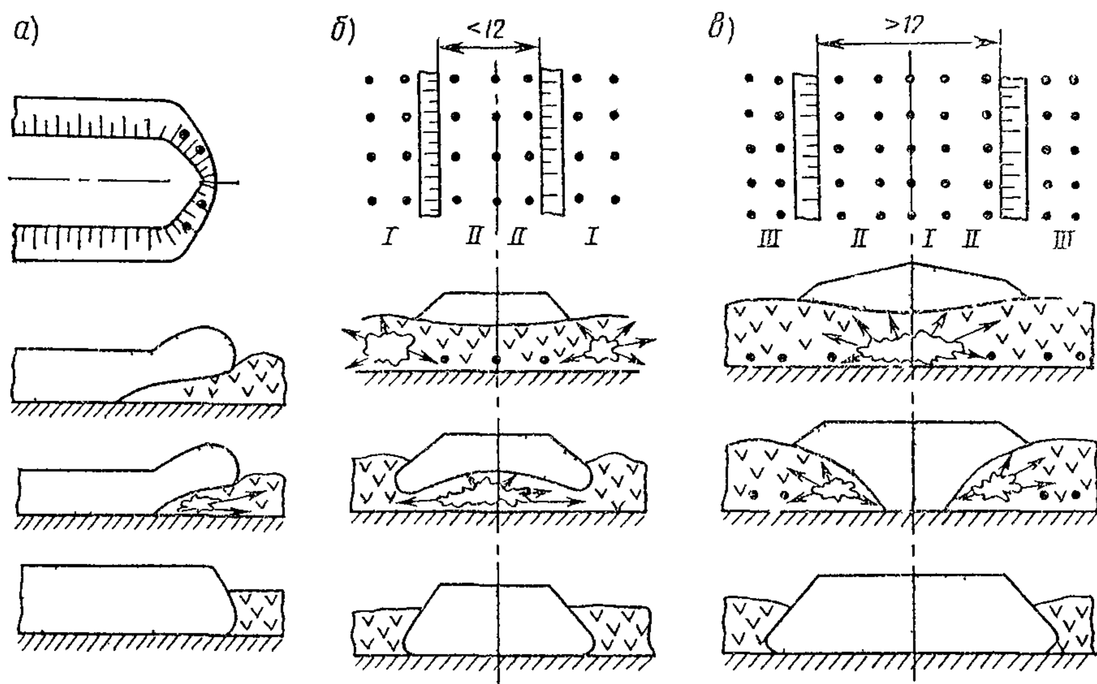
Рис 125 Технологические схемы взрывного выторфования
