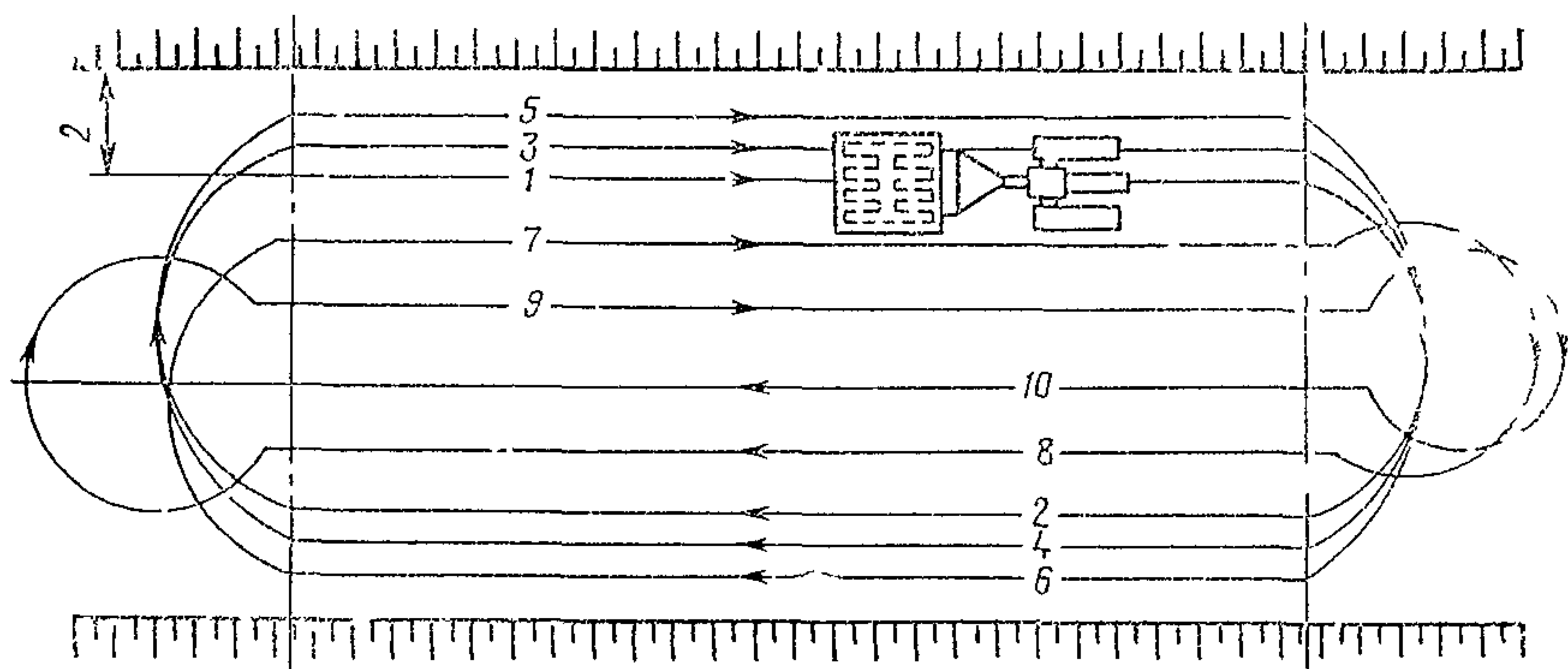
Рис 42 Схема работы прицепного катка на пневматических шинах
