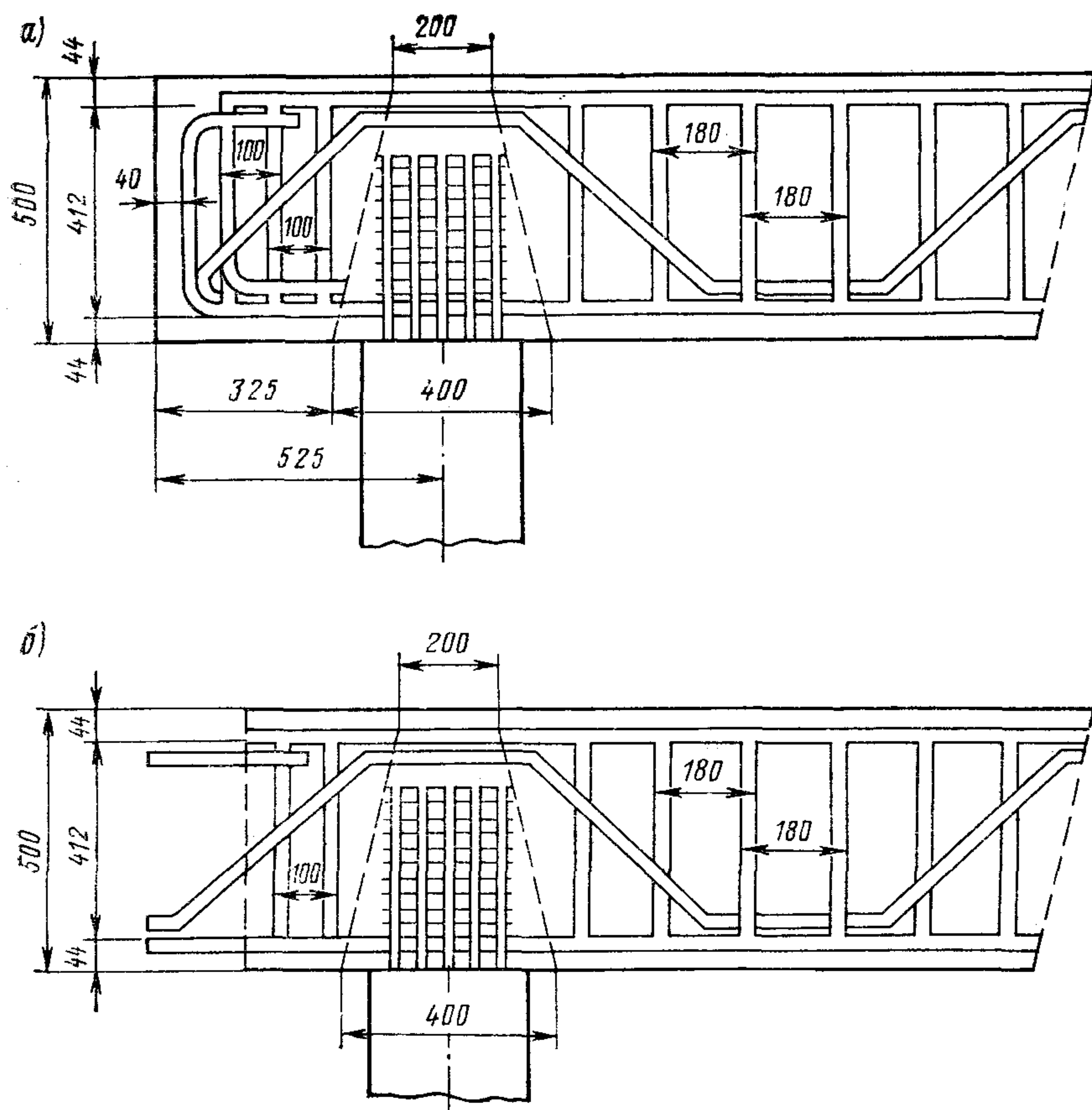
Рис. 6.11. Узел существующей свайной опоры: а — армирование ригеля до уширения; б — обрубка бетона на конце ригеля с оголе- нием арматуры
