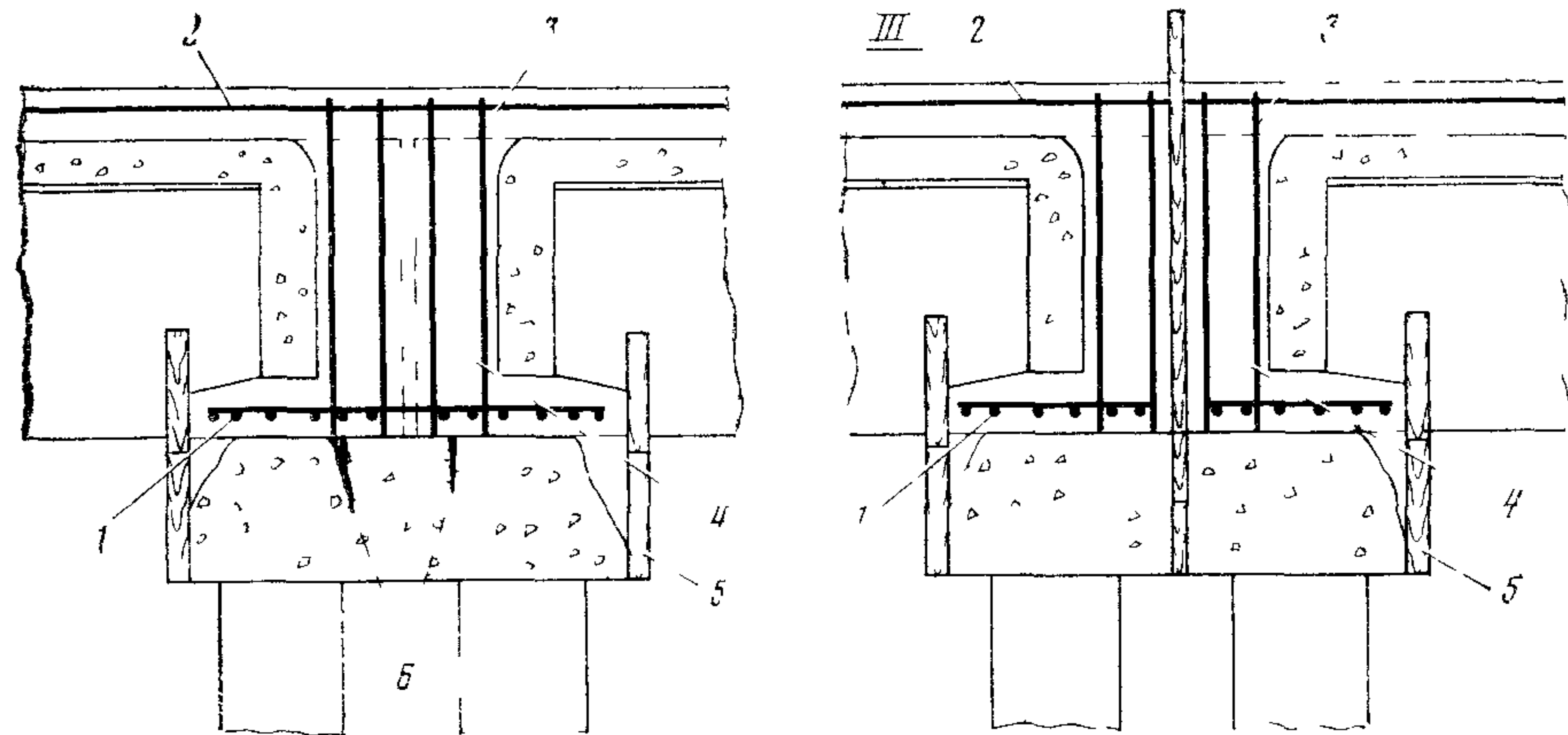
Рис. 6.5. Узлы II и III (см. рис. 6.3).
