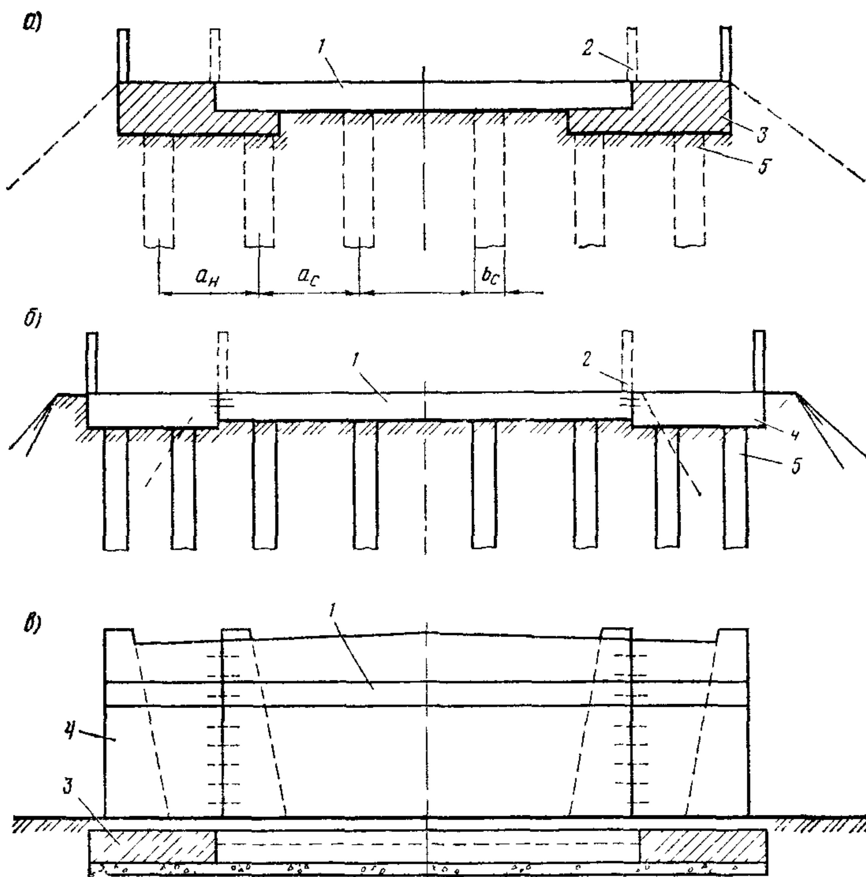
Рис. 3.20. Схемы уширения устоев
