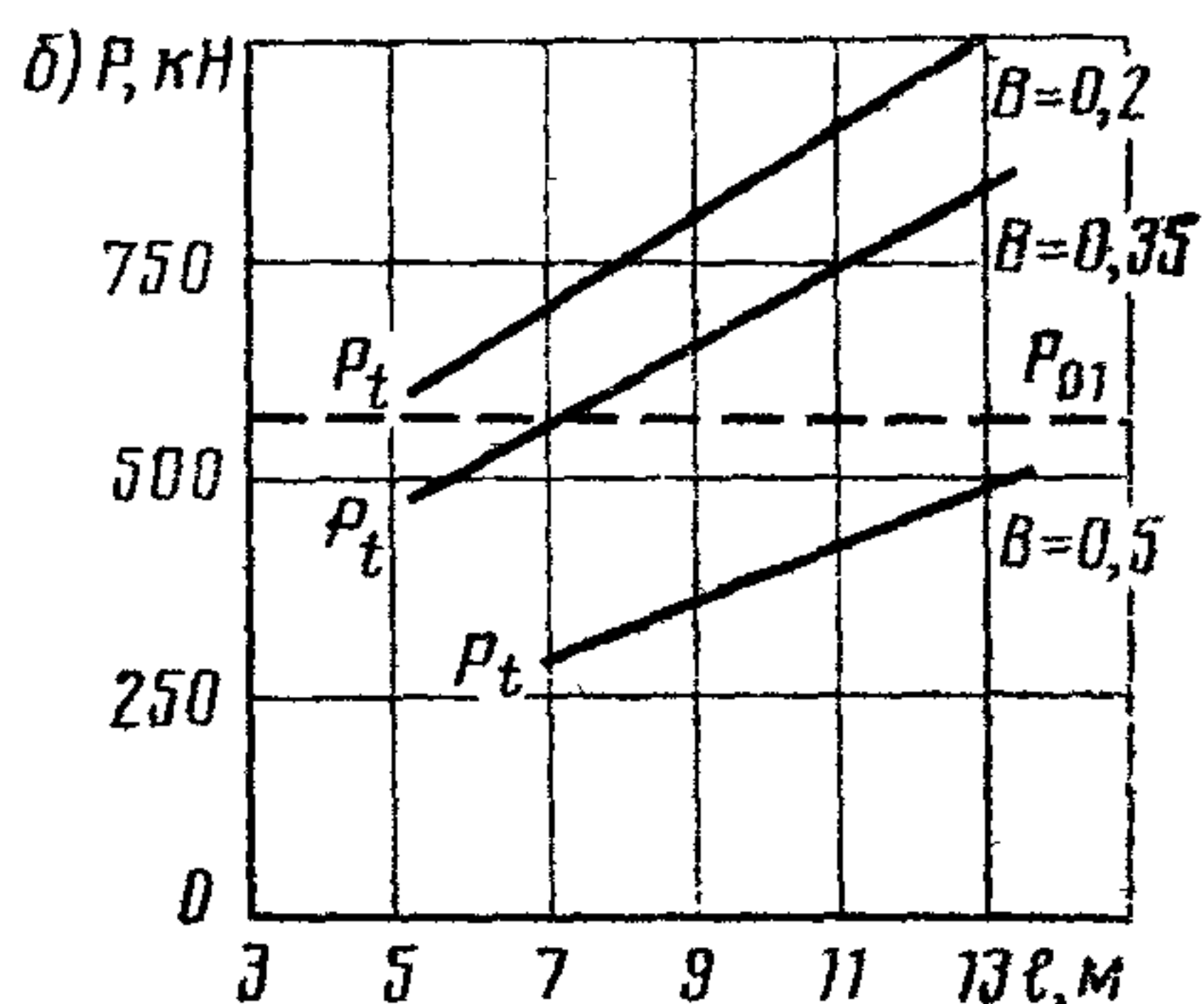
Рис. 2. Несущая способность железобетонных свай сечением 22 \times 22 см (а) и 35 \times 35 см (б) в суглинках с различными коэффициентами консистенции B
