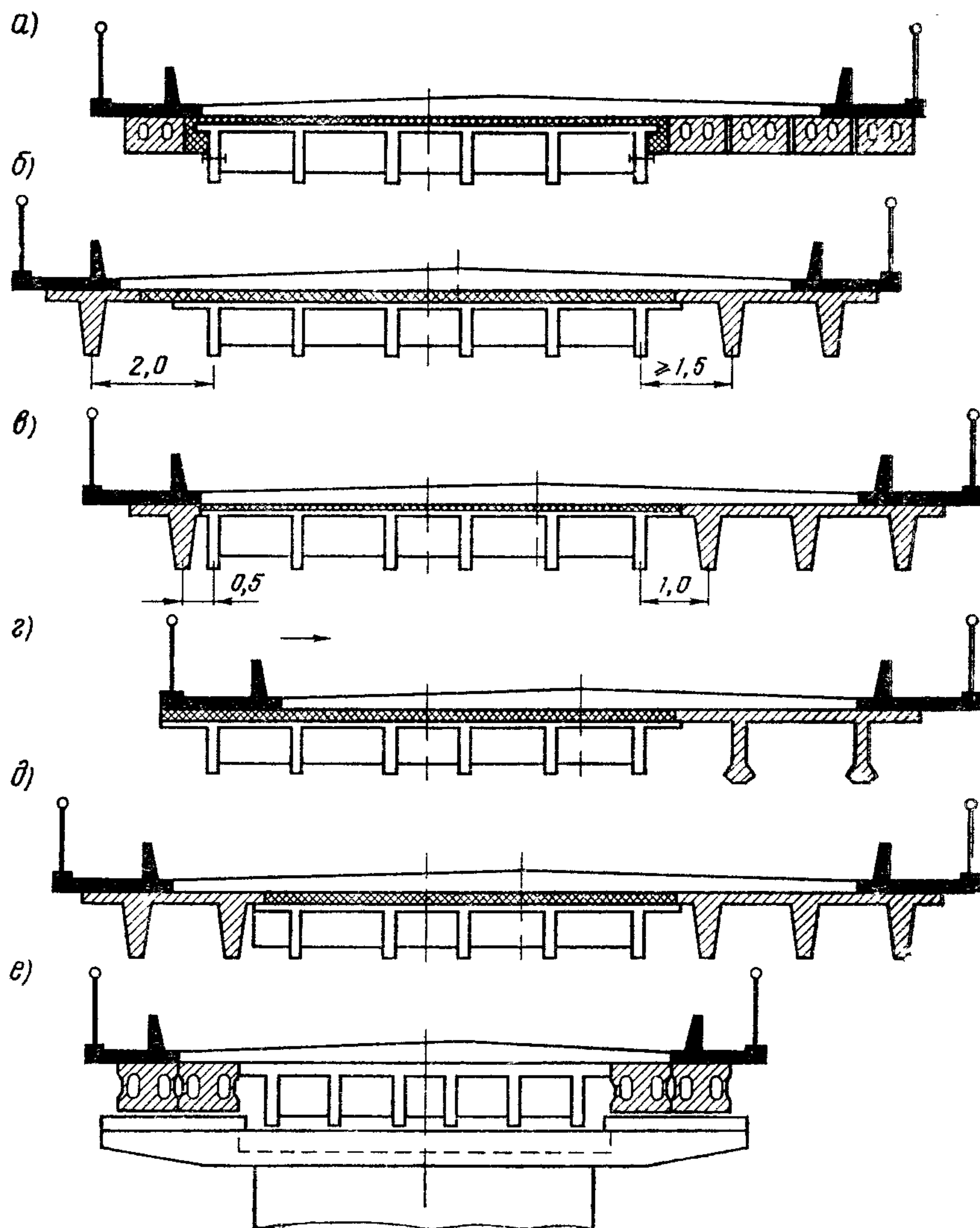
Рис. 3.7. Схемы комбинированных методов уширения сборных диафрагменных пролетных строений
