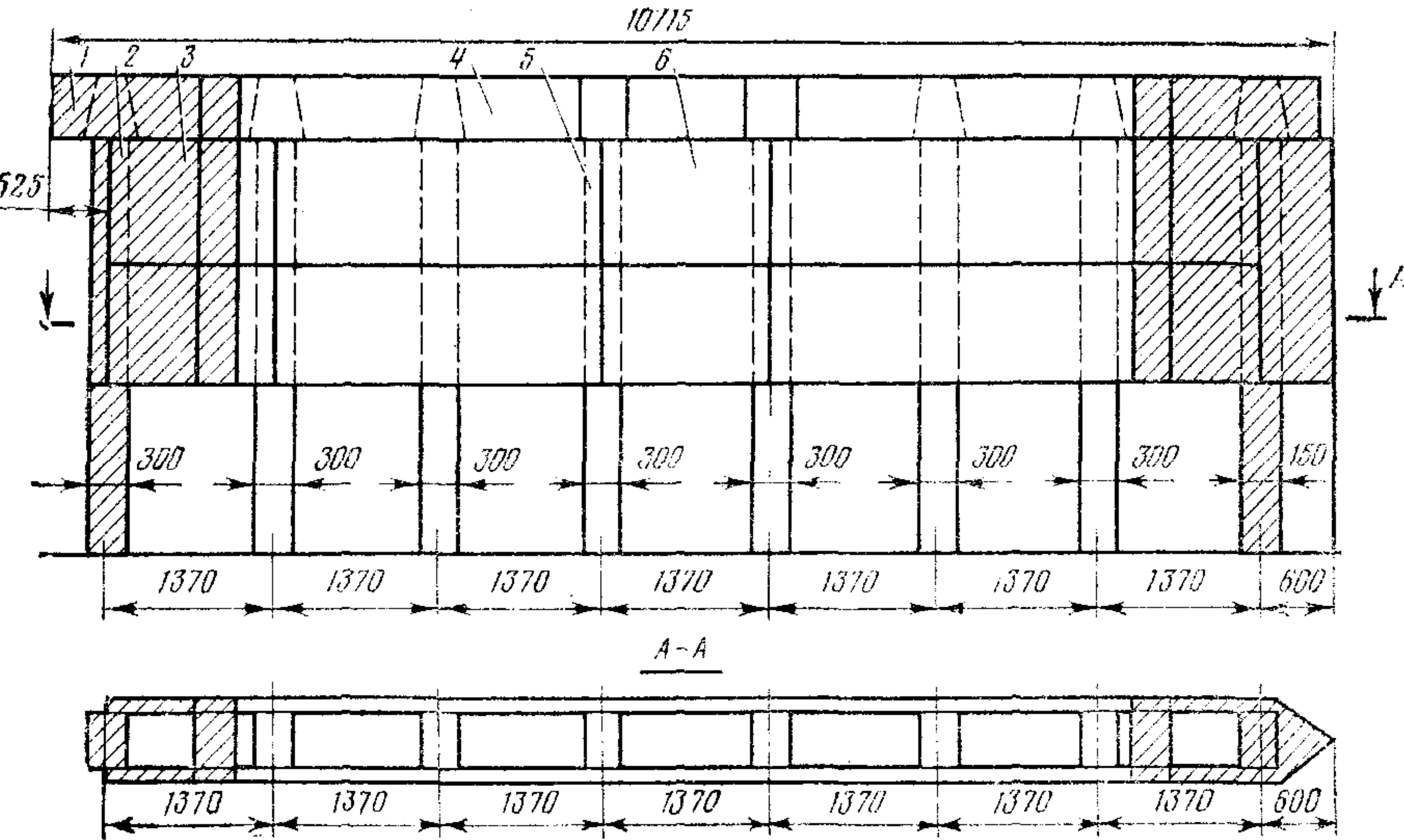
Рис. 6.10. Вид свайной опоры после уширения:
