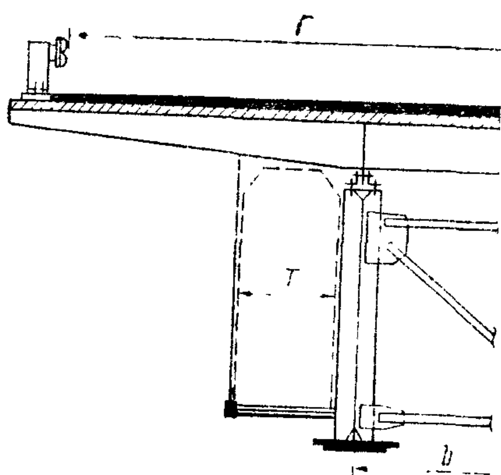
Рис. 3.13. Схема расположения тротуара в пониженном уровне
