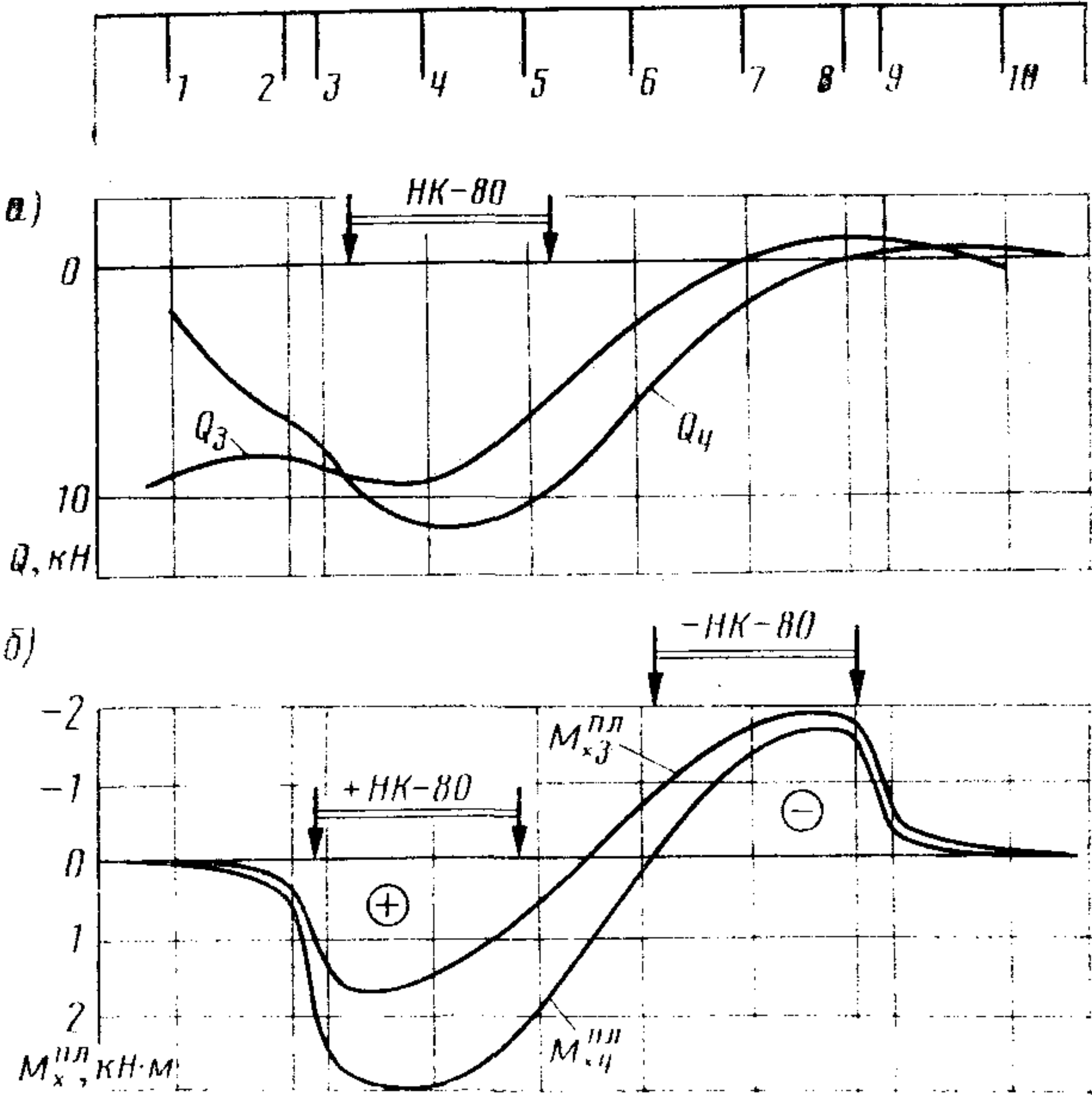
Рис. 8. Эпюры влияния поперечных сил в главных балках на опоре (а) и изгибающих моментов (б) в плите (в l/2 пролетного строения)
