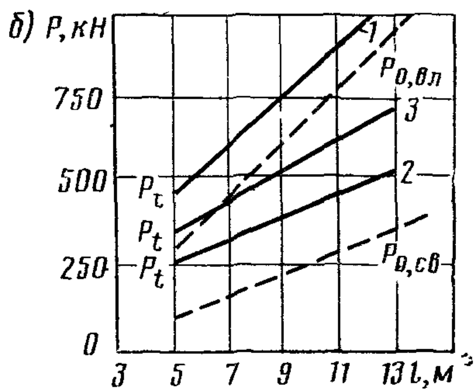
Рис. 9. Несущая способность деревянных свай d=28 см (а) и d=40 см (б) в песках влажных P_{0,вл} и средней влажности P_{0,св} : 1 — крупных; 2 — мелких; 3 — средней крупности
