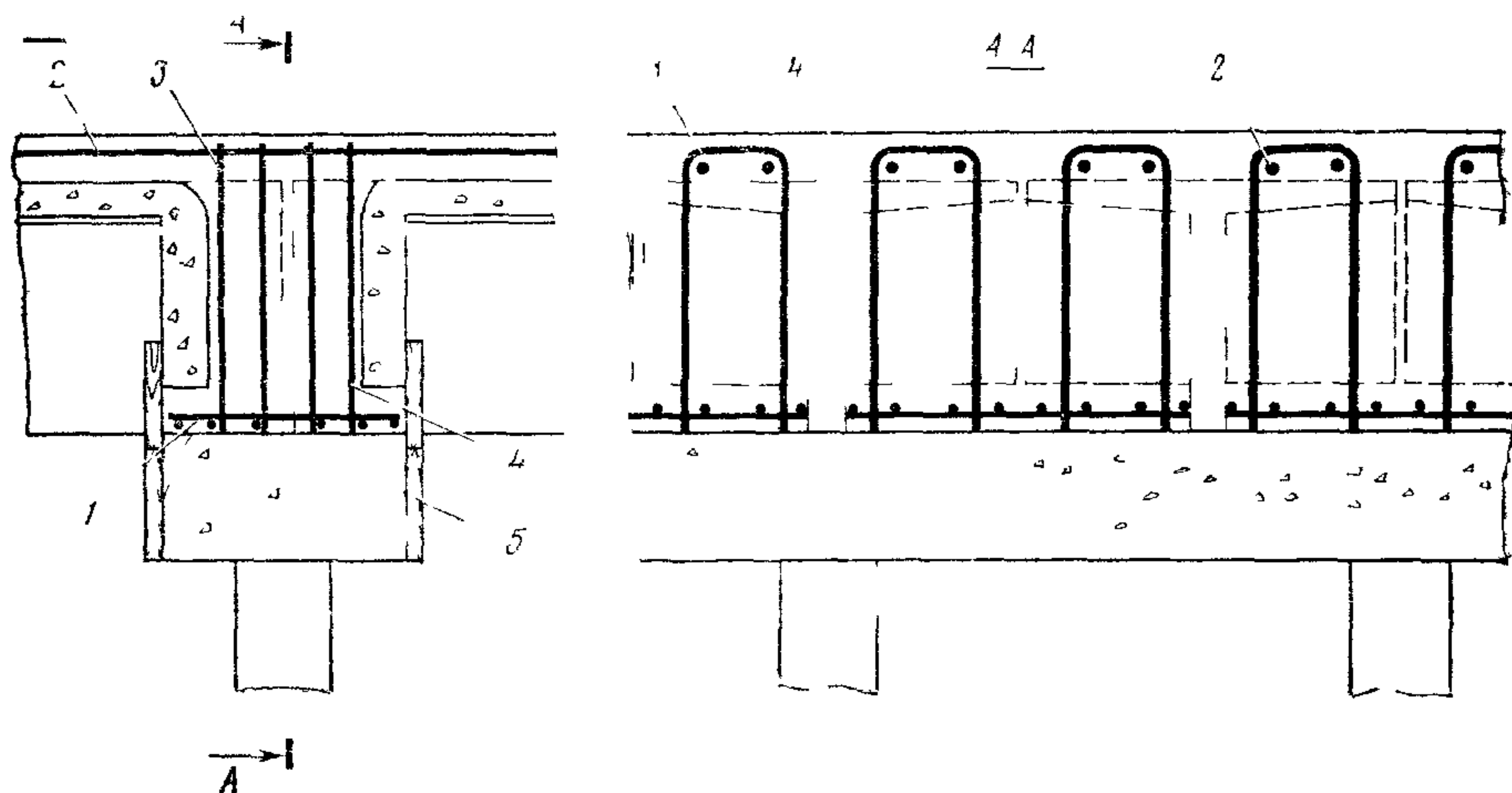
Рис. 64. Узел I (см рис 63)
