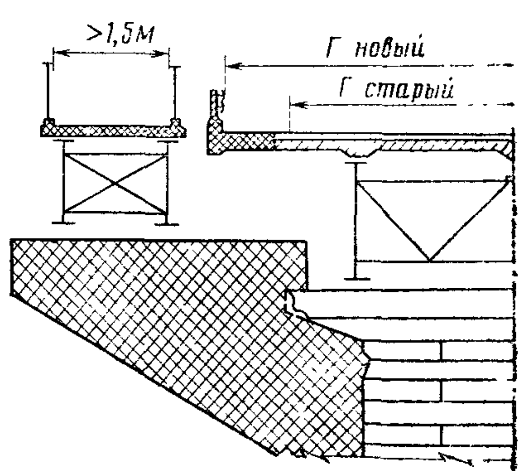
Рис. 3.14. Схема выноса пешеходного движения на отдельно стоящее пролетное строение
