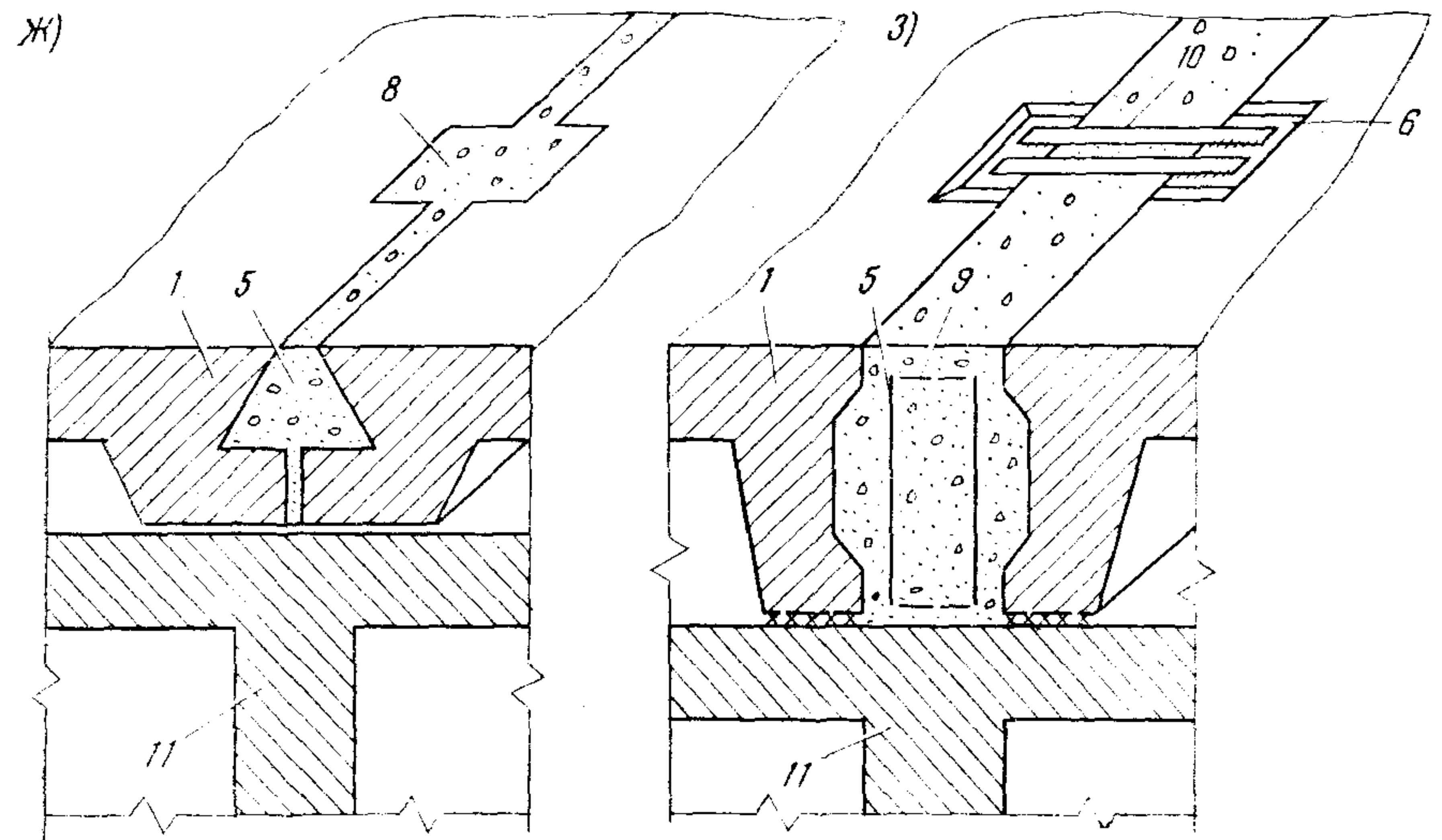
Рис. 4.6. Стыки сборных блоков накладной плиты:
