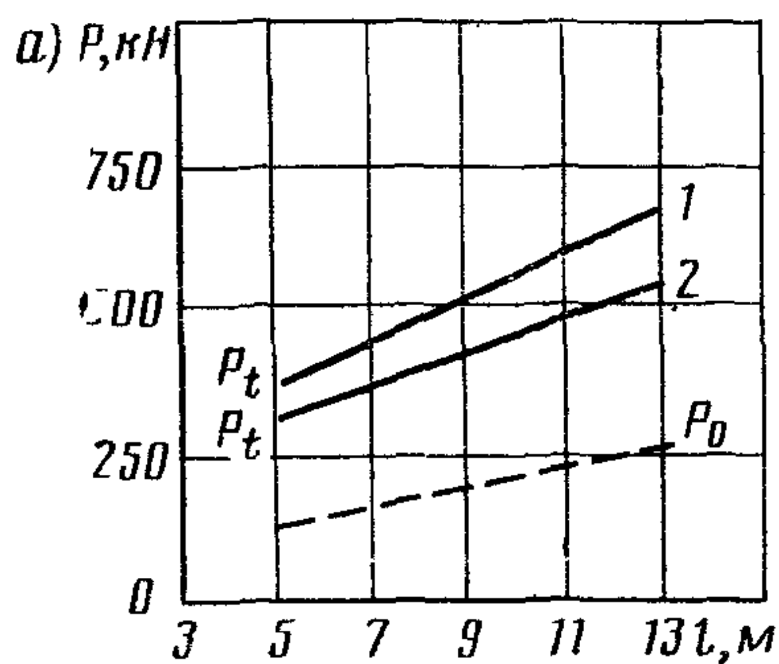
Рис. 9. Несущая способность деревянных свай d=28 см (а) и d=40 см (б) в песках влажных P_{0,вл} и средней влажности P_{0,св} : 1 — крупных; 2 — мелких; 3 — средней крупности
