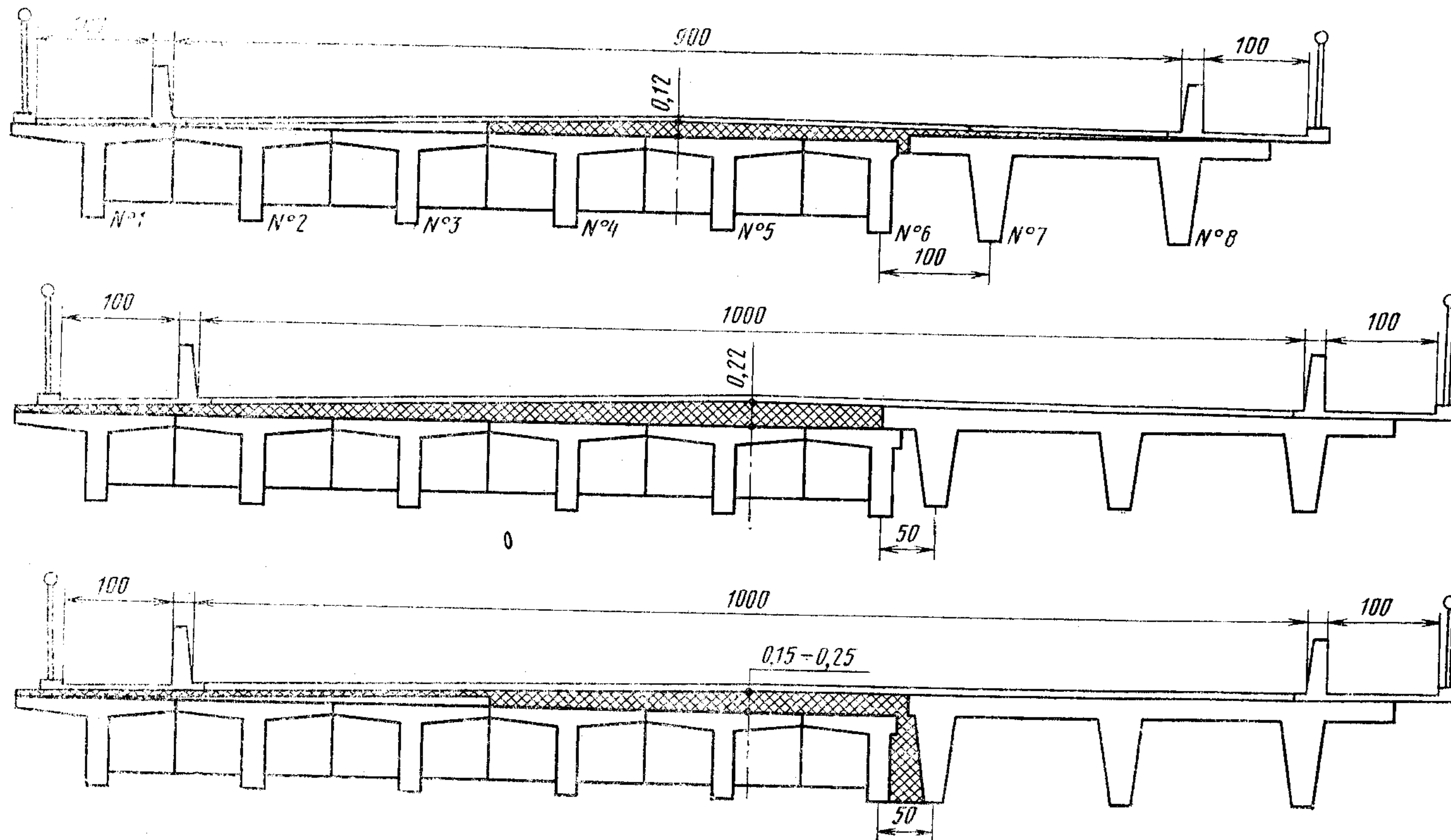
Рис. 6.9. Уширение пролетных строений из балок по типовому проекту 56 с помощью приставляемых с одной стороны балок со смещением тротуарных блоков
