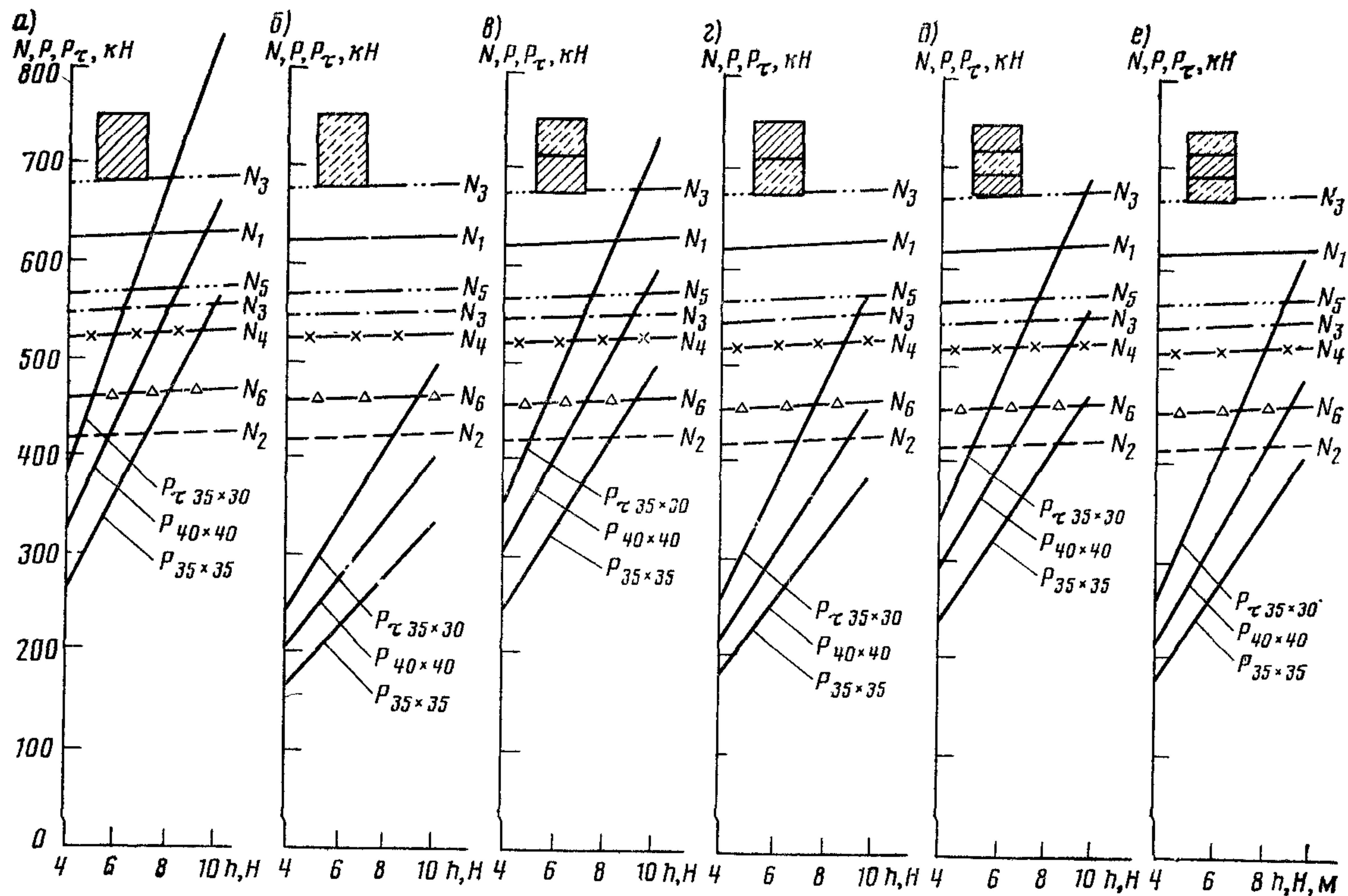
Рис. 3. Расчетные усилия N_i , приходящиеся на голову свай при различном их погружении под промежуточной опорой моста с длиной пролетных стрел 11,36 м
