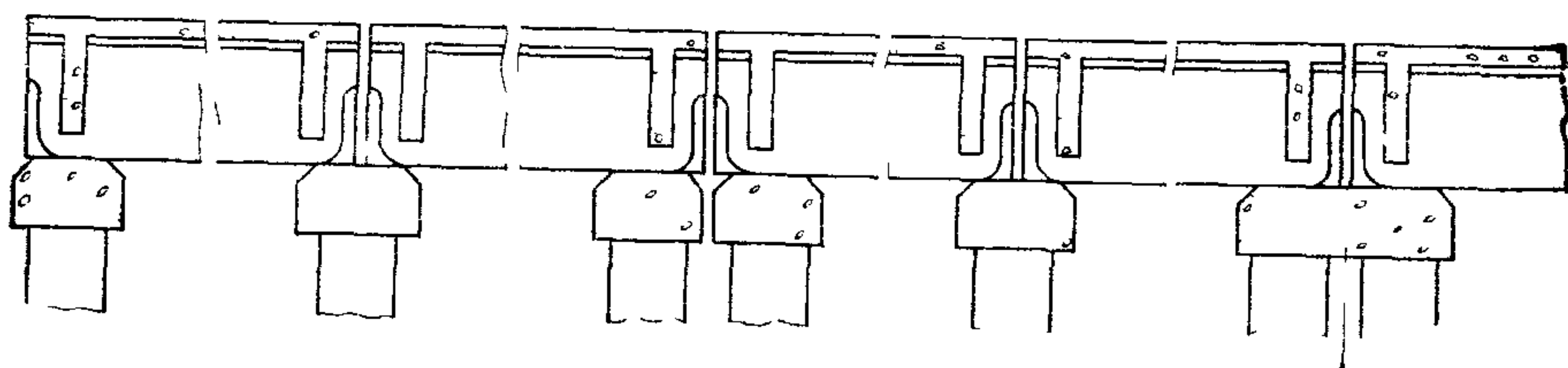
Рис 62 Исходная схема секционного моста с возможными дефектами в виде сколов торцов балок
