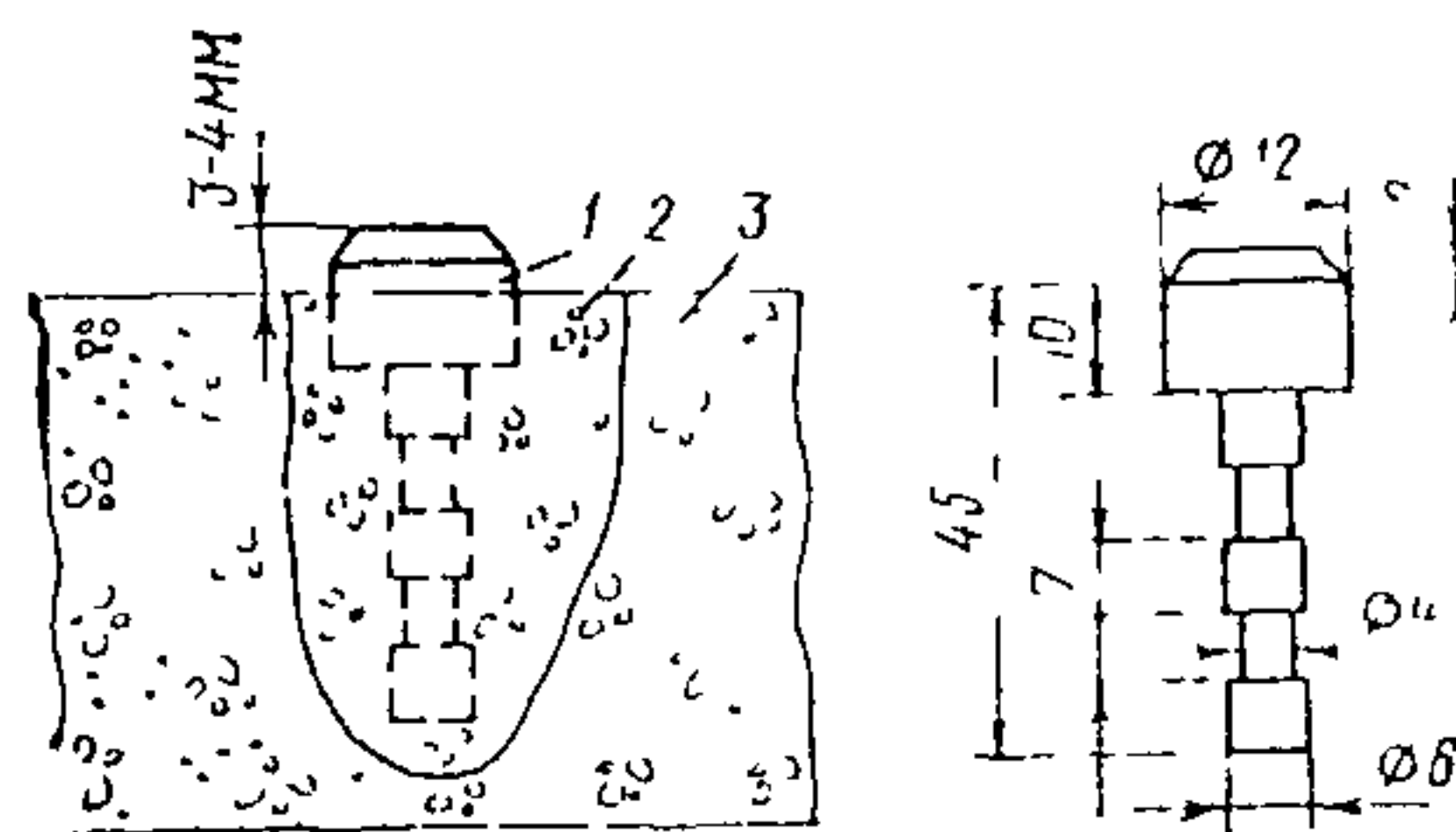
Рис. 12.2 Марка и ее закрепление в бетоне конструкции
