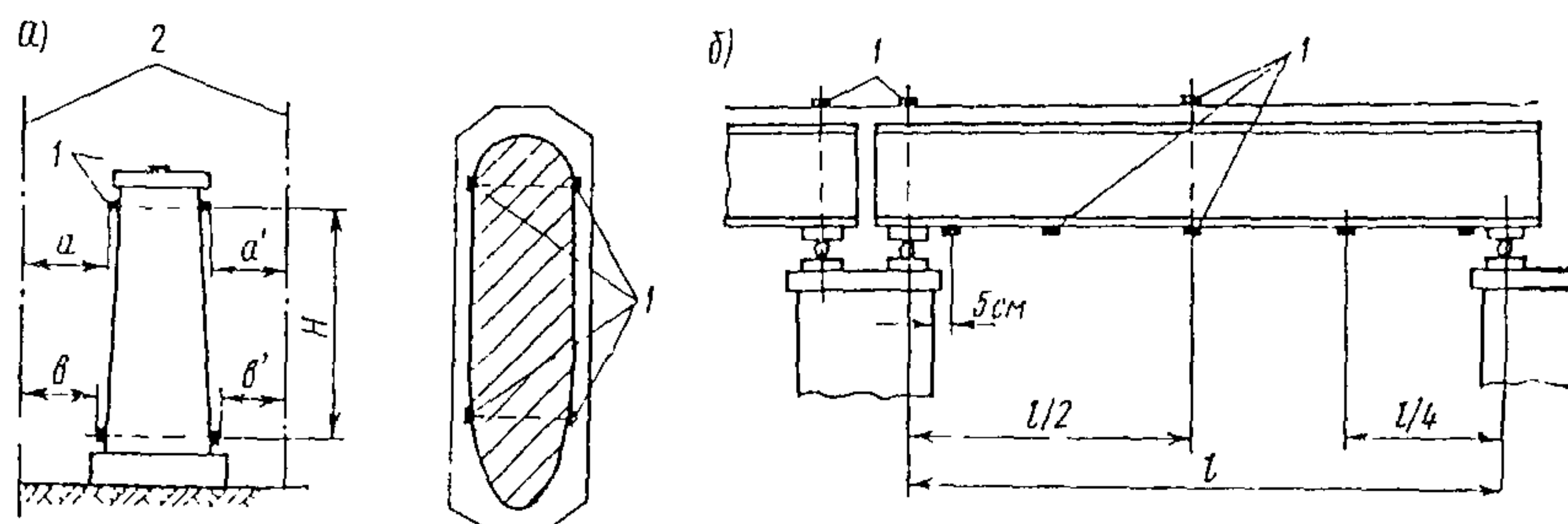
Рис. 12.1. Схема расположения закрепленных точек:
