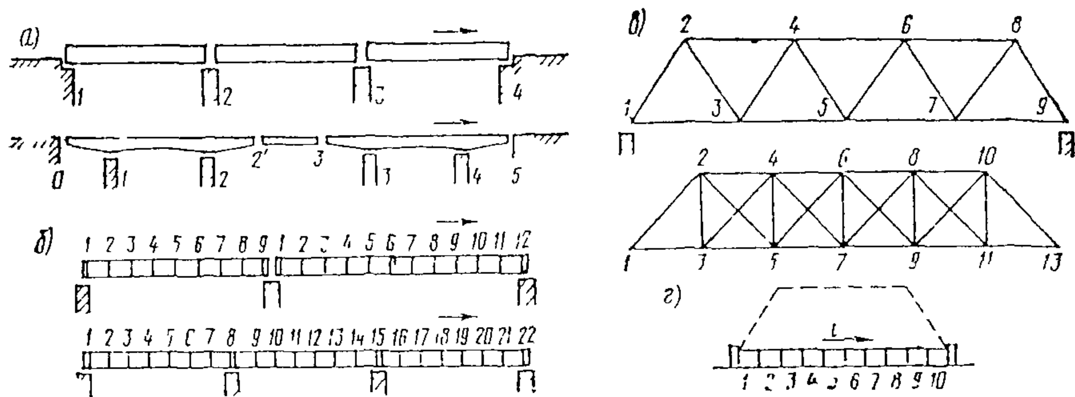
Рис 1.1 Схема обозначения элементов искусственного сооружения а — опор пролетных строений, б — диафрагм и панелей, в — элементов сквозных ферм; г — звеньев труб. Стрелкой показано направление хода километража для мостов
