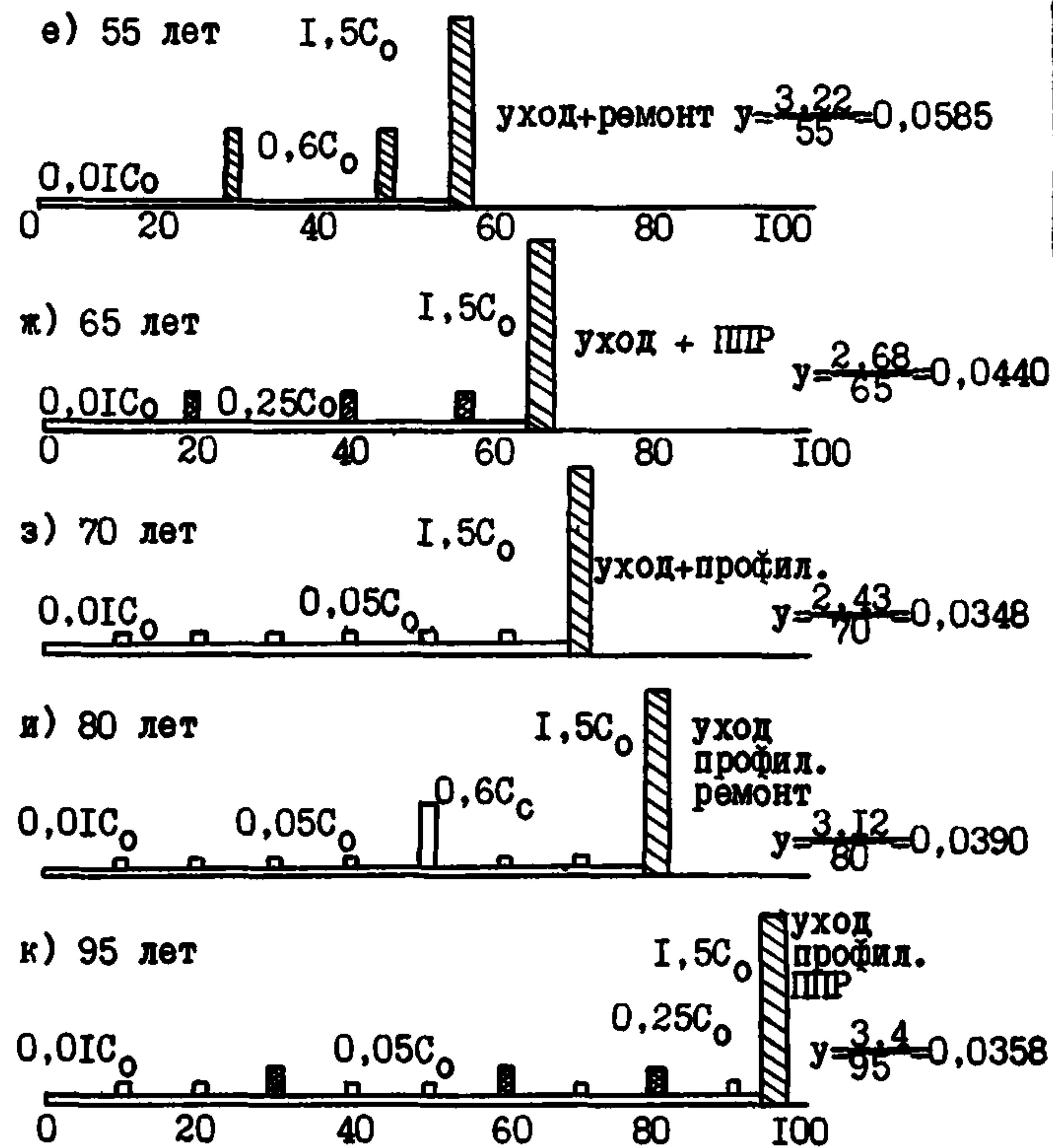
Рис. I. Возможные схемы эксплуатации моста (учитывается лишь физический износ)
