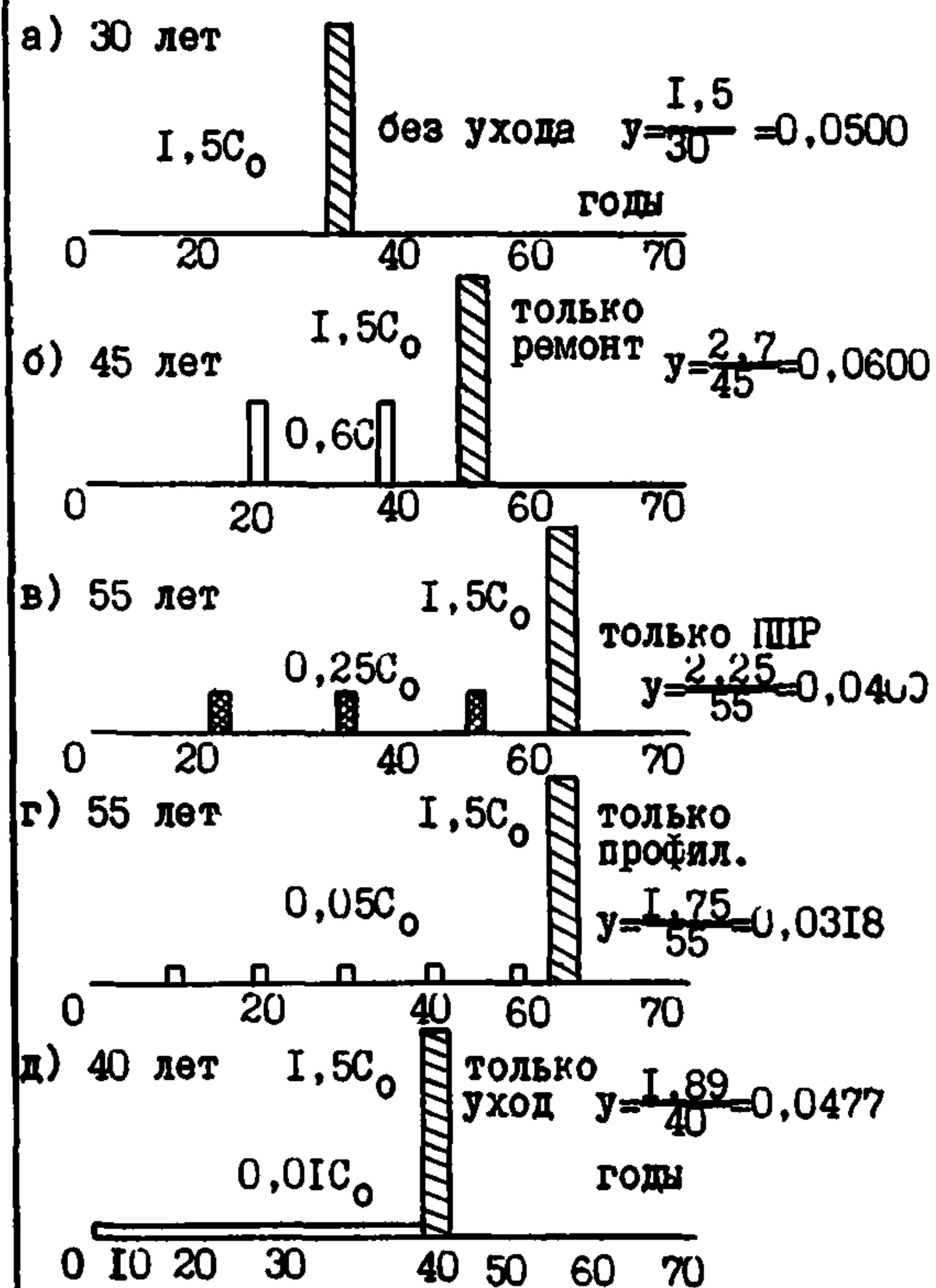
Рис. I. Возможные схемы эксплуатации моста (учитывается лишь физический износ)
