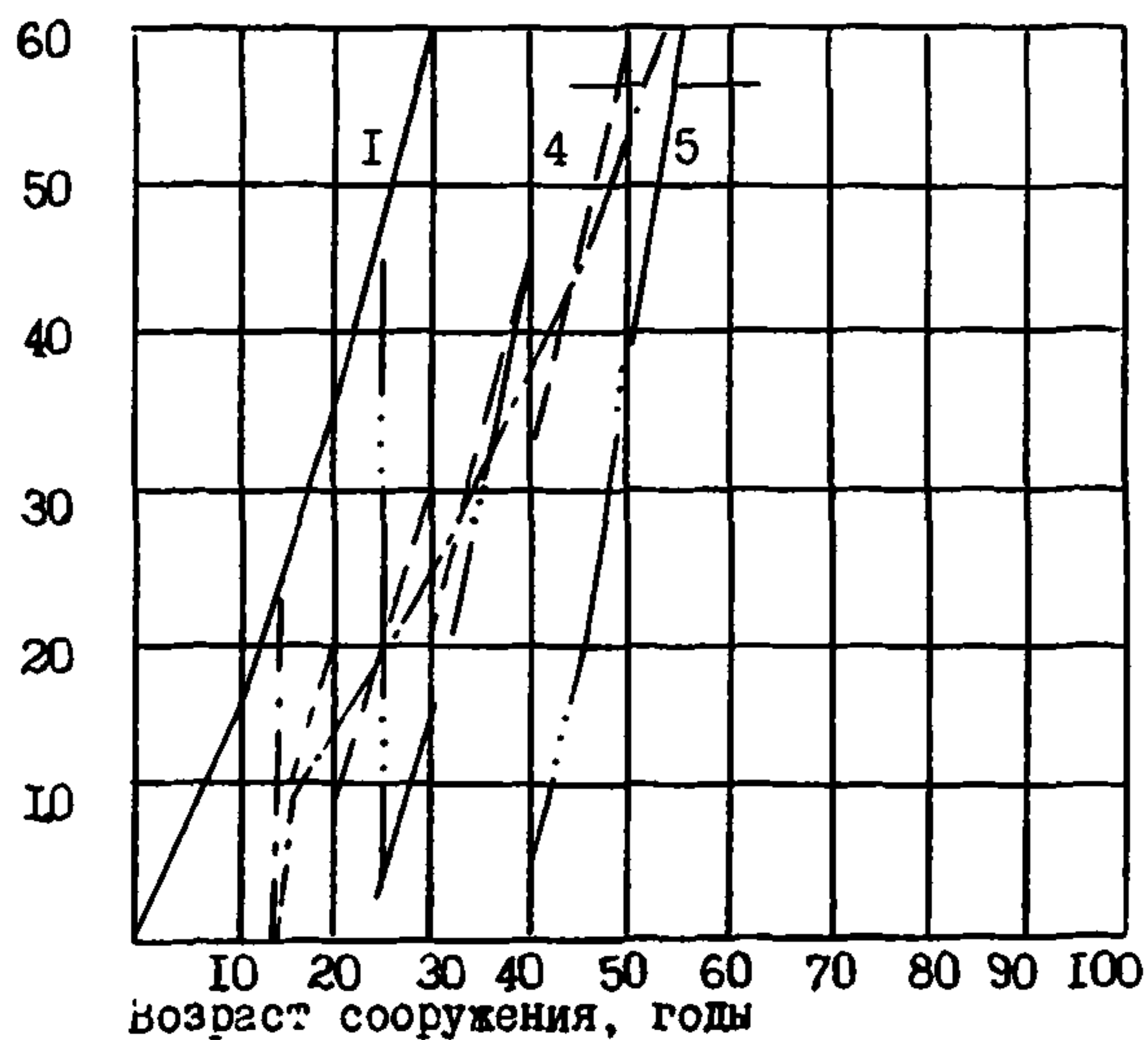
Рис. 2. Графики долговечности моста с ж/б пролетными строениями:
