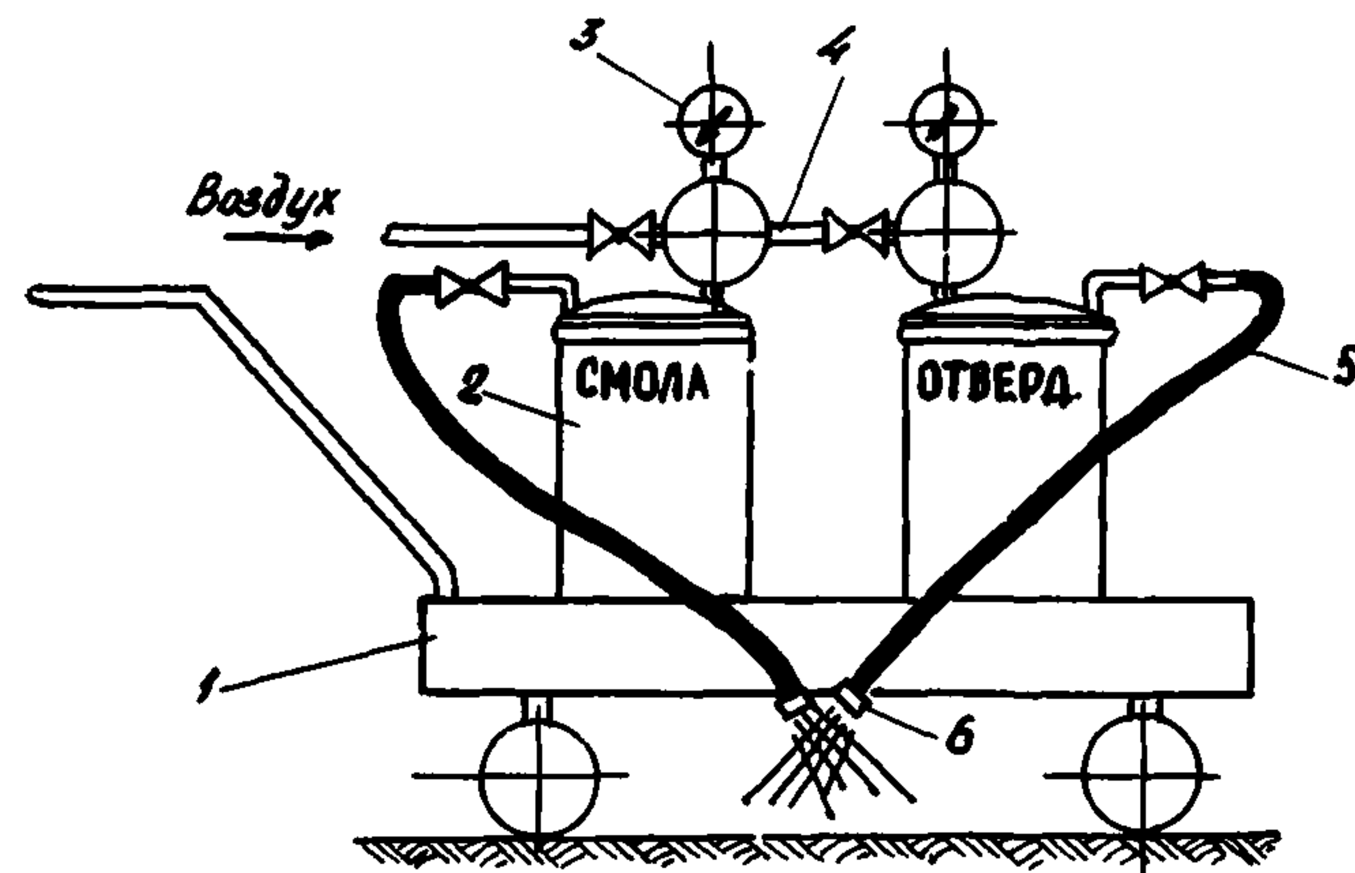
Рис.2. Схема распределителя материалов РД-601
