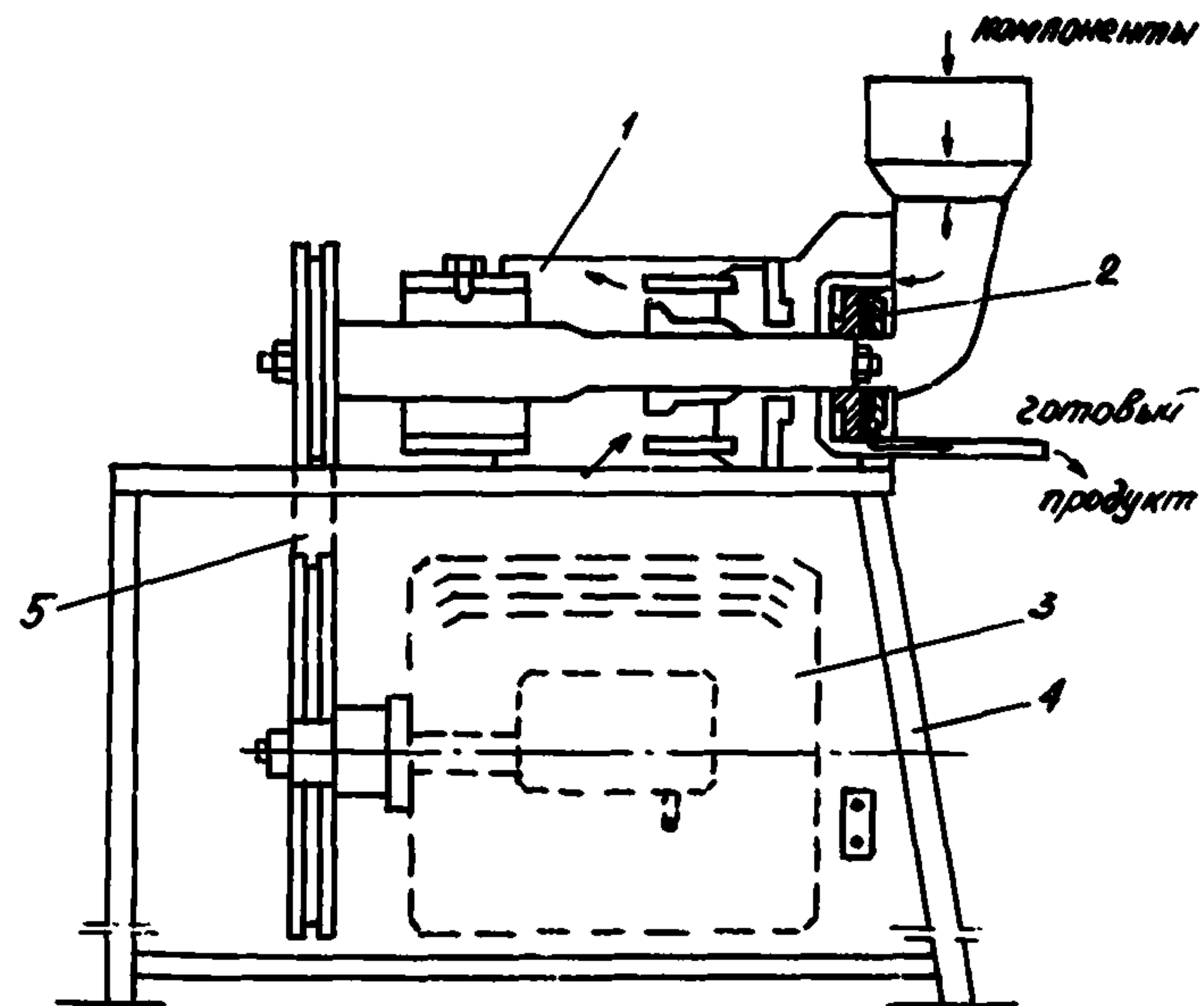
Рис.2. Схема распределителя материалов РД-601
