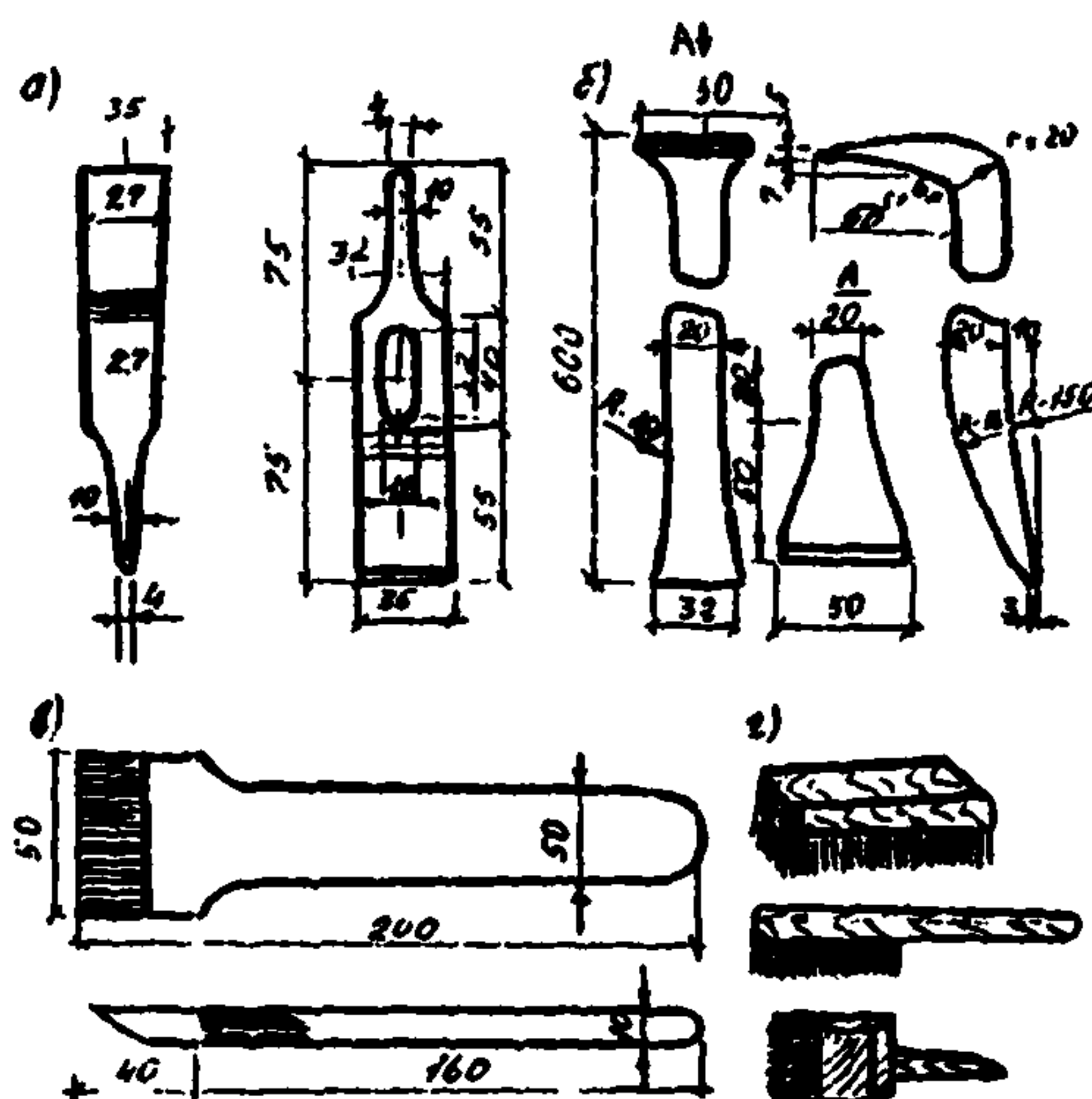
Рис. 1. Ручной инструмент для очистки: а - молоток для удаления ржавчины и окалины; б - зубило для удаления окалины; в - стальной скребок для снятия пластовой ржавчины; г - щетка из стальной проволоки для удаления плохо держащихся красок, рыхлой ржавчины и т.п.
