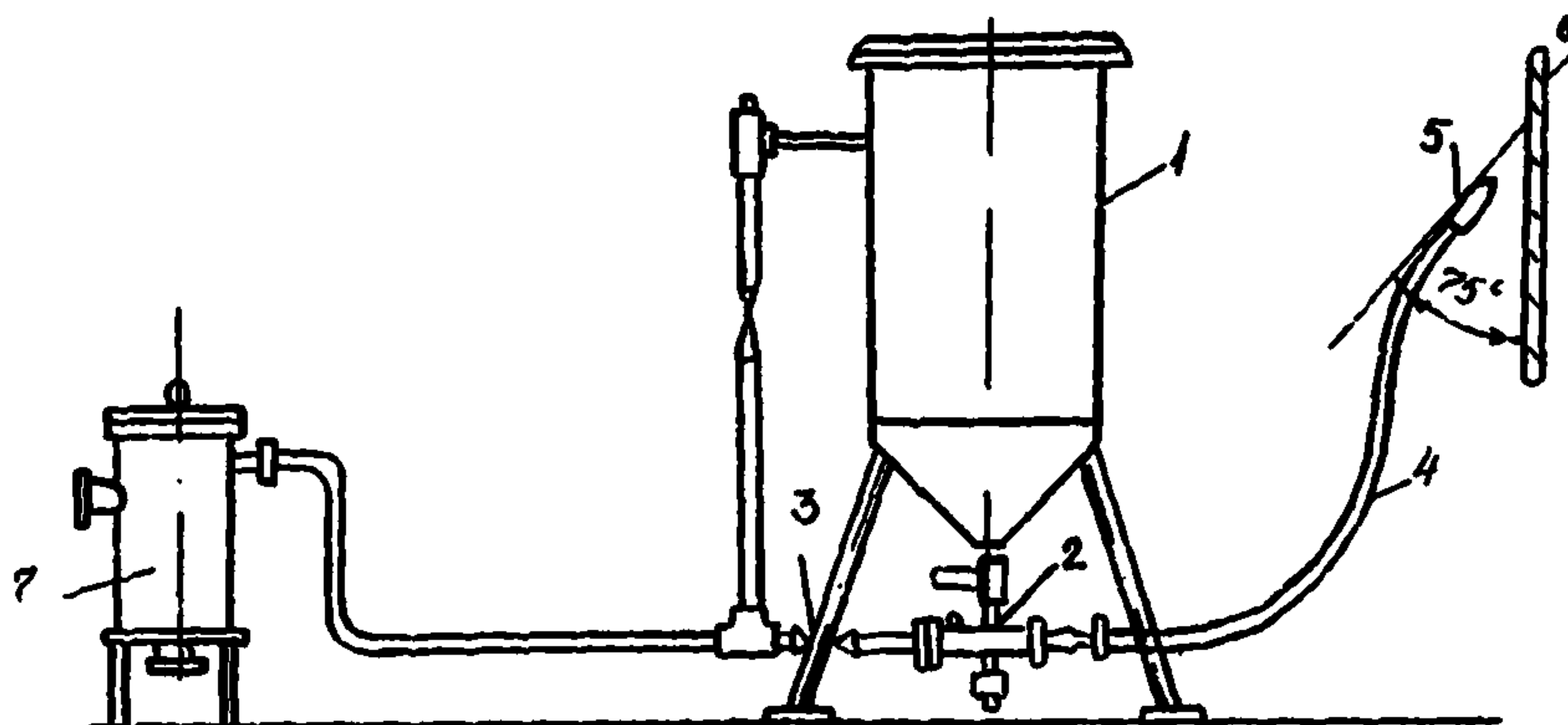
Рис. 2. Схема установки пескоструйного аппарата 1 - корпус аппарата; 2 - камера смешения сжатого воздуха и песка; 3 - вентиль коммуникации сжатого воздуха; 4 - резиновый шланг подачи песка в сопло; 5 - сопло; 6 - очищаемая поверхность; 7 - масловодоотделитель.
