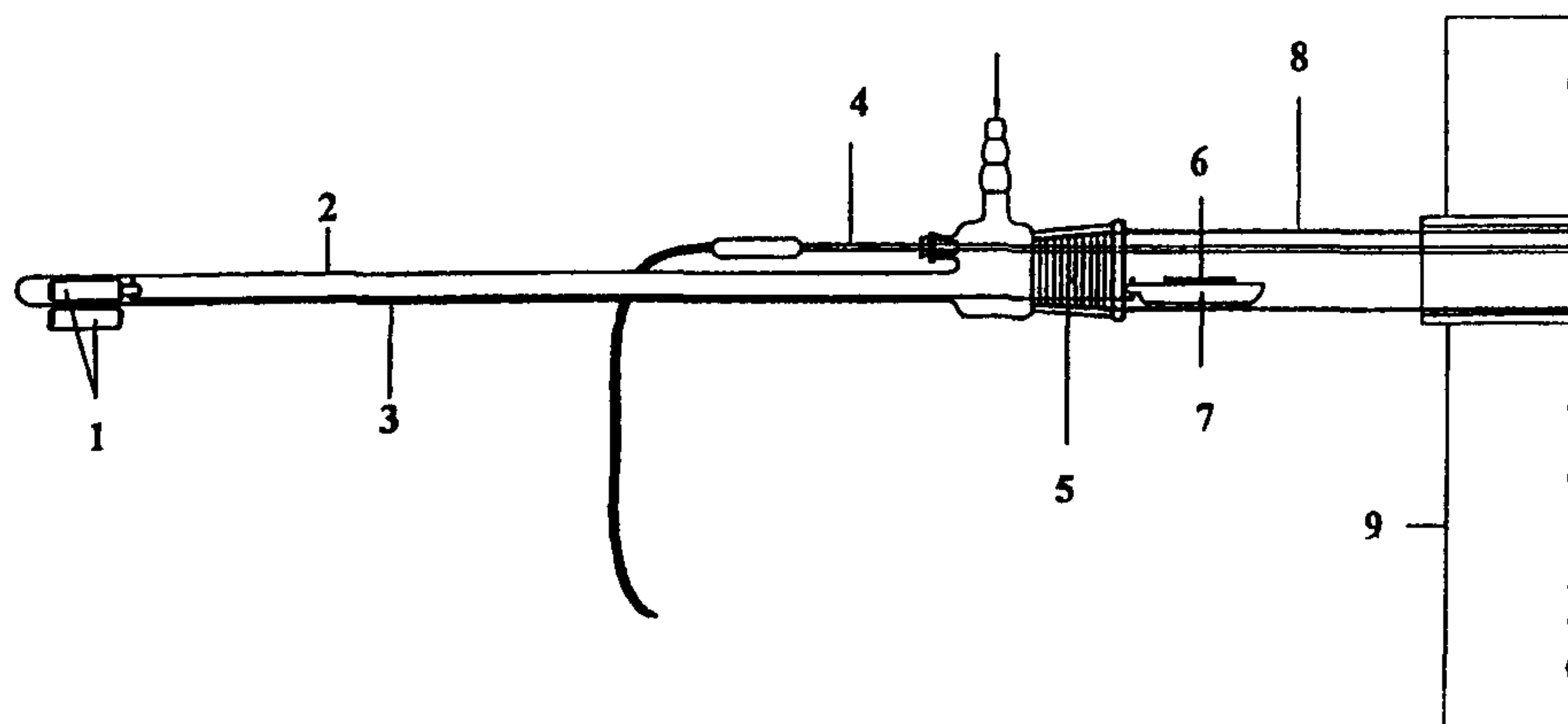
Рисунок 1 — Устройство для введения лодочки в зону нагрева трубчатой печи
