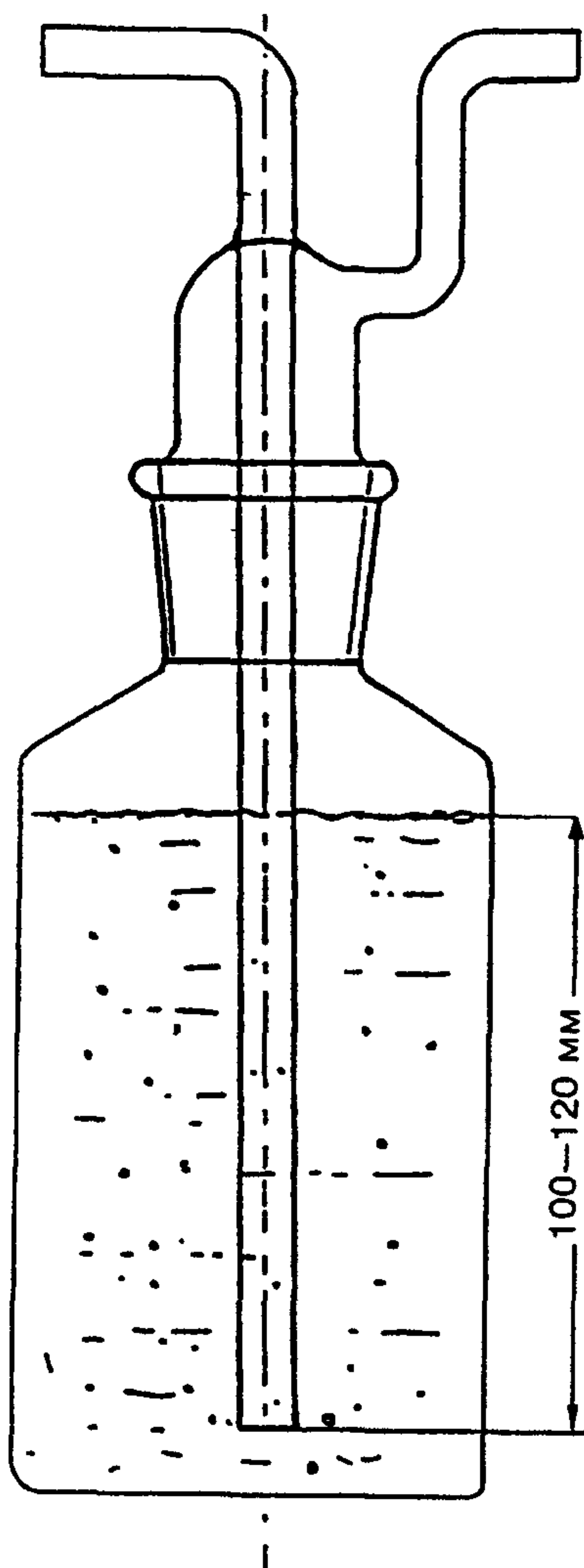
Рисунок 2 — Сосуд-смеситель
