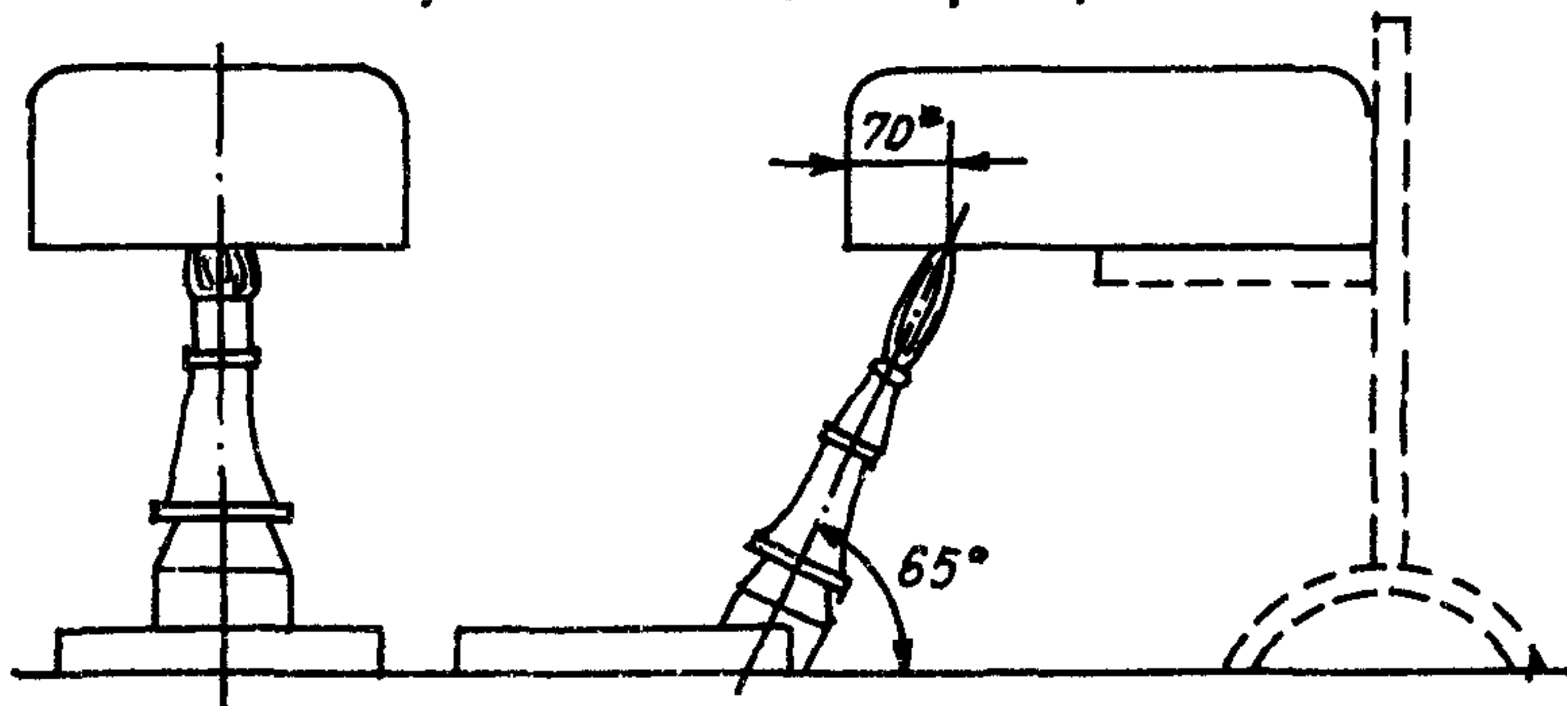
Рис. 2. Расположение горелки при горизонтальном расположении образца
