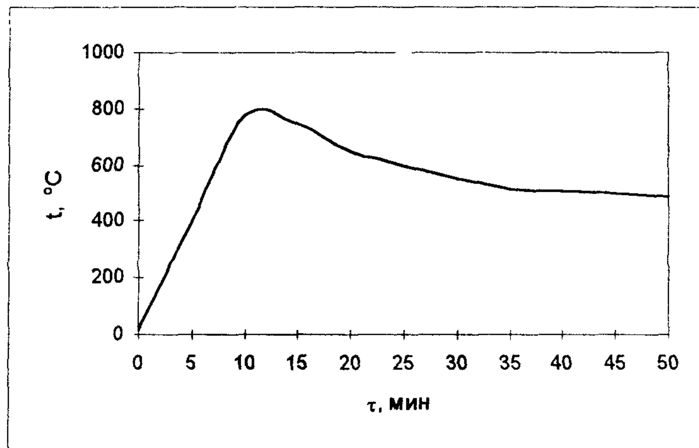
График реального температурного режима пожара
