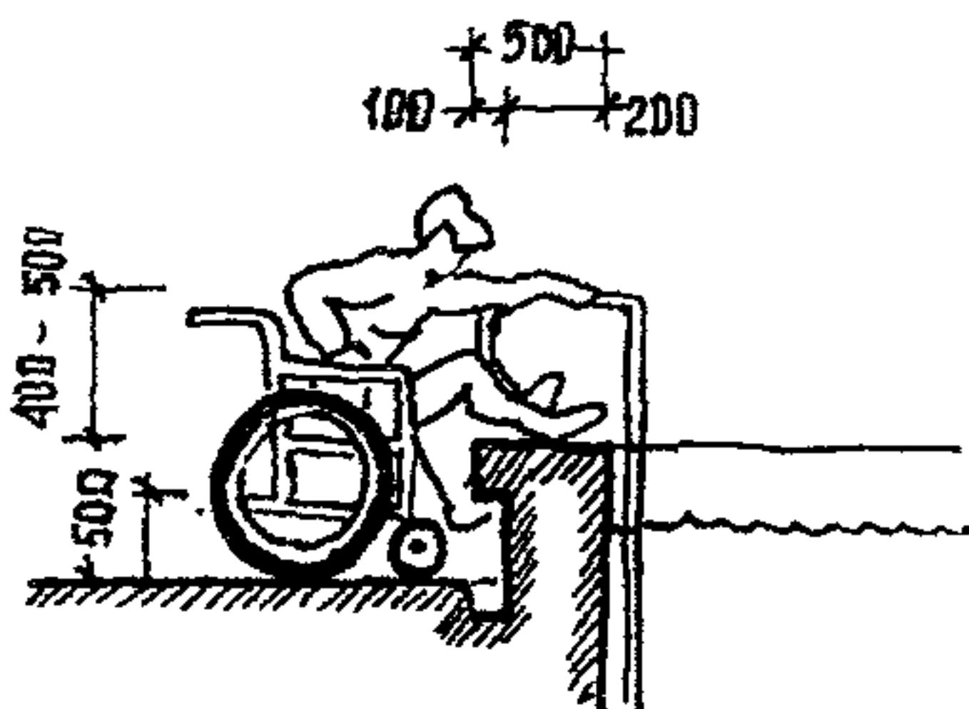
2а - без пандуса
