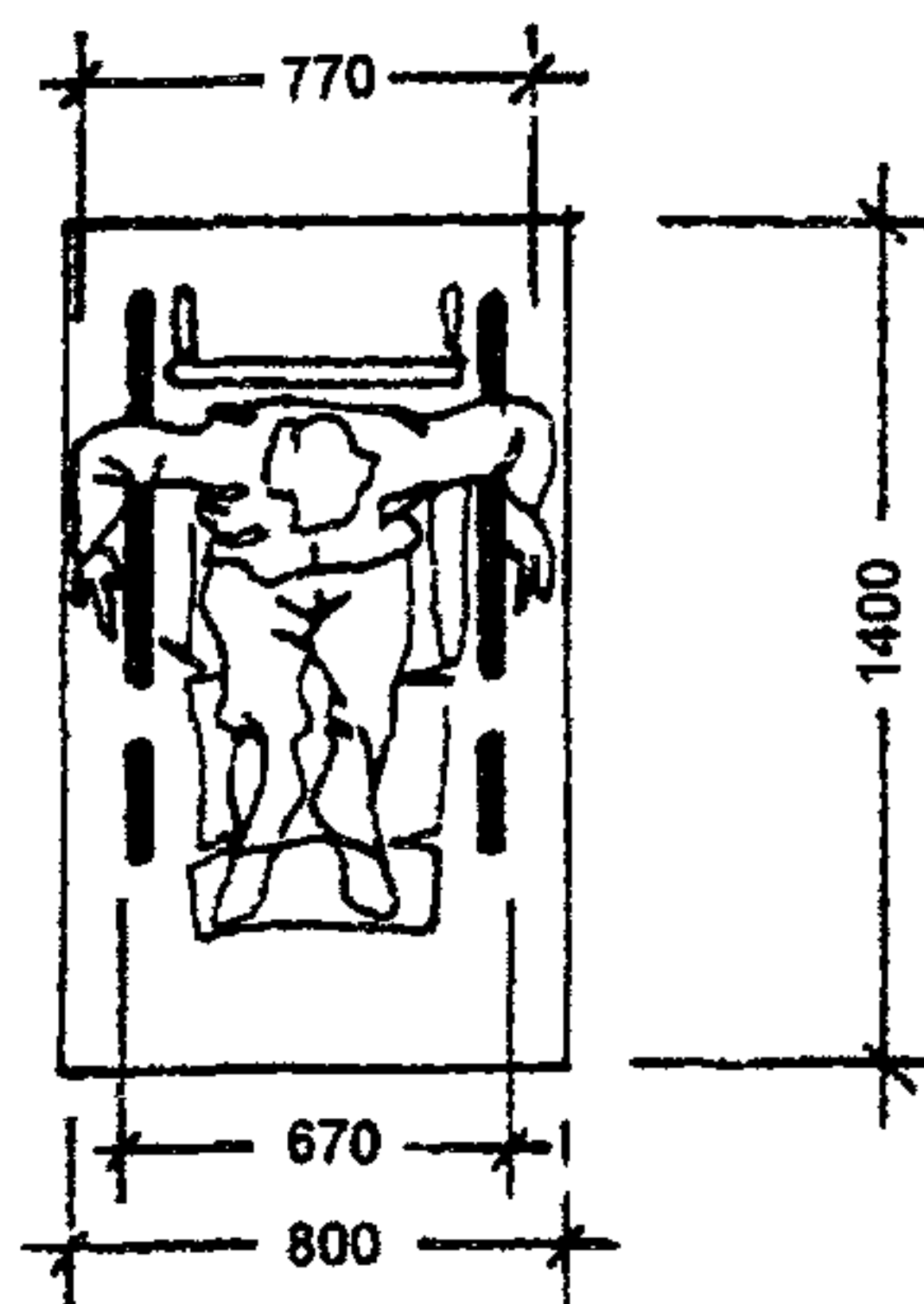
РИС 35 ГАБАРИТЫ КОЛЯСОК, ПРИМЕНЯЕМЫХ ДЛЯ ПЕРЕДВИЖЕНИЯ ИНВАЛИДОВ-ОПОРНИКОВ
