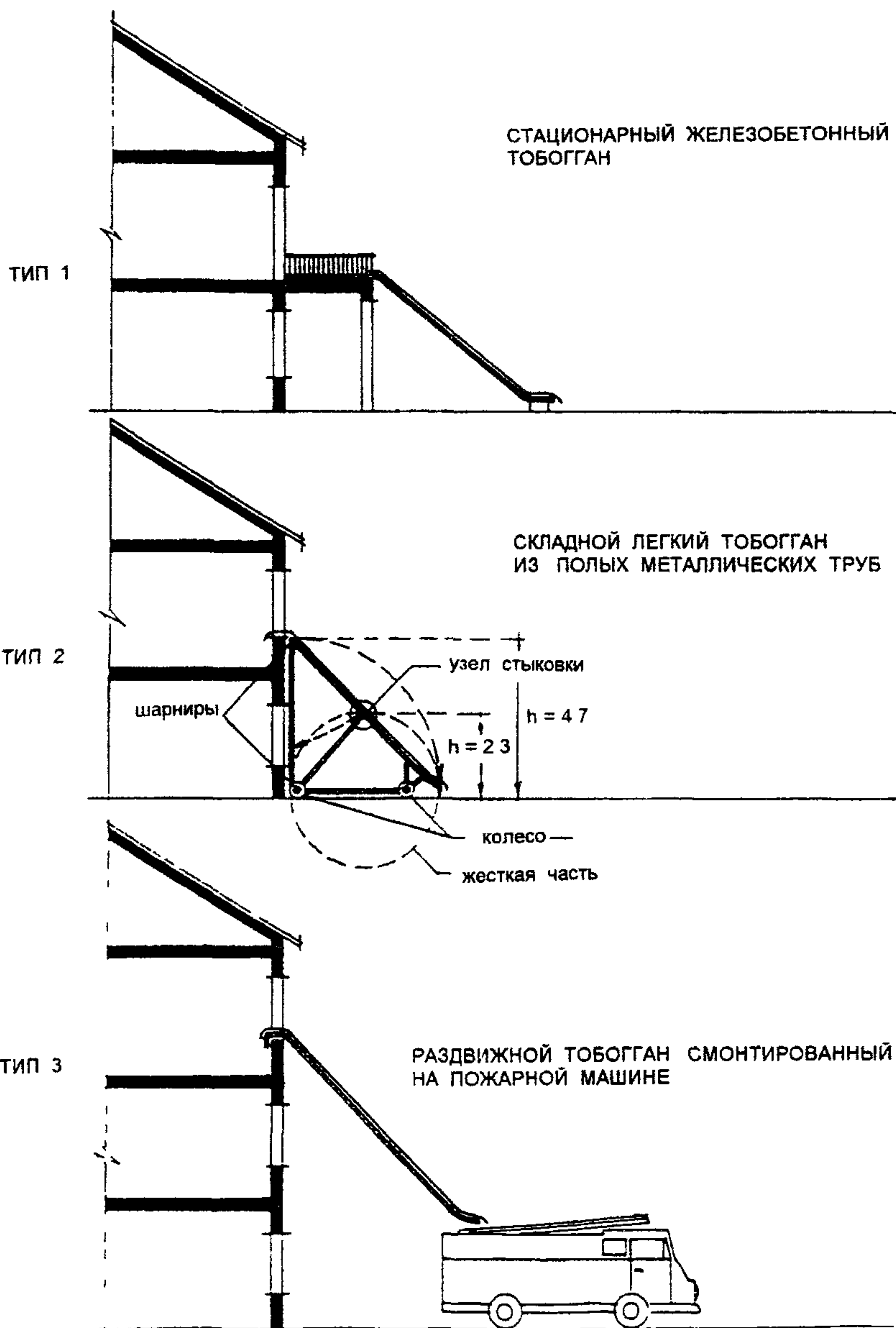
РИС 3 10 СХЕМЫ ТОБОГГАНОВ
