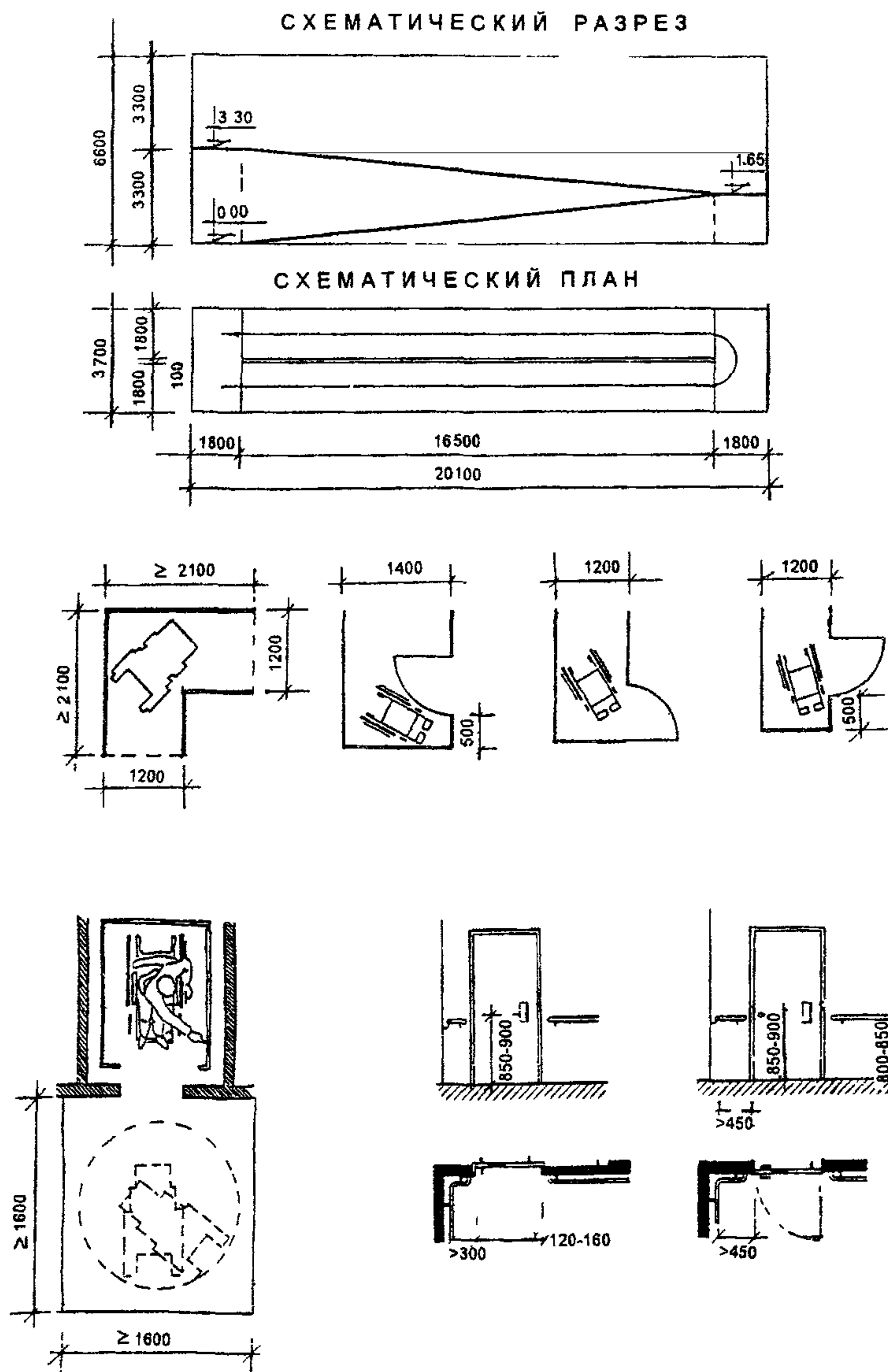
РИС 3 6 ГАБАРИТНЫЕ СХЕМЫ ПАНДУСОВ, ПОВОРОТОВ В КОРИДОРАХ, ОТКРЫВАНИЯ ДВЕРЕЙ, ЛИФТОВЫХ ПЛОЩАДОК, ЛИФТОВЫХ ДВЕРЕЙ
