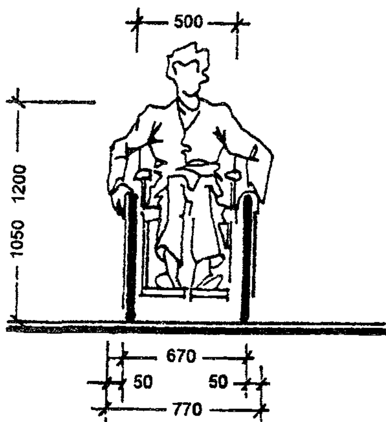
РИС 35 ГАБАРИТЫ КОЛЯСОК, ПРИМЕНЯЕМЫХ ДЛЯ ПЕРЕДВИЖЕНИЯ ИНВАЛИДОВ-ОПОРНИКОВ
