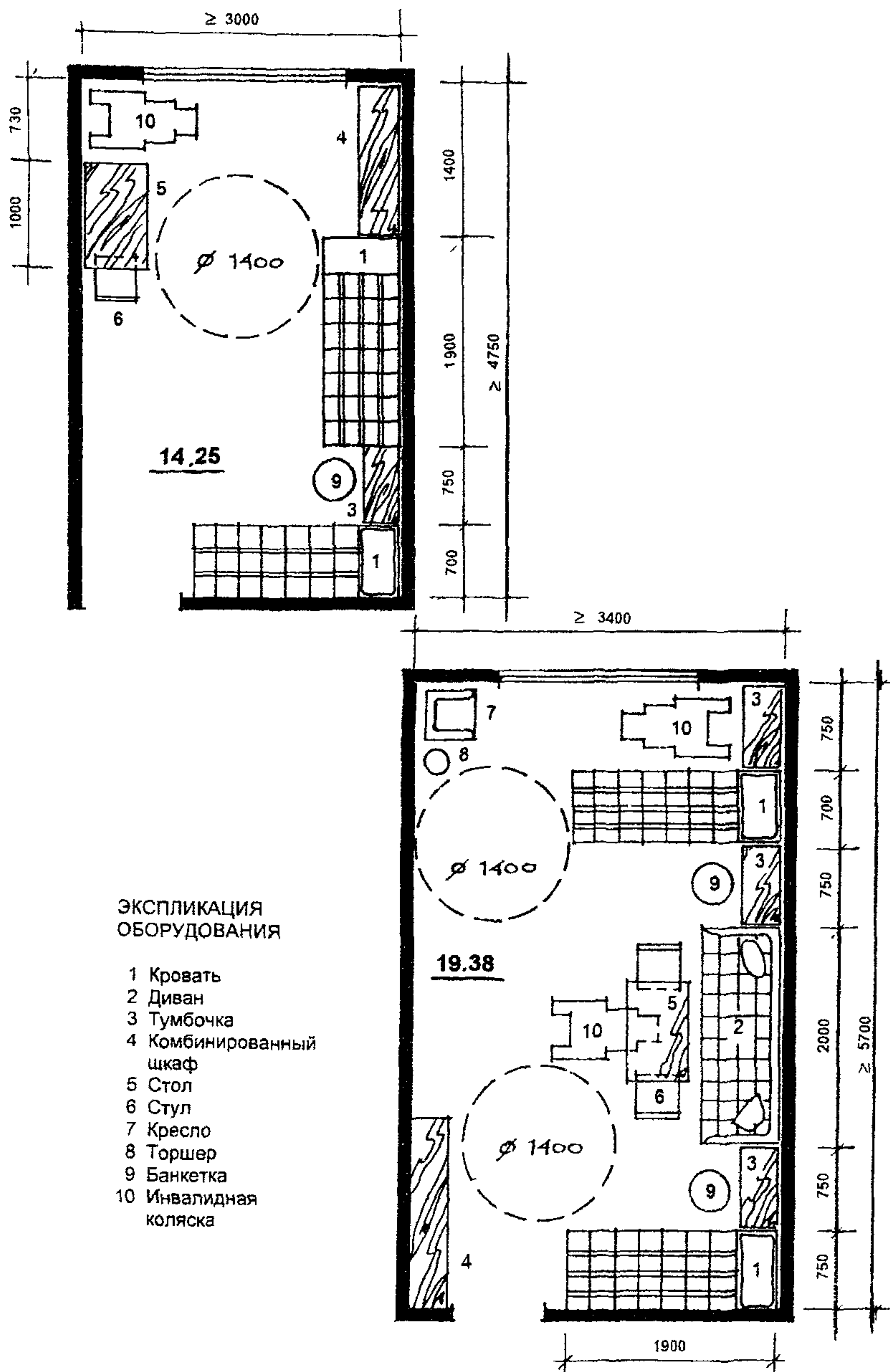
РИС 4 2 ПЛАНИРОВОЧНЫЕ СХЕМЫ СПАЛЬНЫХ КОМНАТ НА 2 И 3 МЕСТА
