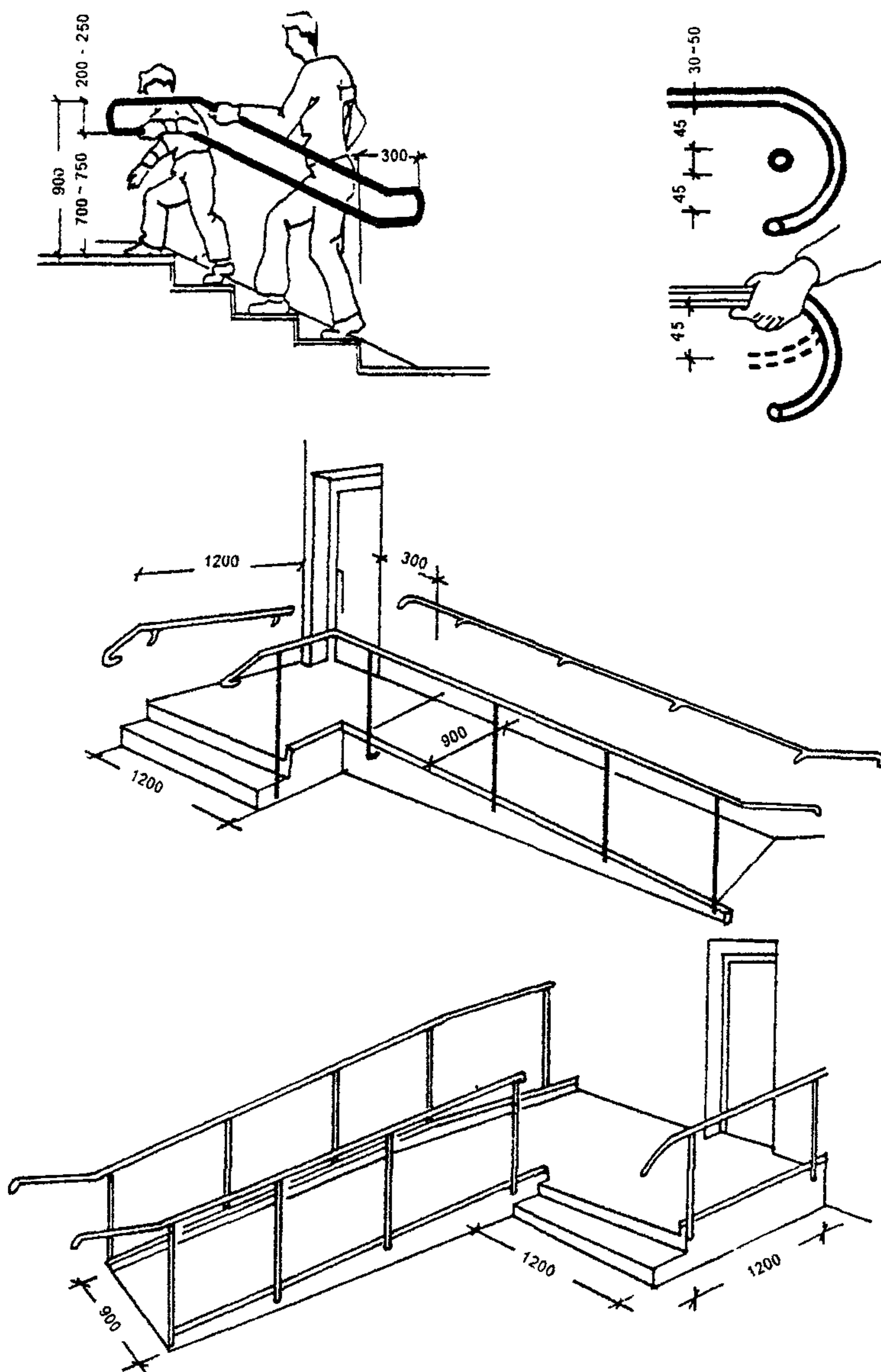
РИС 3 8 ПРИМЕРЫ УСТРОЙСТВА ВХОДНЫХ ЛЕСТНИЦ И ПАНДУСОВ
