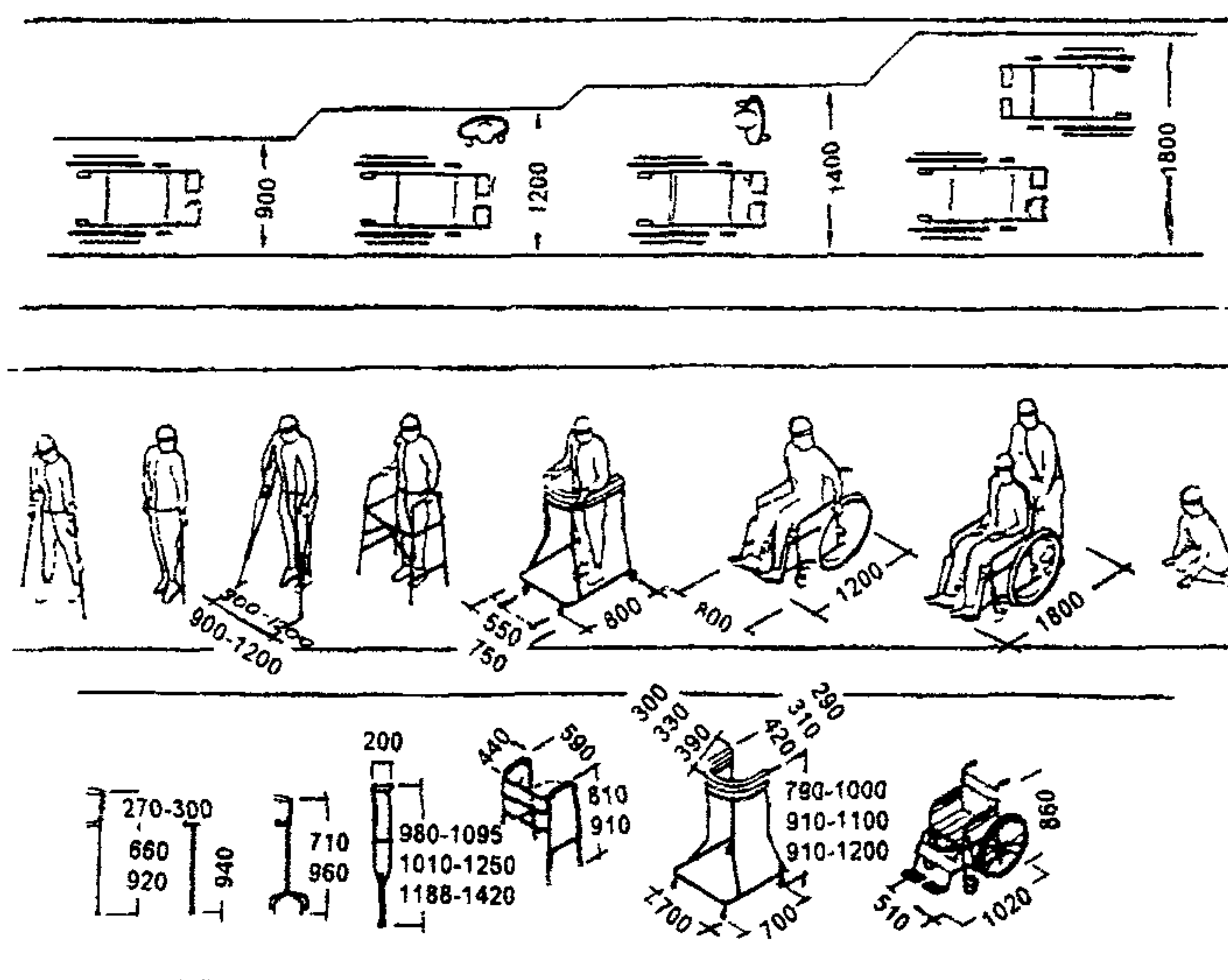
РИС.3.4 НЕОБХОДИМЫЕ ГАБАРИТЫ КОММУНИКАЦИЙ, УСТРОЙСТВ И СРЕДСТВ ПЕРЕДВИЖЕНИЯ ИНВАЛИДОВ
