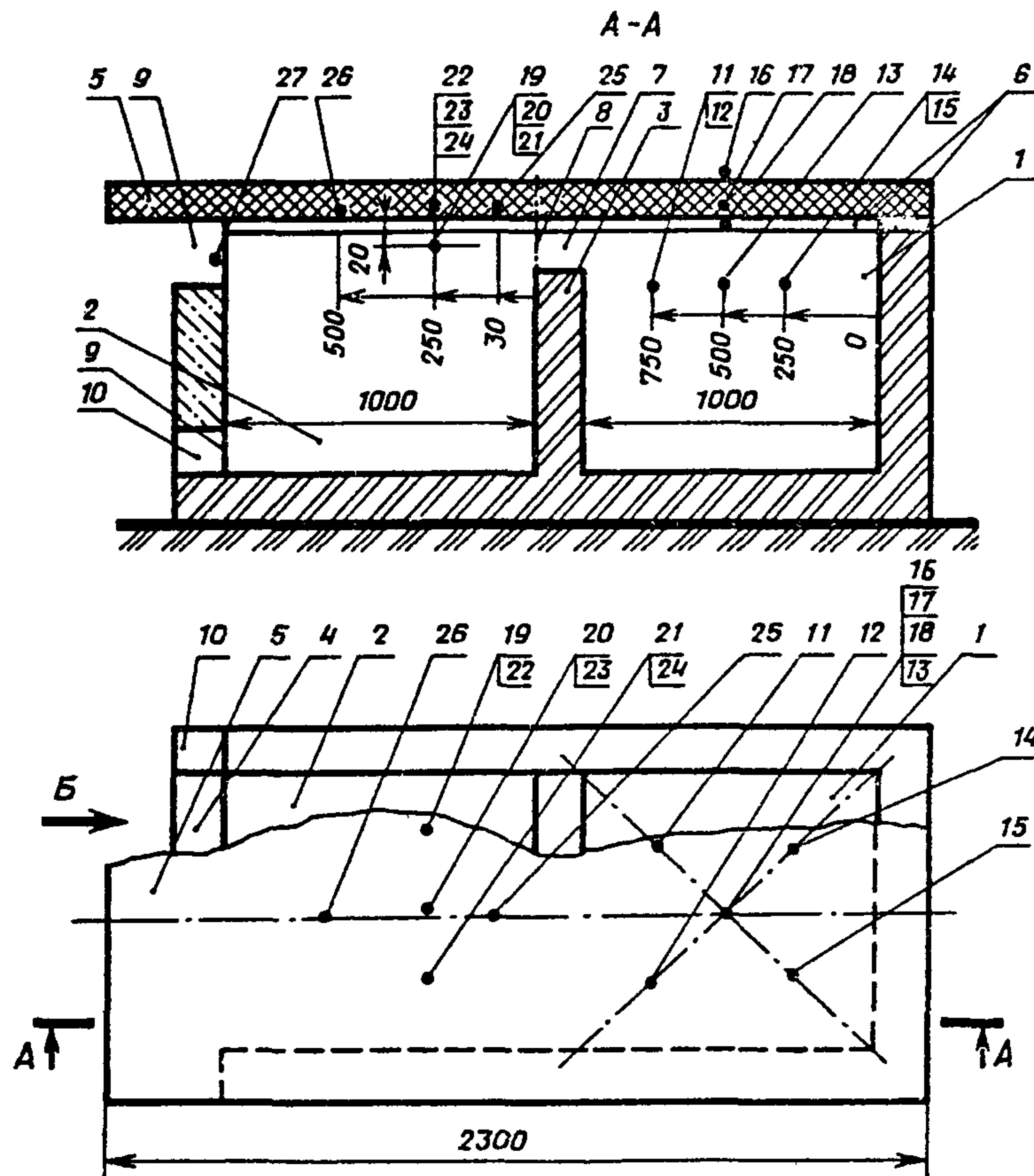
Рисунок 2 — Схема печи для испытаний горизонтальных конструкций и установки на ней образца конструкции
