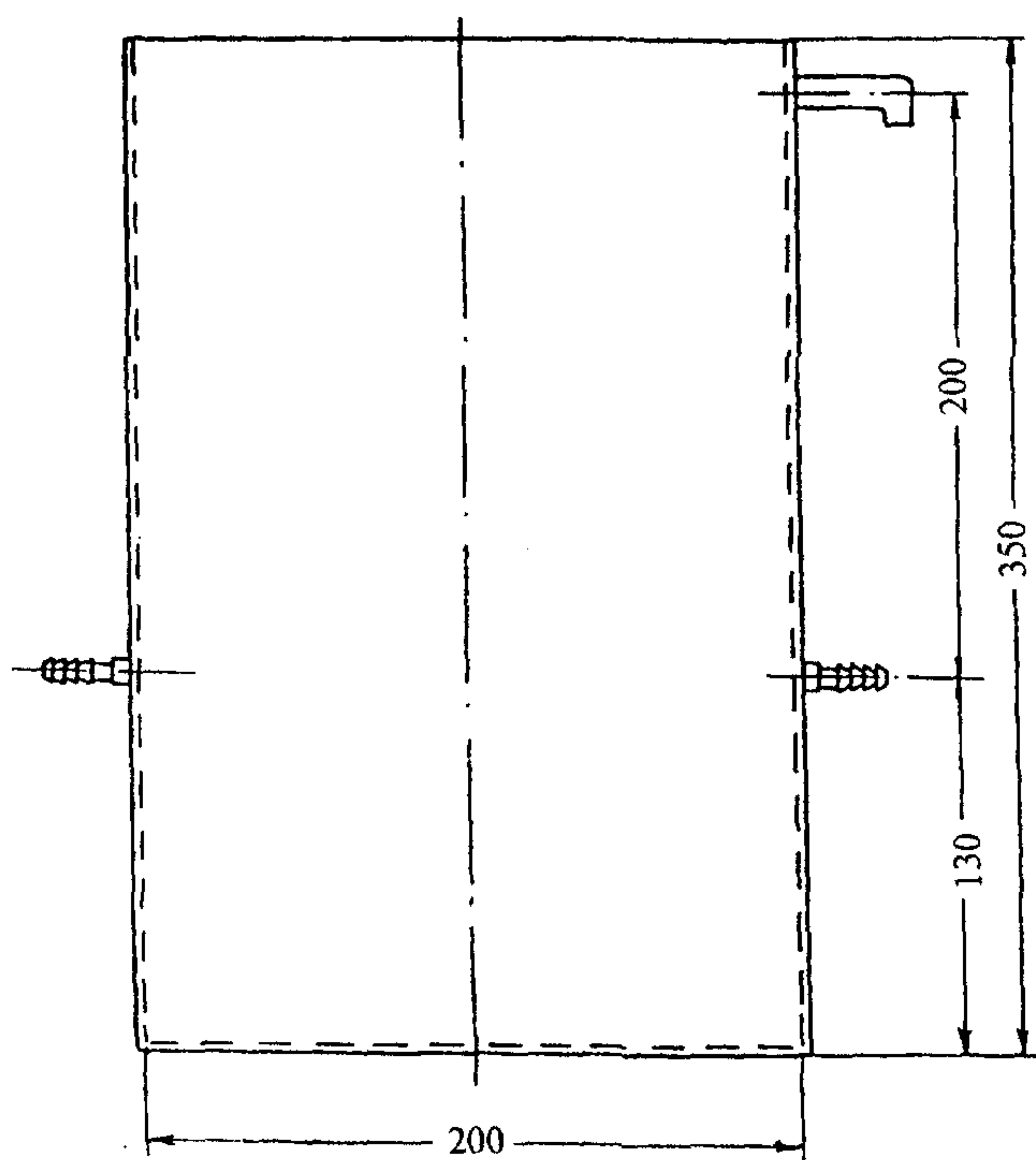
Рисунок 1 — Сосуд для отмучивания
