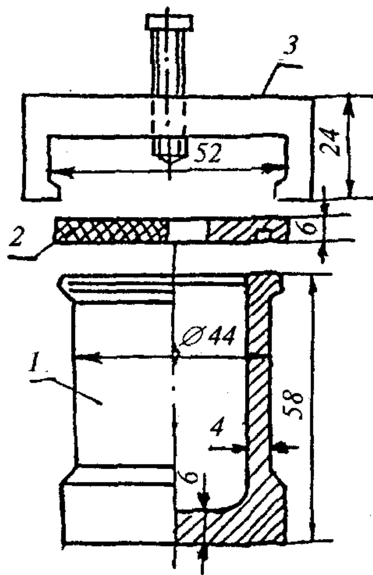
Рисунок 10 — Сосуд из коррозионно-стойкого материала
