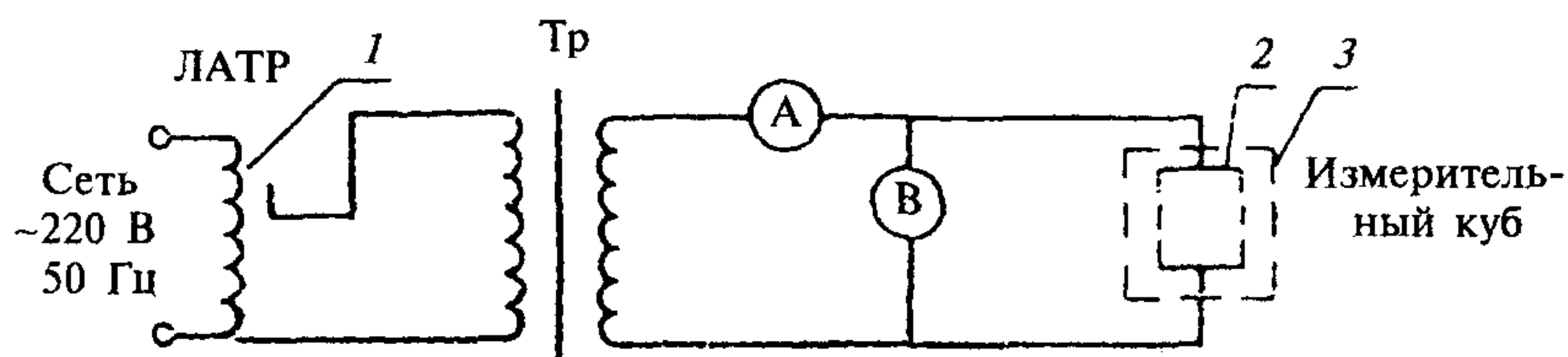
1 — лабораторный регулировочный трансформатор (ЛАТР); 2 — электрод; 3 — измерительный куб
