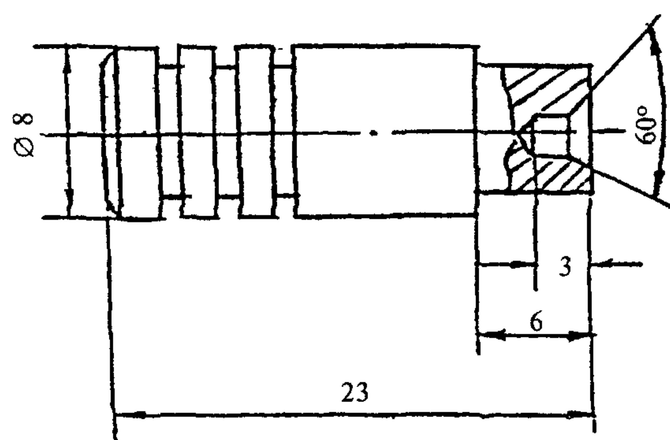
Рисунок 13 — Репер для испытаний
