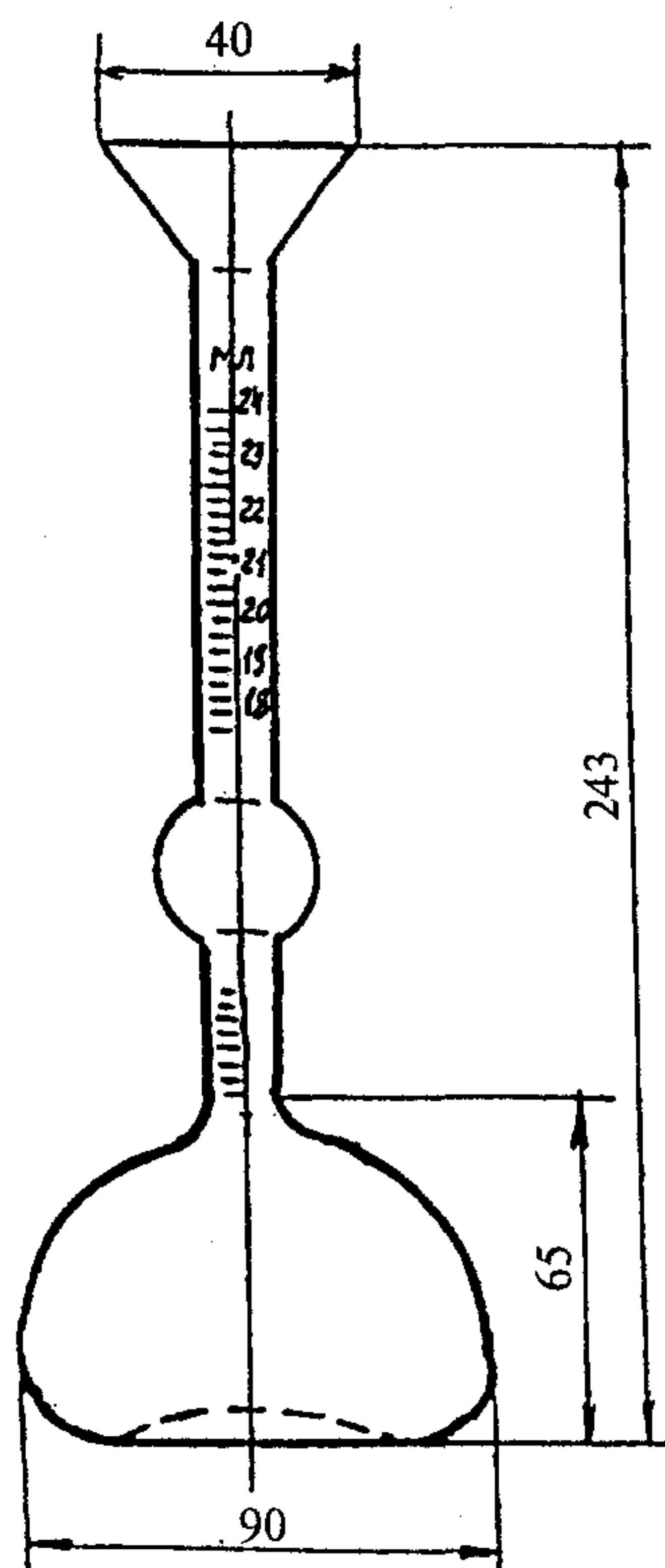
Рисунок 8 — Прибор Ле Шателье
