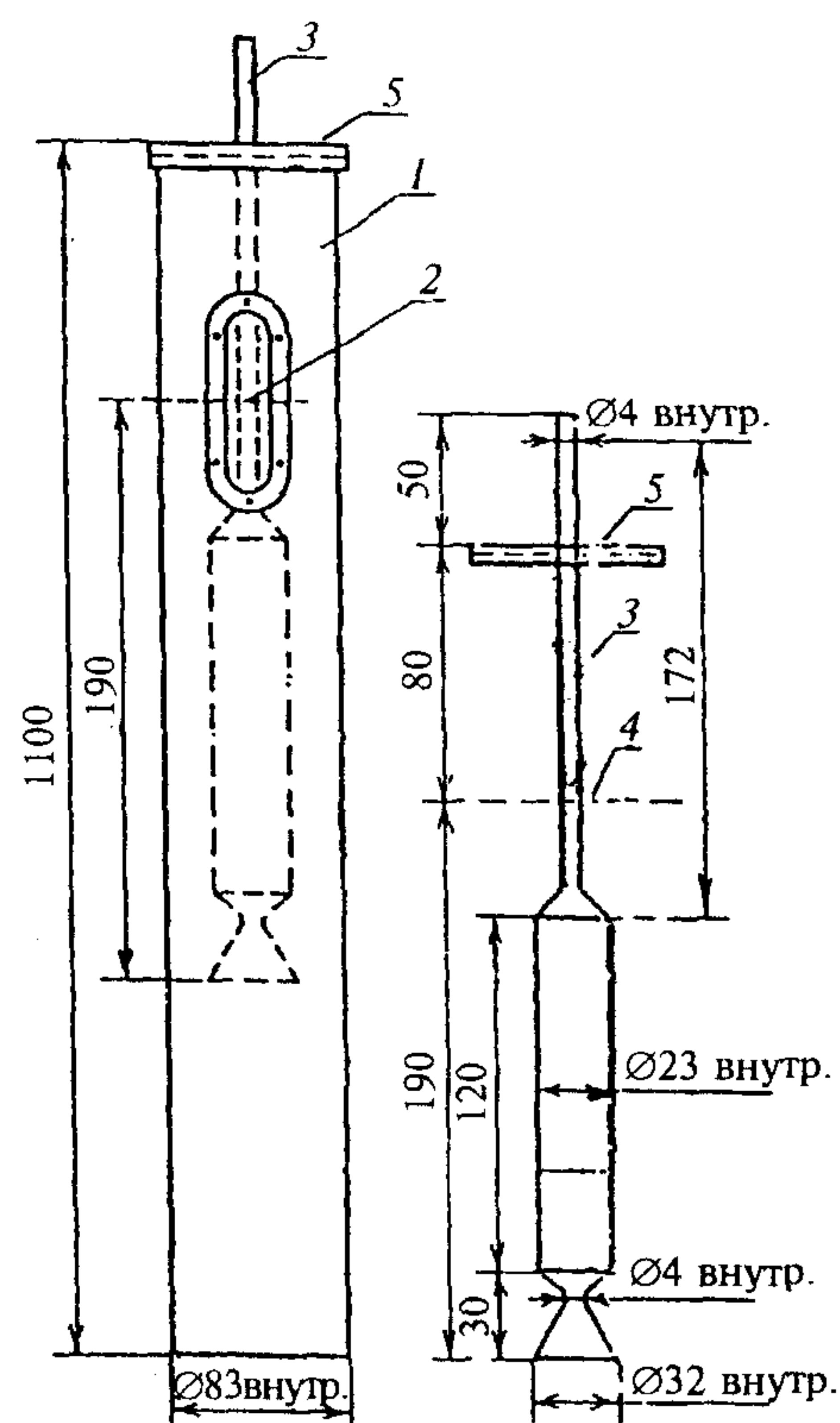
Рисунок 2 — Металлический цилиндр и мерная пипетка
