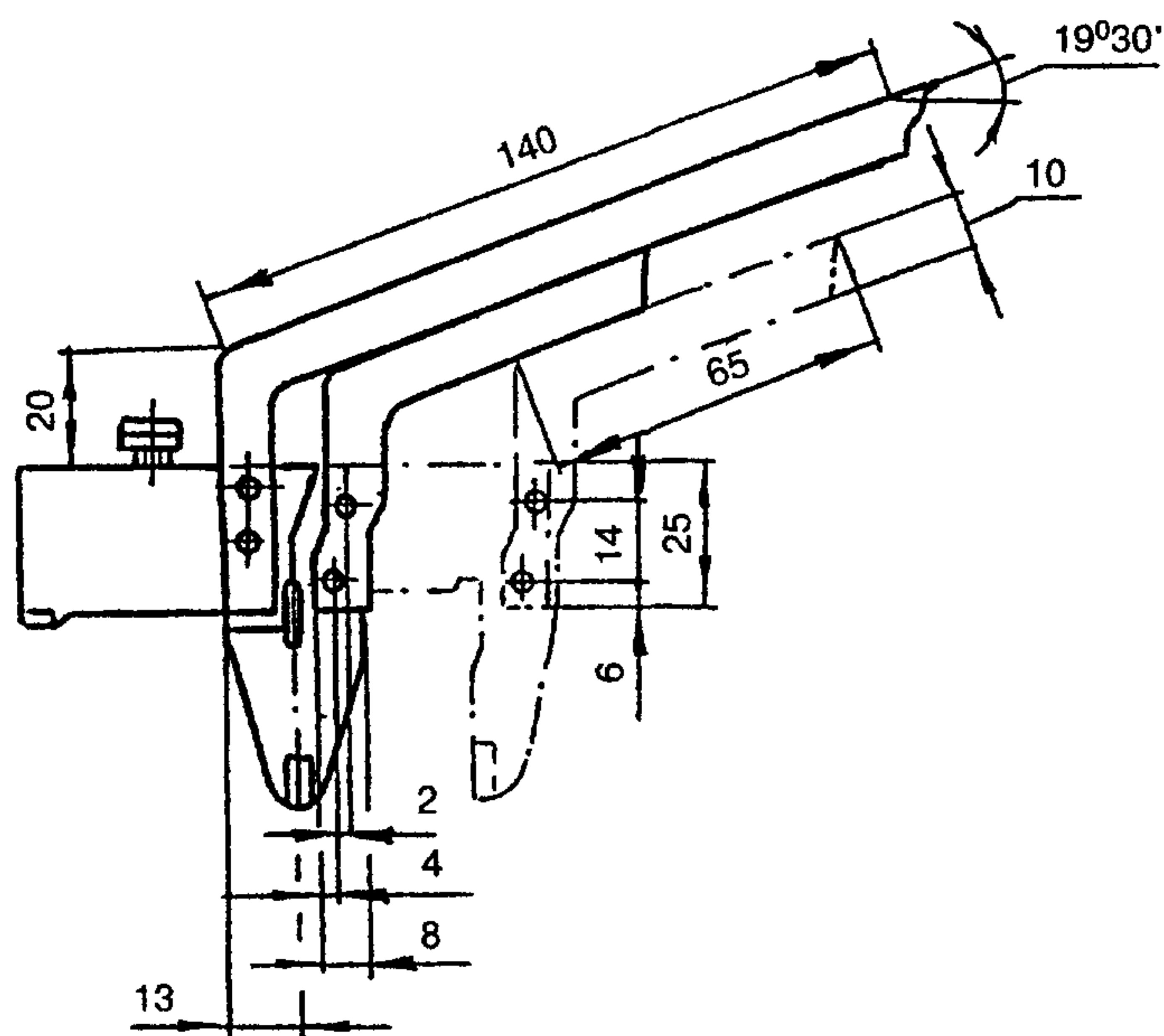
Рисунок 3 — Передвижной шаблон
