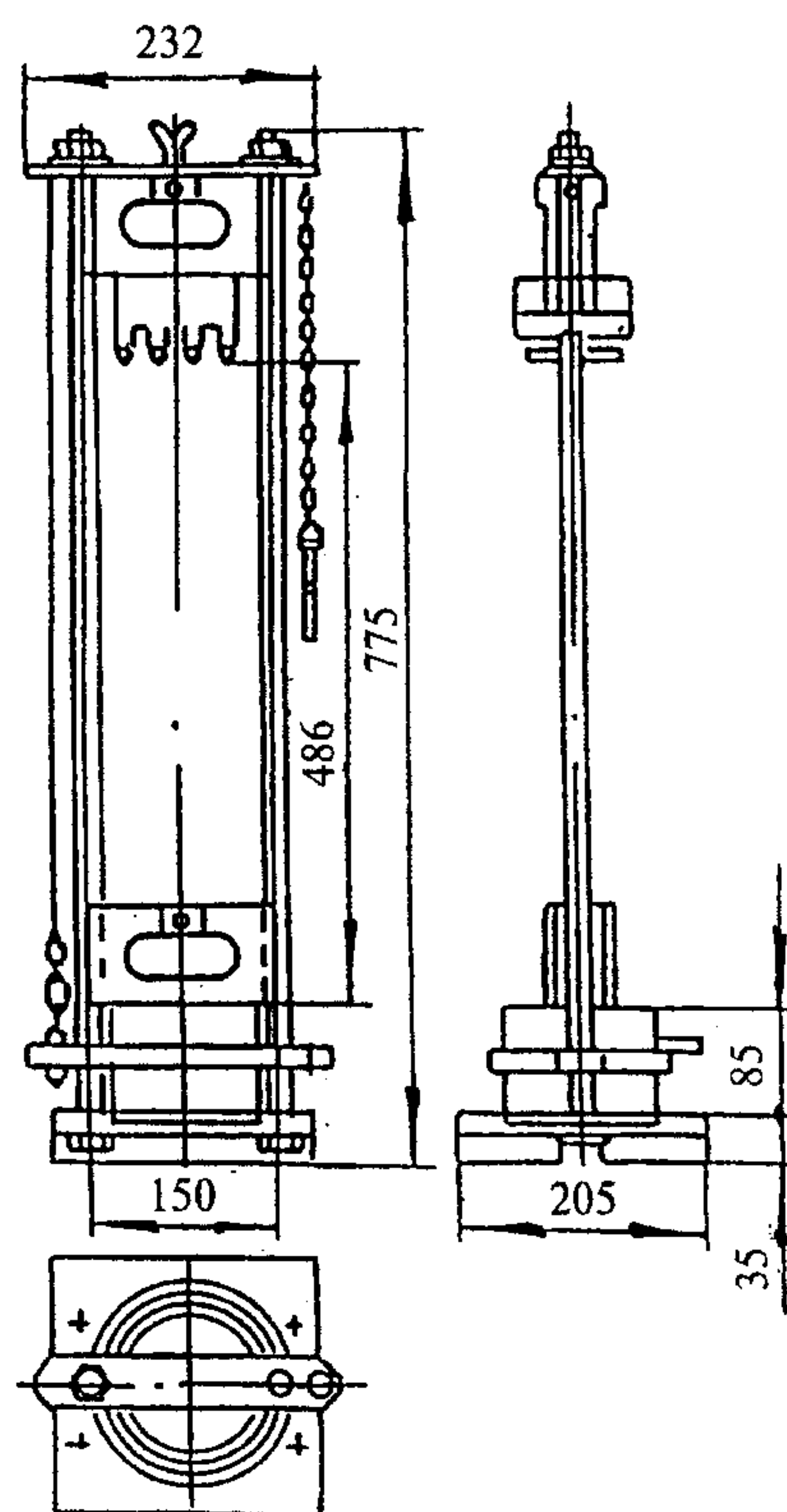
Рисунок 7 — Копер ПМ
