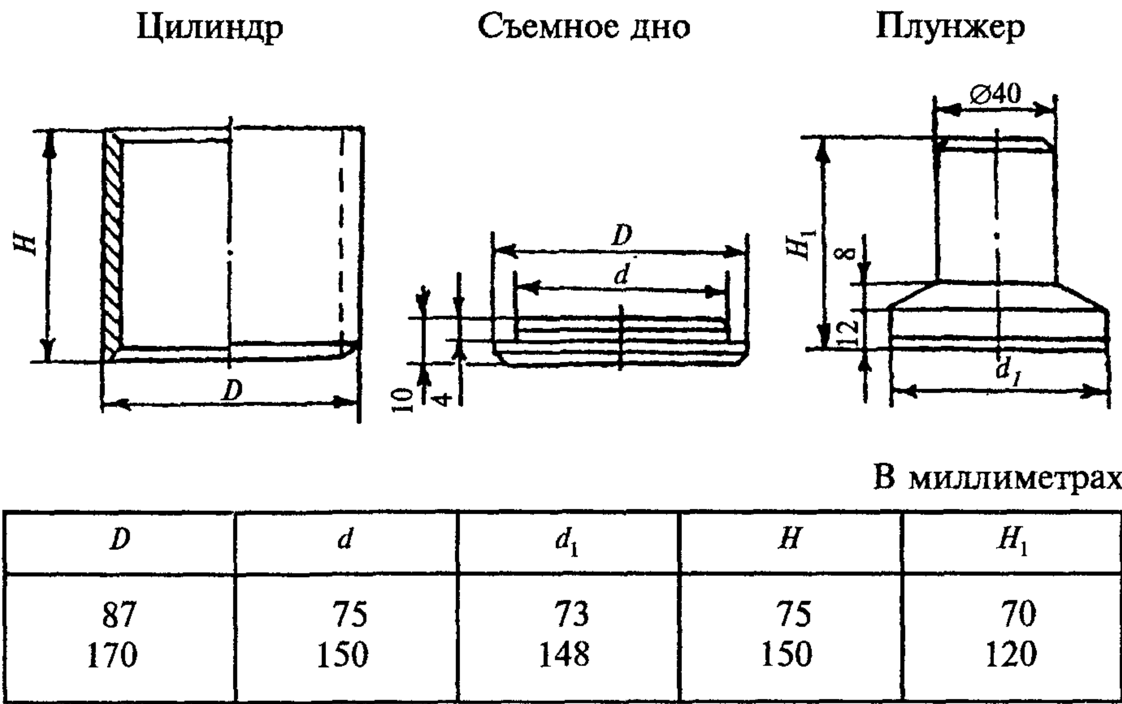
Рисунок 4 — Цилиндры стальные
