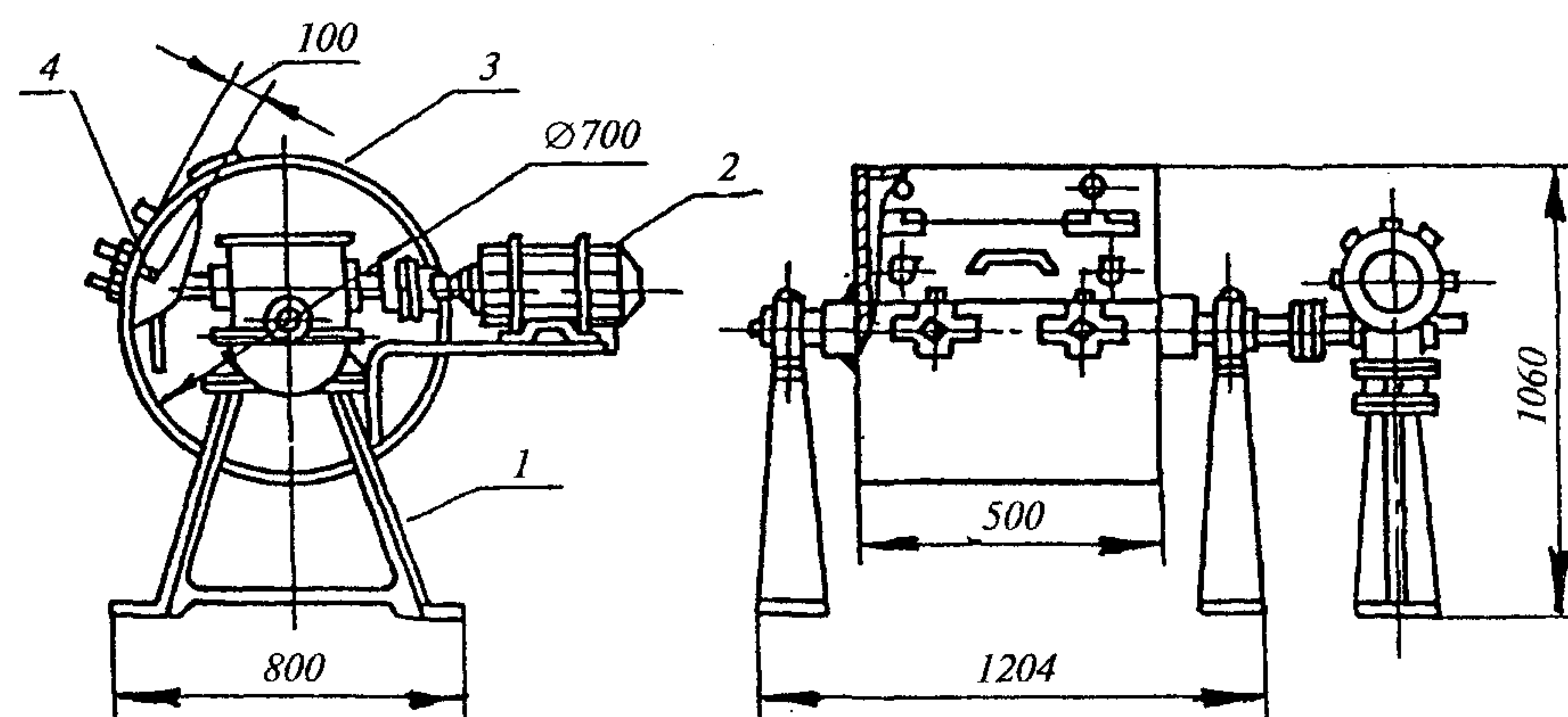
1 — станина; 2 — двигатель; 3 — барабан; 4 — полка барабана
