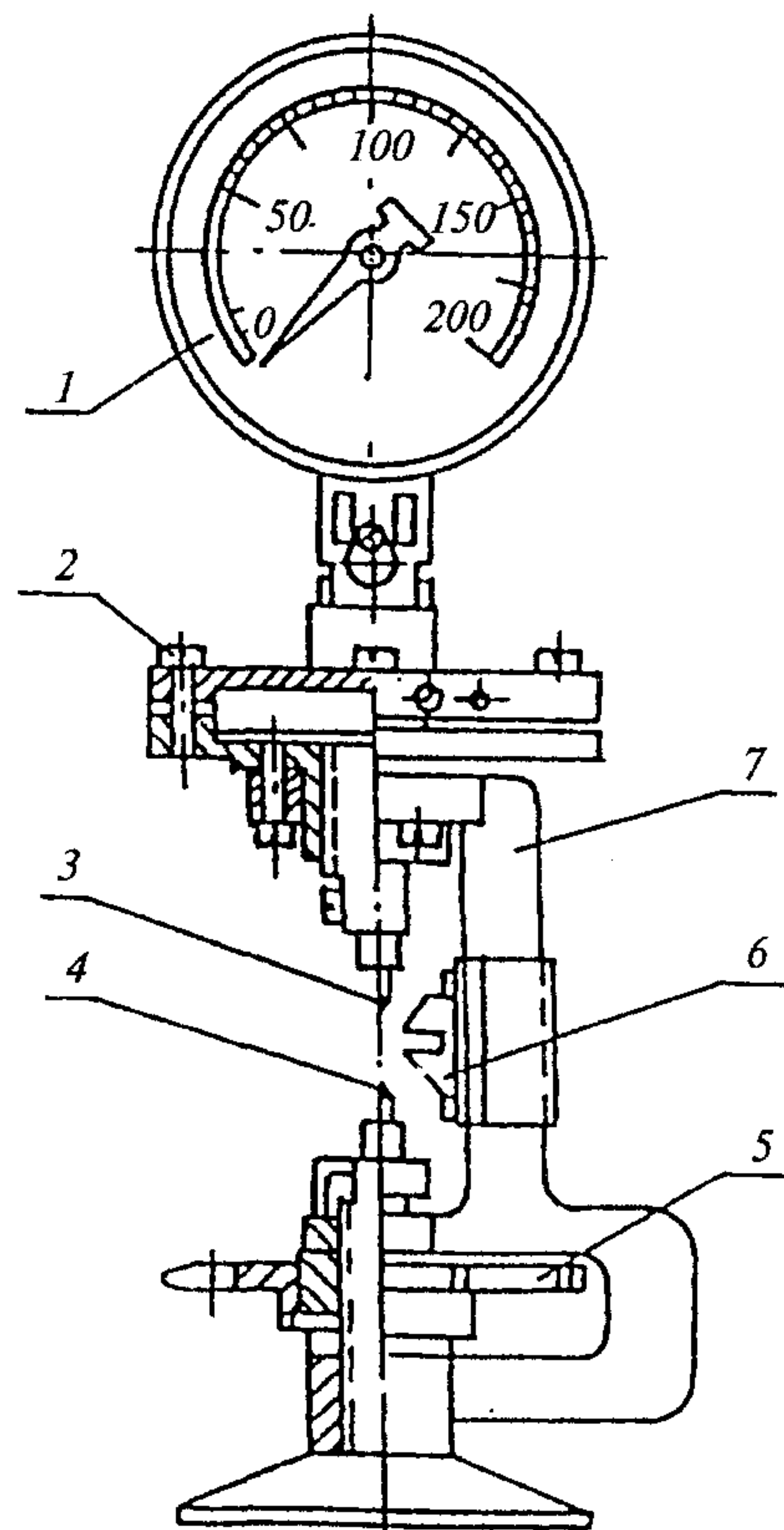
Рисунок 5 — Механический индикатор прочности камня (Т-3)
