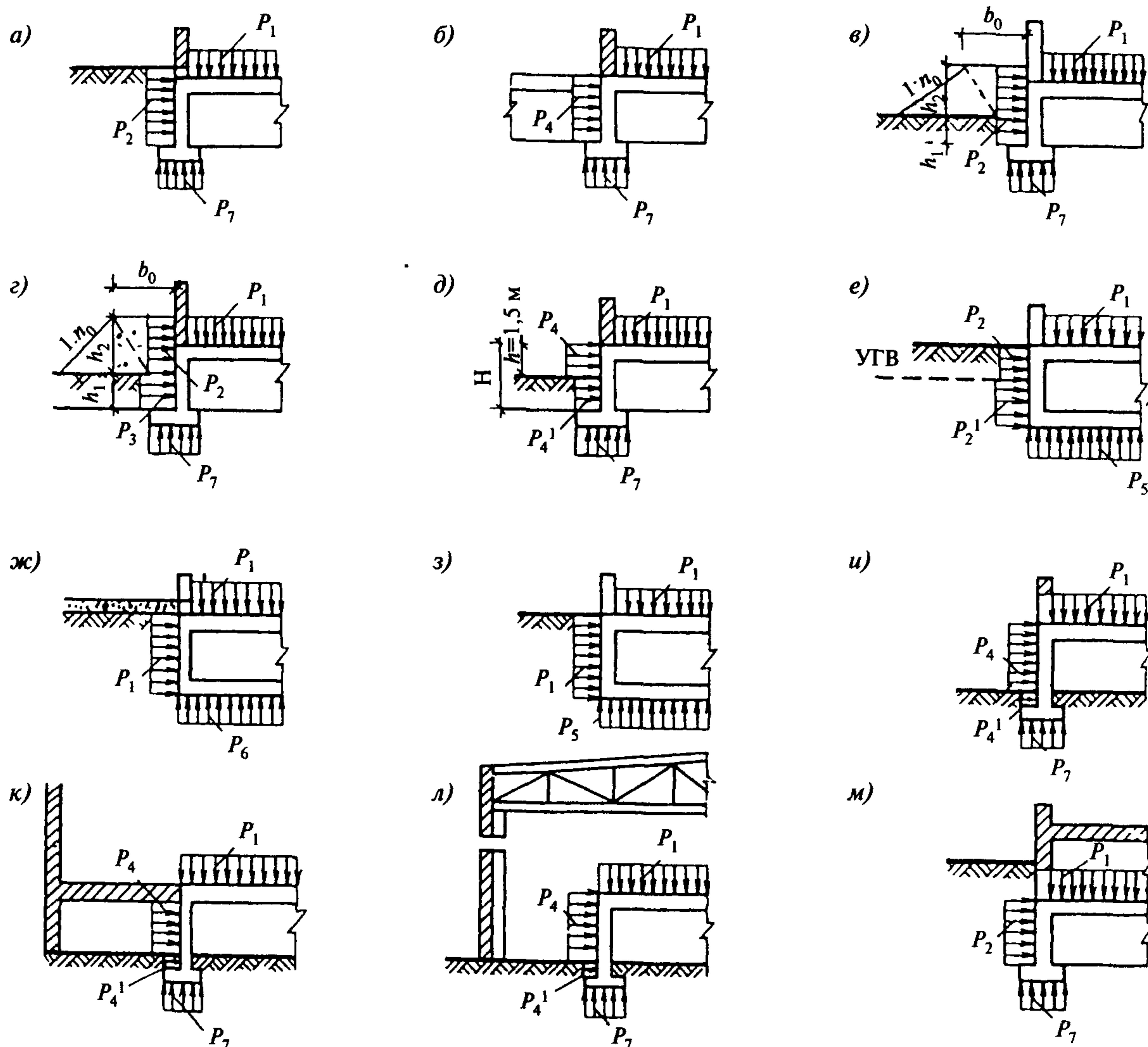
Схемы приложения динамических нагрузок на конструкции
