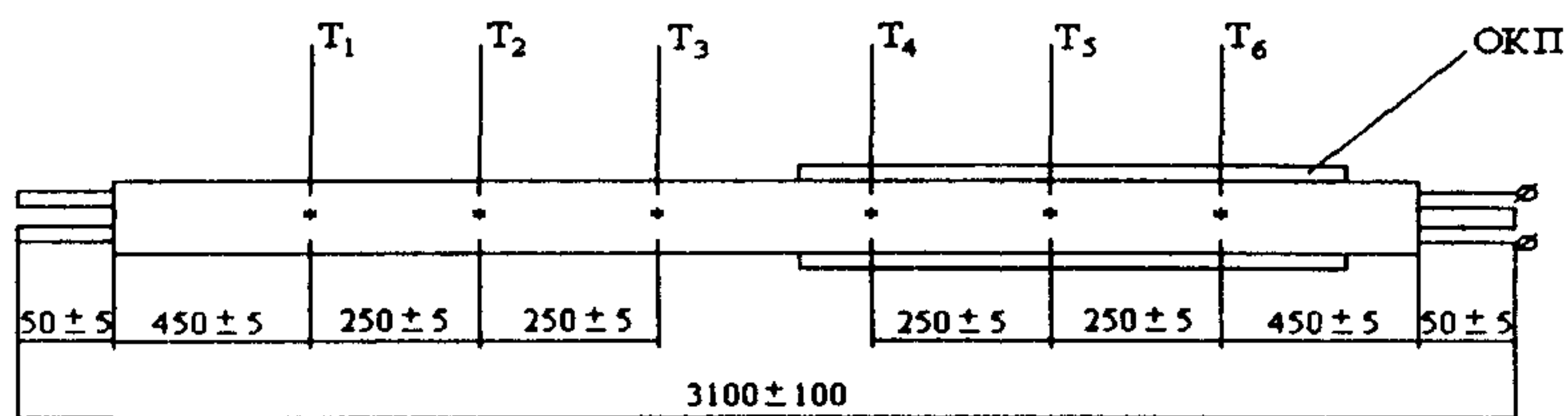
Размещение термоэлектрических преобразователей
