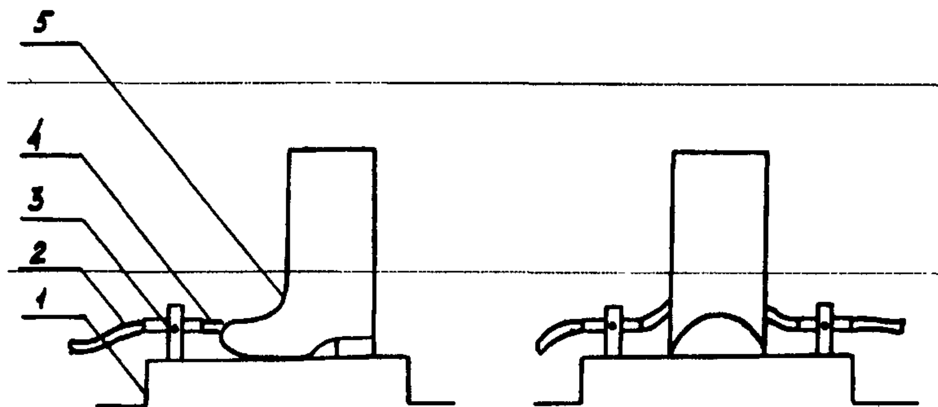
Схема установки по проверке огнезащитных свойств резиновой обуви:
