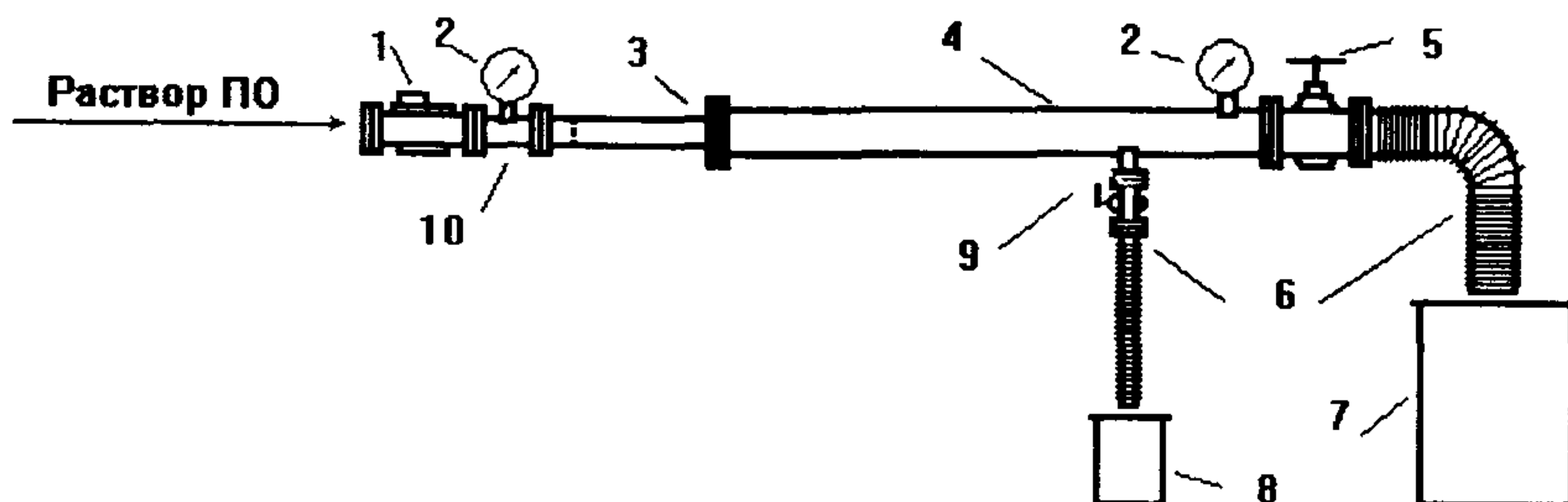
Рис. 1. Схема установки для испытания высоконапорных генераторов:
