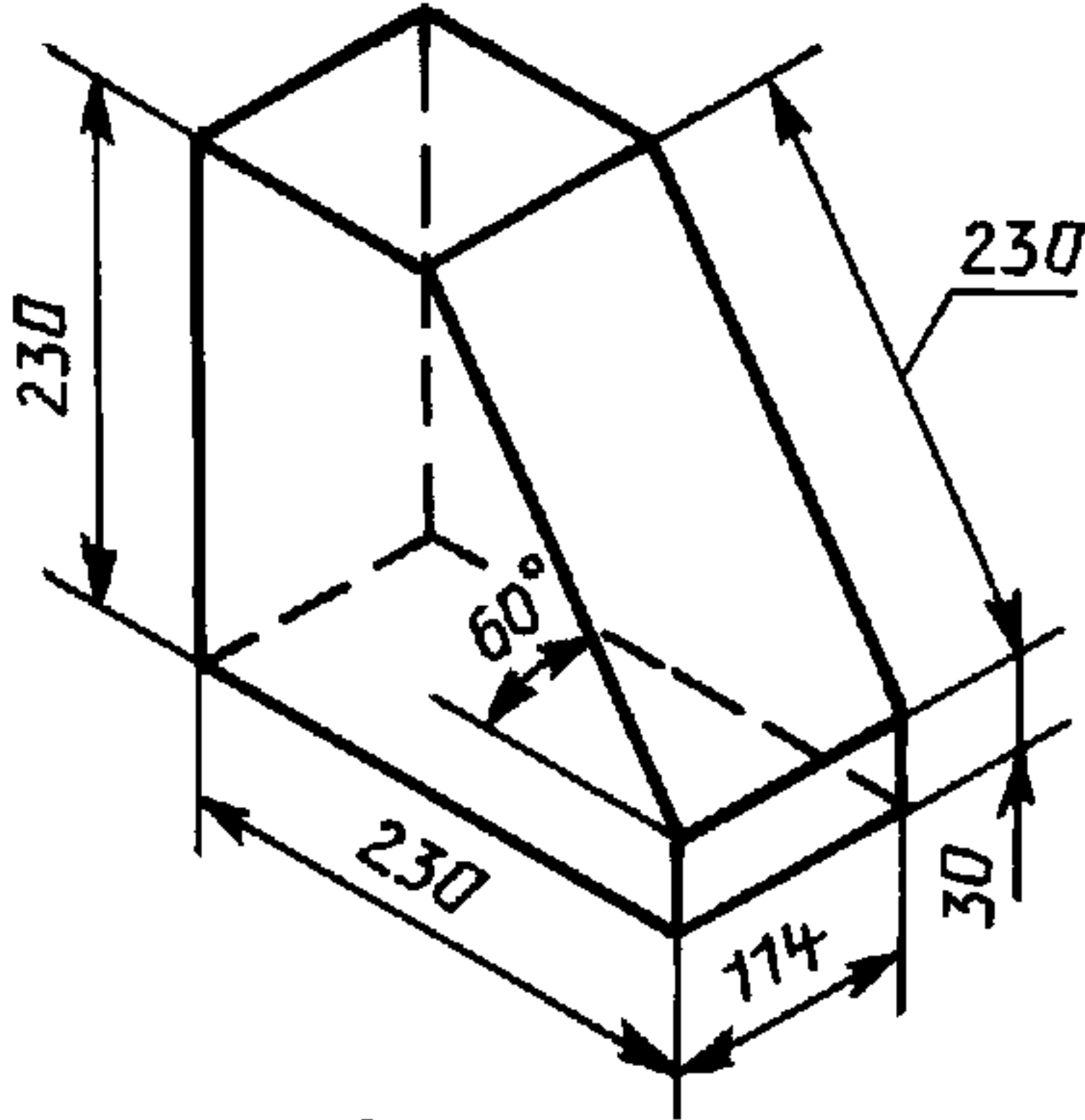
Объем 4,72 дм³
