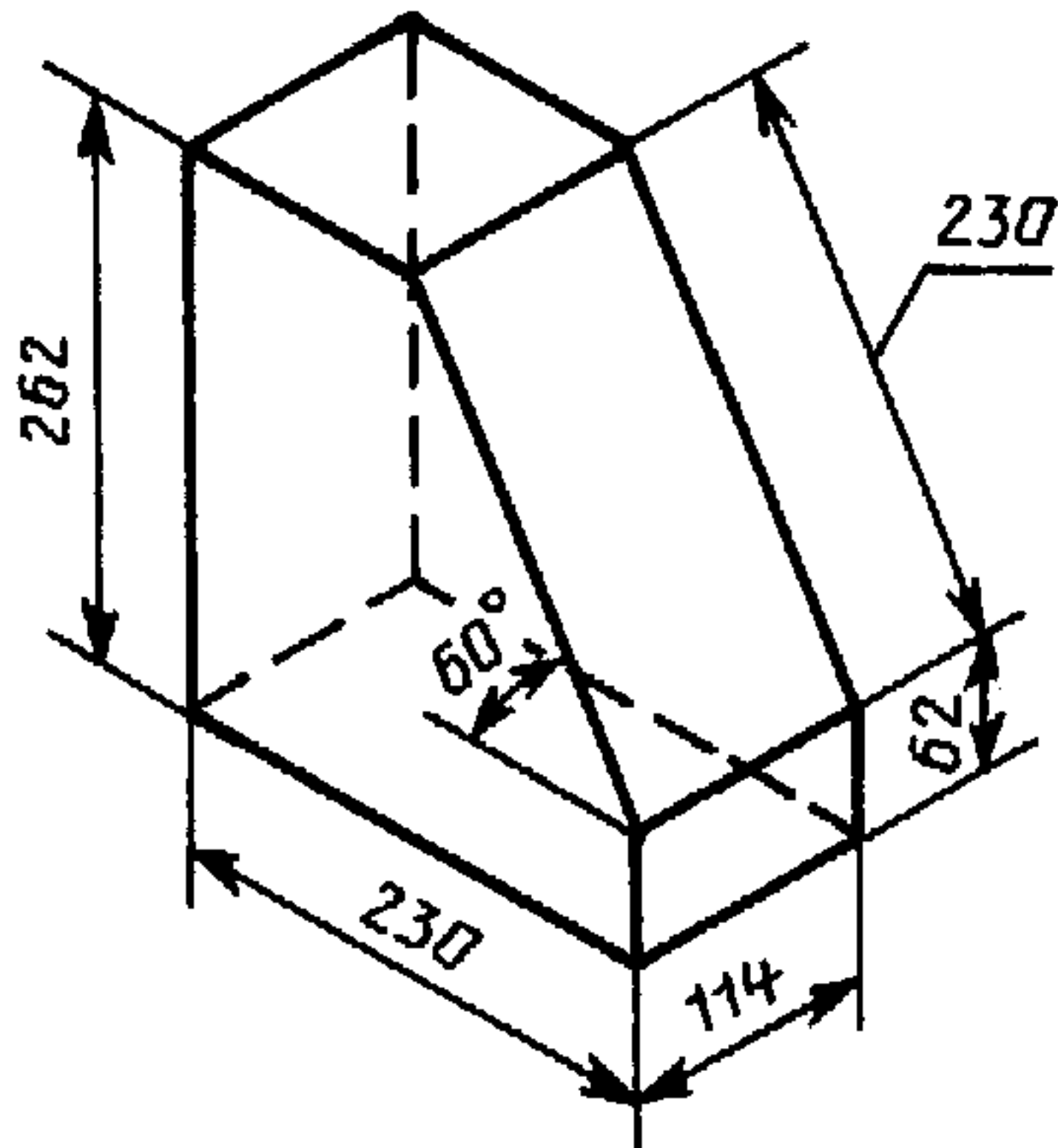
Объем 5,57 дм³
