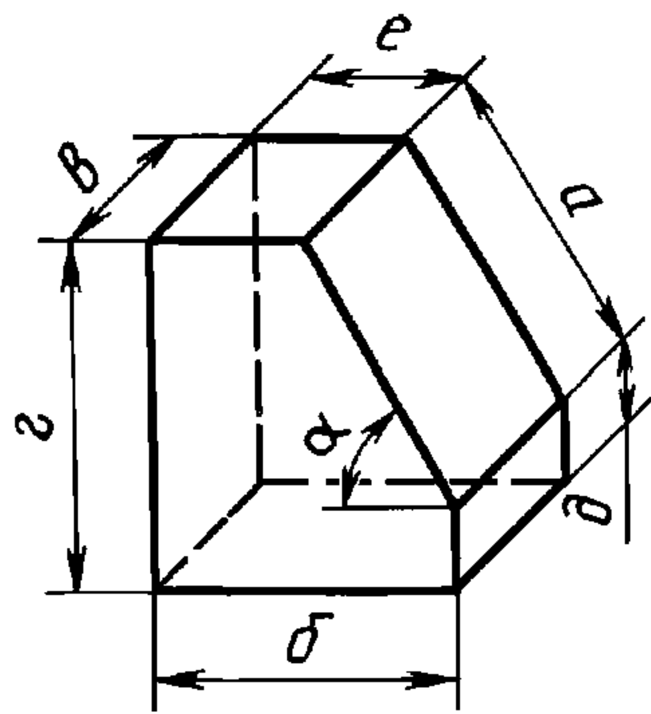
Кирпич пятовый
