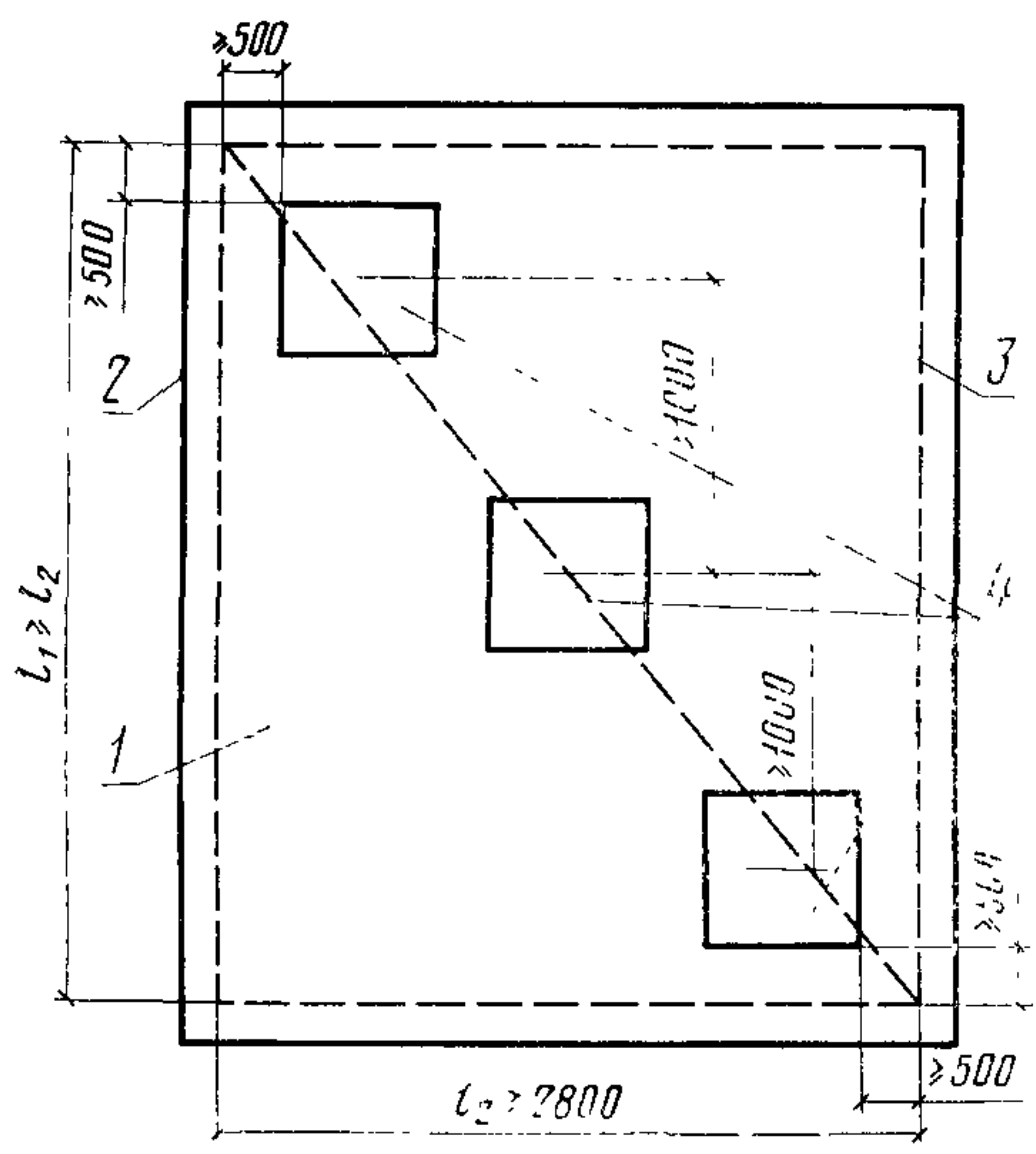
1—перекрытие; 2—край перекрытия между помещением высокого уровня и помещением низкого уровня; 3—край проема перекрытия; 4—положение образцов
