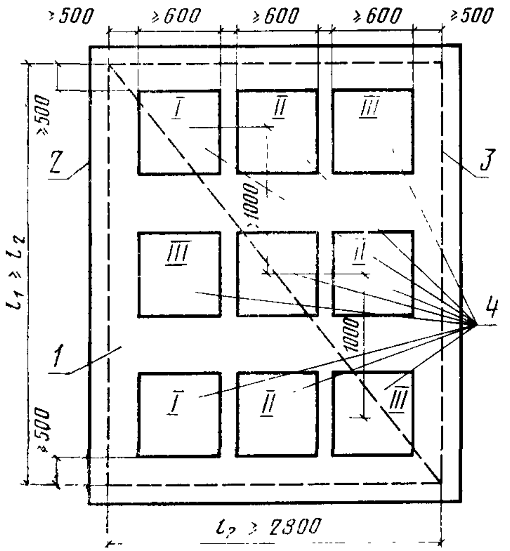
1—перекрытие; 2—край перекрытия между помещением высокого уровня и помещением низкого уровня; 3—край проема перекрытия; 4—положение частей образцов
