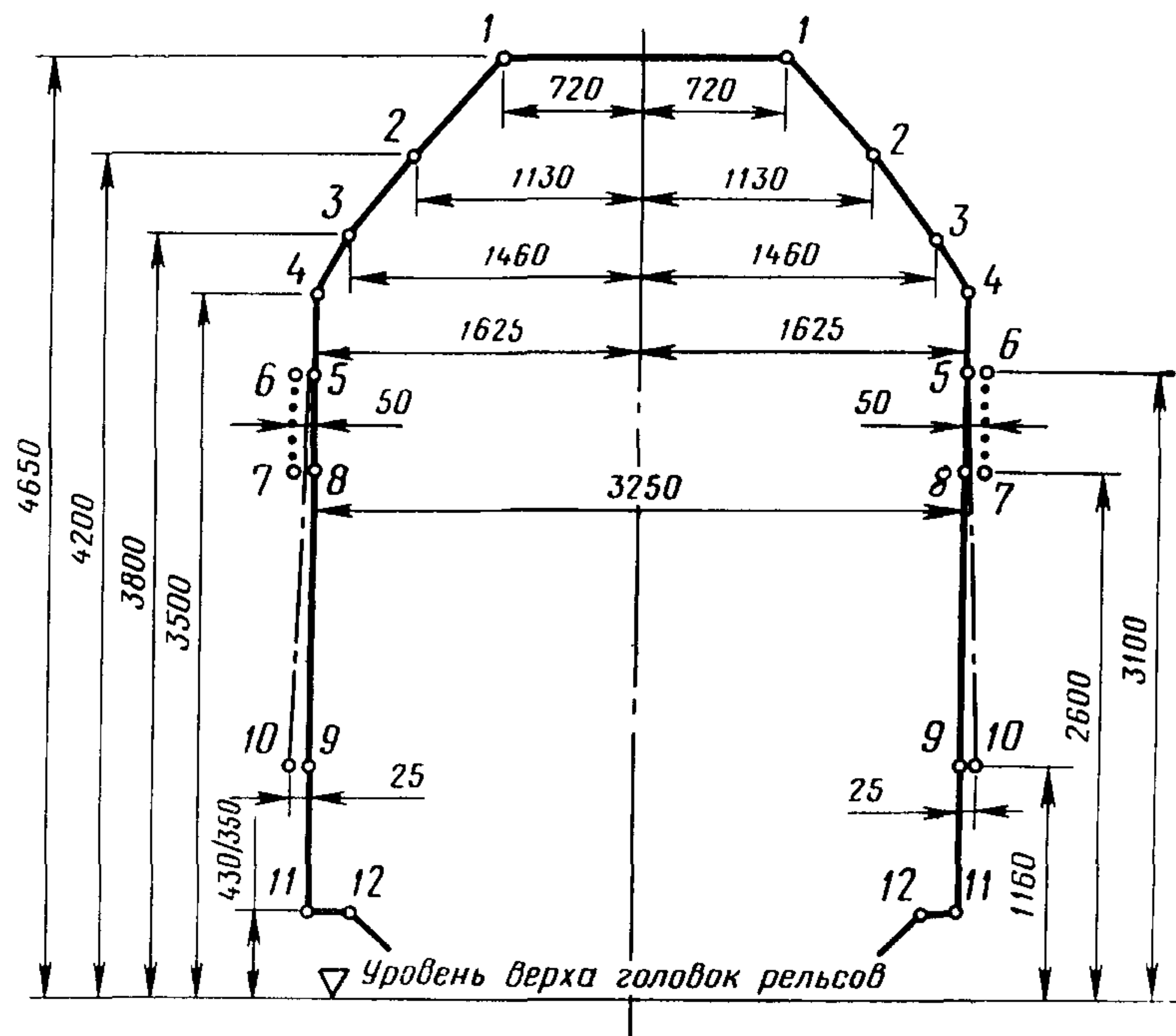
ГАБАРИТ 0-ВМ Верхнее очертание габарита
