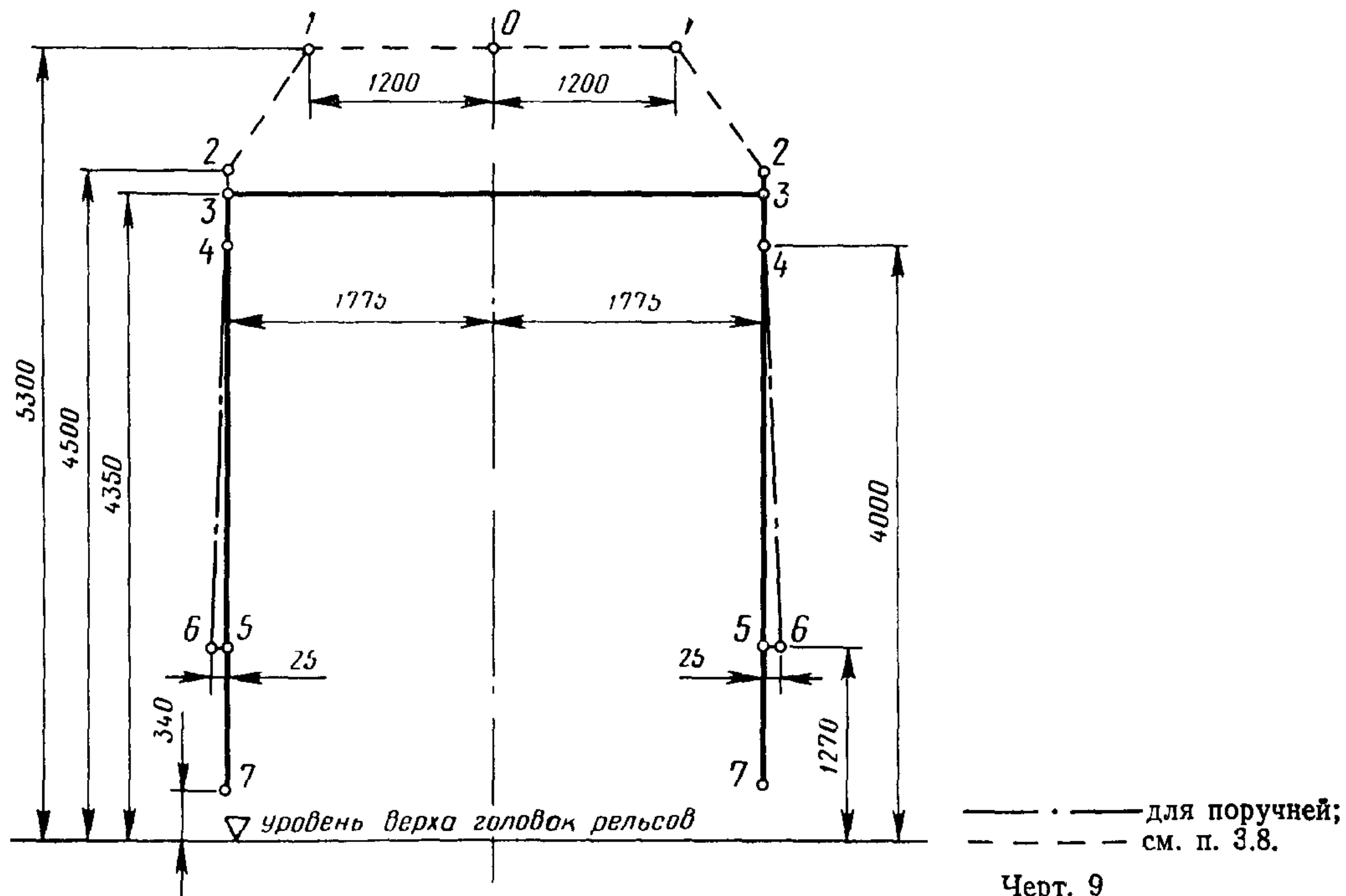
ГАБАРИТ 1-Т Верхнее очертание габарита
