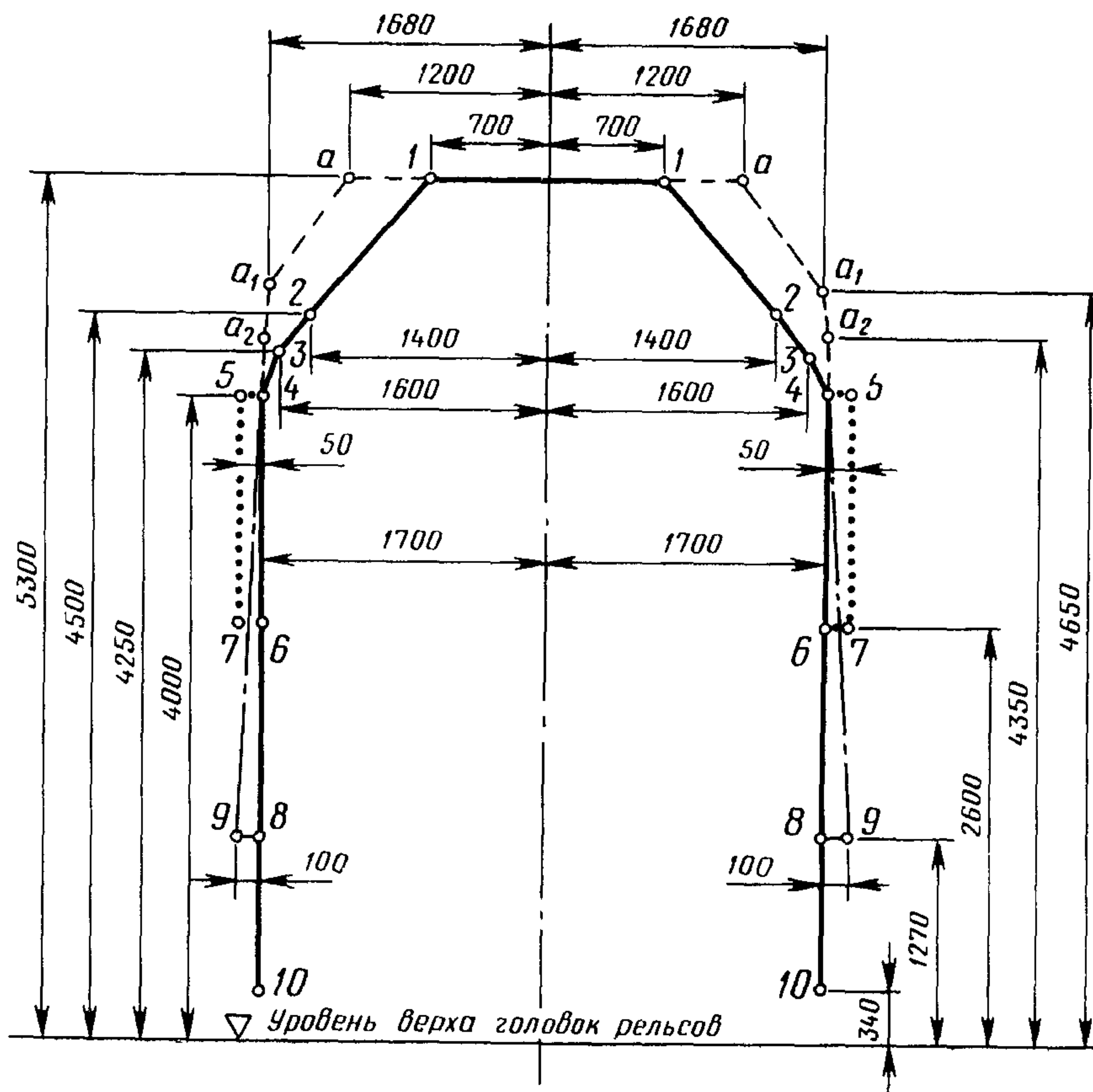
ГАБАРИТ 1-Т Верхнее очертание габарита
