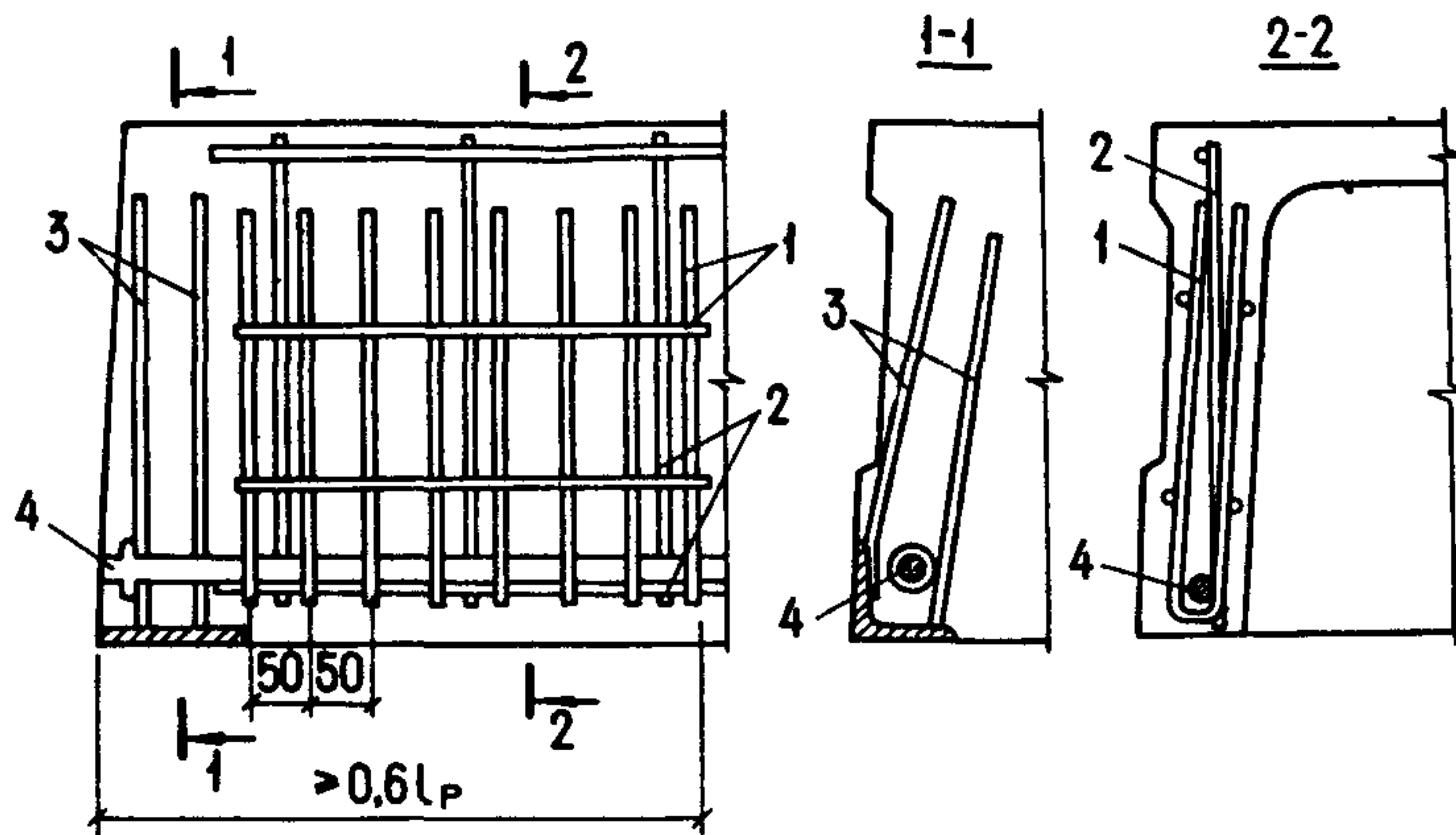
Черт. 63. Армирование конца ребра плиты перекрытия
