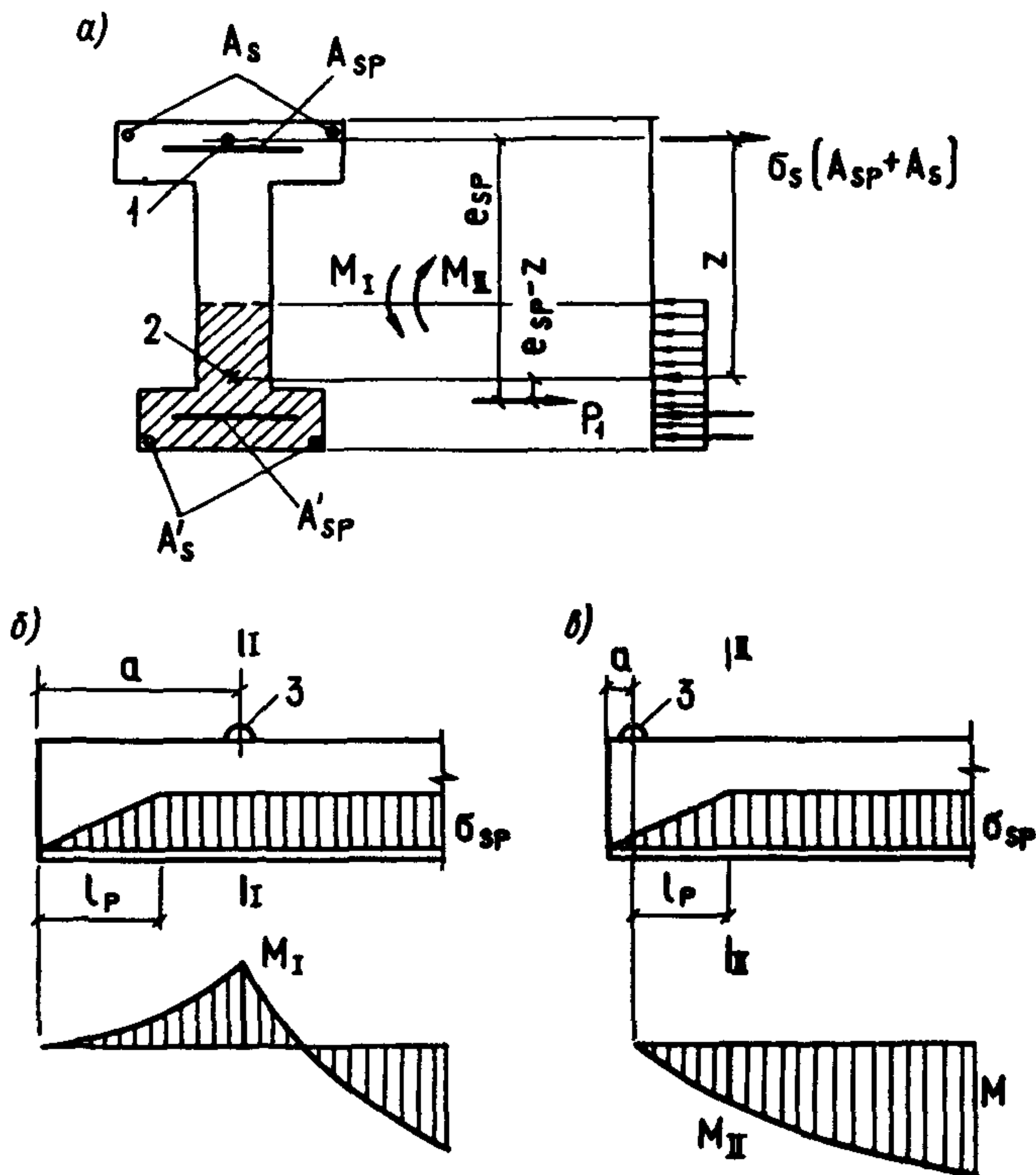
Черт. 47. Определение ширины раскрытия трещин, нормальных к продольной оси элемента, в стадии изготовления
