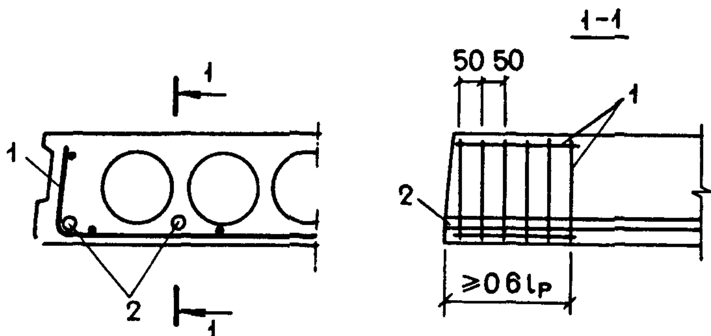
Черт. 62. Армирование конца многопустотного настила
