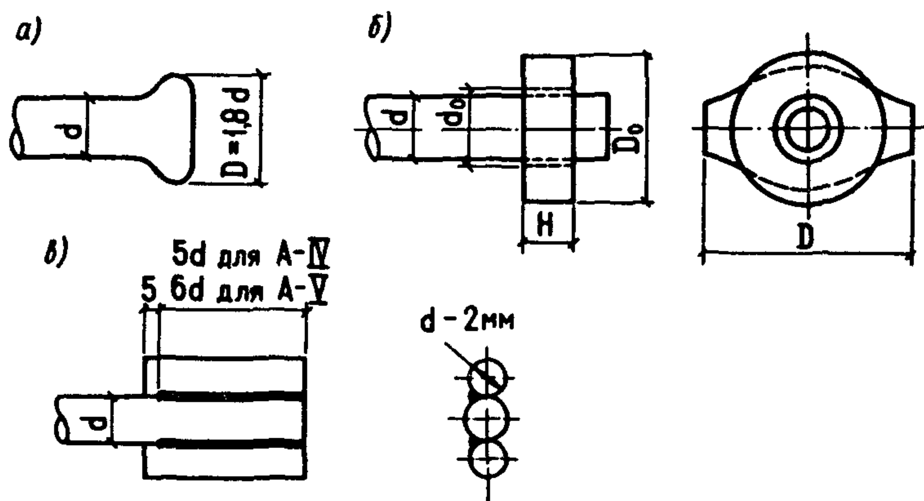
Черт. 59. Временные технологические анкера на напрягаемой стержневой арматуре а — высаженная головка; б — обжатая шайба (размеры см. табл. 48); в — приваренные коротыши
