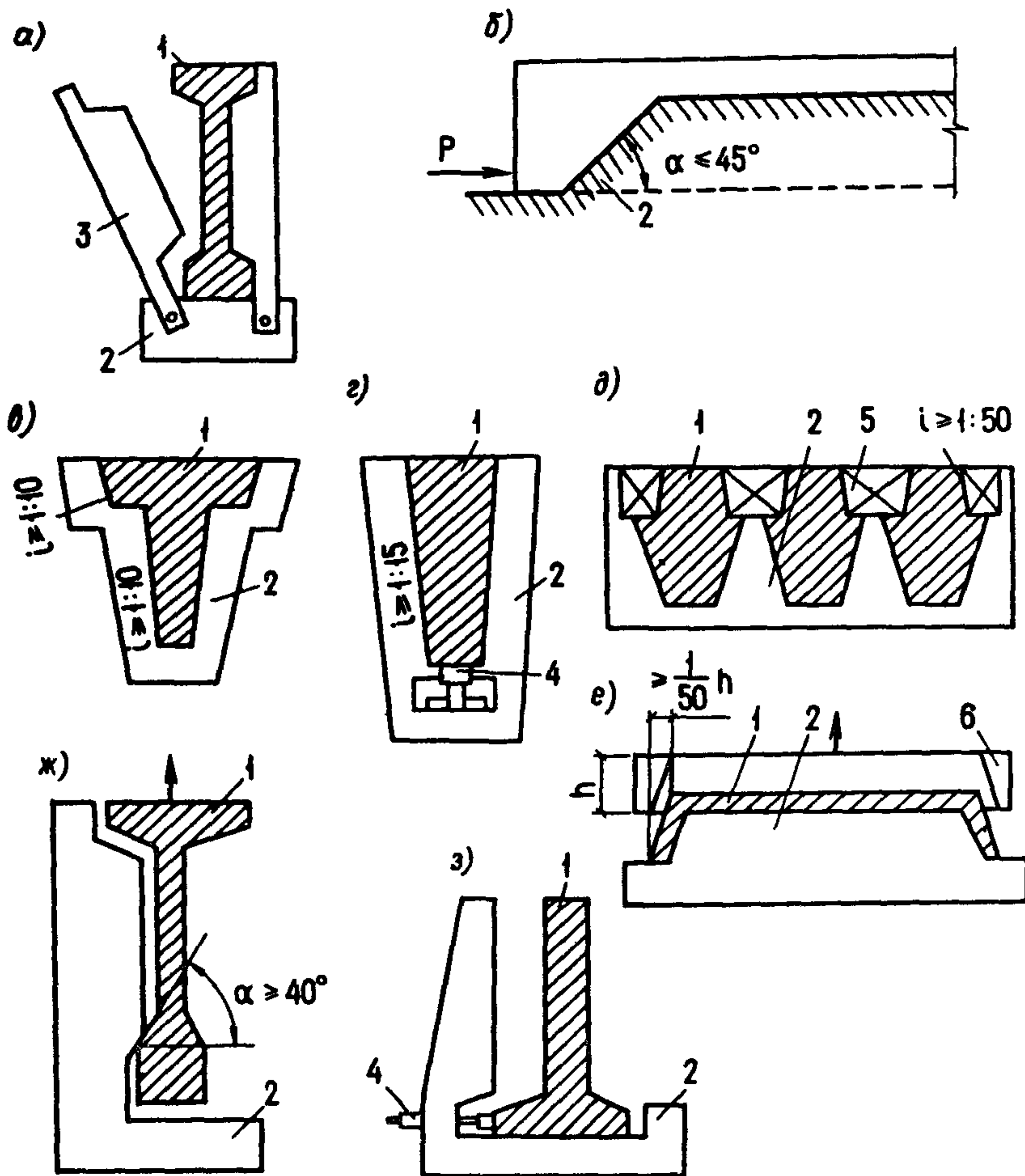
Черт. 55. Технологические уклоны
