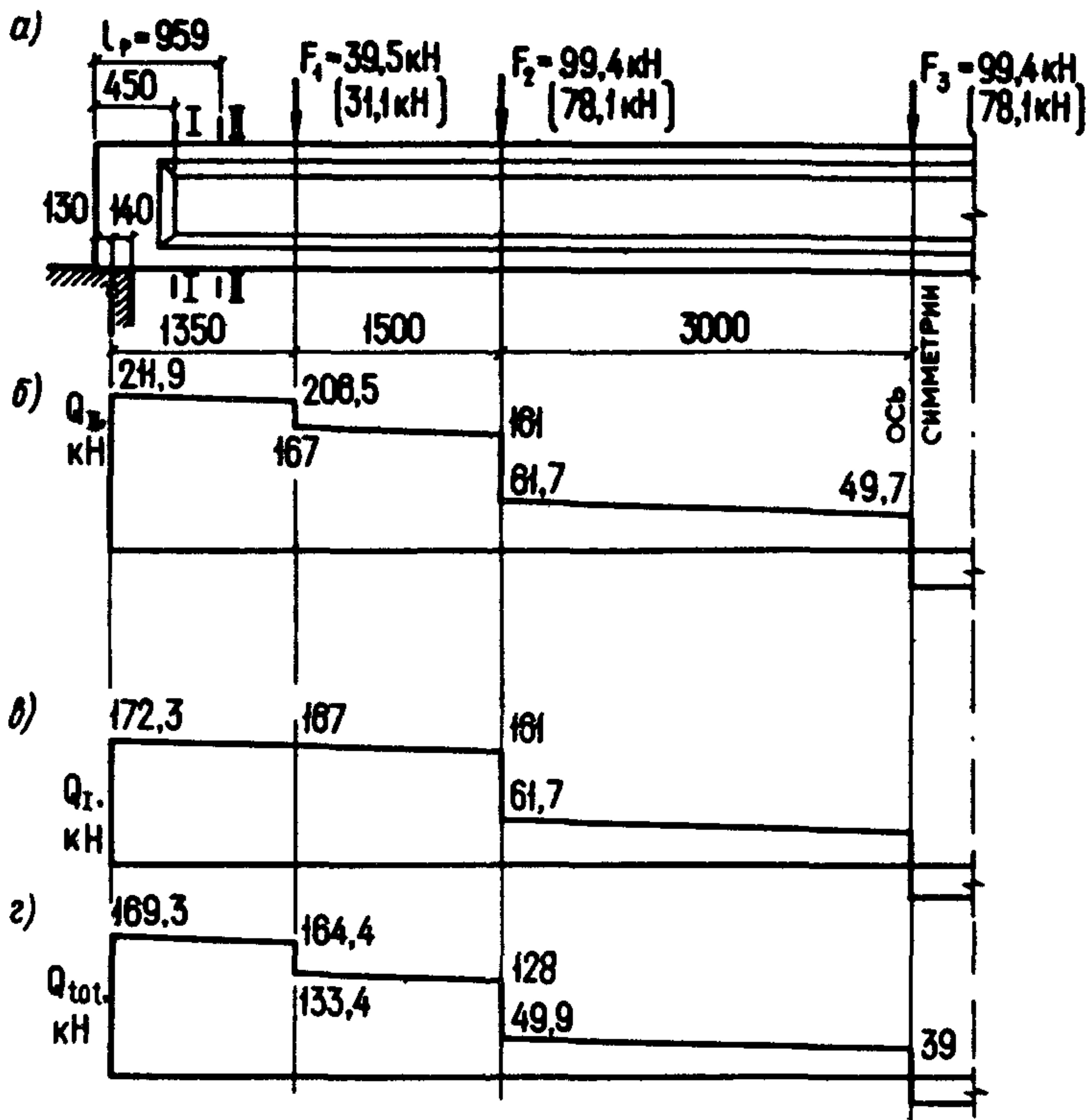
Черт. 2. Эпюры поперечных сил балки покрытия
