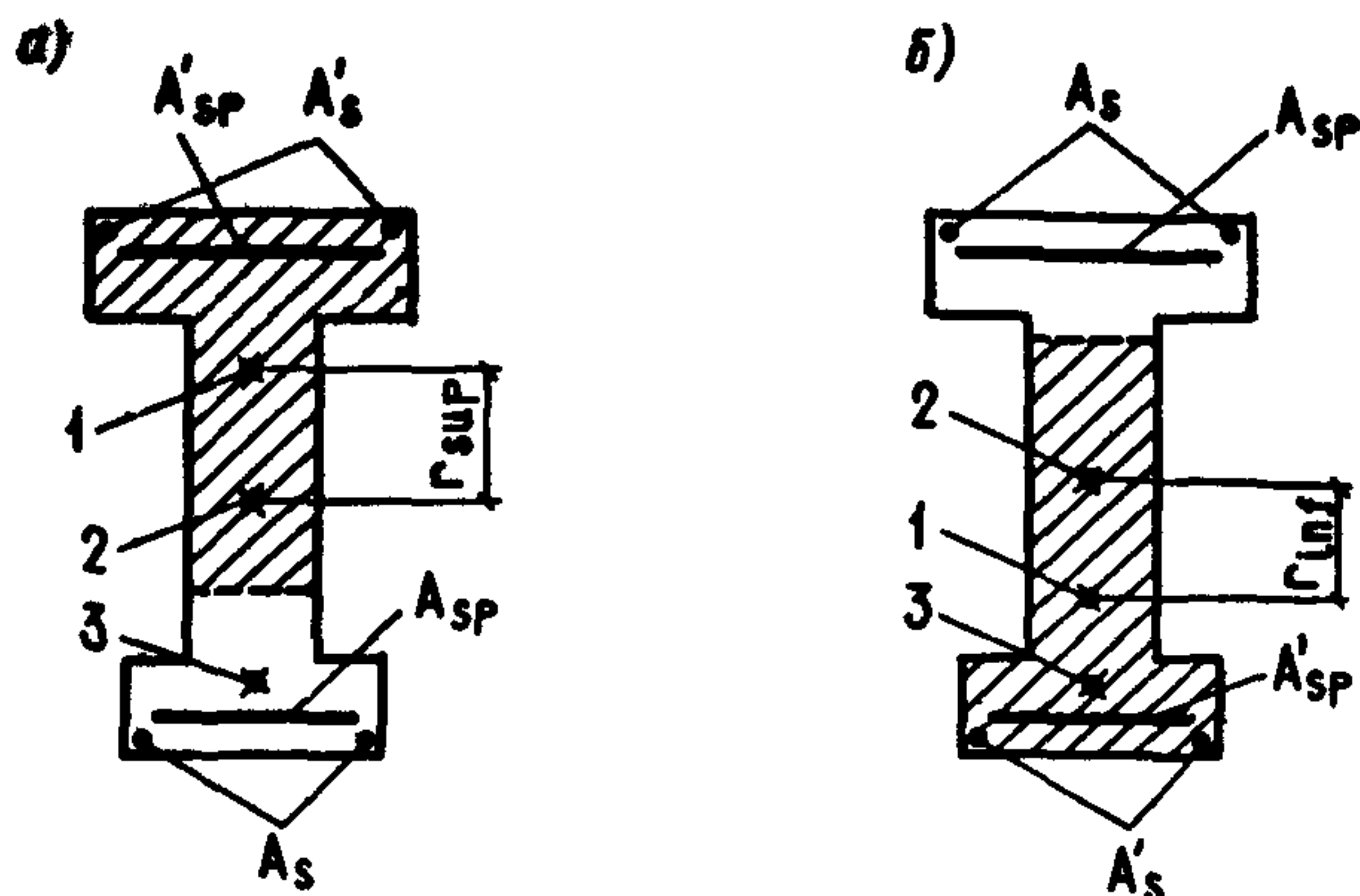
Черт. 39. Определение величин r_{sup} и r_{inf}
