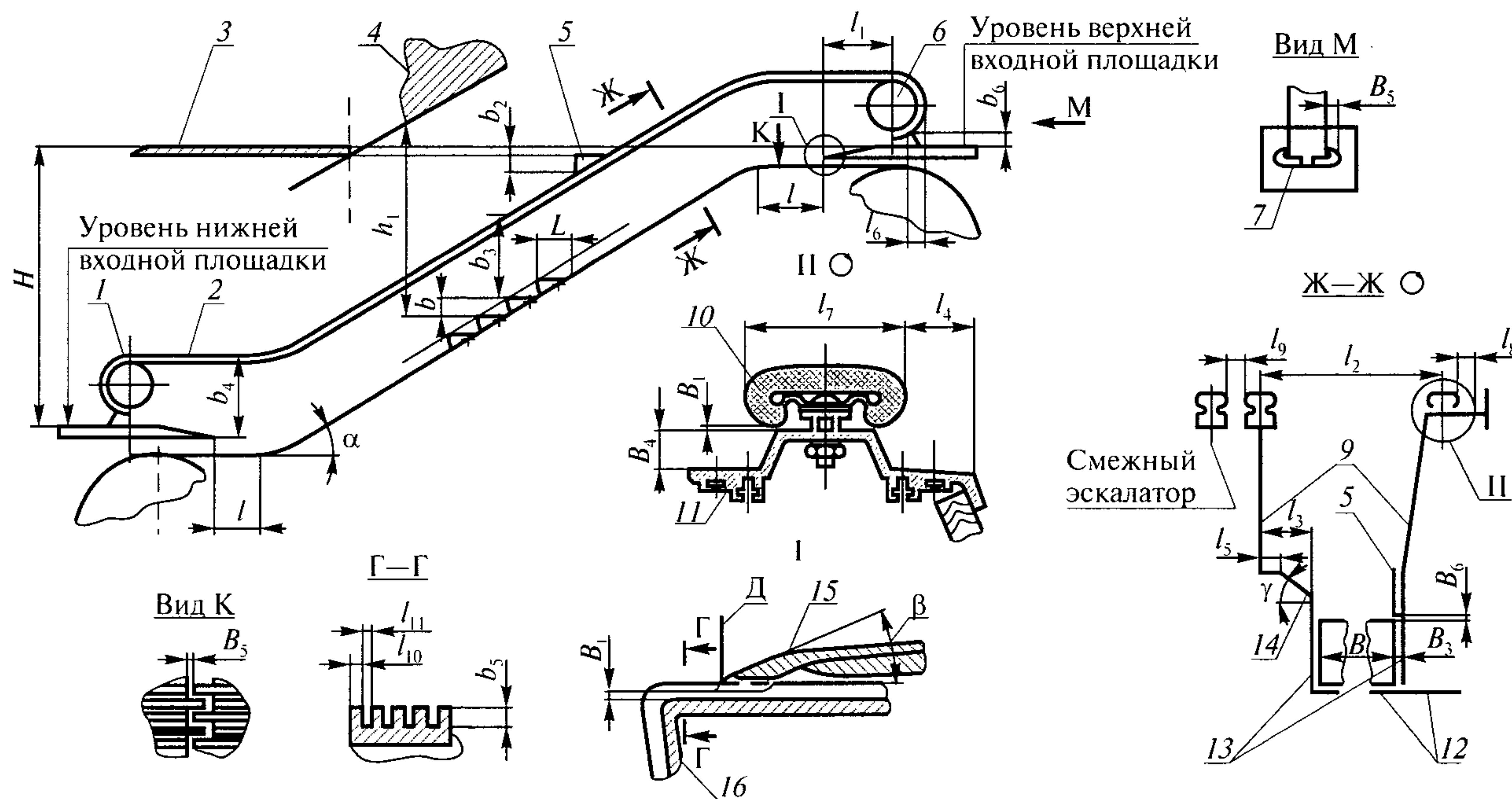
Рис. 1. Схема устройства эскалатора:
