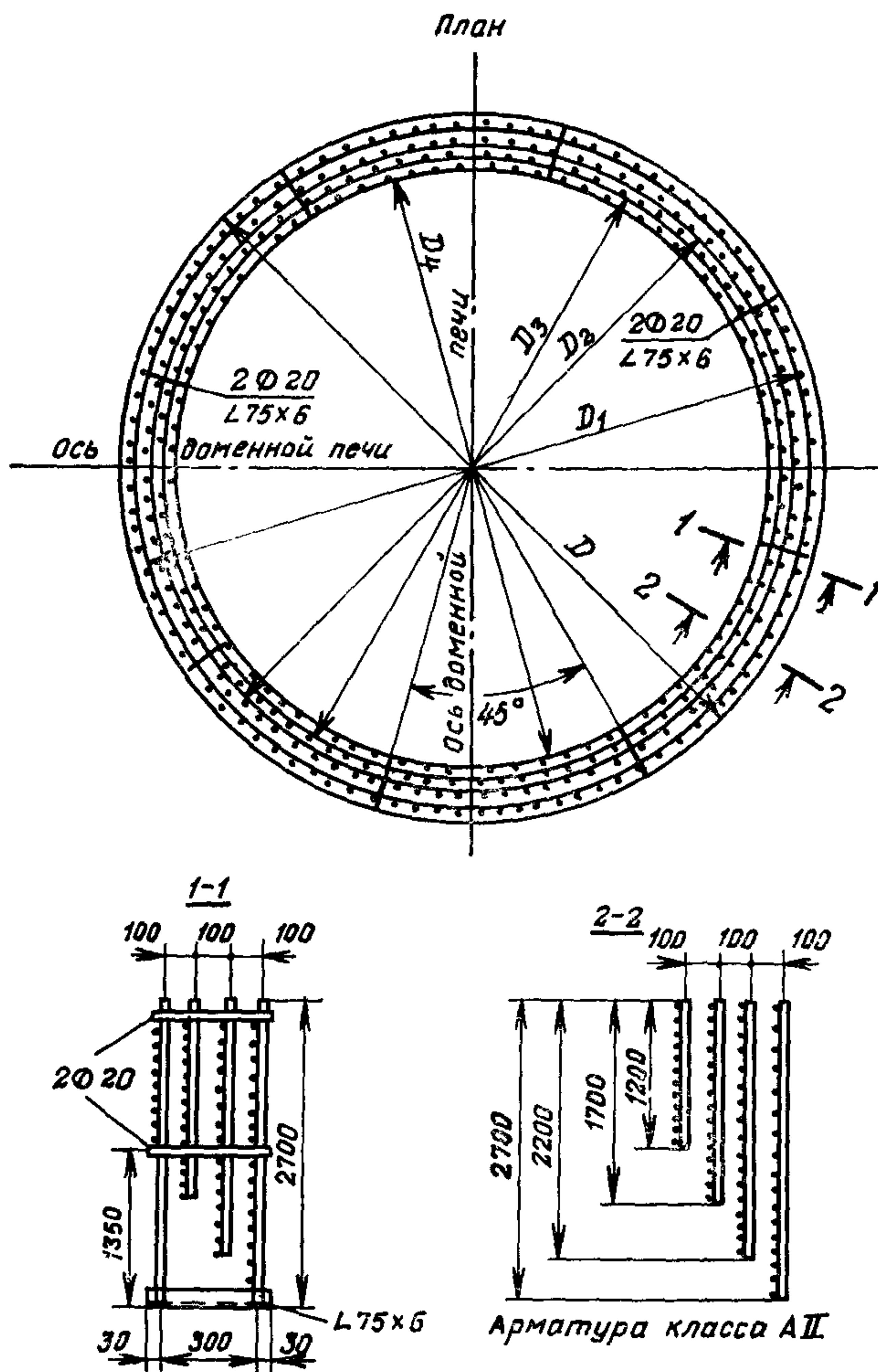
Рис. 9. Характер армирования жаростойкого массива
