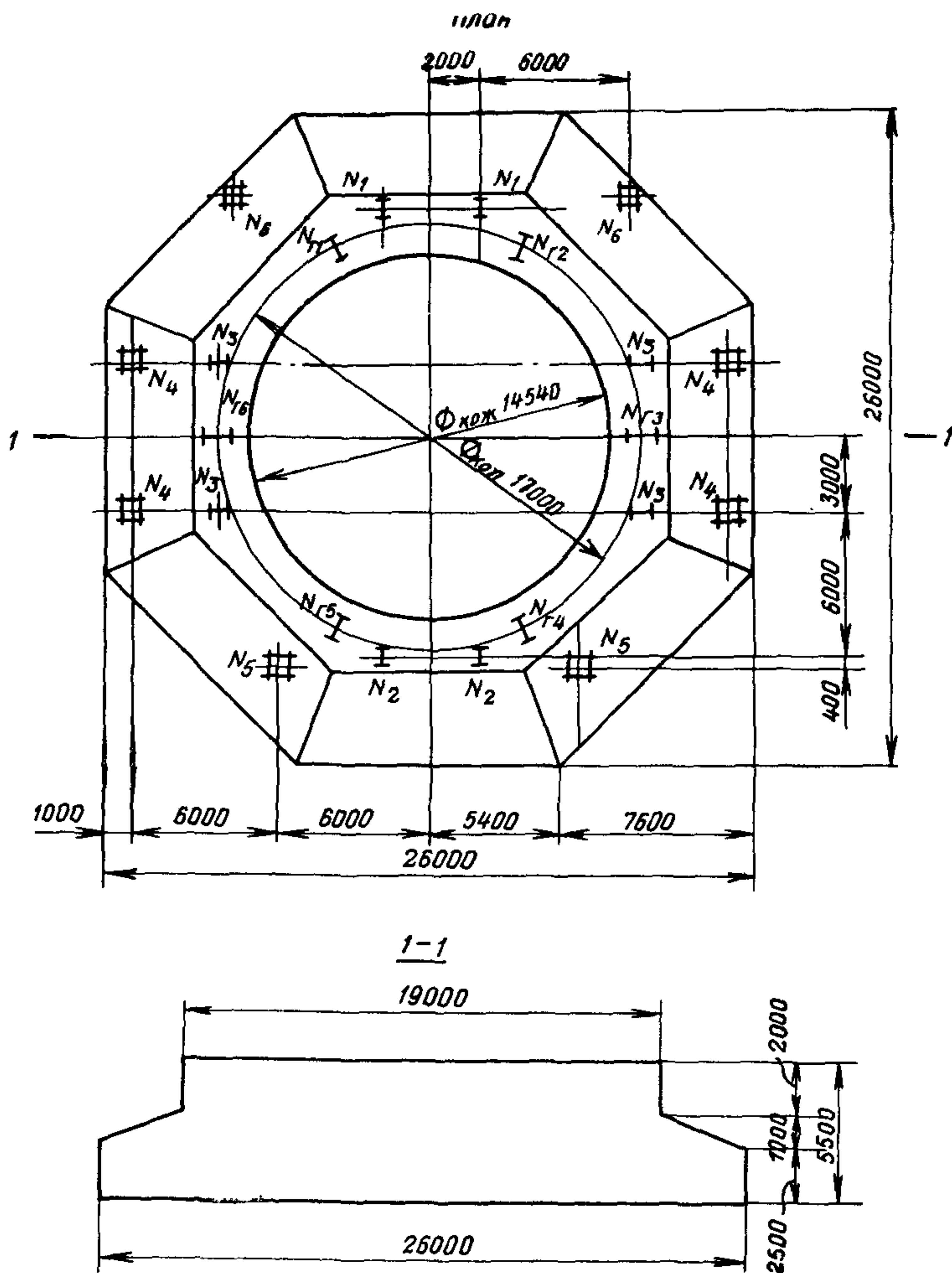
Рис. 11. Схема фундамента доменной печи
