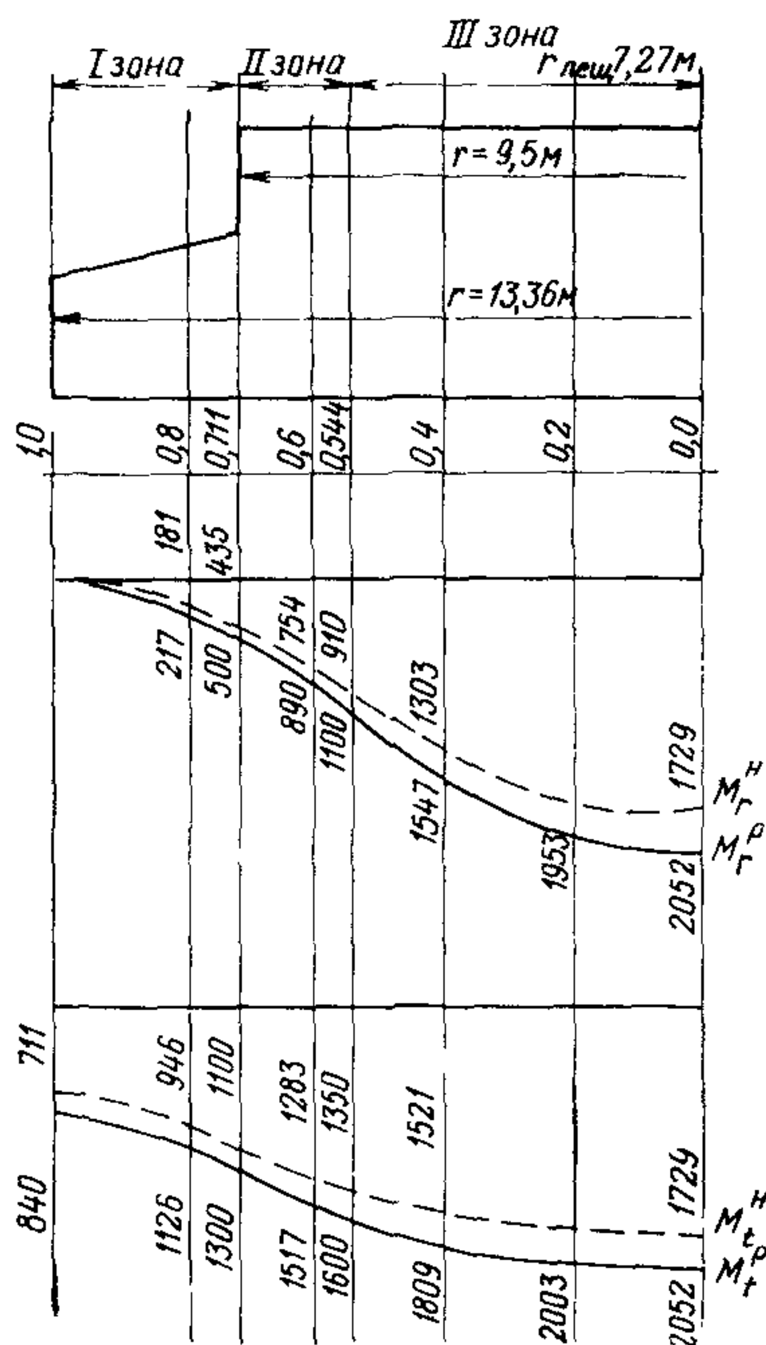
Рис. 13. Эпюры суммарных значений M_r и M_t , вычисленные по таблицам для абсолютно жесткой плиты
