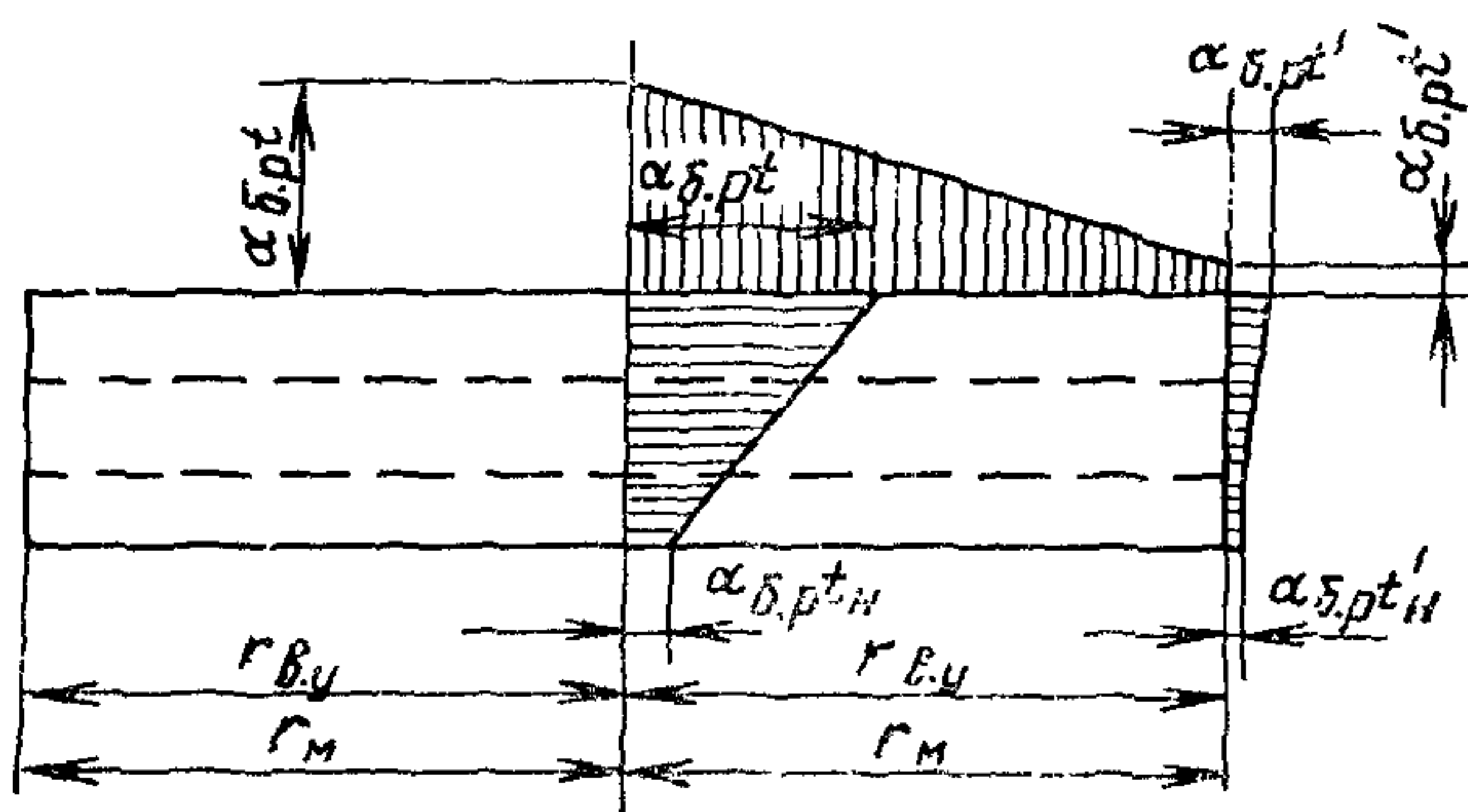
Рис. 1. Расчетная схема распределения свободных температурных деформаций по радиусу и высоте массива (плиты) фундамента
