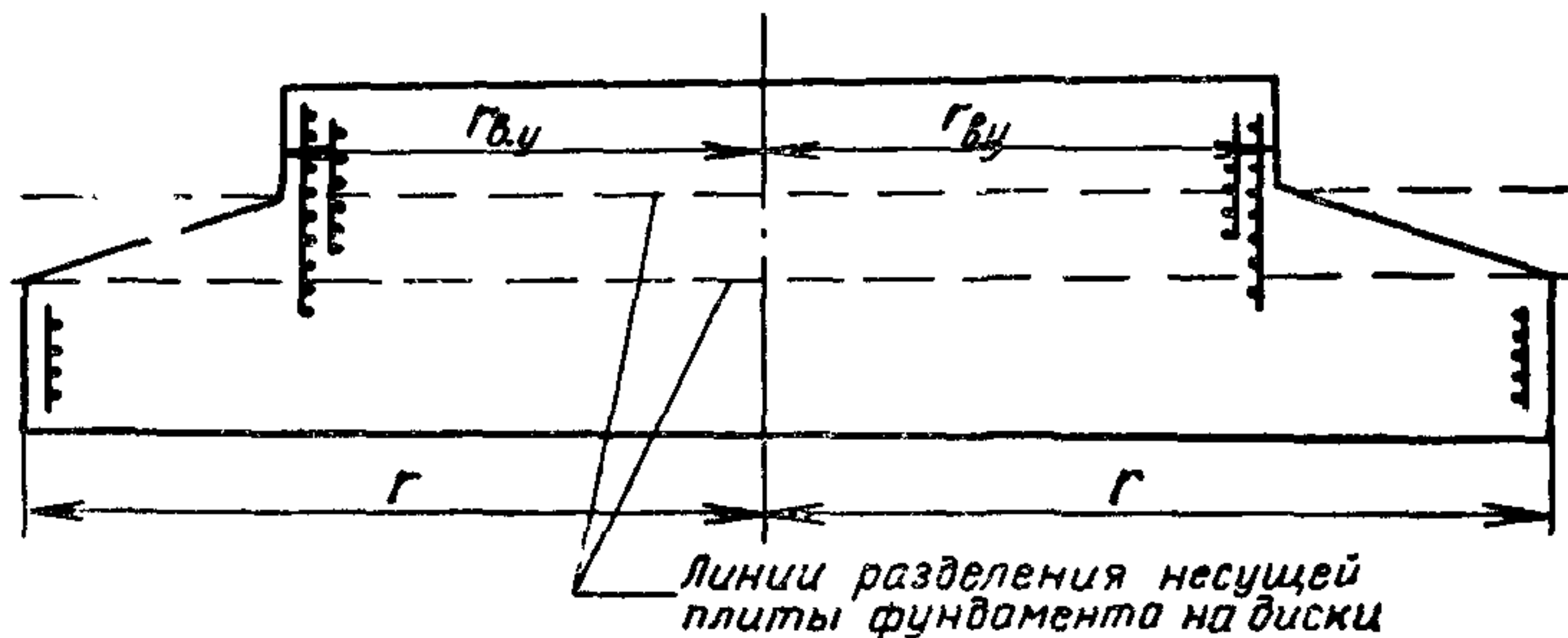
Рис. 2. Схема разделения несущей плиты на горизонтальные диски
