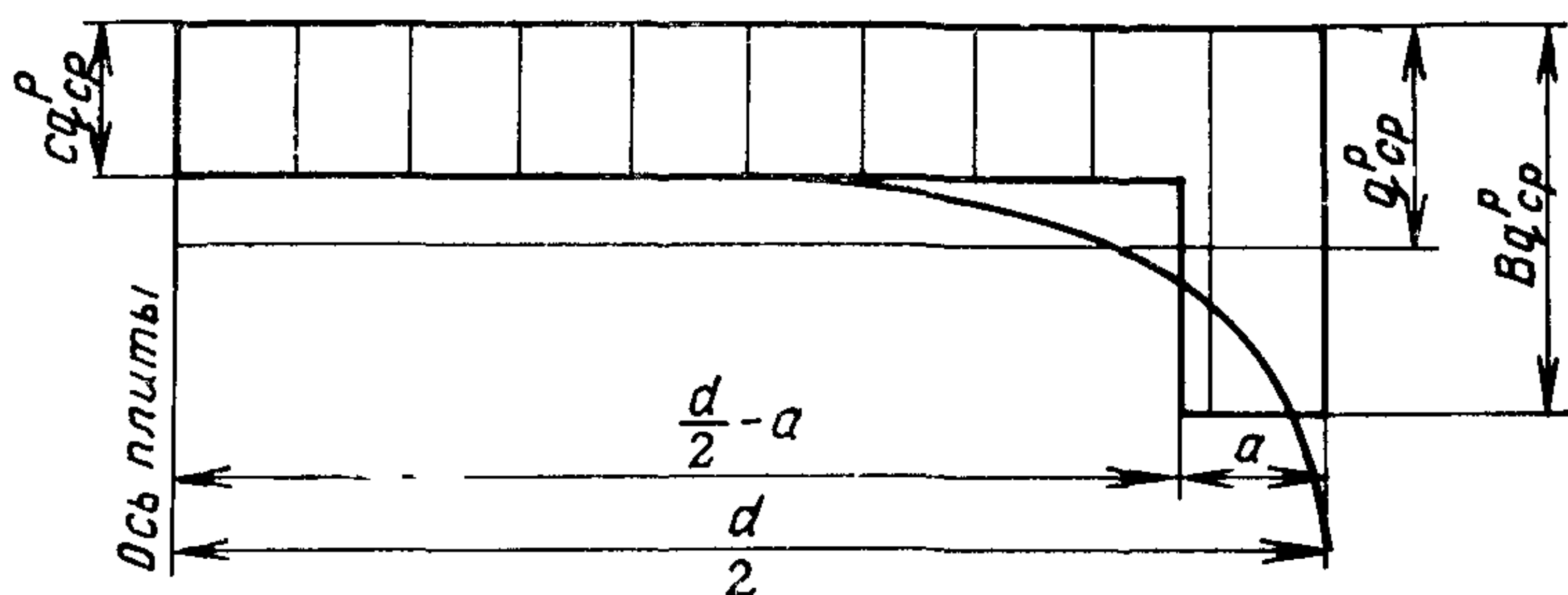
Рис. 4. Эюра реактивных давлений грунта при расчете фундаментных плит по методу предельного равновесия
