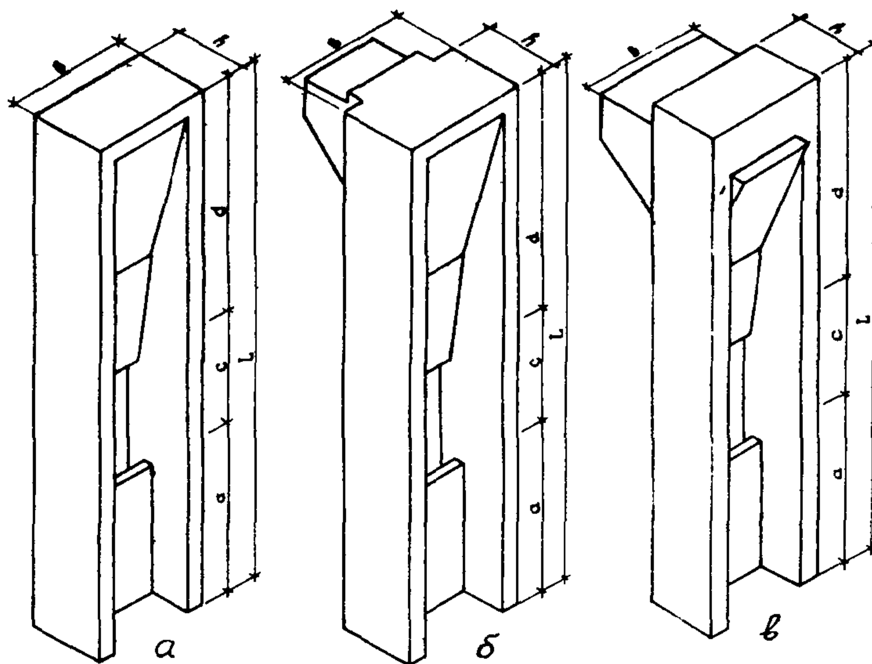
Рис. 2. Типы свай СВД а — без консоли; б, в — с консолями
