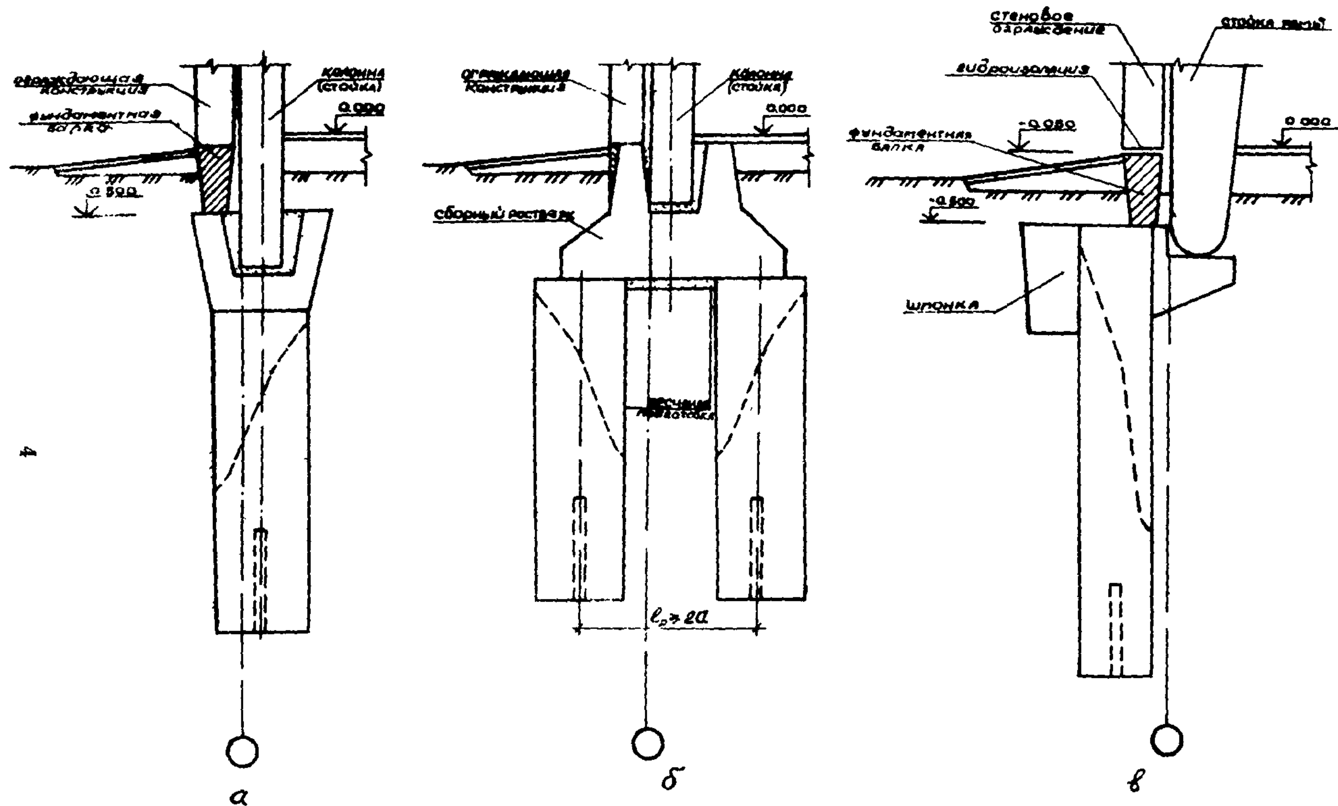
Рис. I. Узлы опирания на свайные фундаменты а - опирание колонн на одну сваю; б - опирание колонны на ростверк по двум сваям; в - опирание стойки рамы на консоль сваи
